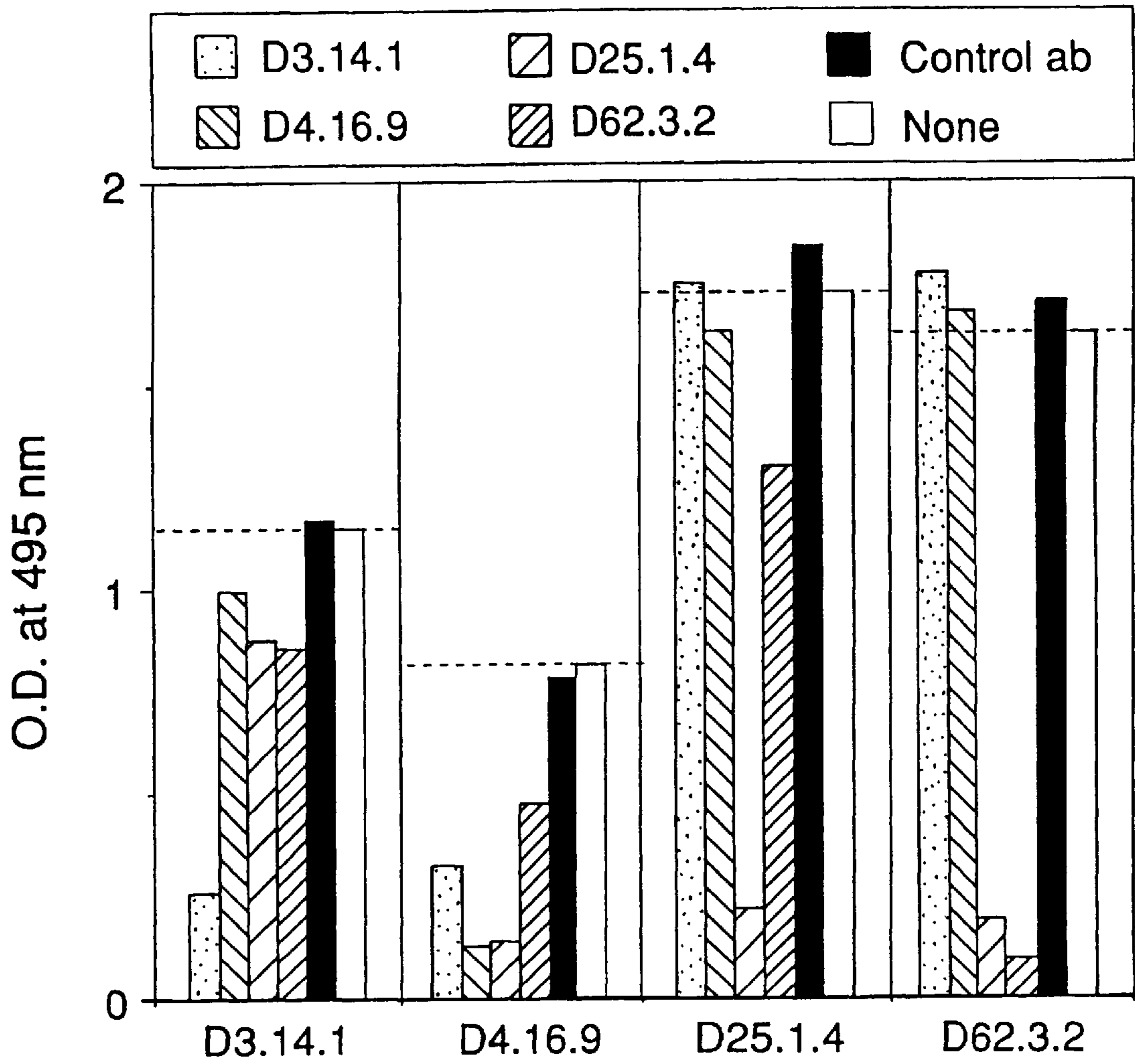
HRP-mAbs FIG. 3
