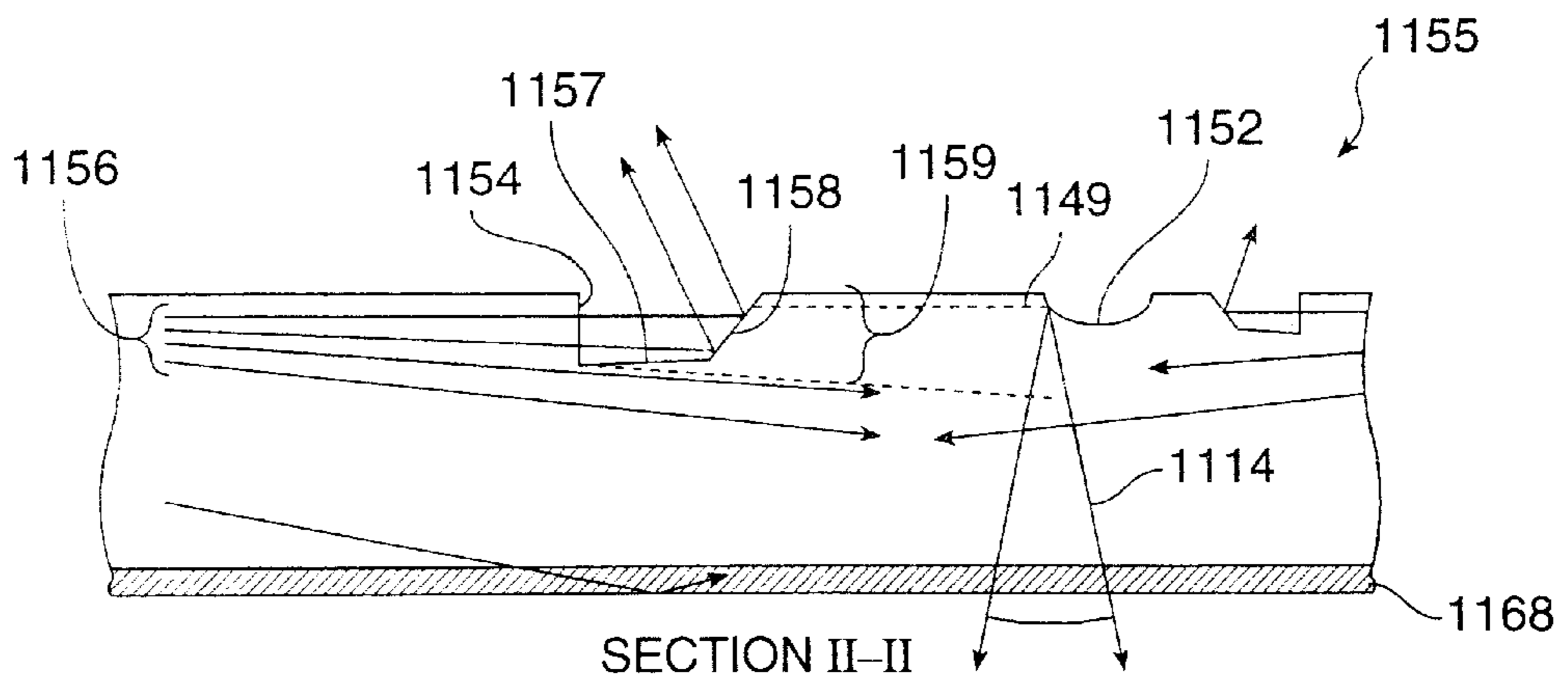
SECTION II-II FIG. 69
