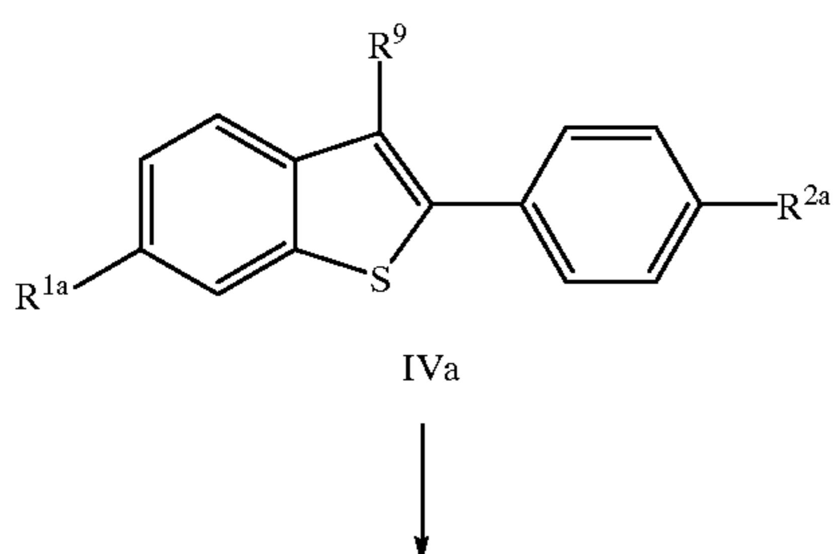
Scheme VI
