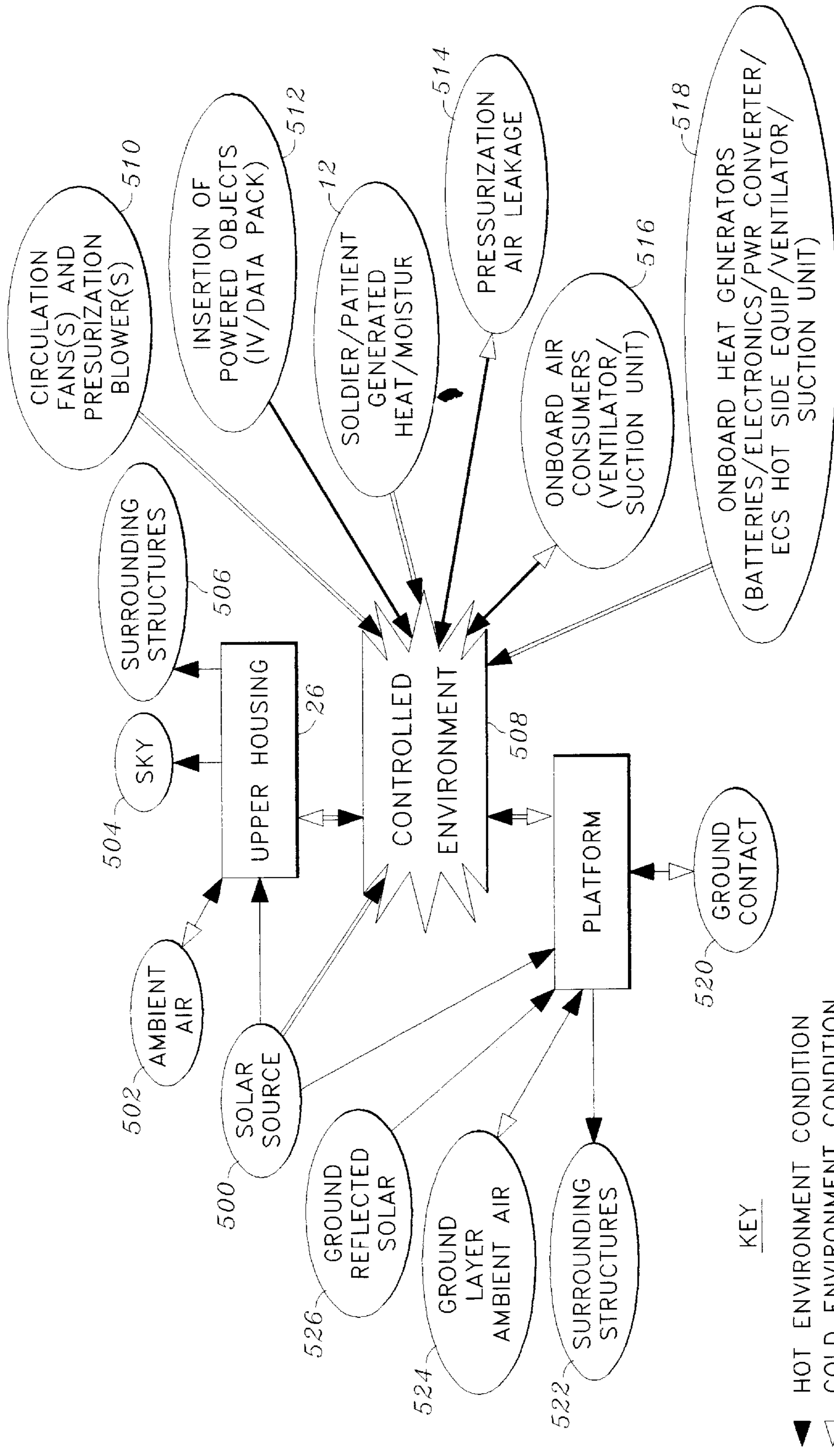
FIG. 28
