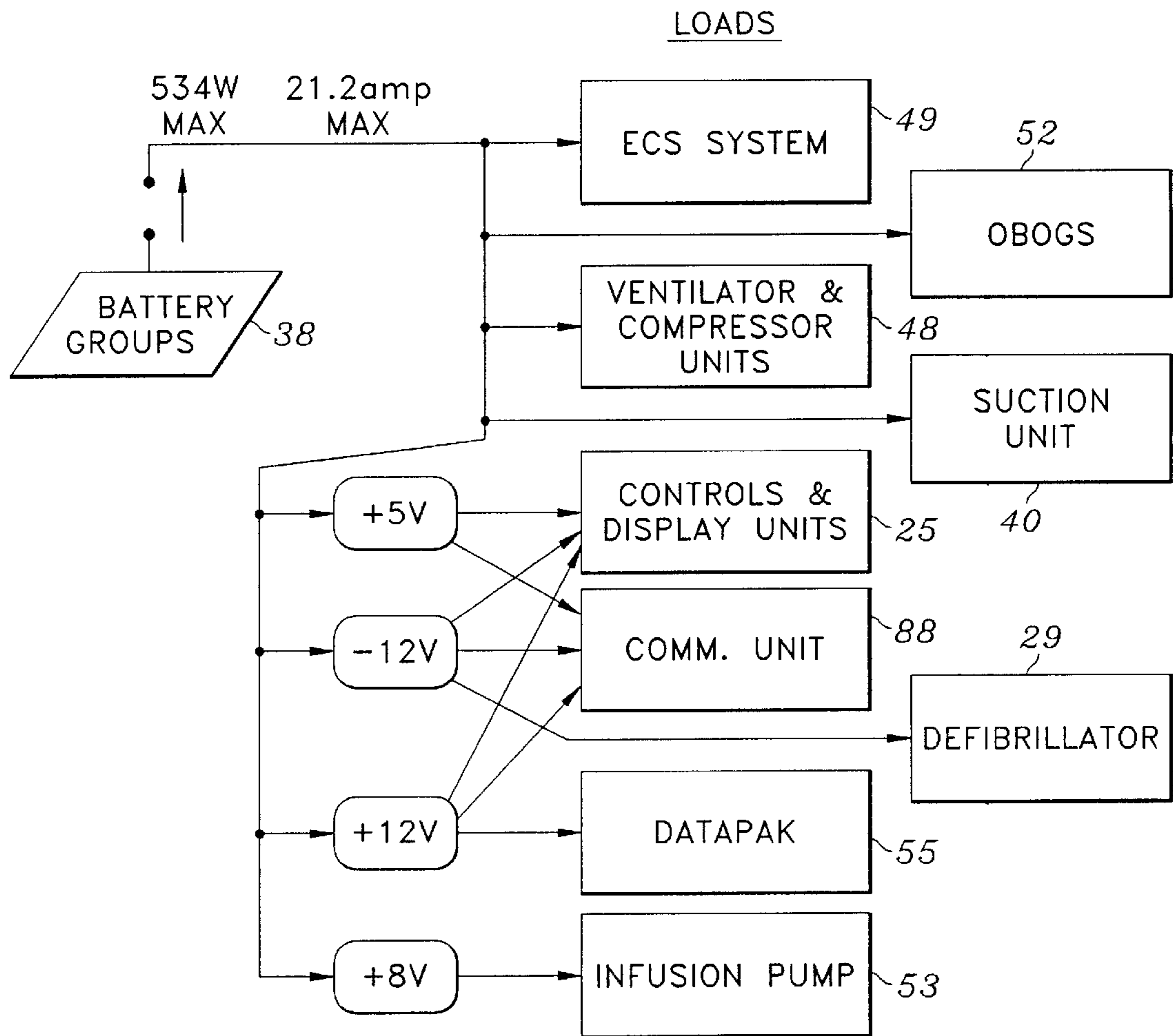
FIG. 16
