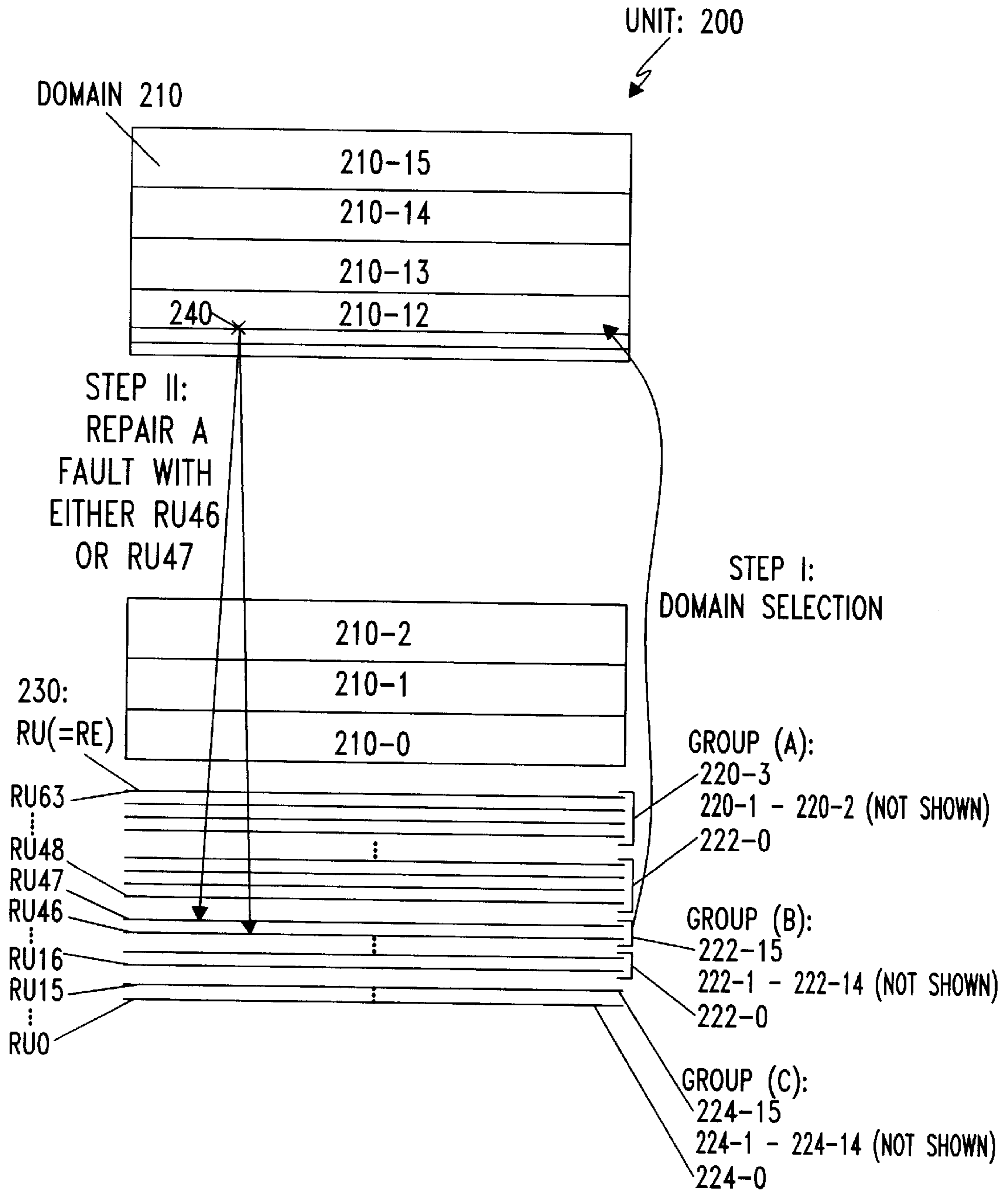
FIG. 2b
