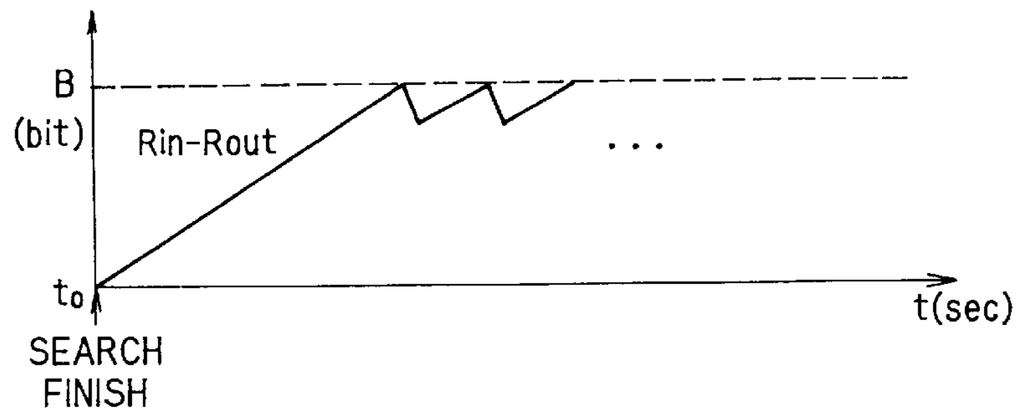
FIG. 13A
