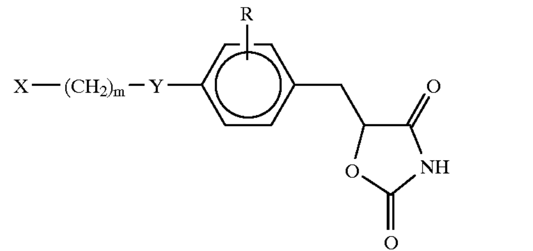
(I-4)
