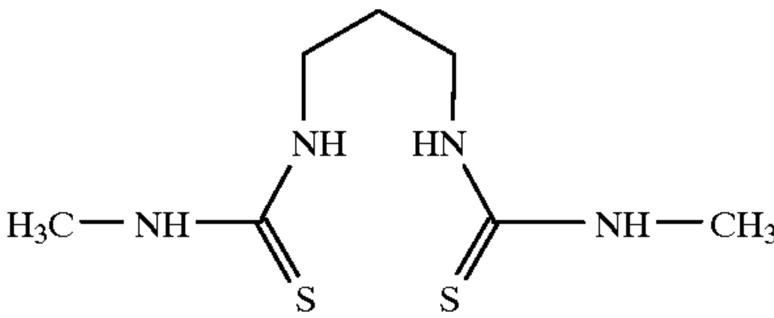
DTU-CH 3
