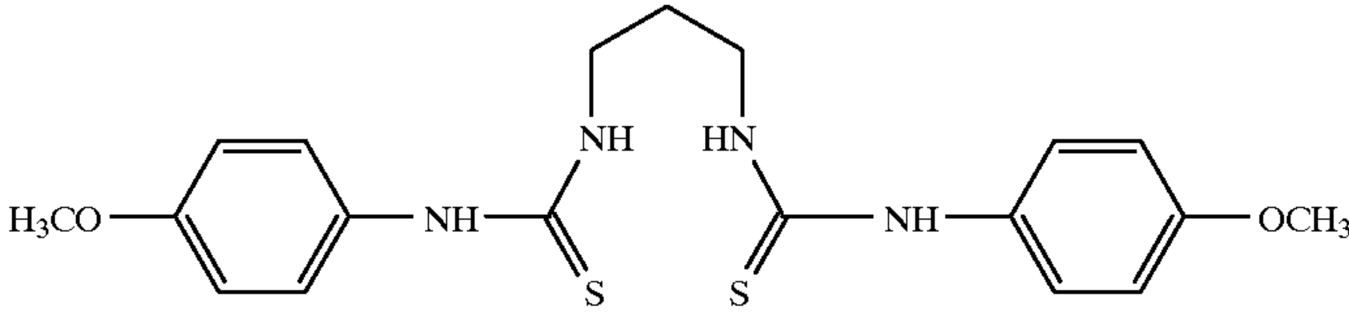
DTU-PhOCH
