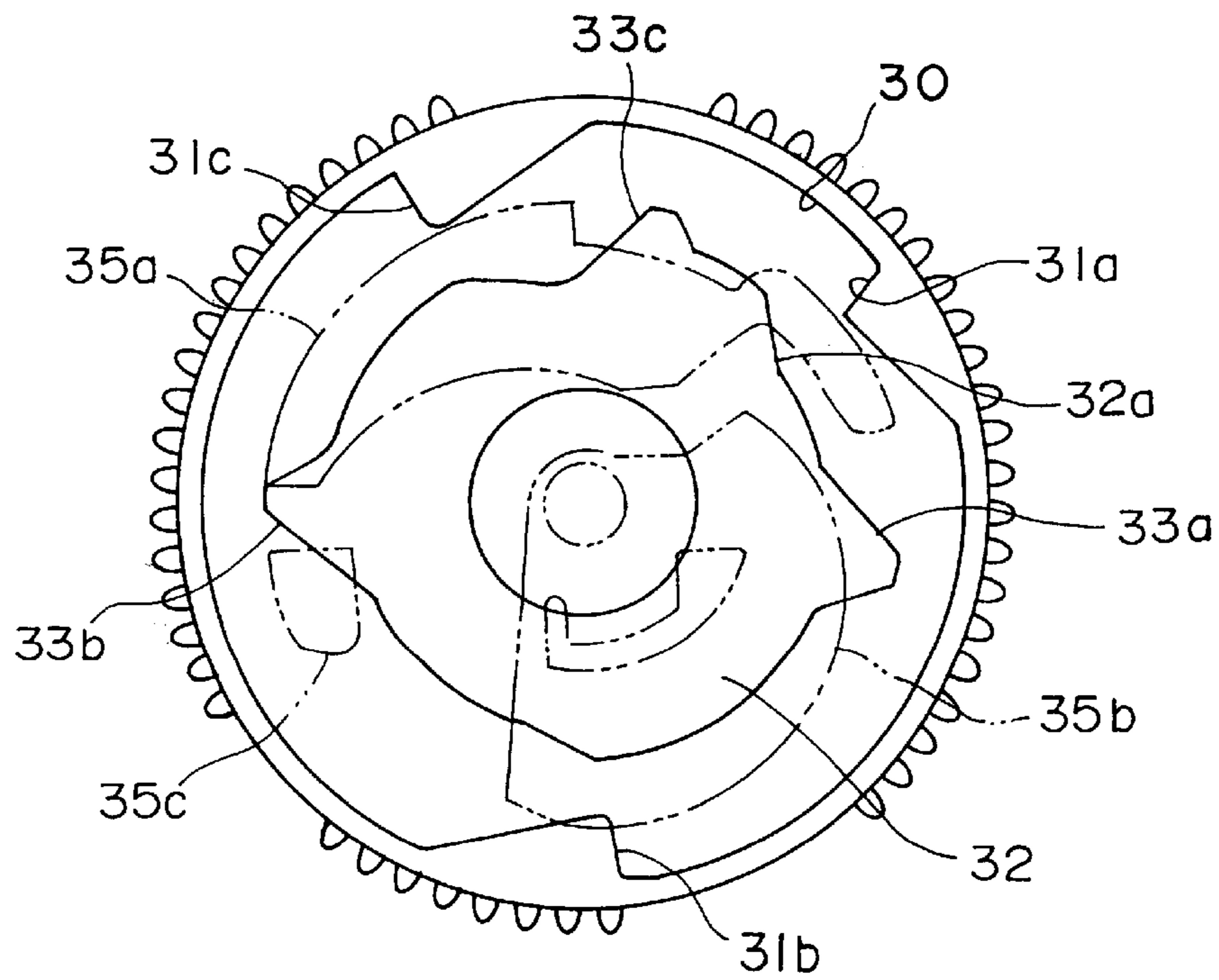
FIG. 8
