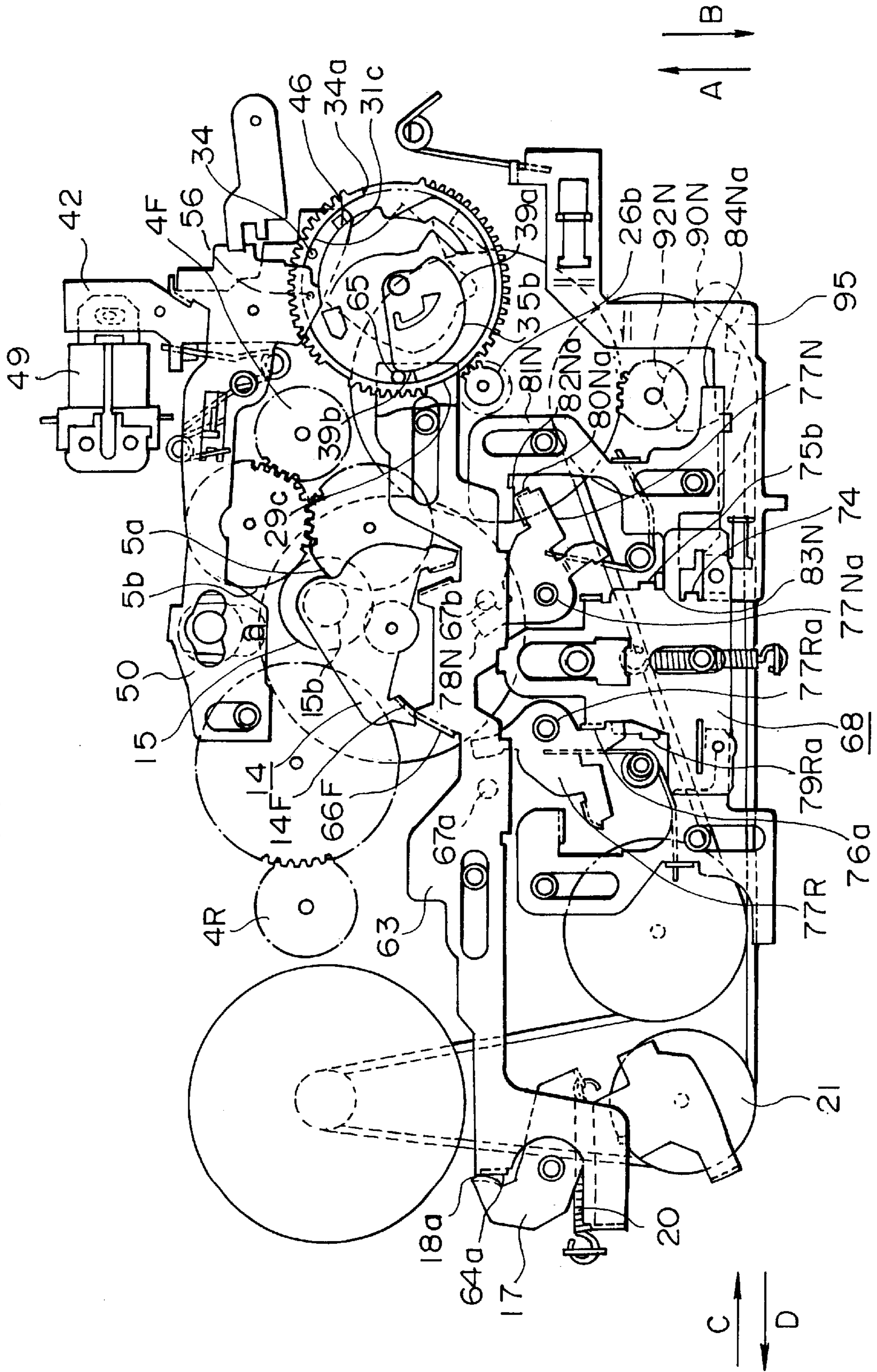
FIG. 13
