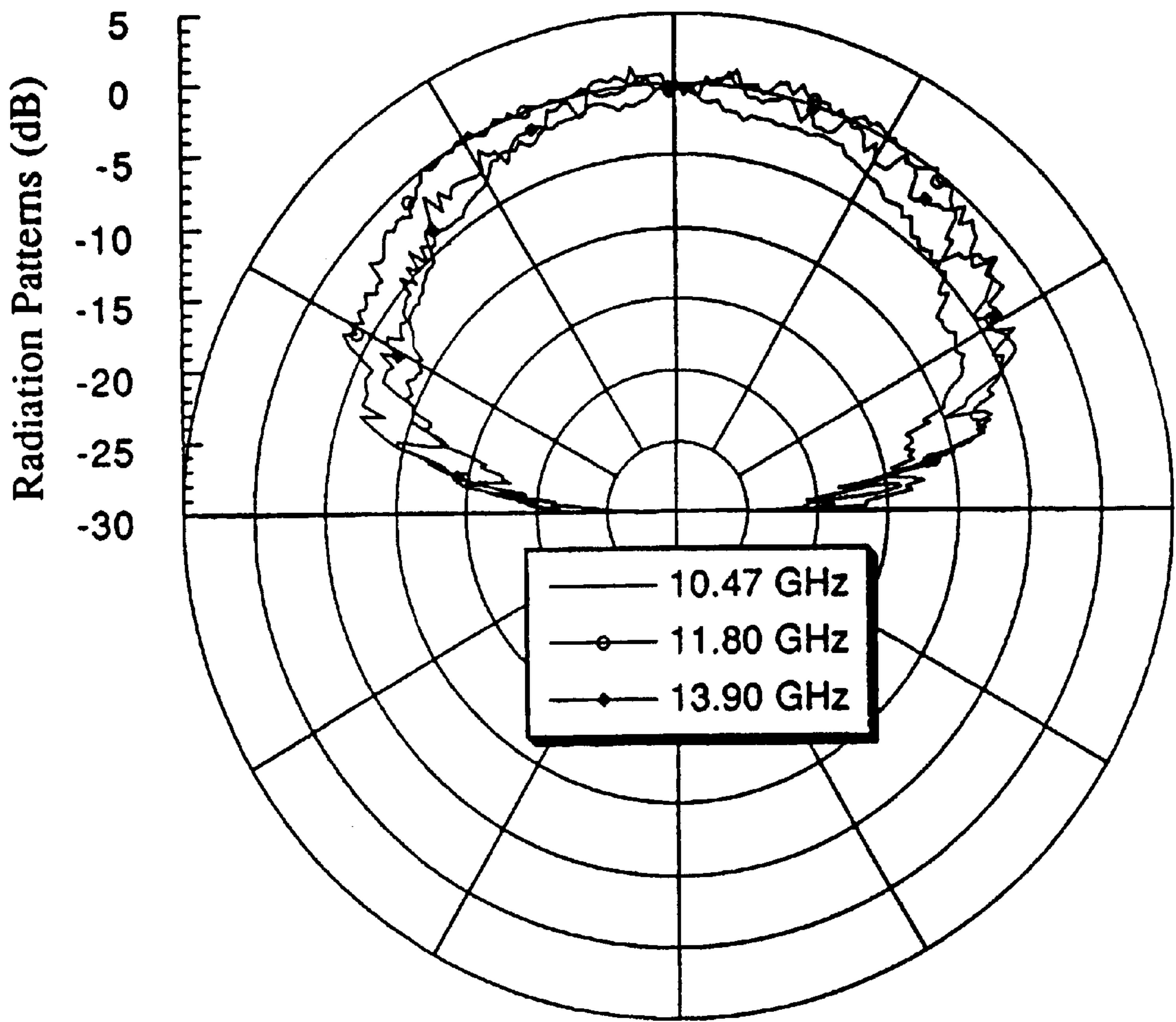
Figure 4a) H-Plane Pattern
