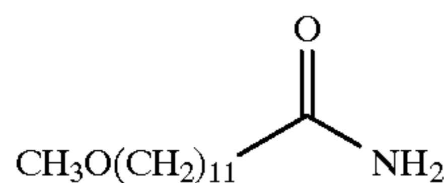
12-Methoxydodecanamide
