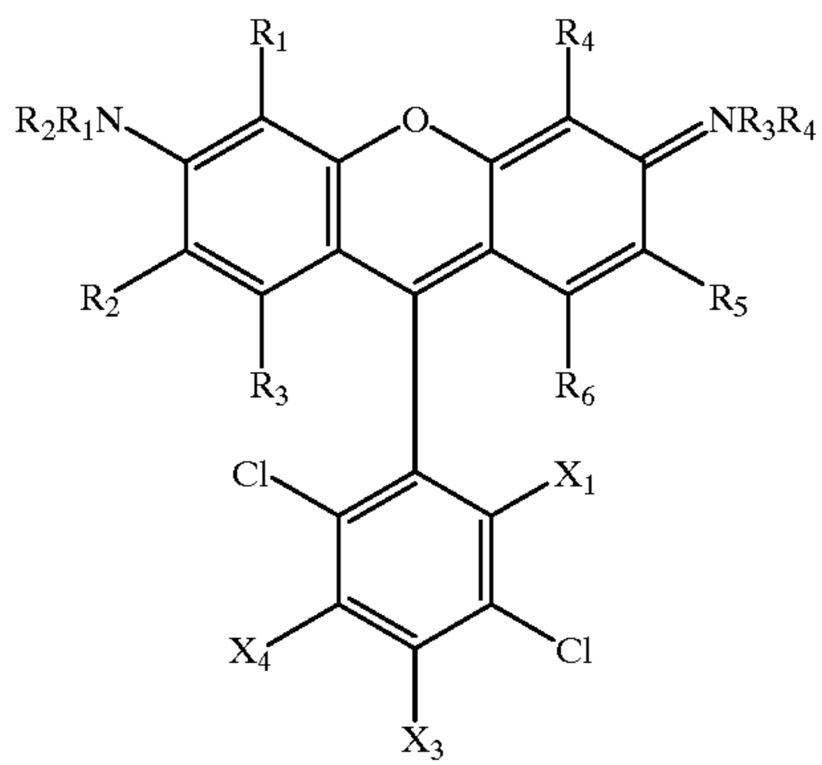
4,7 Dichlororhodamine
