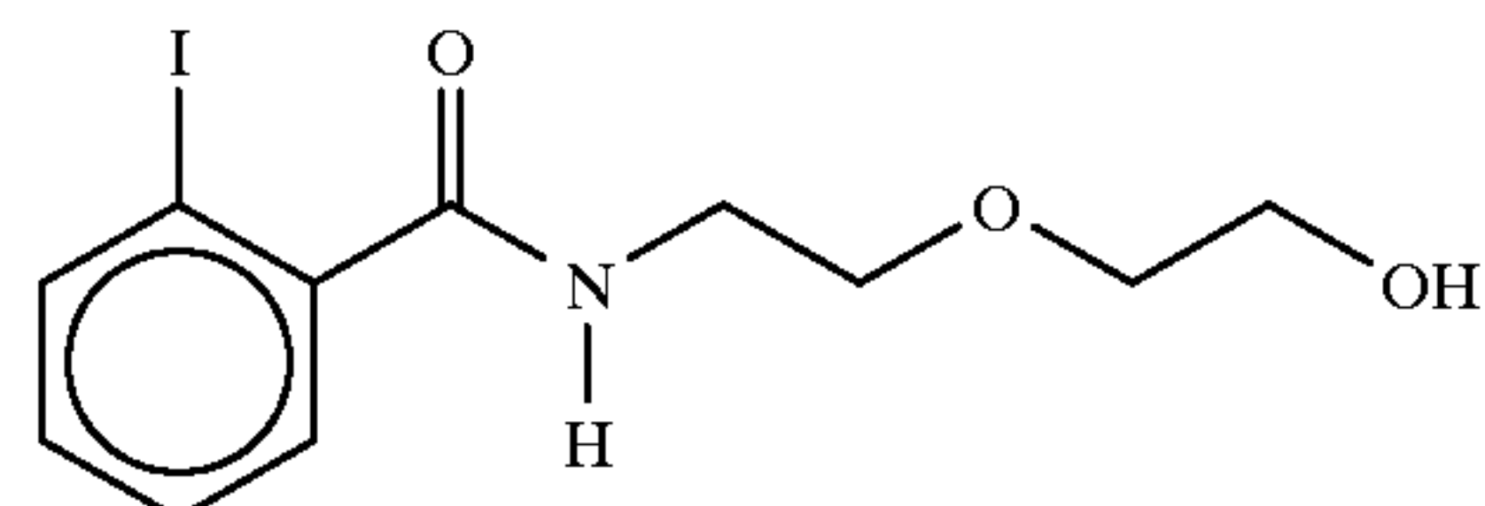
2-[N-(2-iodobenzoyl)aminoethoxy]ethanol
