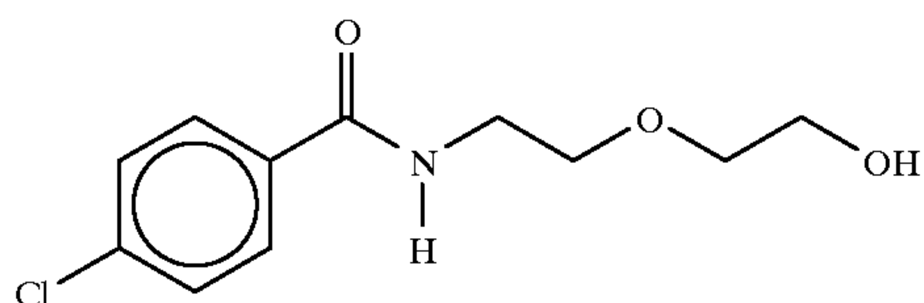
2-[2-N-(4-chlorobenzoyl)aminoethoxy]ethanol
