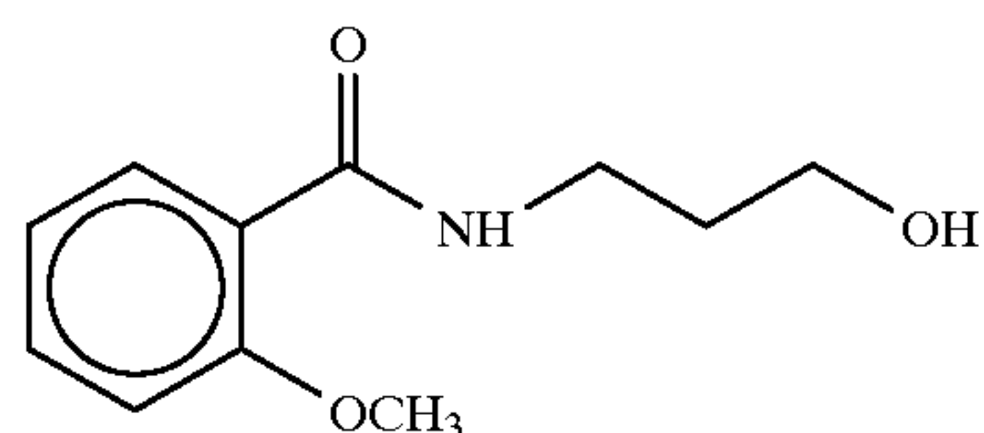
3-(2-methoxybenzoylamino)-1-propanol
