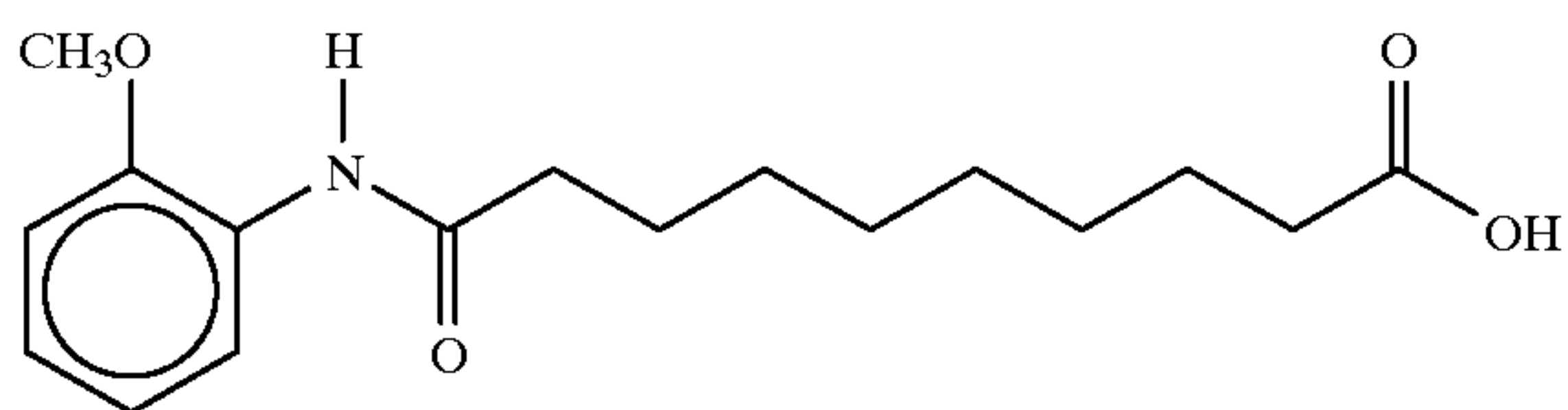
10-(N-2-Methoxyanilino)sebacic acid
