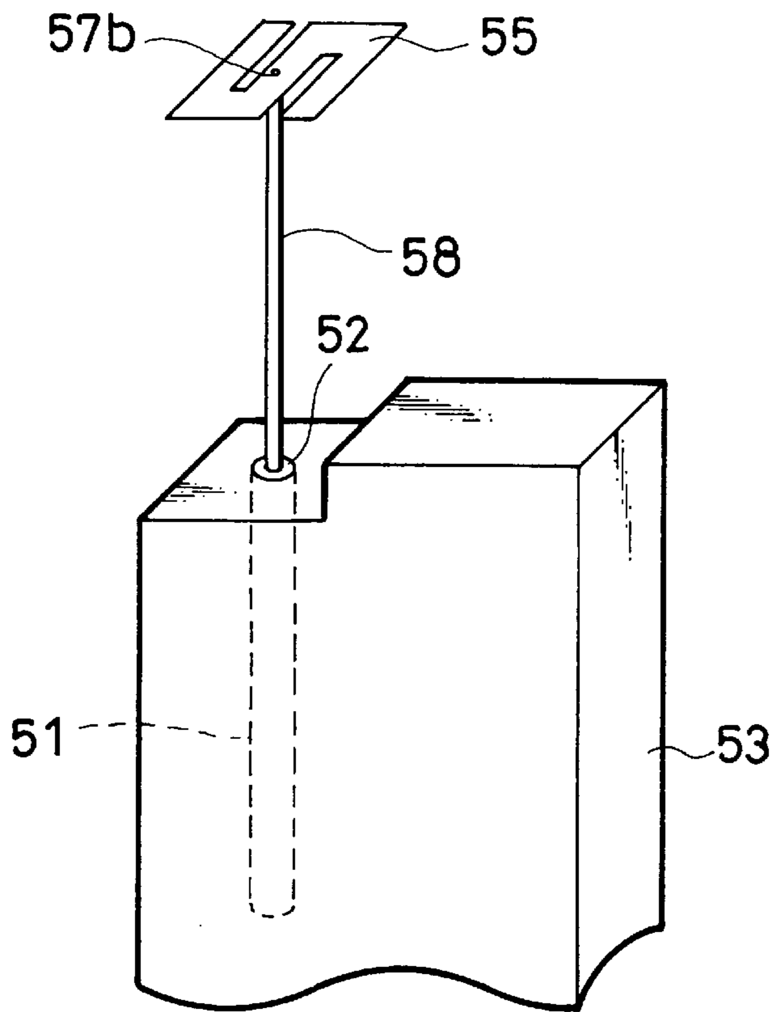
FIG. 30B
