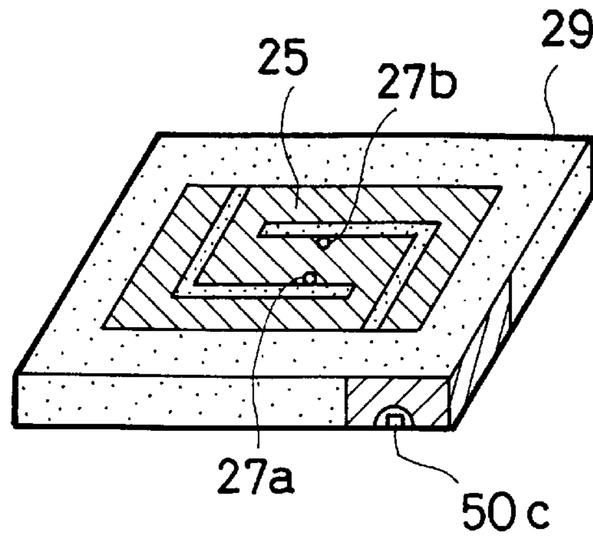
FIG. 27B
