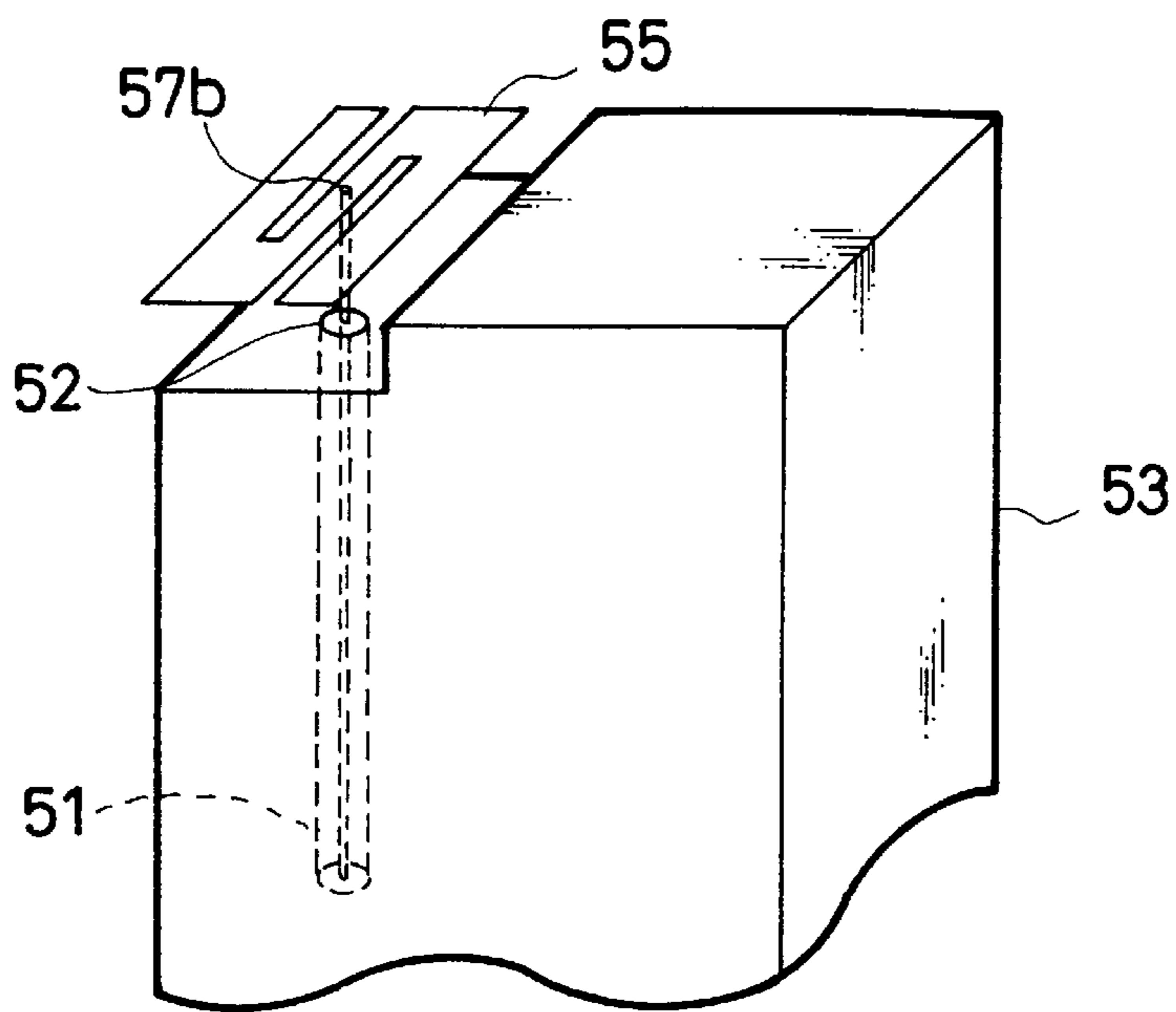
FIG. 30A
