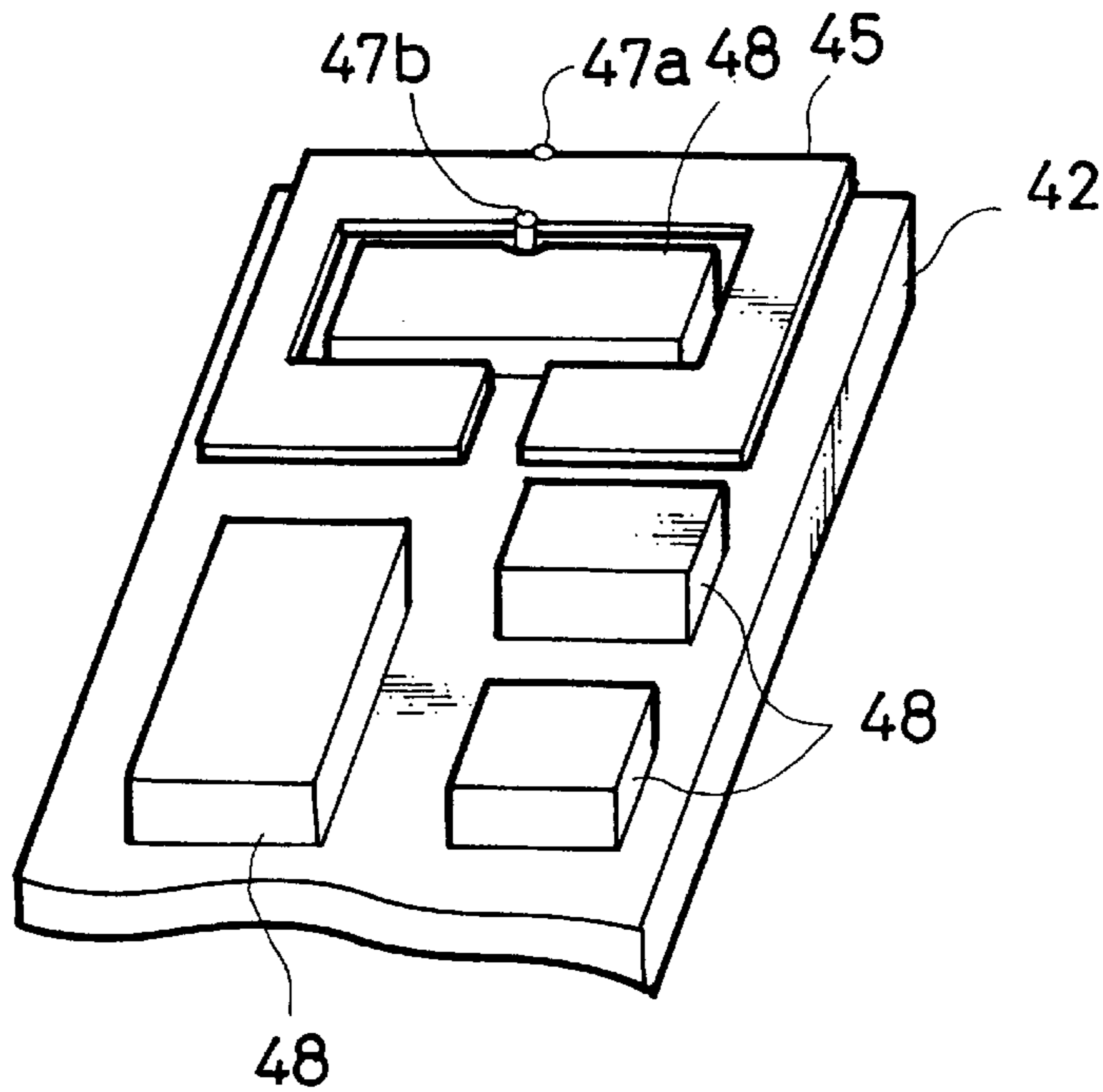
FIG. 29B
