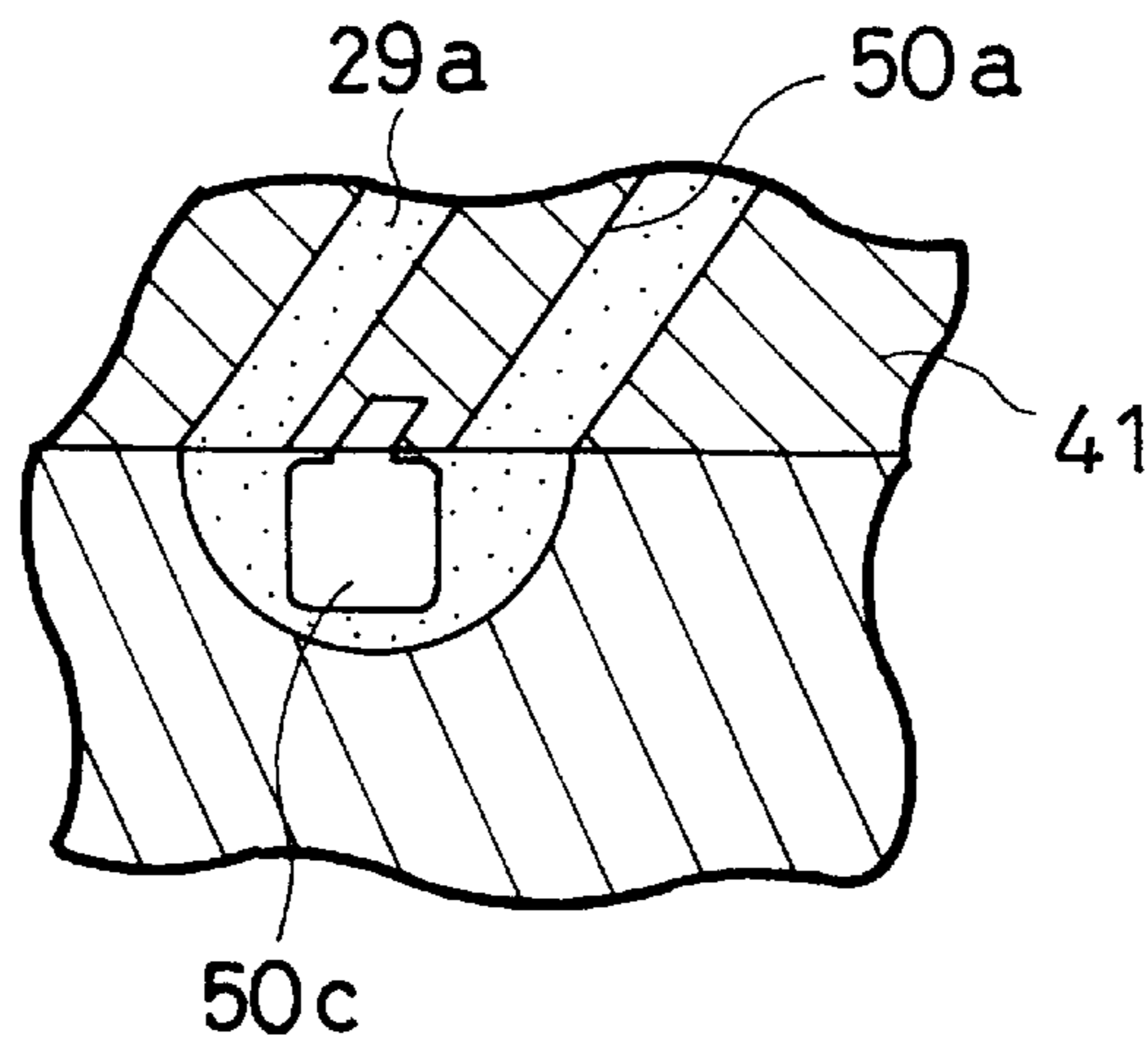
FIG. 27C
