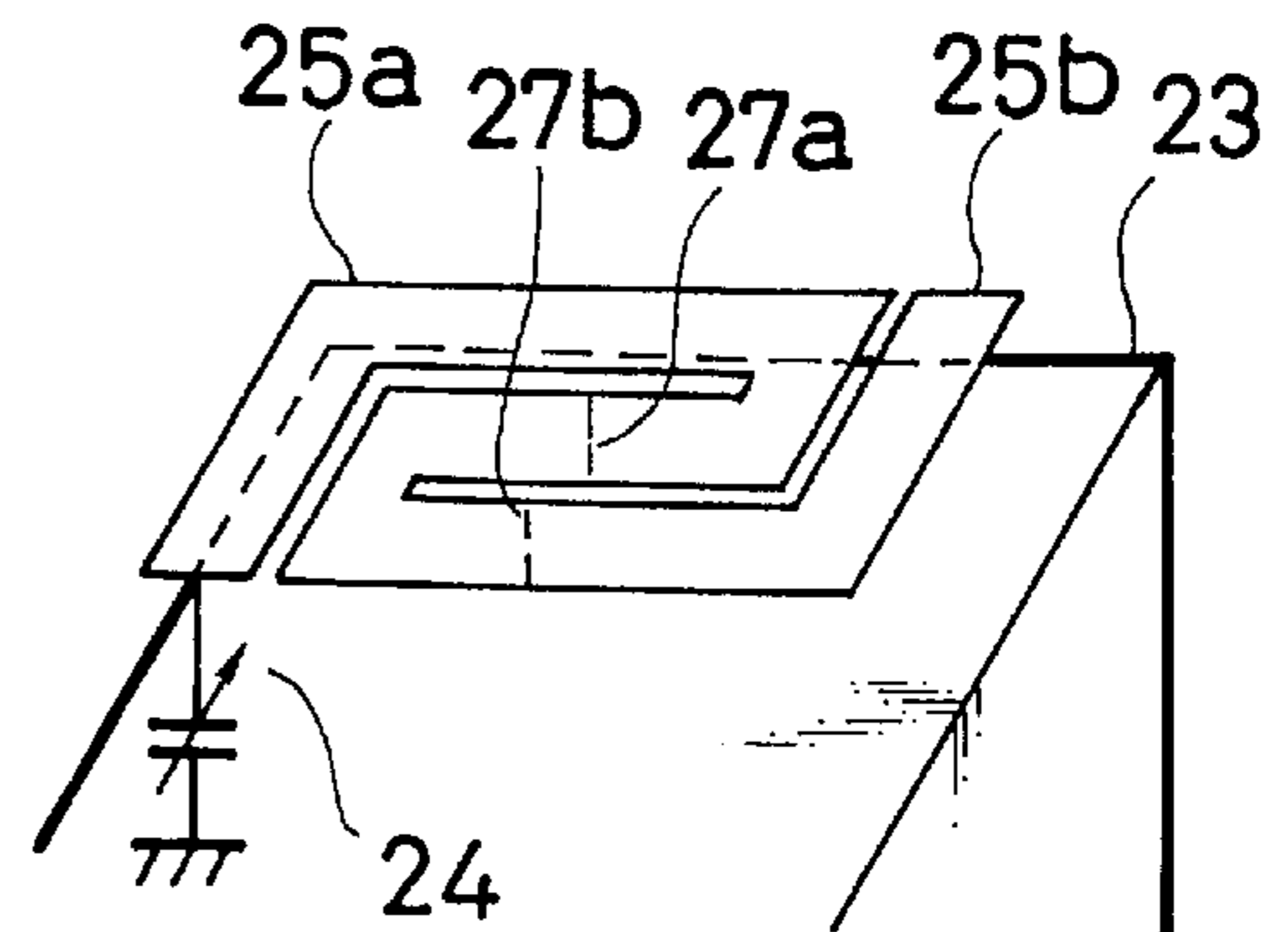
FIG. 17E
