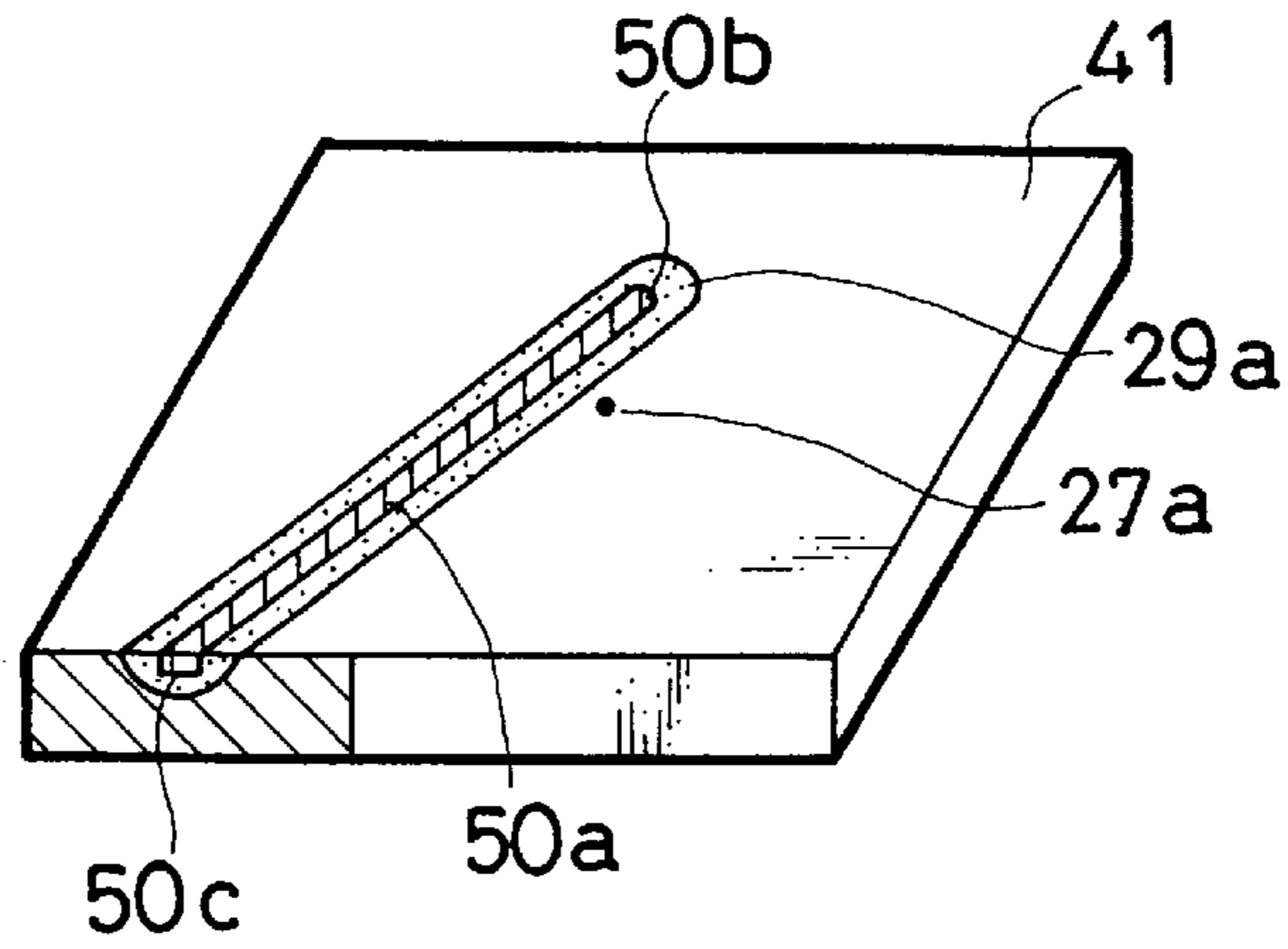
FIG. 27B
