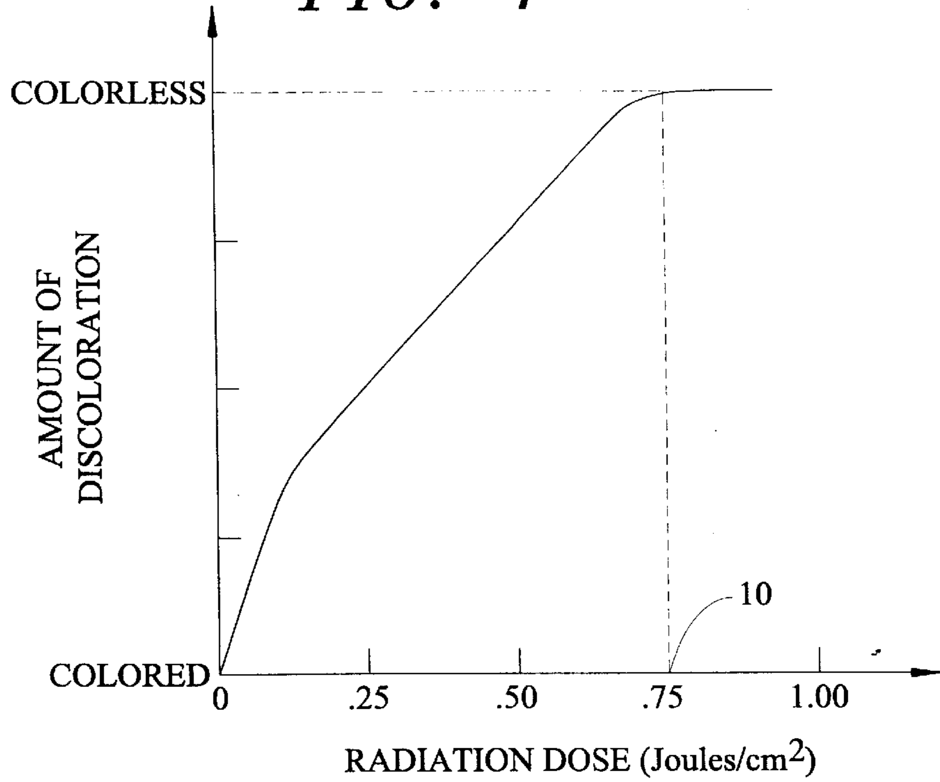
FIG. 4
