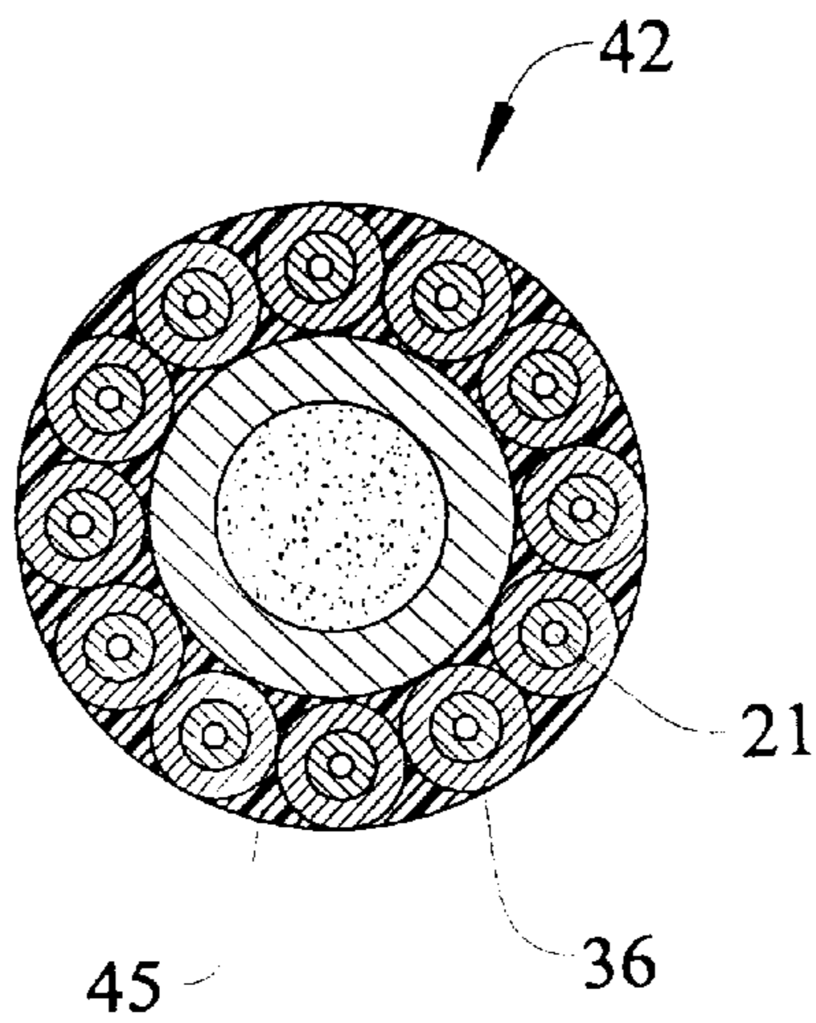
FIG. 11
