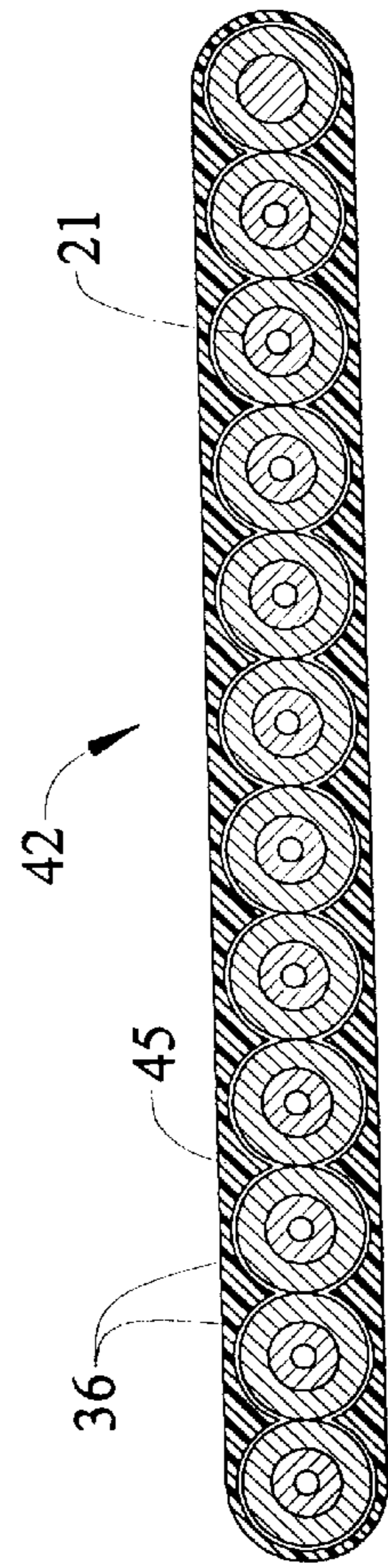
FIG. 7
