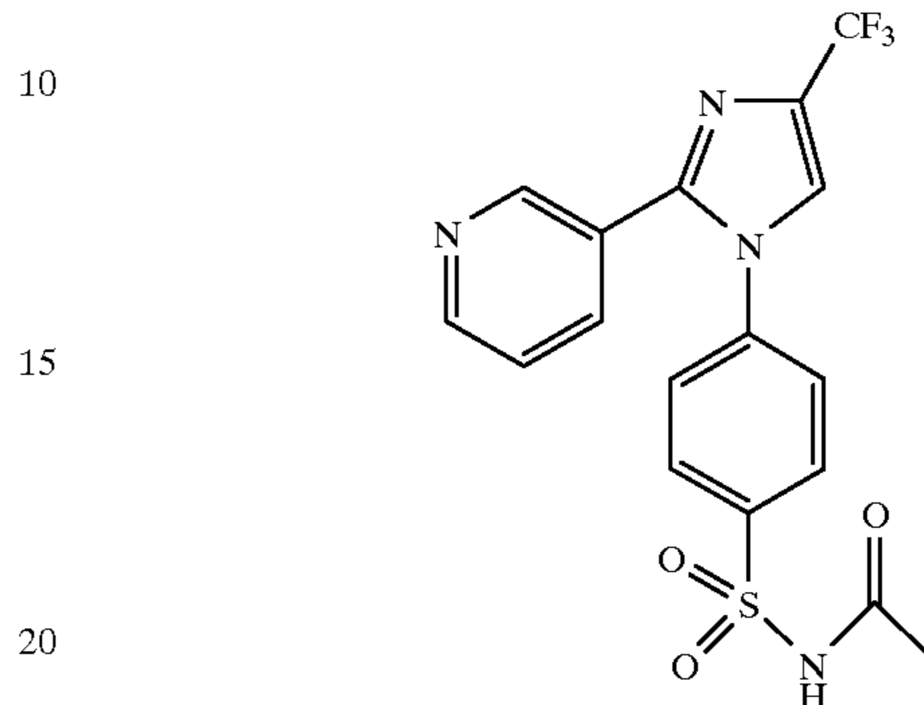
N-[[4-[2-(3-Pyridinyl)-4-(trifluoromethyl)-1H-imidazol-1-yl]phenyl]sulfonyl]acetamide
