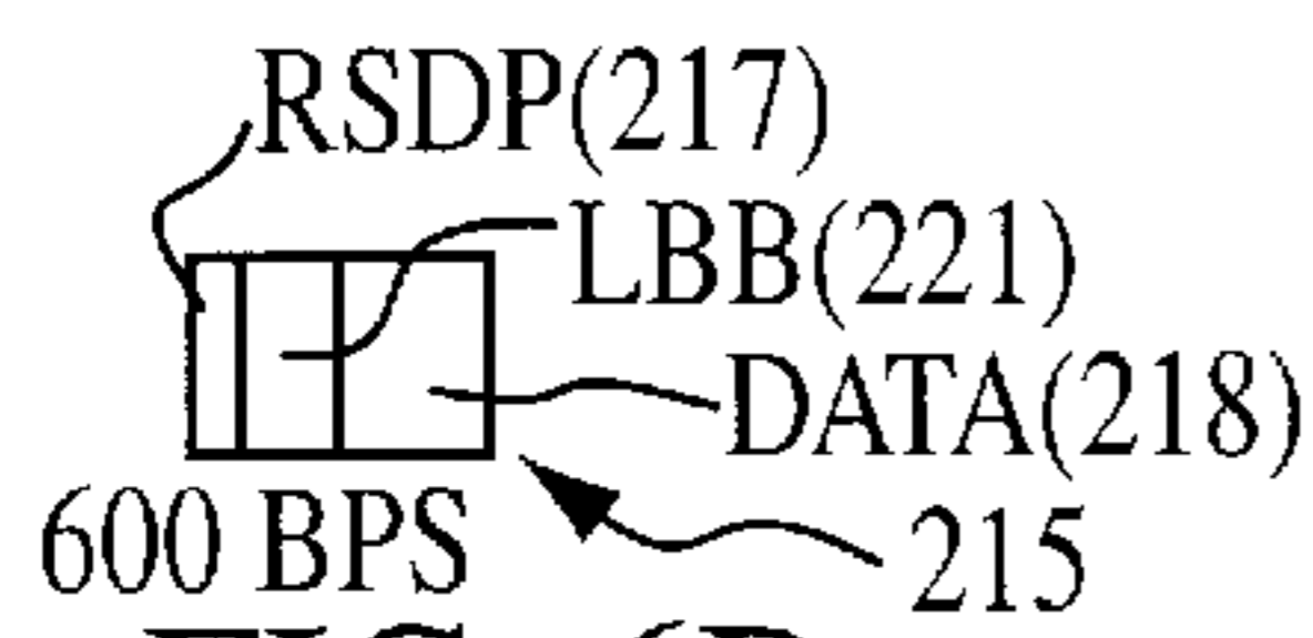
FIG. 6B FRAME TYPE A
