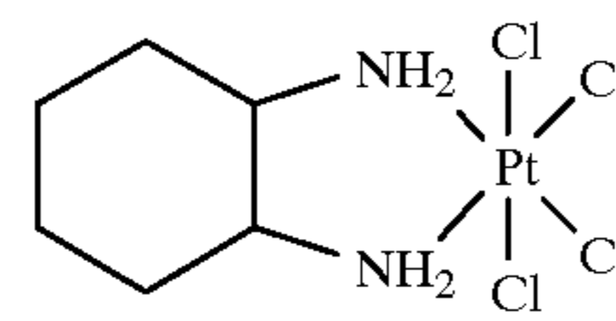
Tetraplatin (Ormaplatin)
