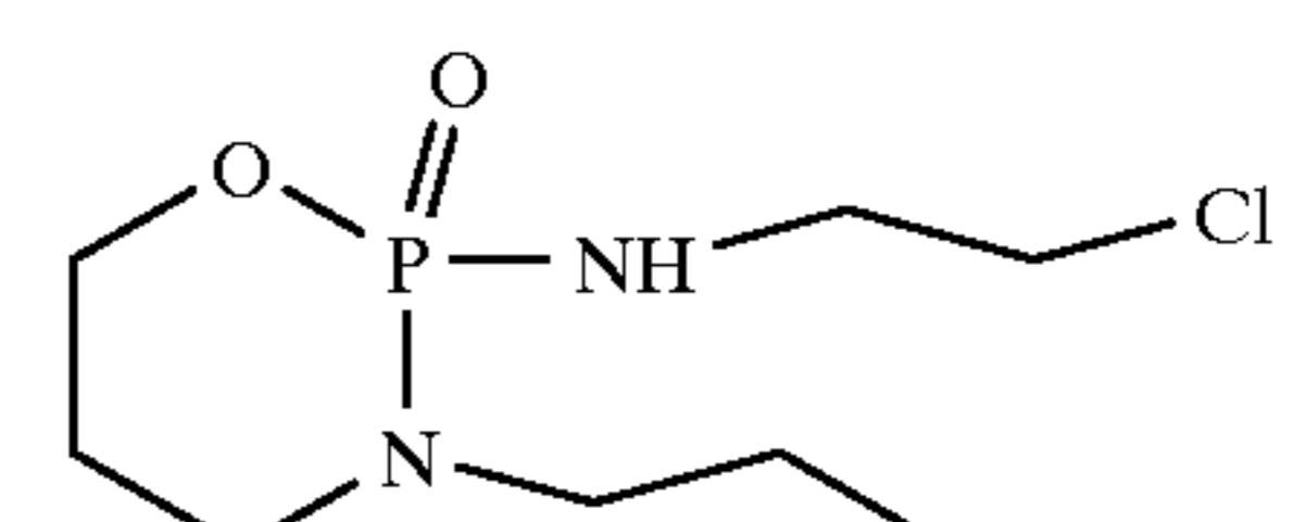
Ifosfamide
