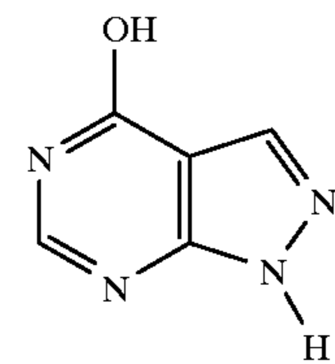
Allopurinol
