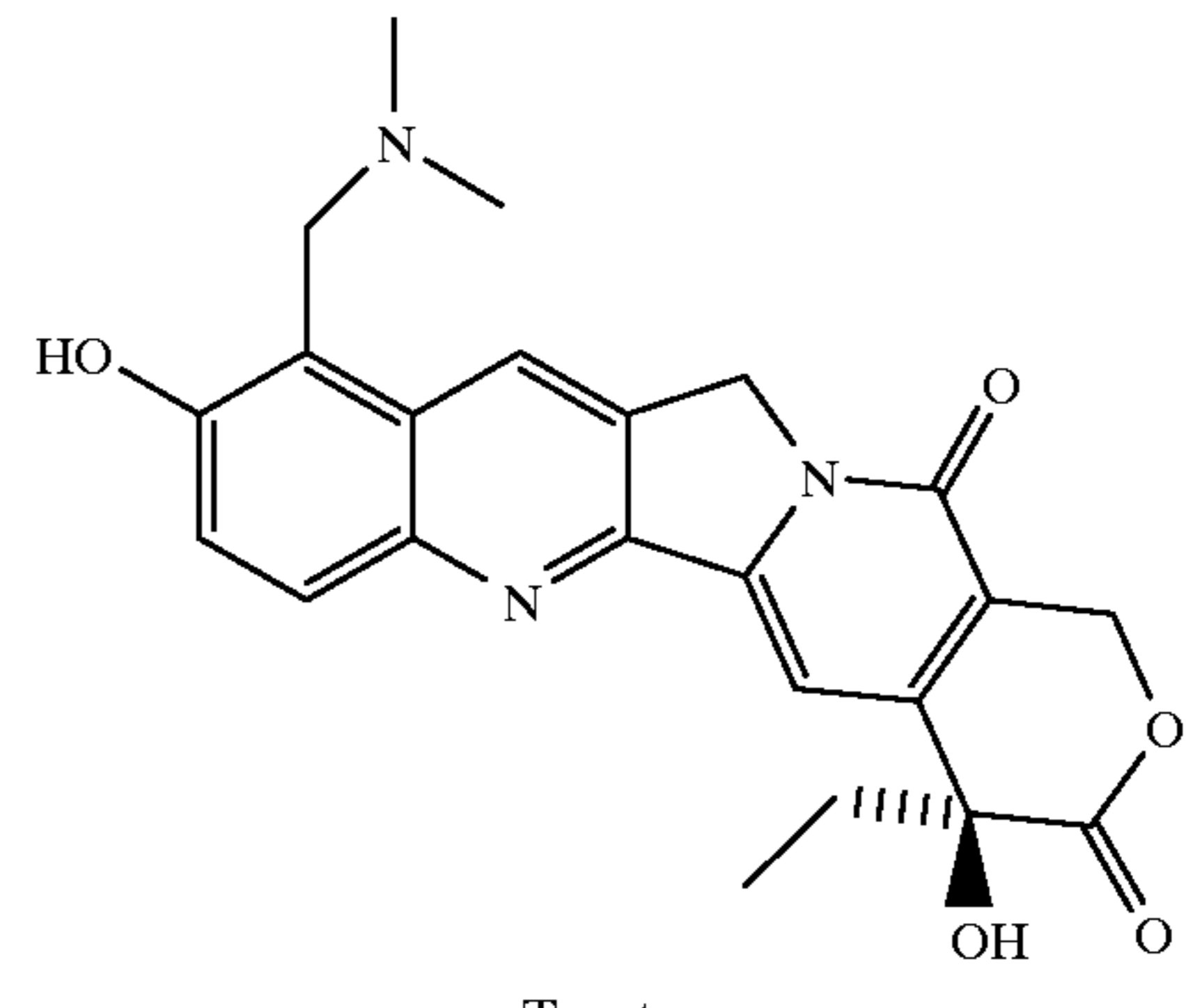
Topotecan
