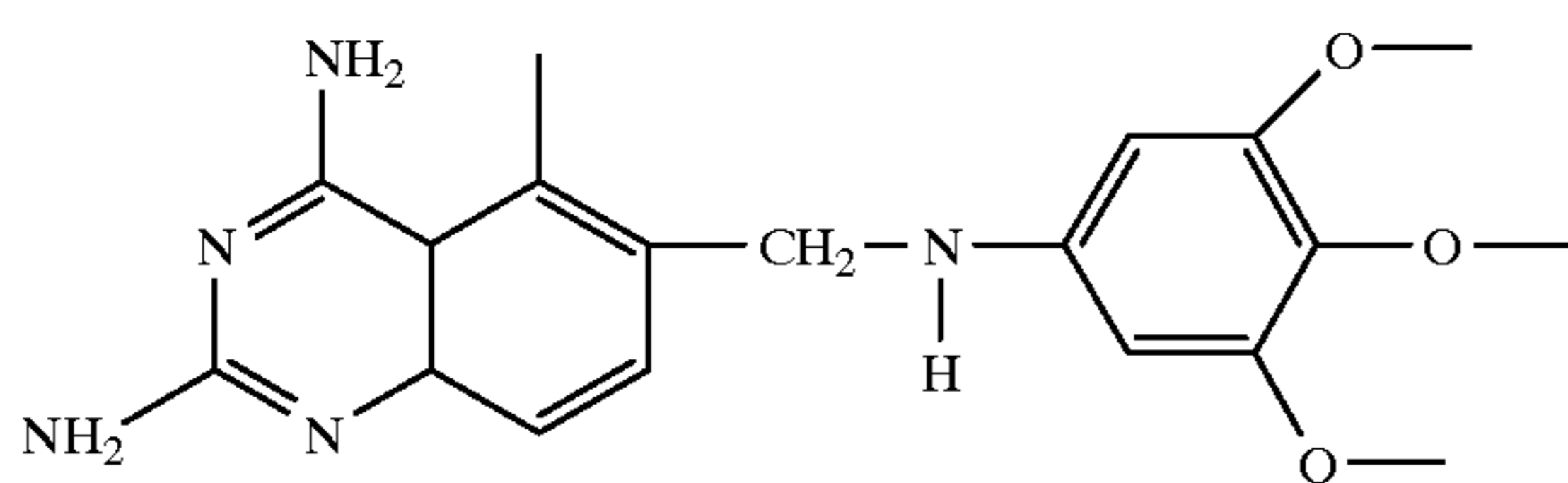
Trimetrexate
