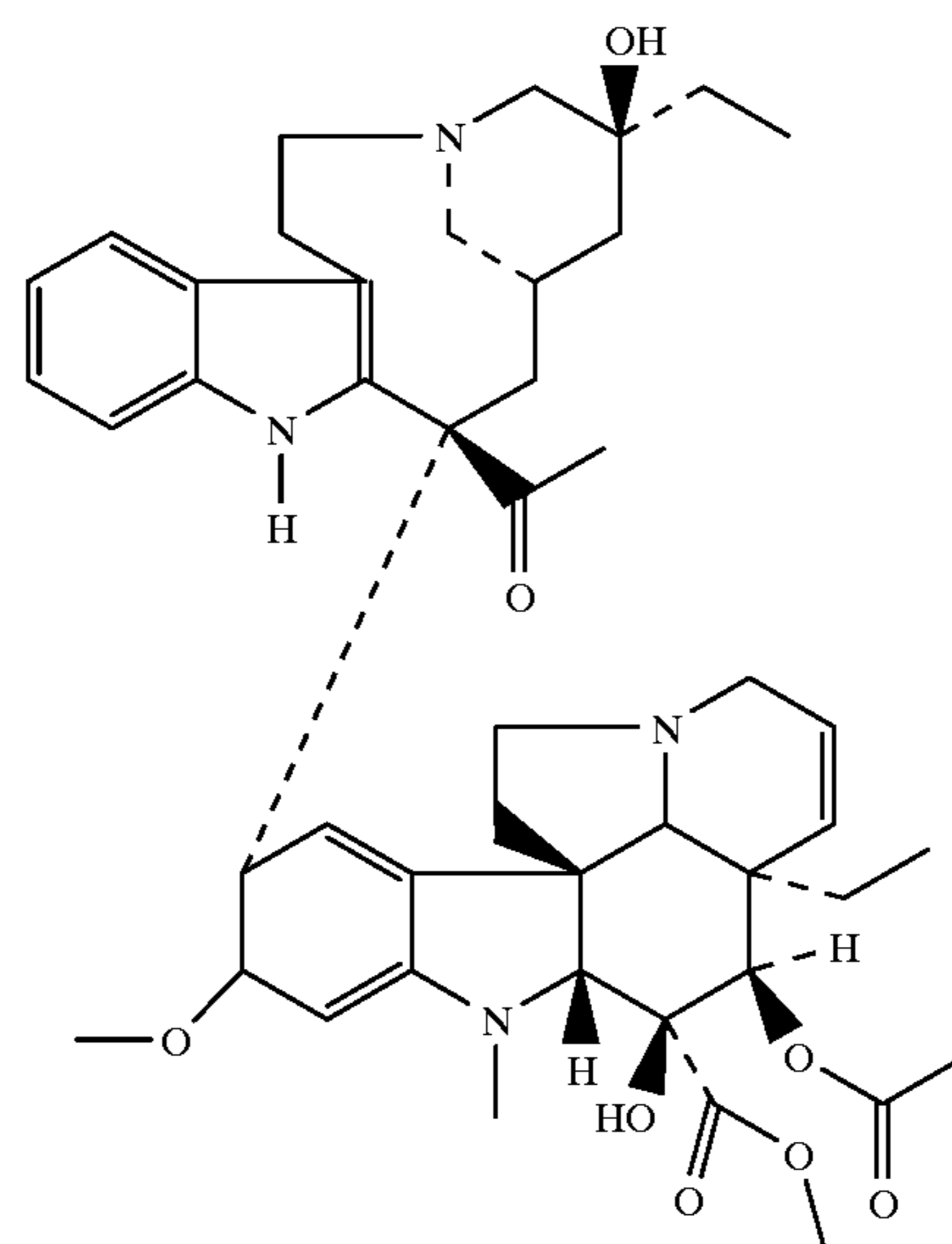
Vinblastine
