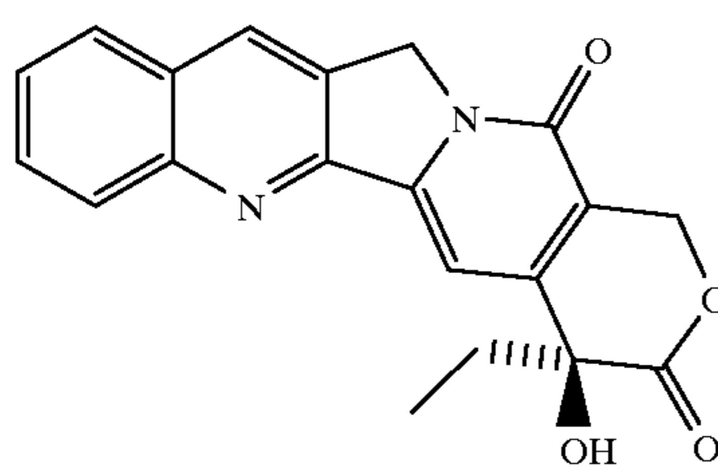
Camptothecin
