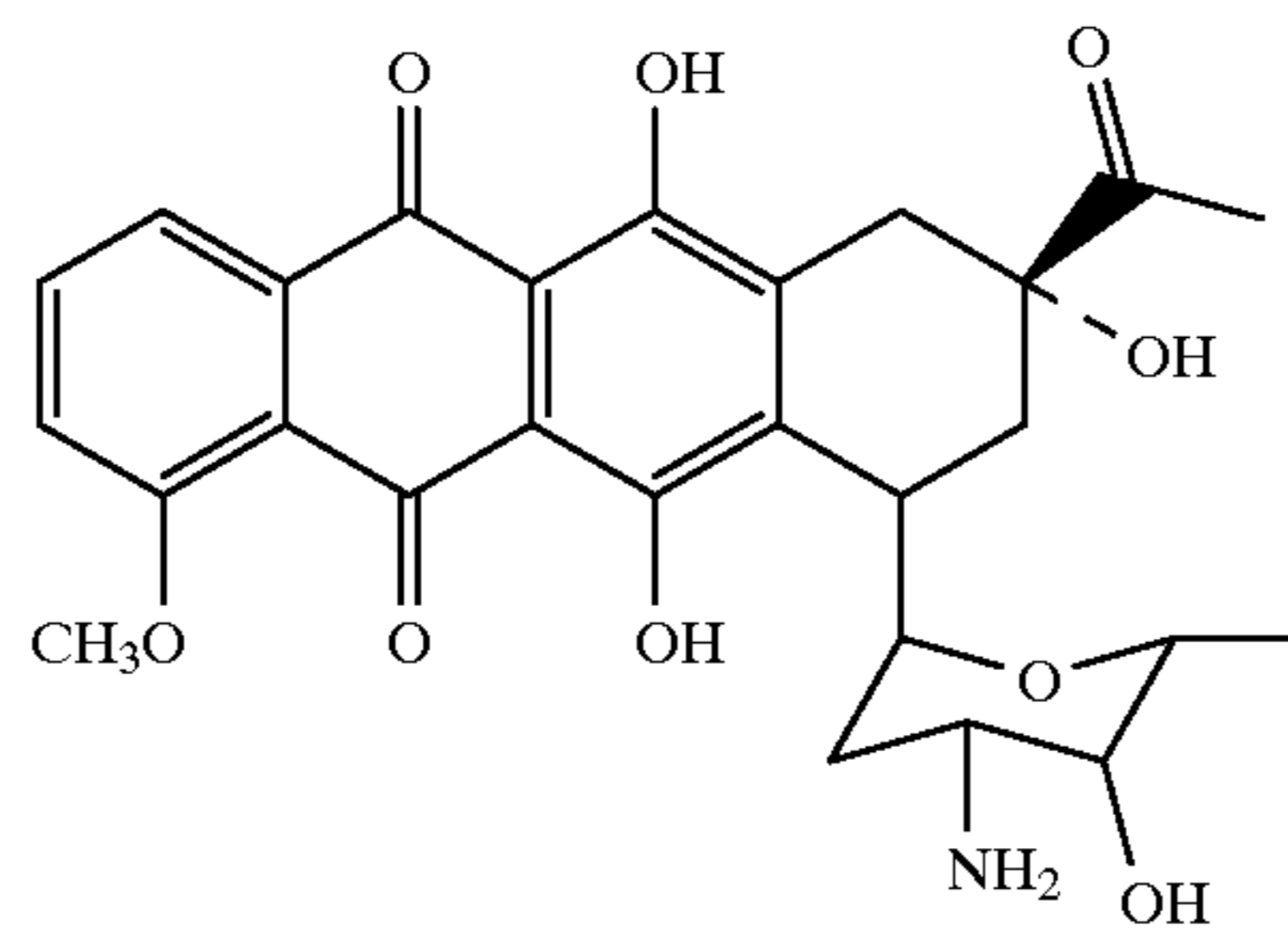
Daunorubicin
