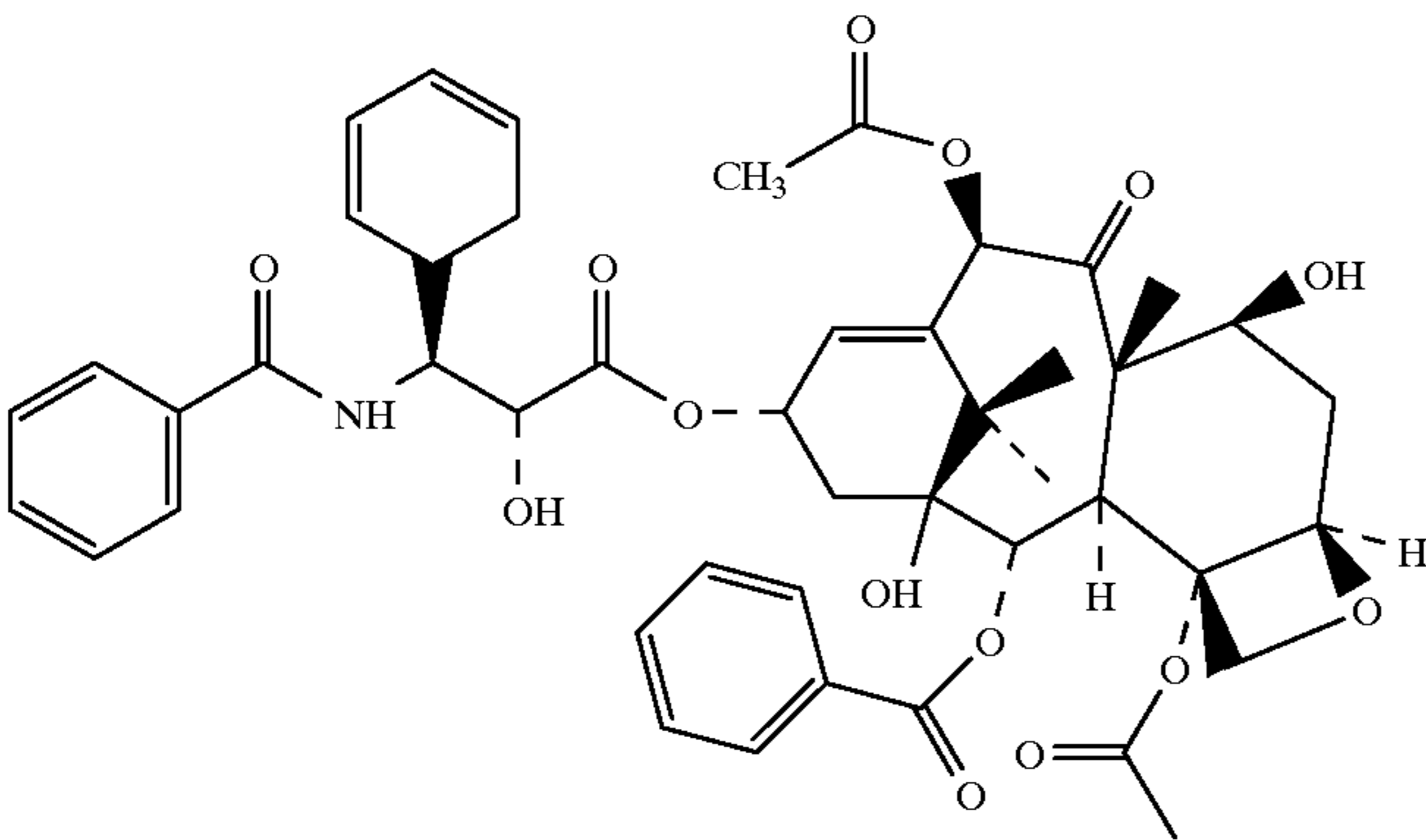
Taxol
