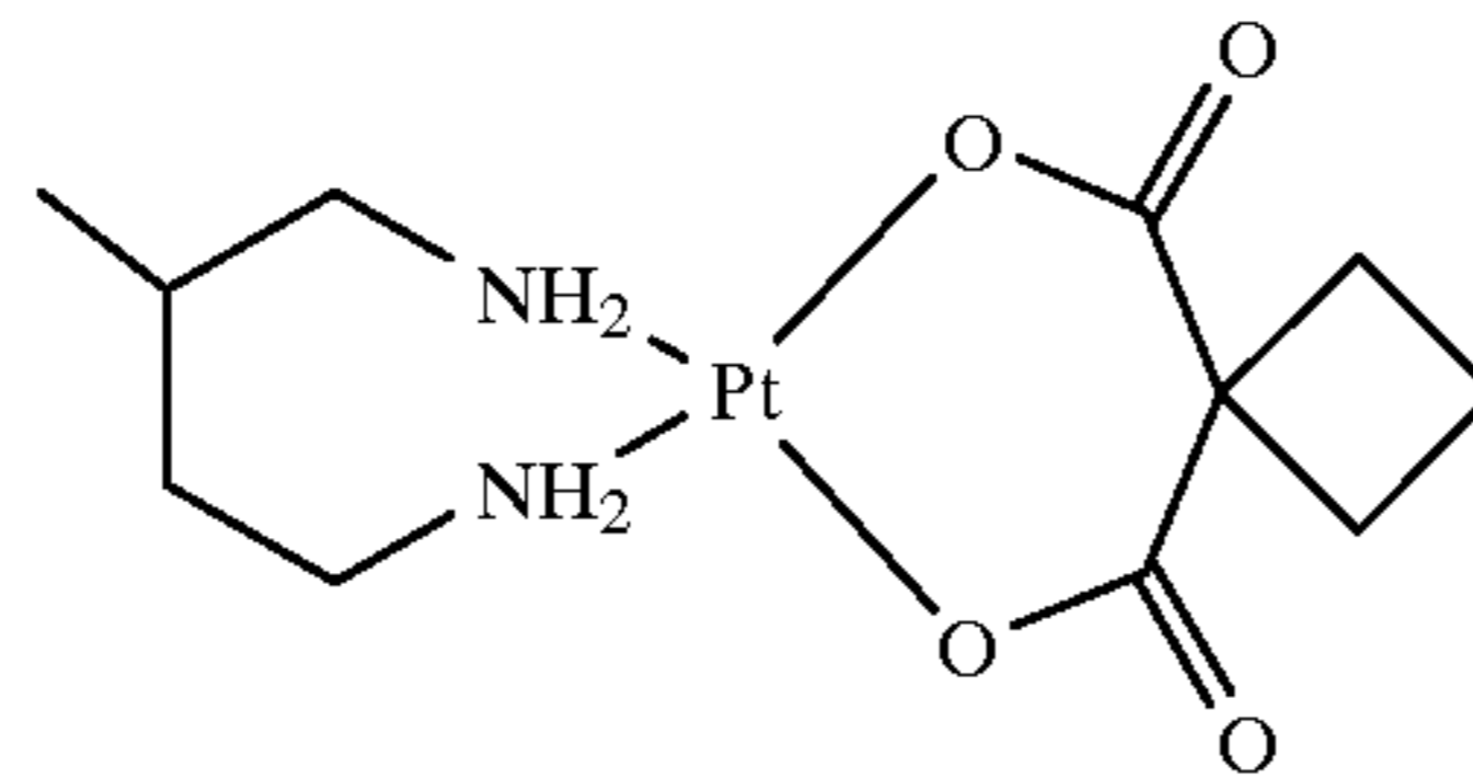
CI-973
