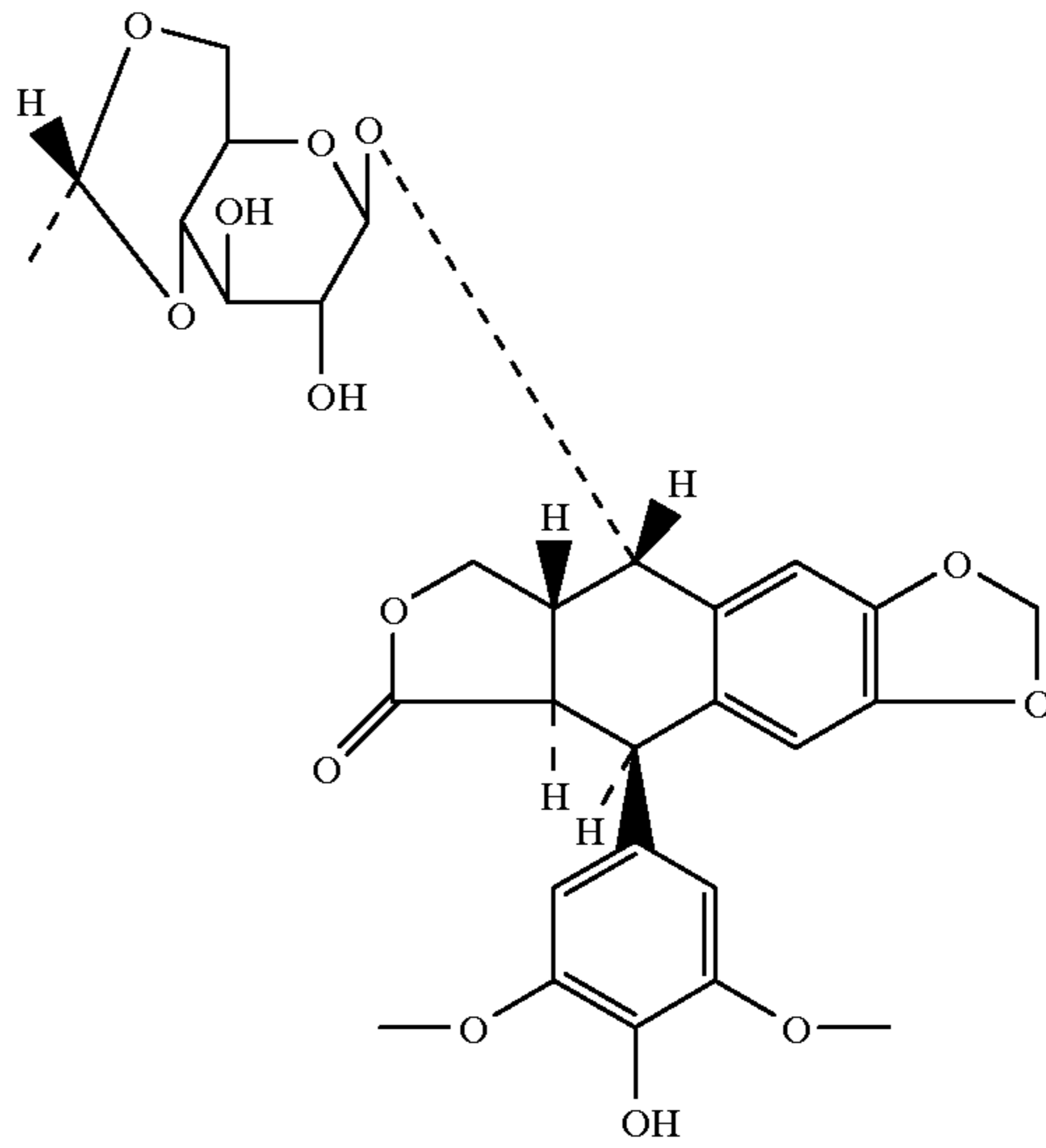
Etoposide
