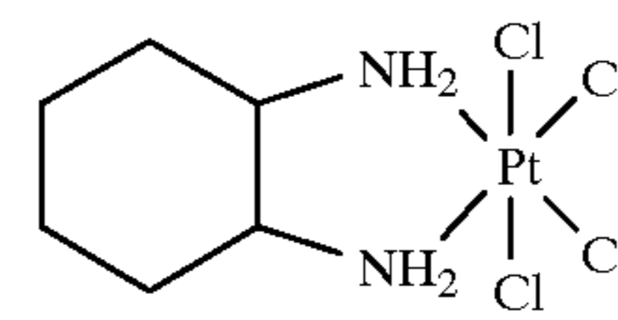
Tetraplatin (Ormaplatin)
