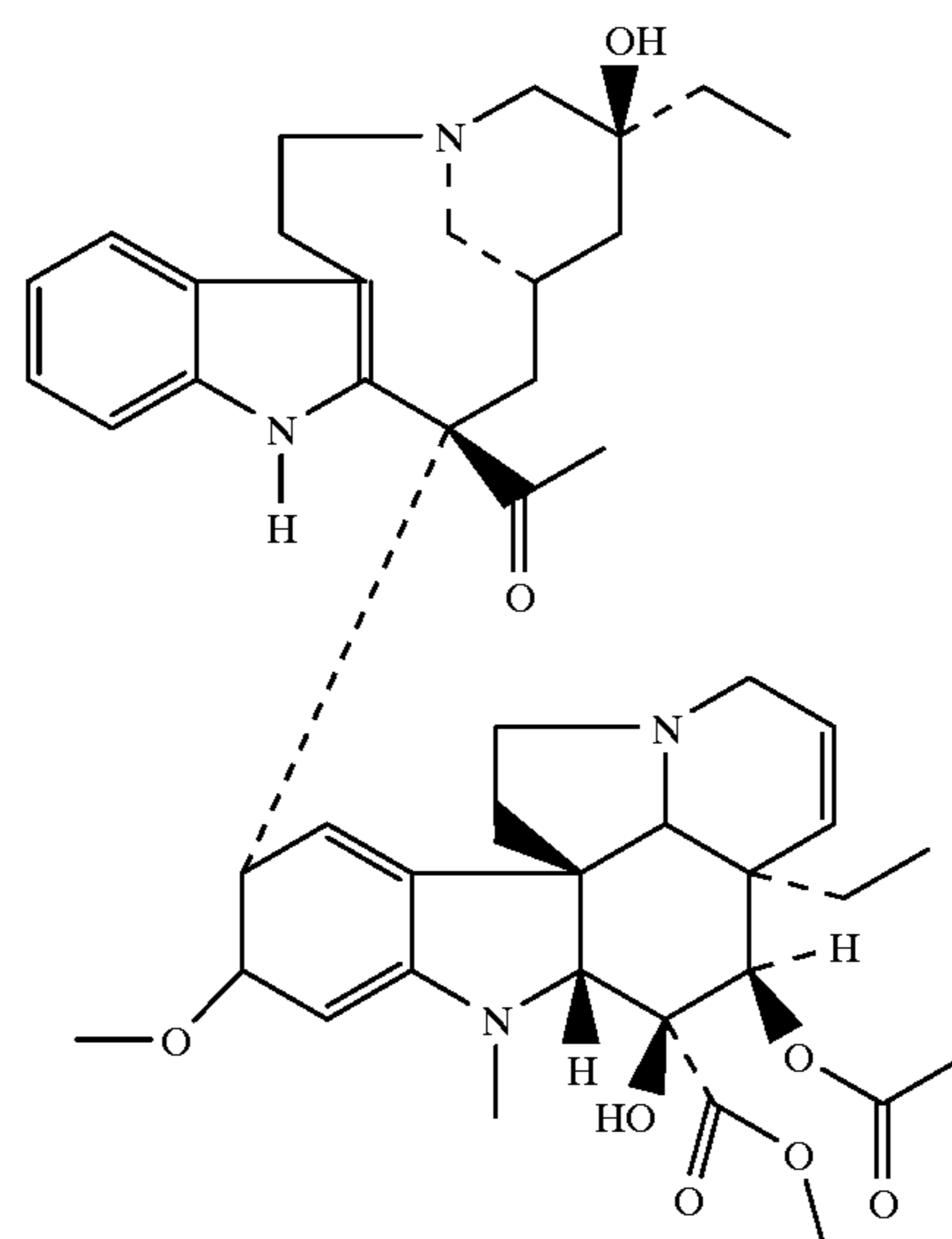
Vinblastine
