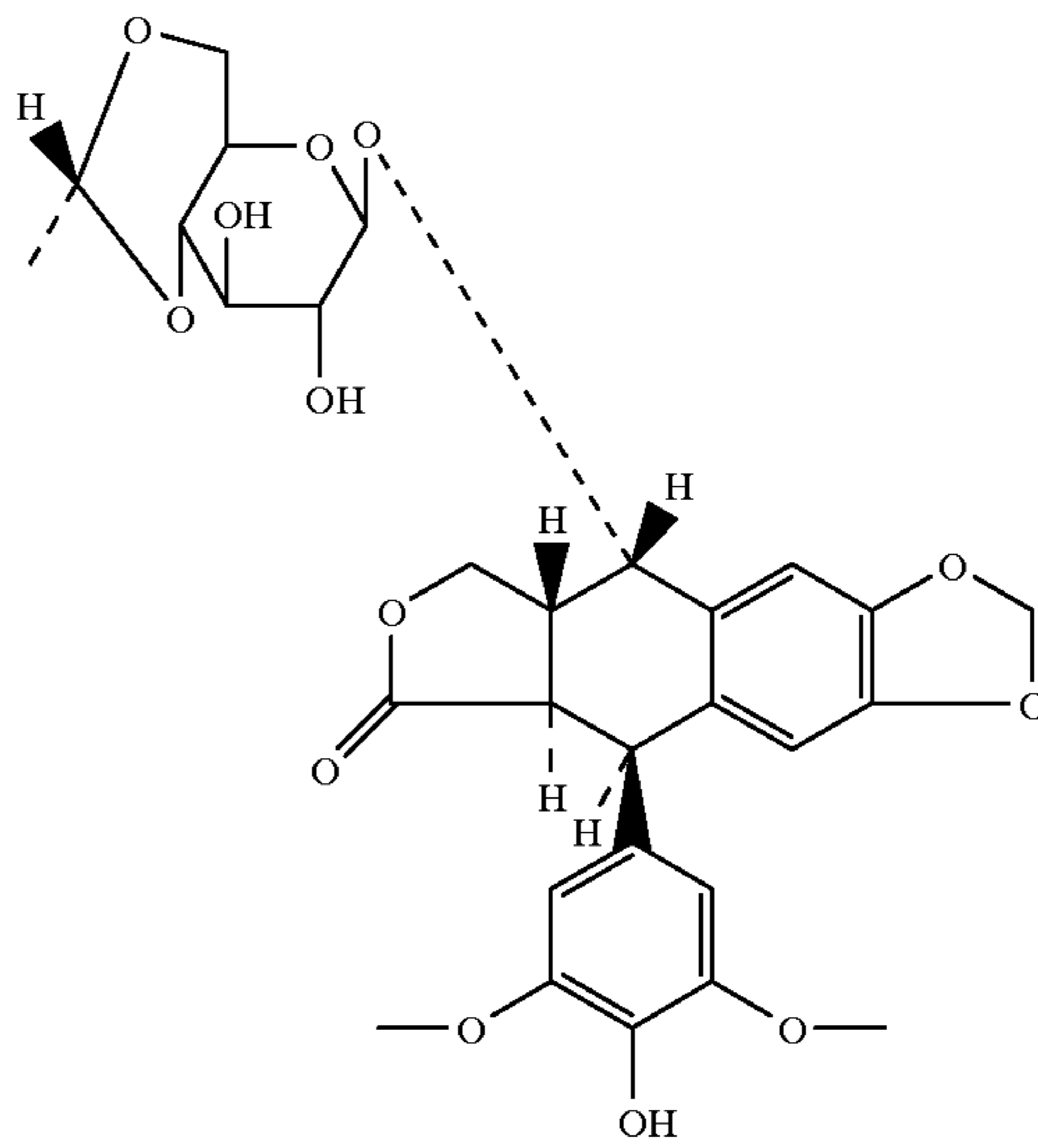
Etoposide
