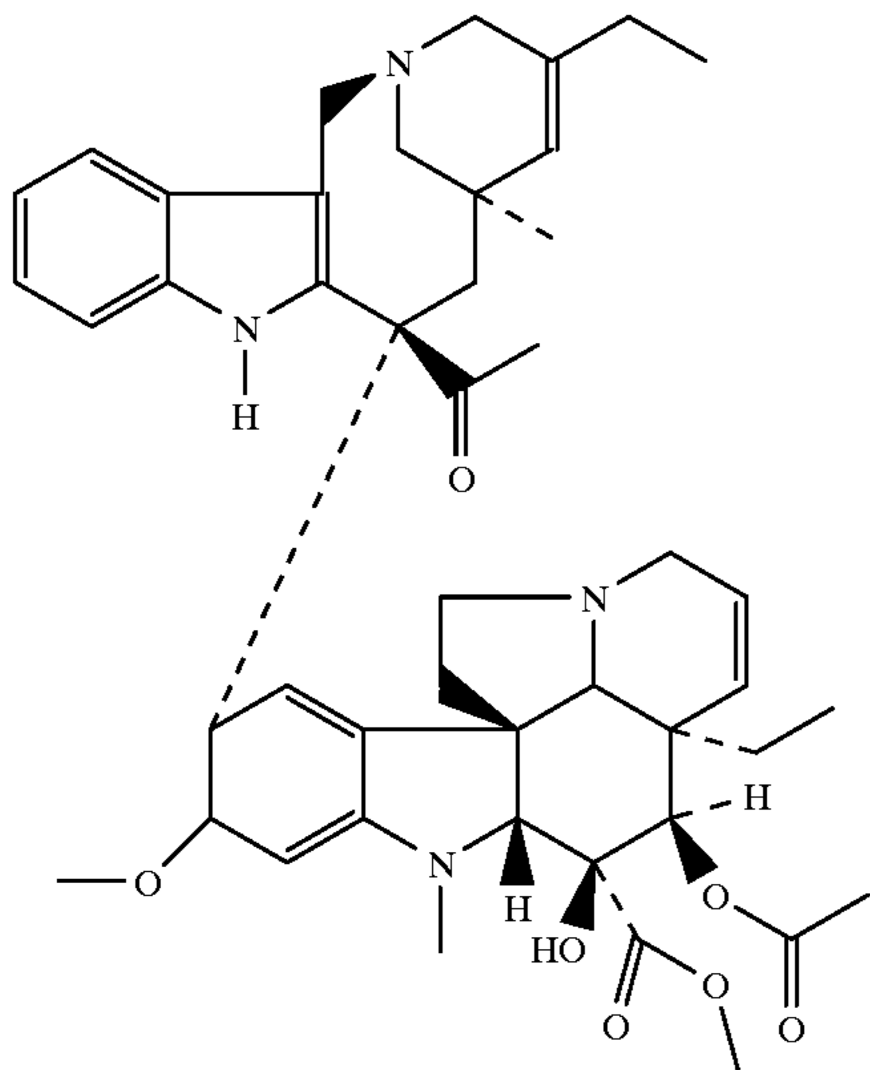
Vinorelbine
