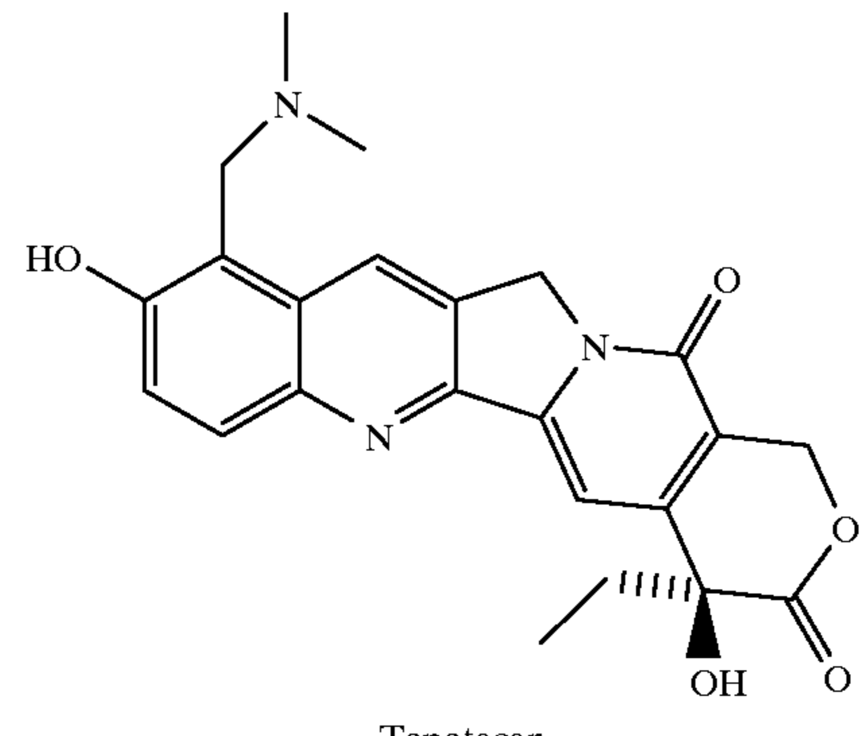
Topotecan
