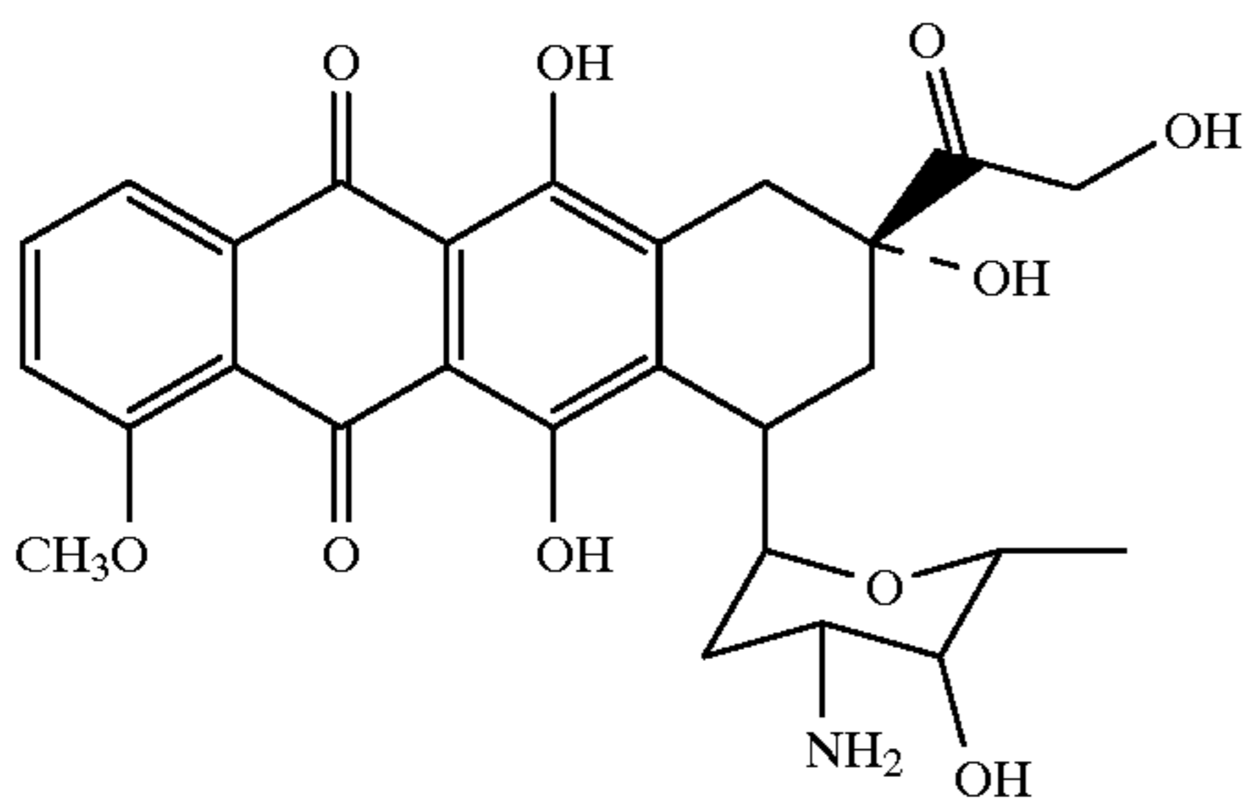
Doxorubicin
