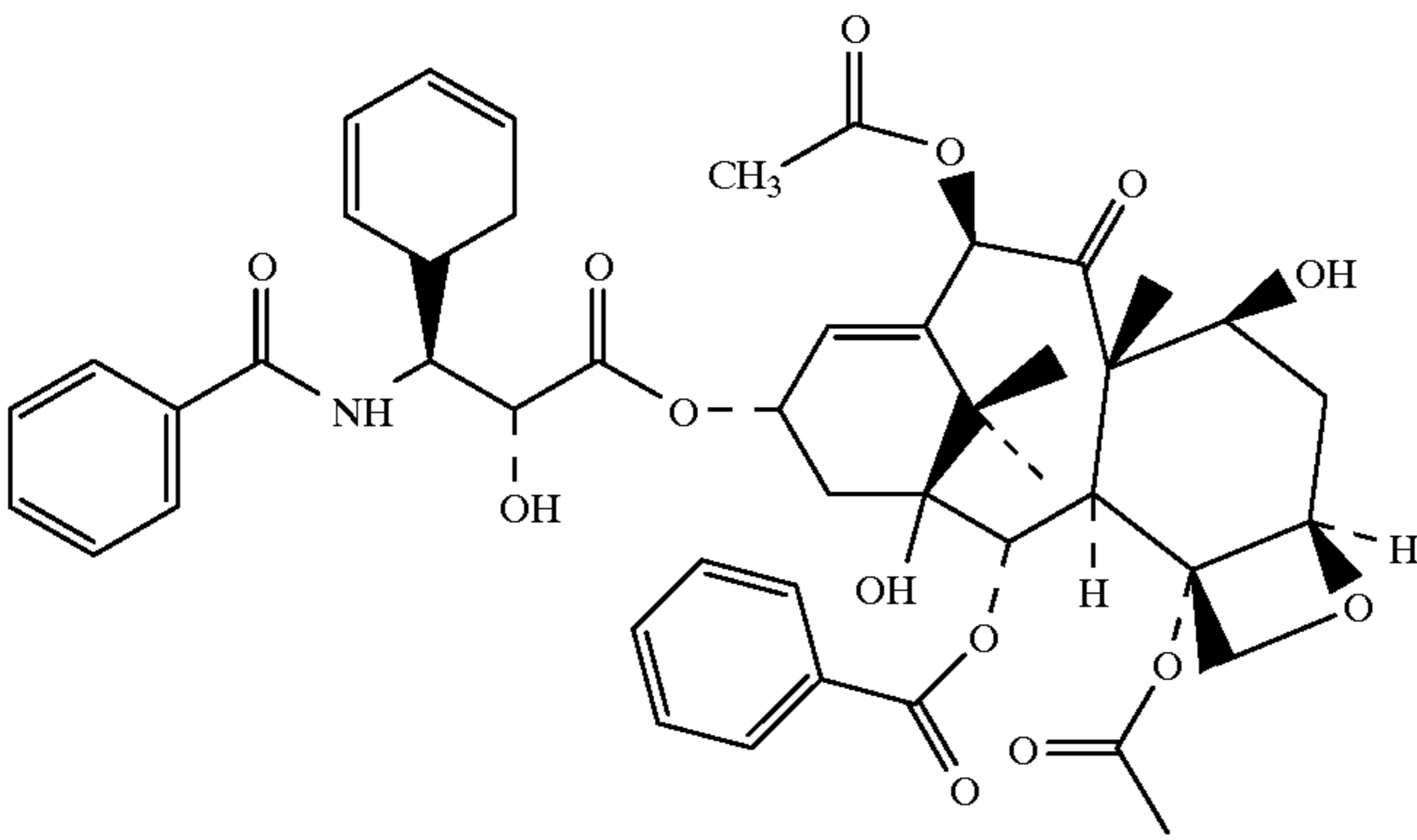
Taxol
