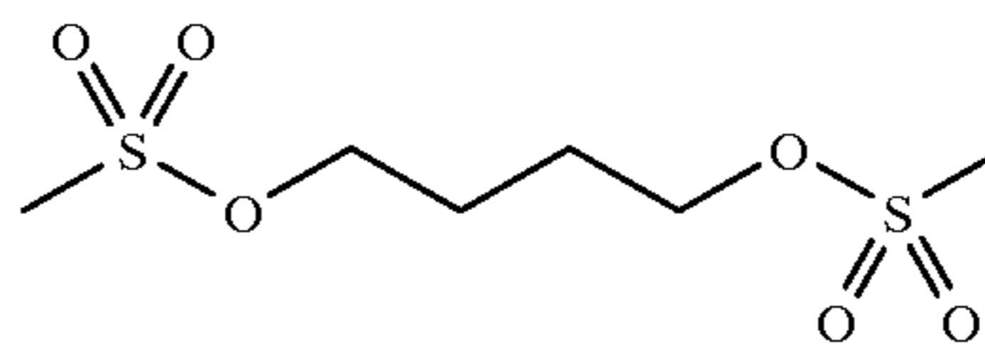
Busulfan
