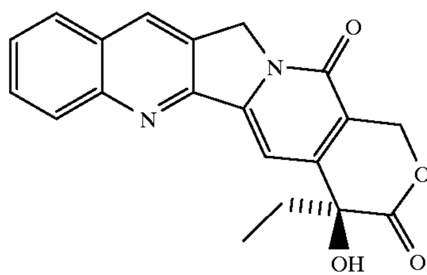
Camptothecin
