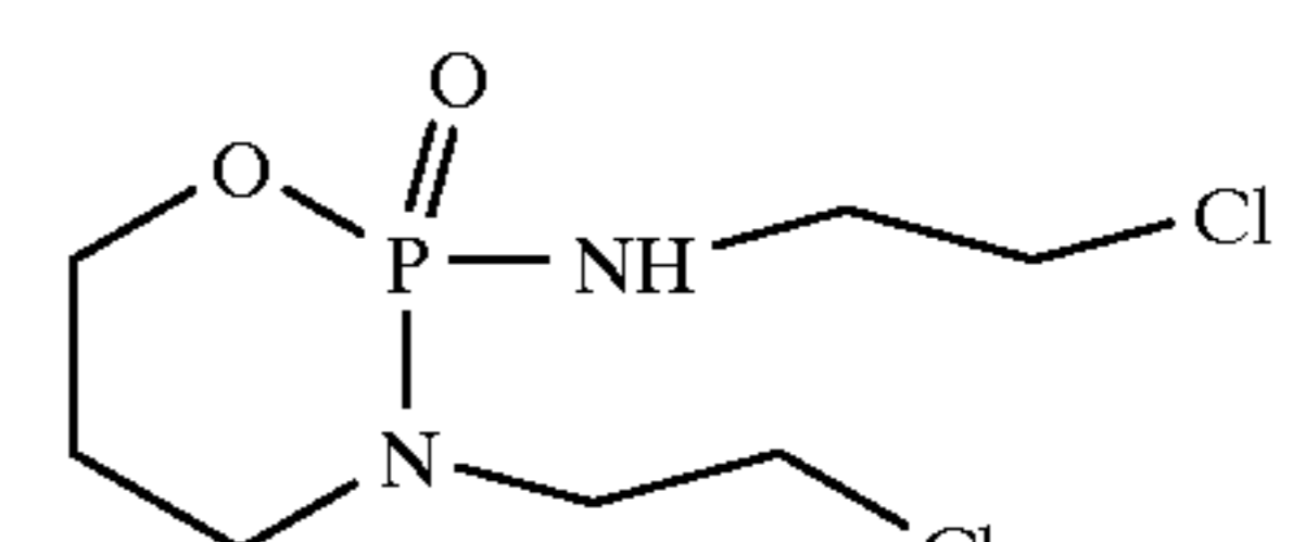
Ifosfamide
