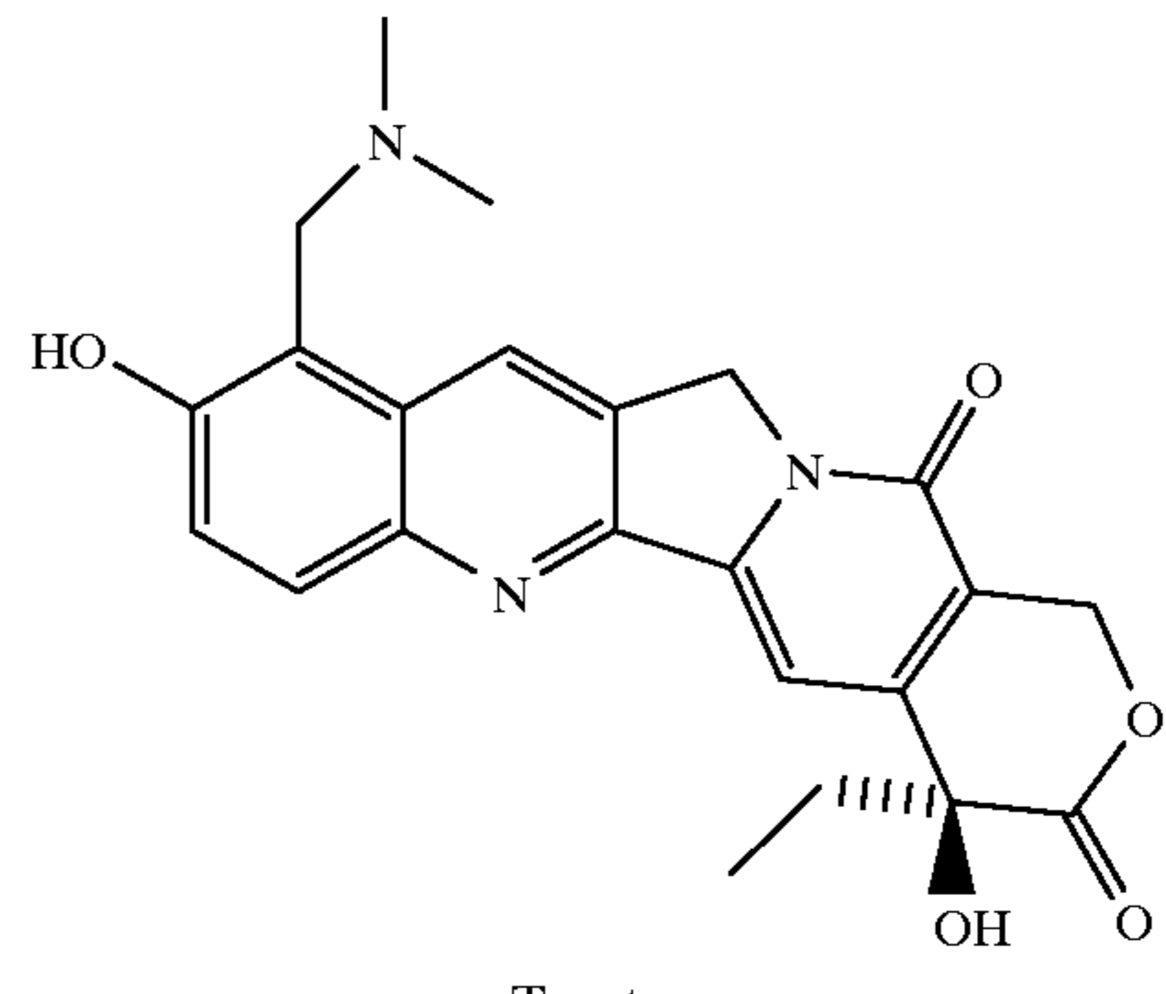
Topotecan
