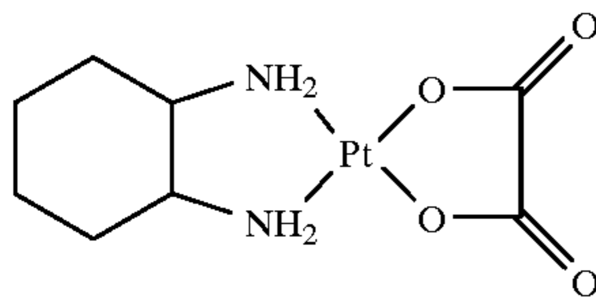
Oxaliplatin
