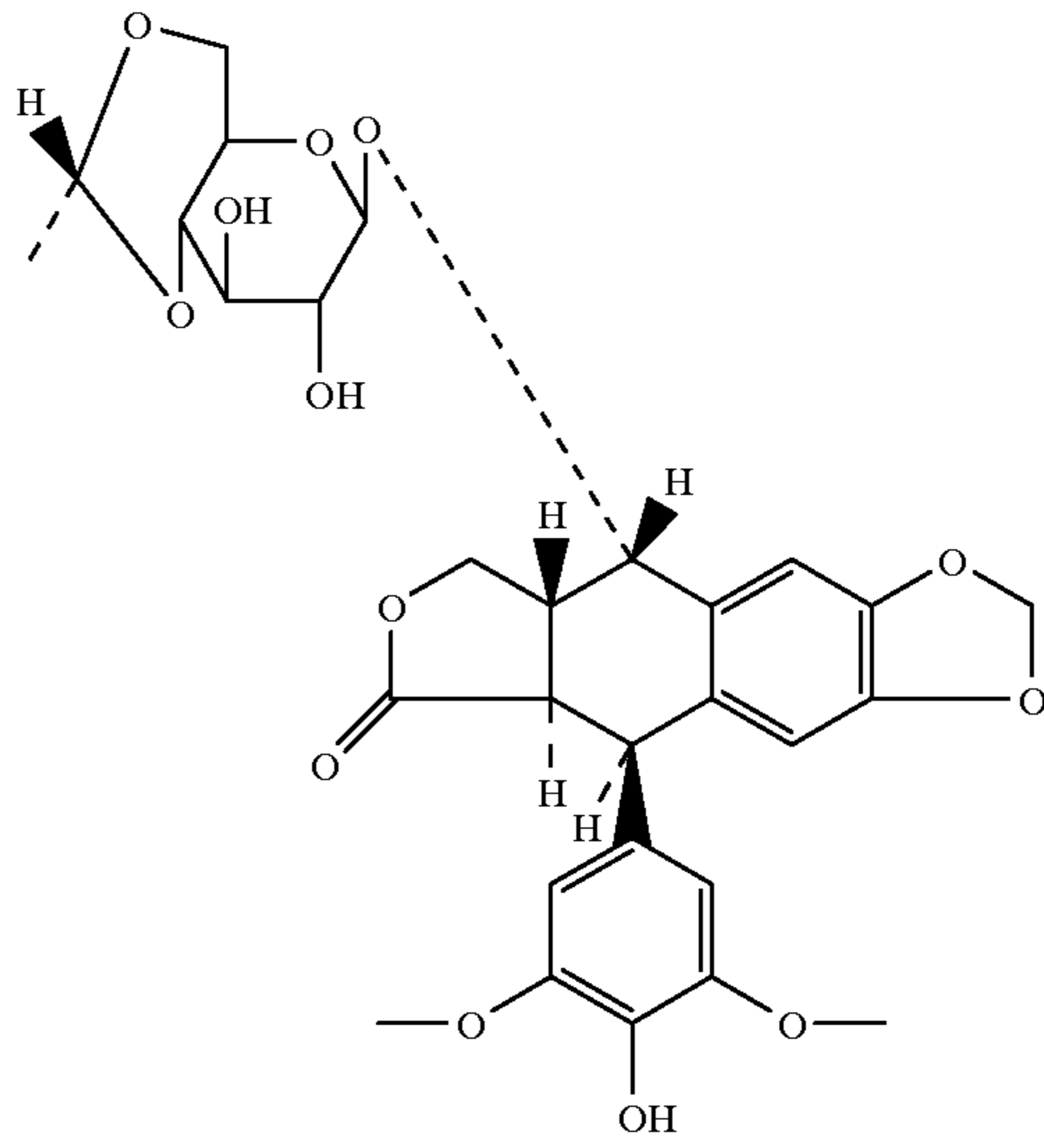
Etoposide
