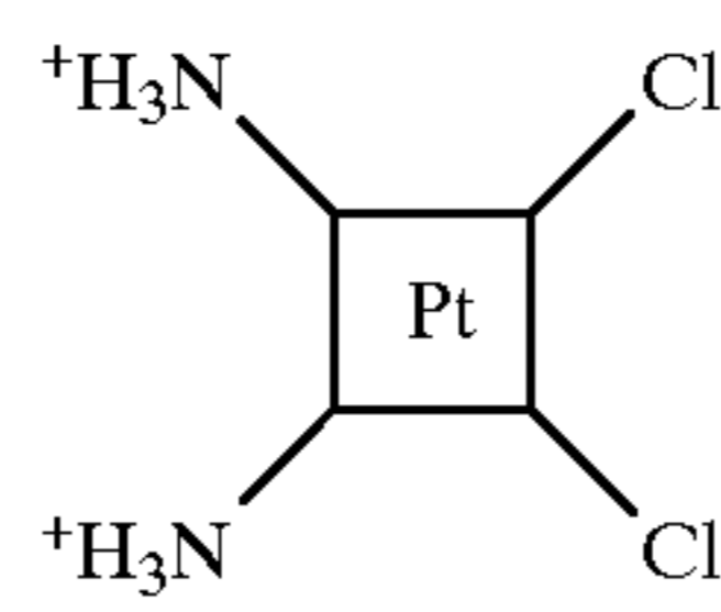
Cisplatin
