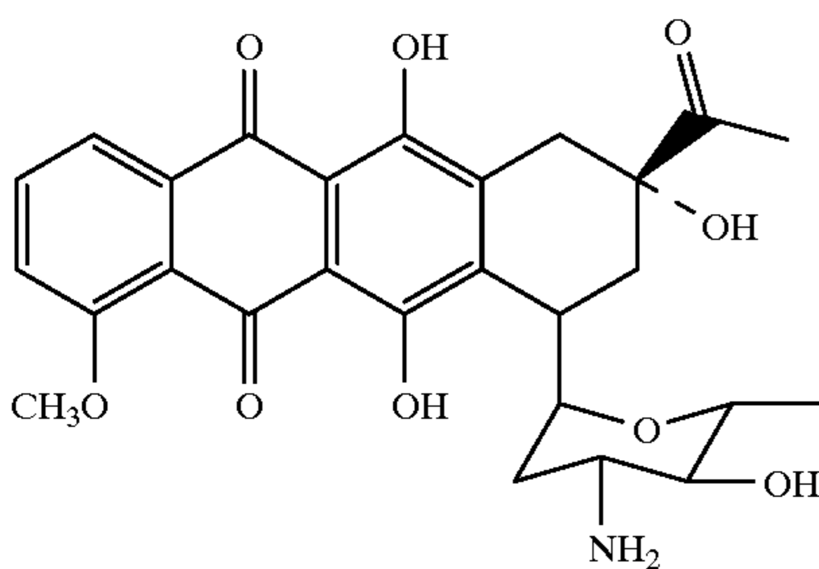
Epirubicin
