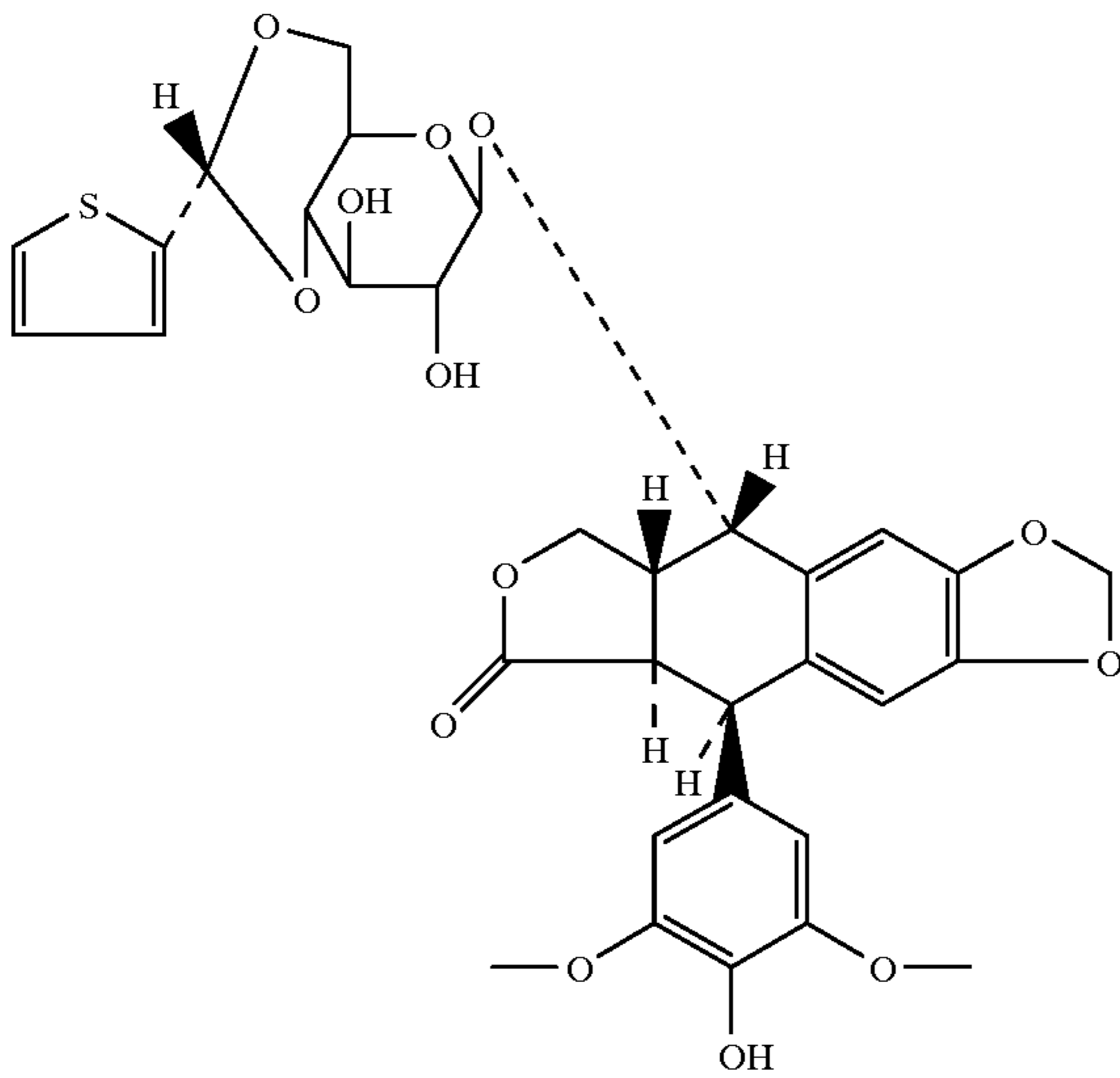
Teniposide
