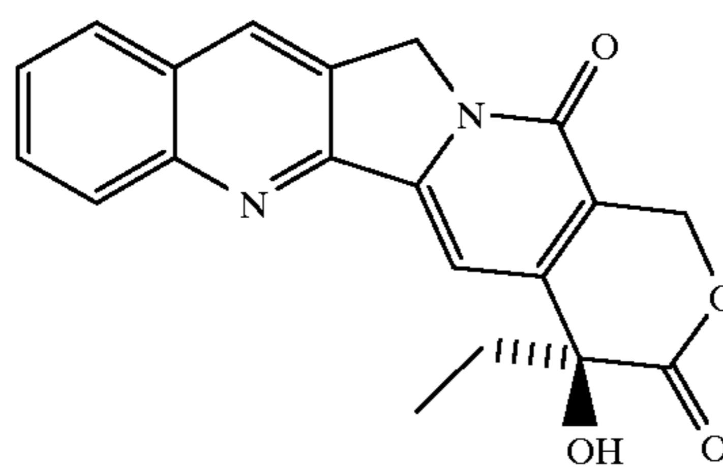
Camptothecin
