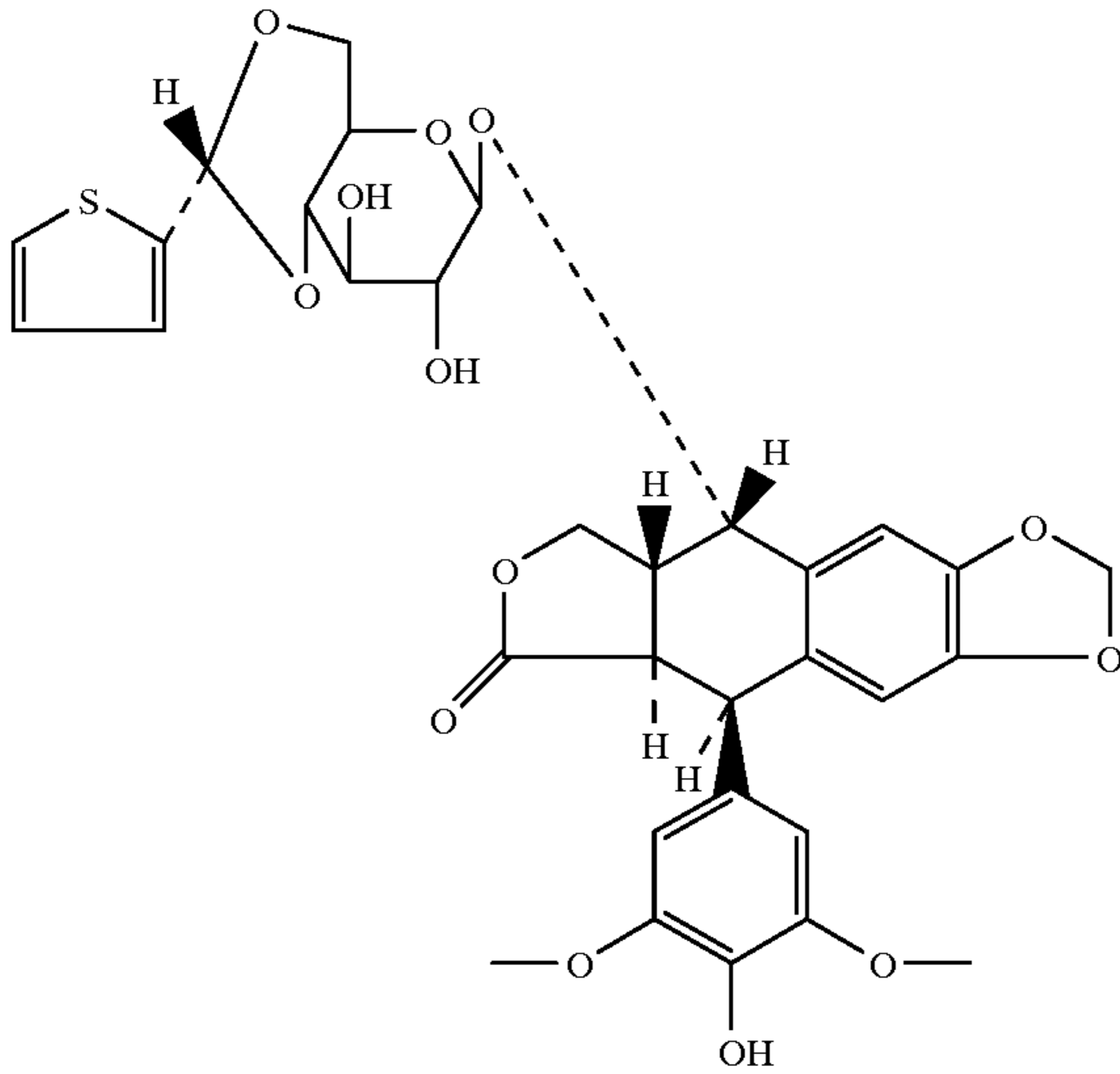
Teniposide
