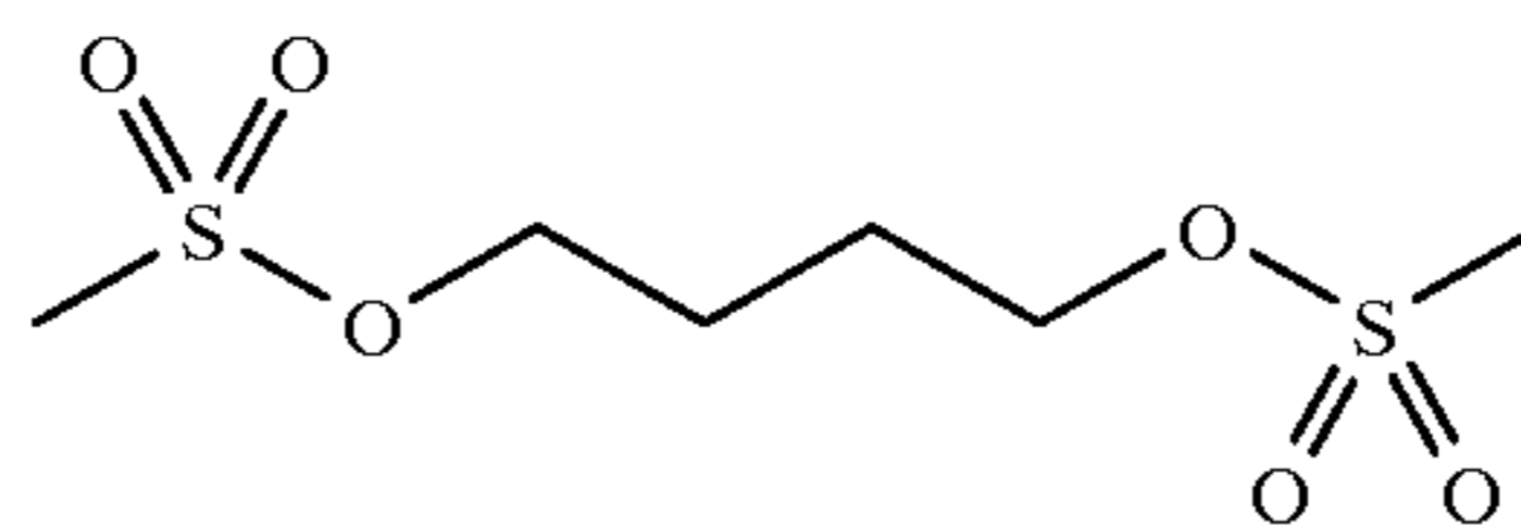
Busulfan
