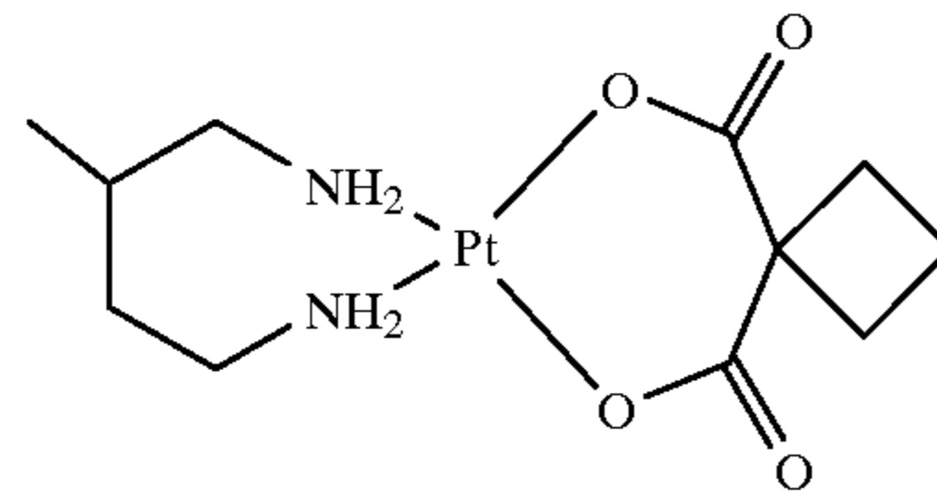
CI-973
