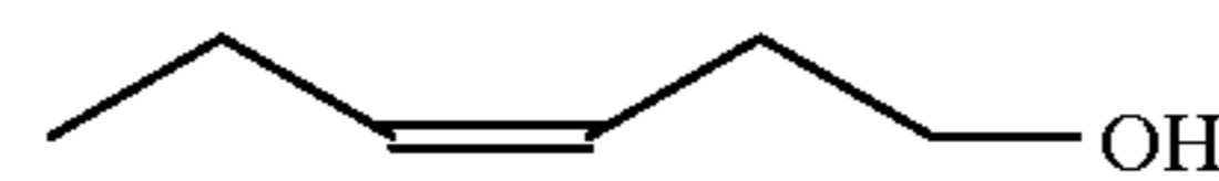
cis-3-hexen-1-ol
