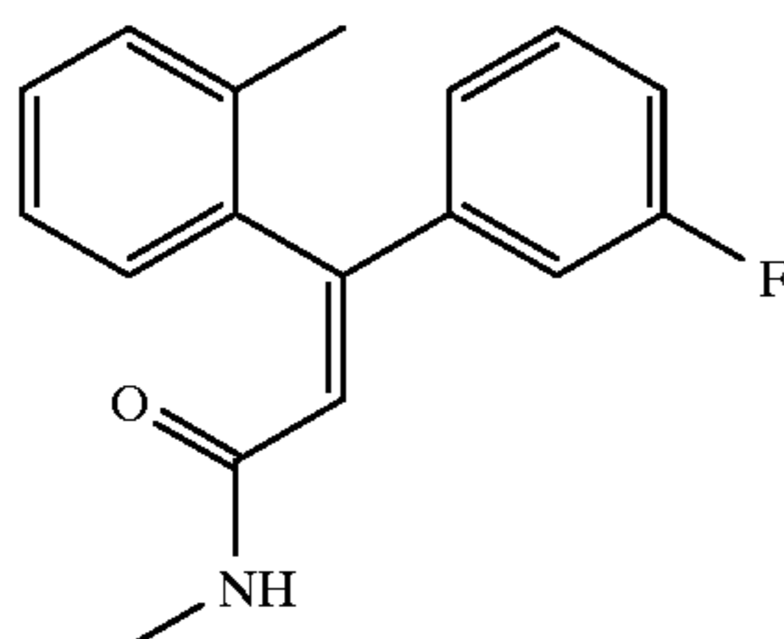
(Z)-3-(3-fluorophenyl)-N-methyl-3-(2-tolyl)-2-propenamide
