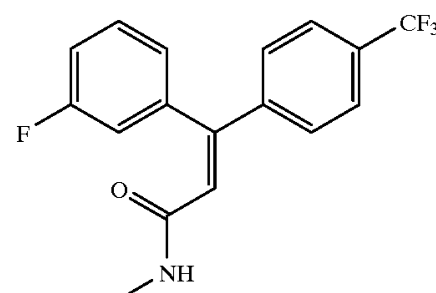
(Z)-3-(4-α,α,α-trifluoromethylphenyl)-3-(3-fluorophenyl)-N-methyl-2-propenamide
