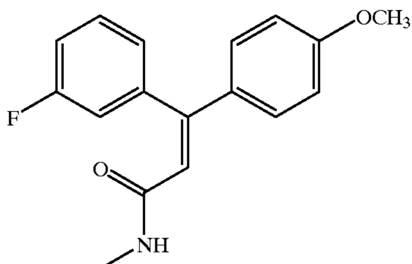
(Z)-3-(4-anisyl)-3-(3-fluorophenyl)-N-methyl-2-propenamide
