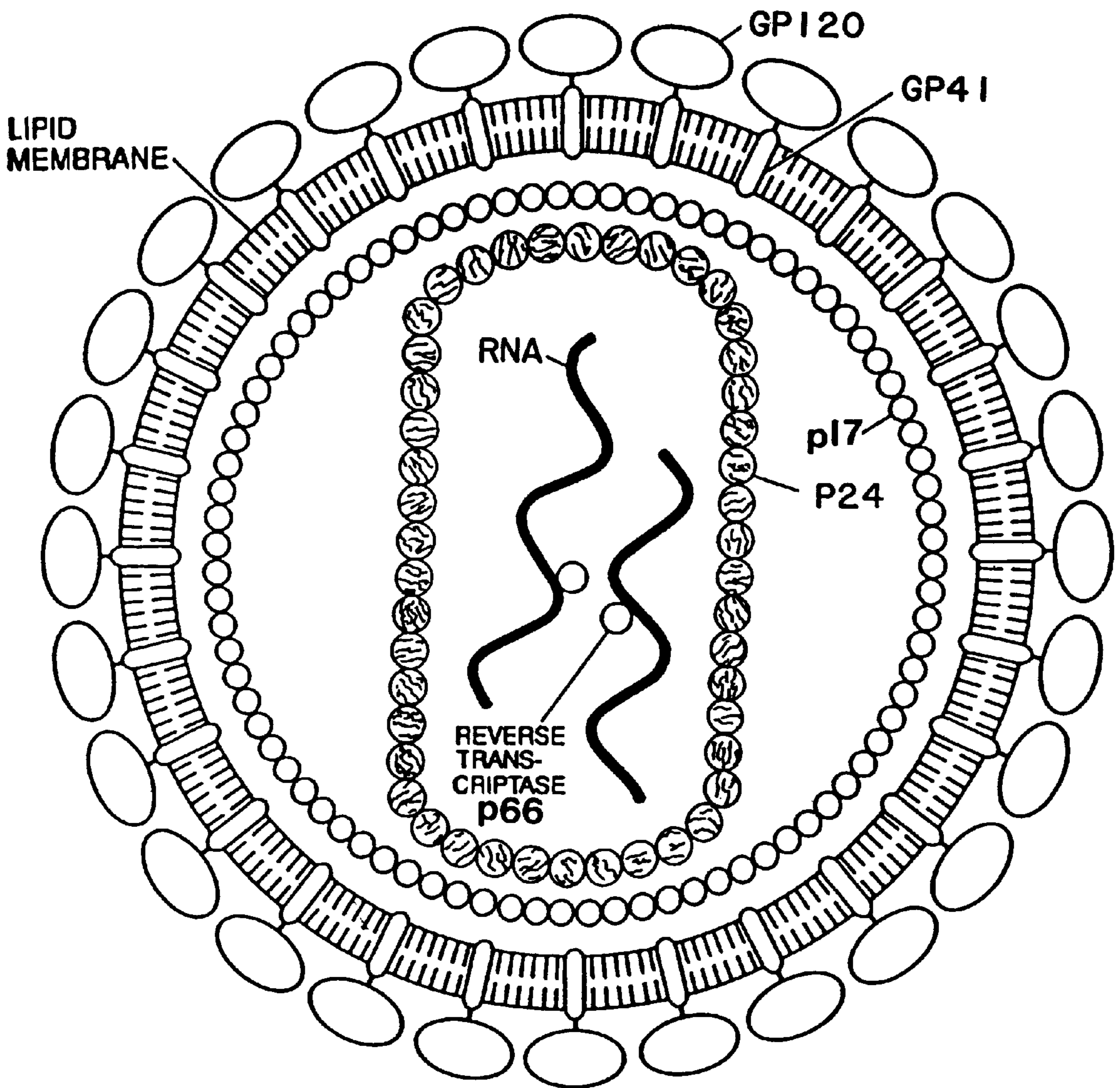
HIV STRUCTURE
