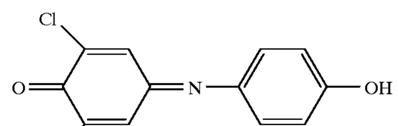
2,6-dichloro-indophenol ("DCI")
