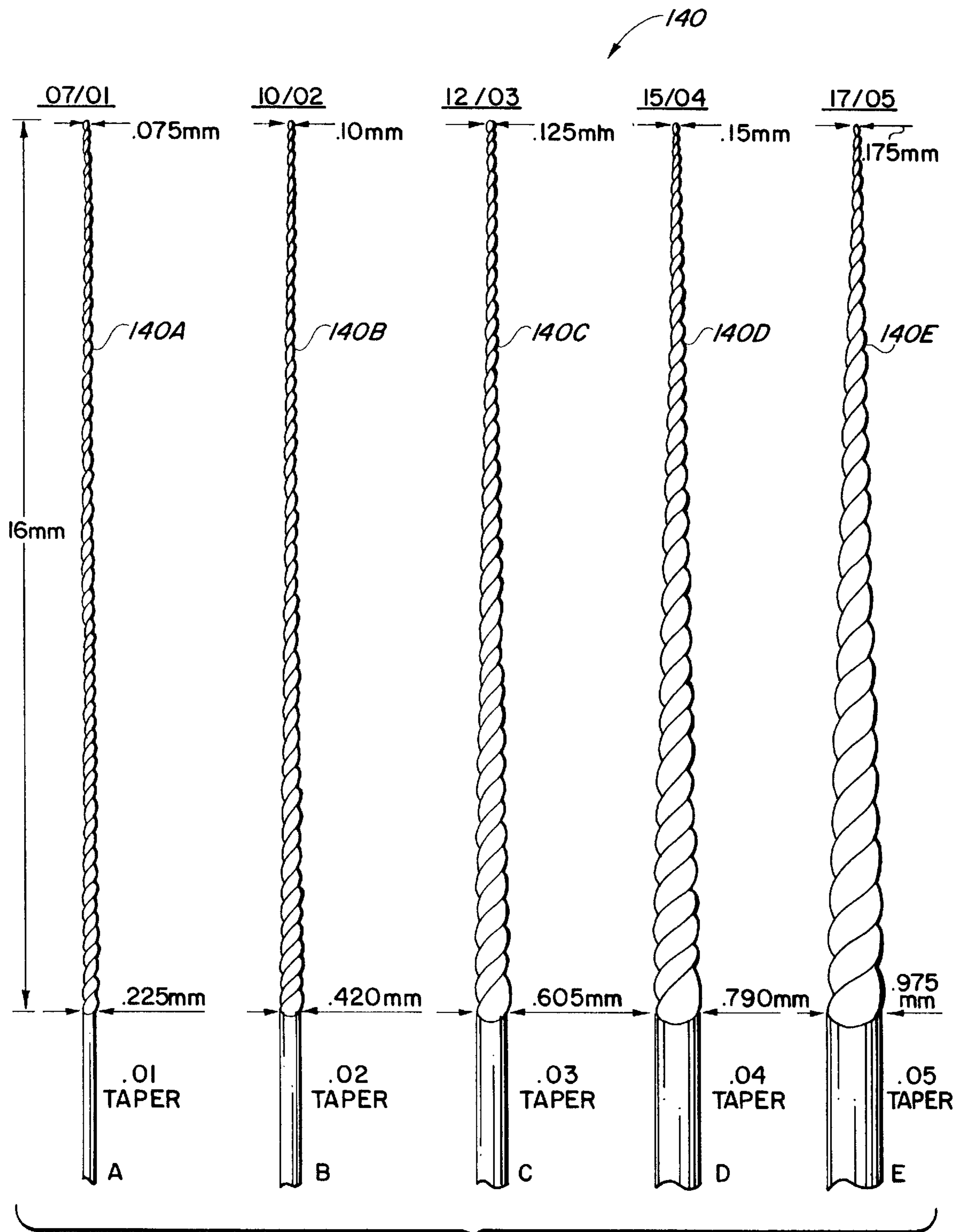
FIG. 15B
