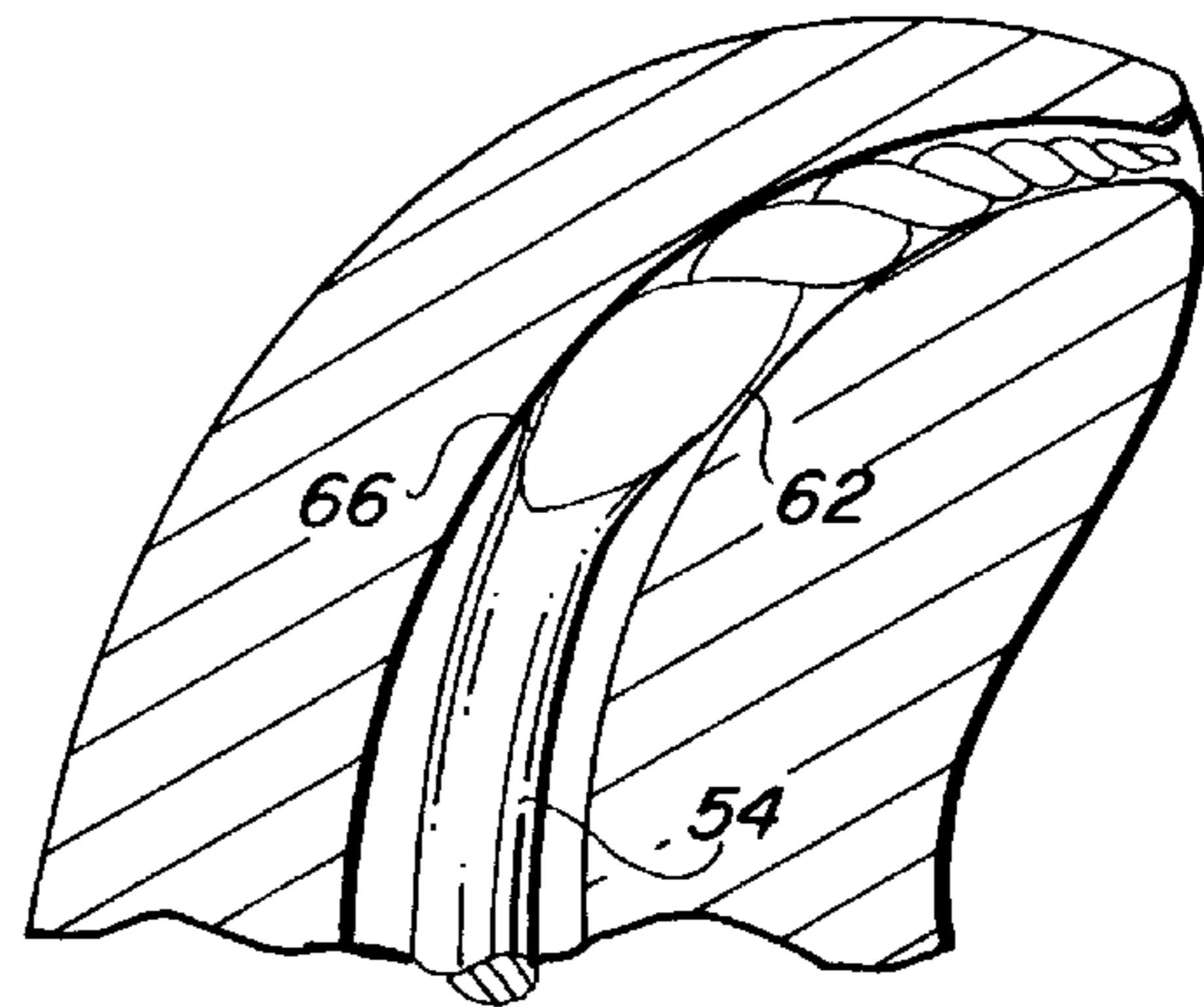
FIG. 6B
