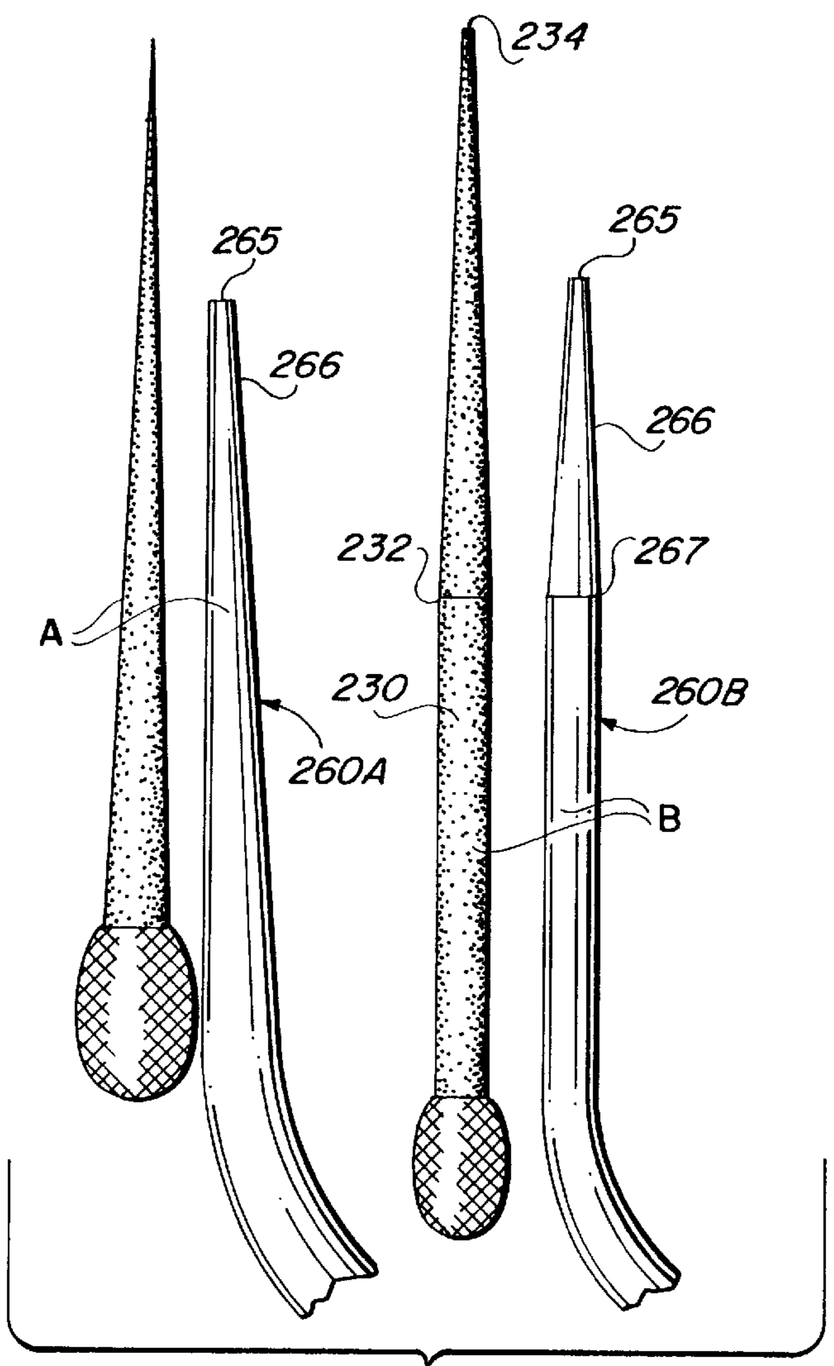
FIG. 18B
