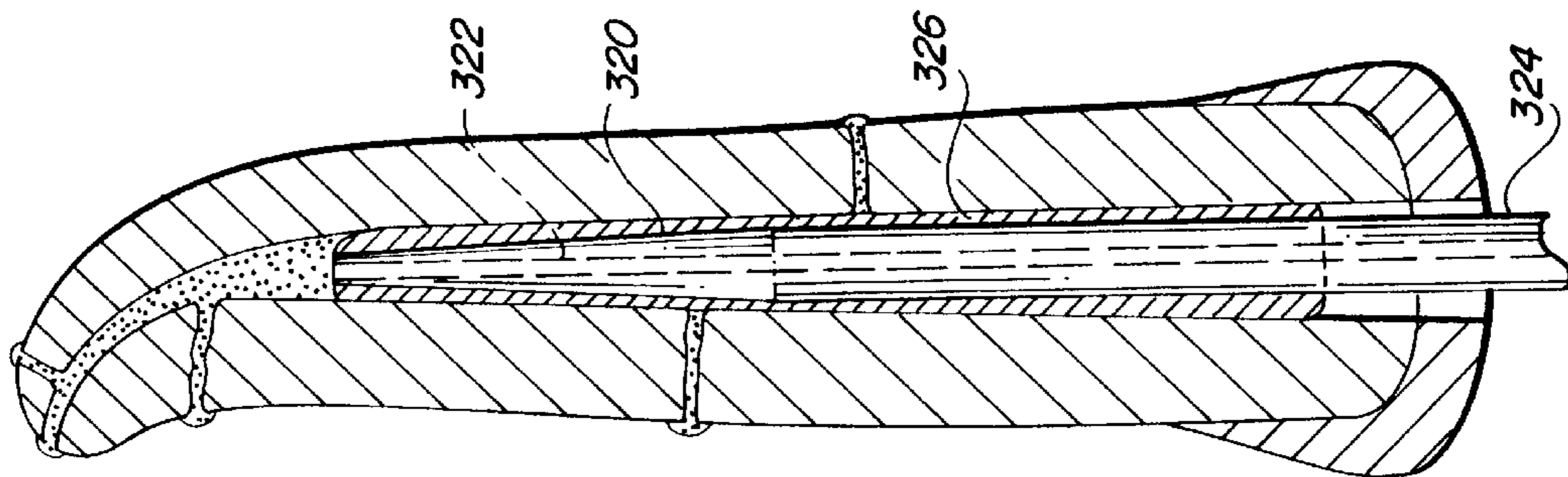
FIG. 21C
