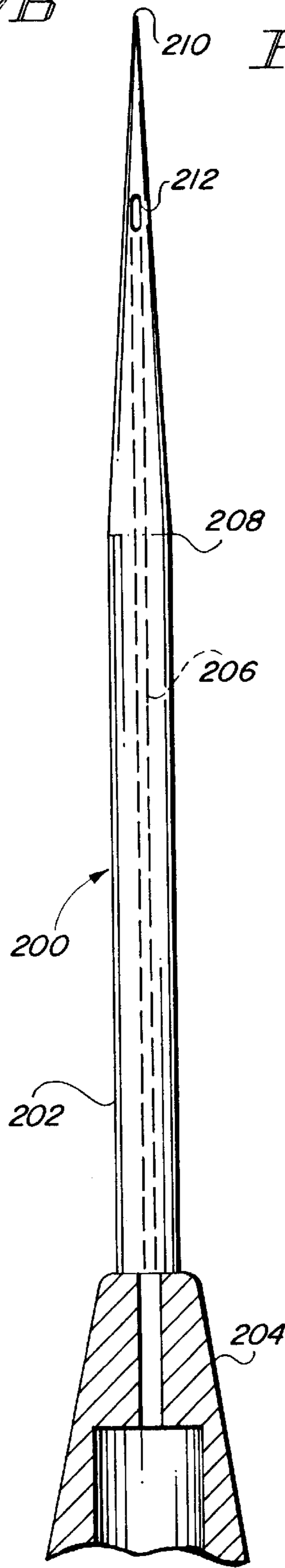
FIG. 17C
