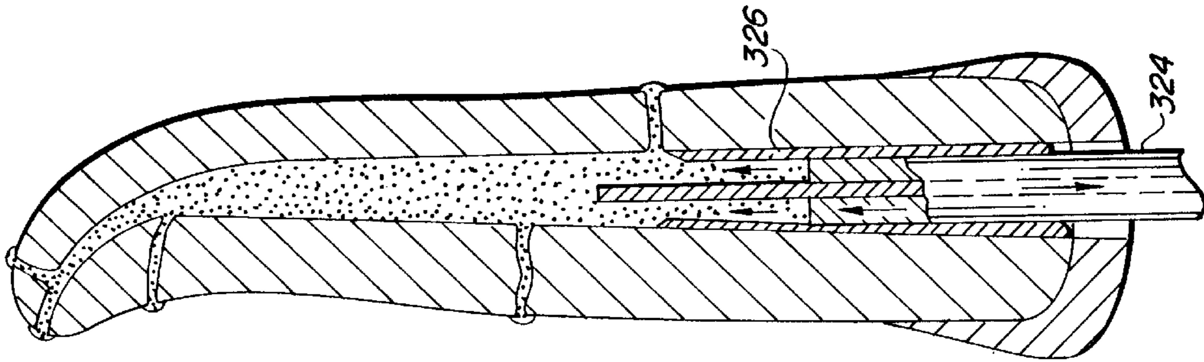
FIG. 21D
