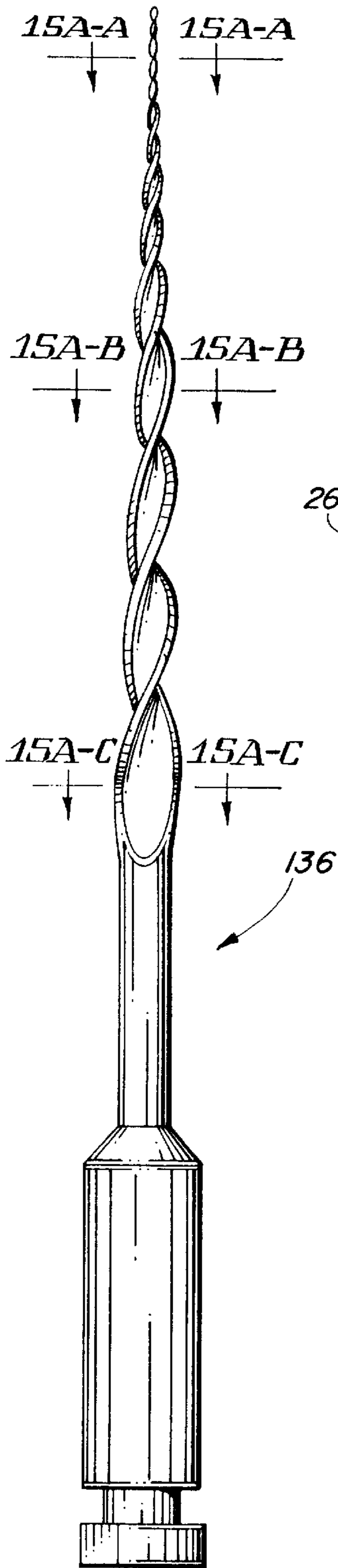
FIG. 15A
