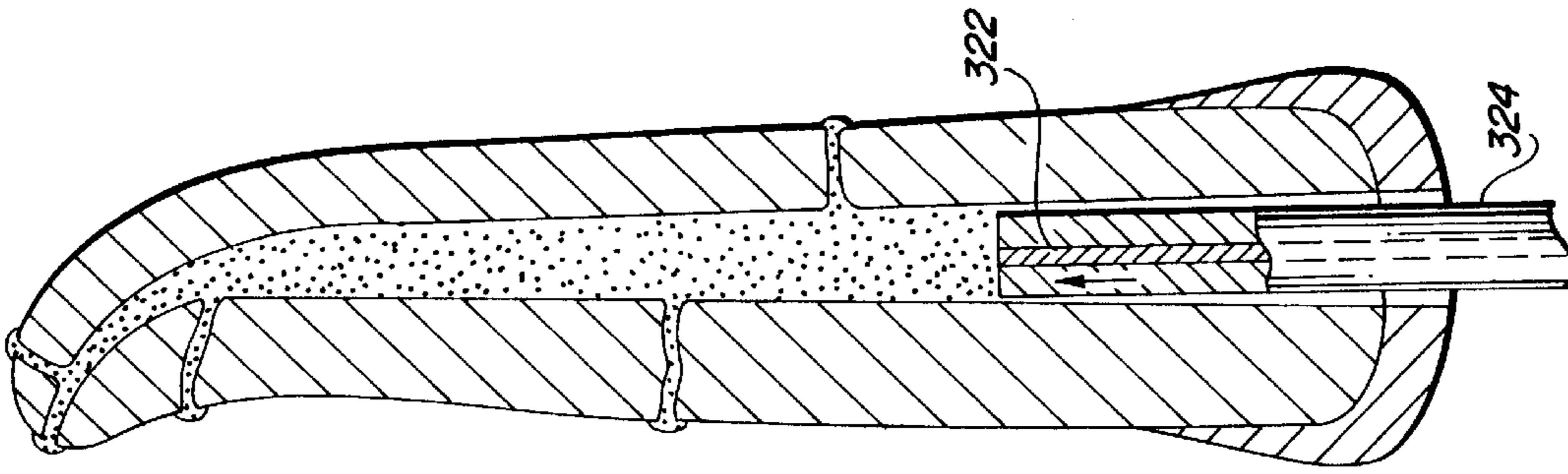
FIG. 21E
