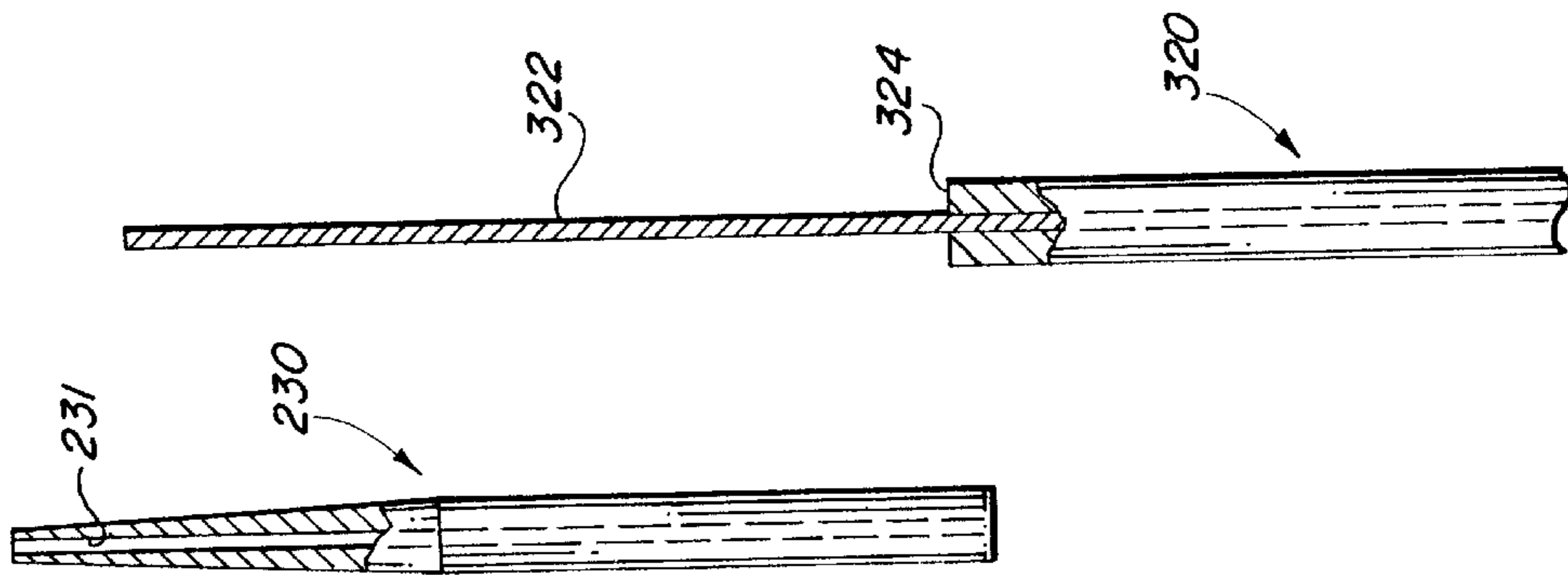
FIG. 21B
