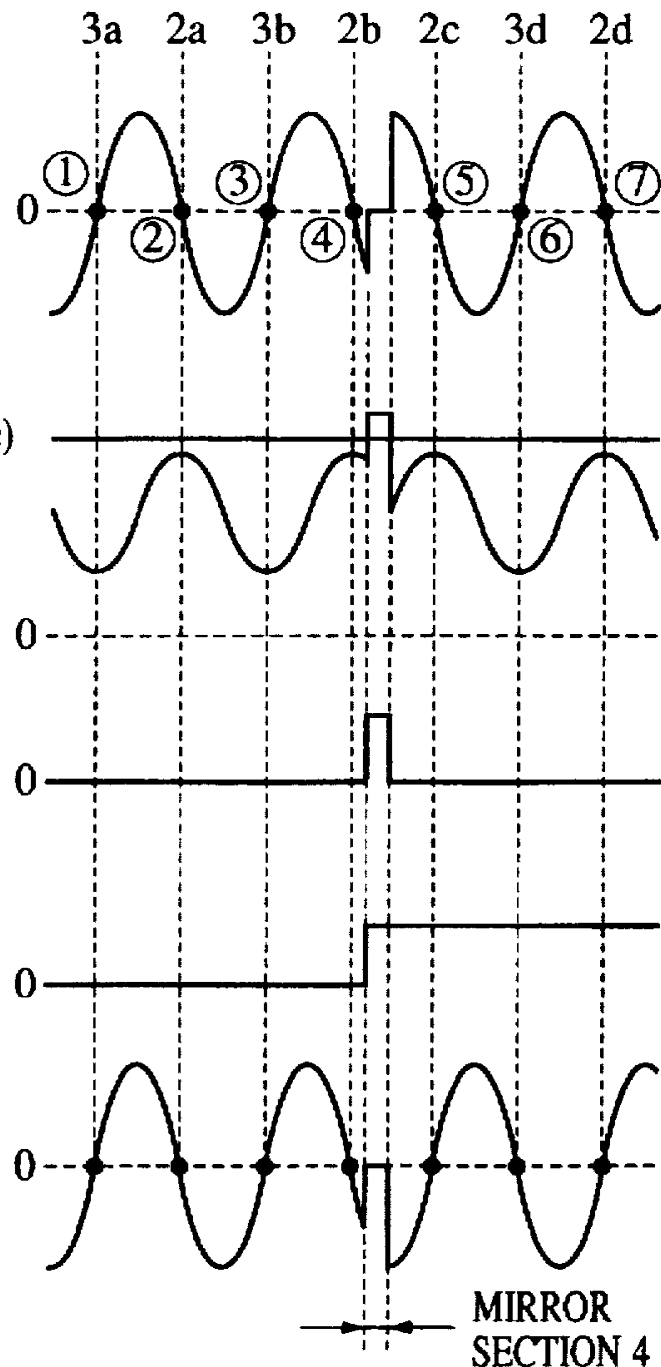
FIG. 6(b)(4) BINARY SIGNAL (d)
