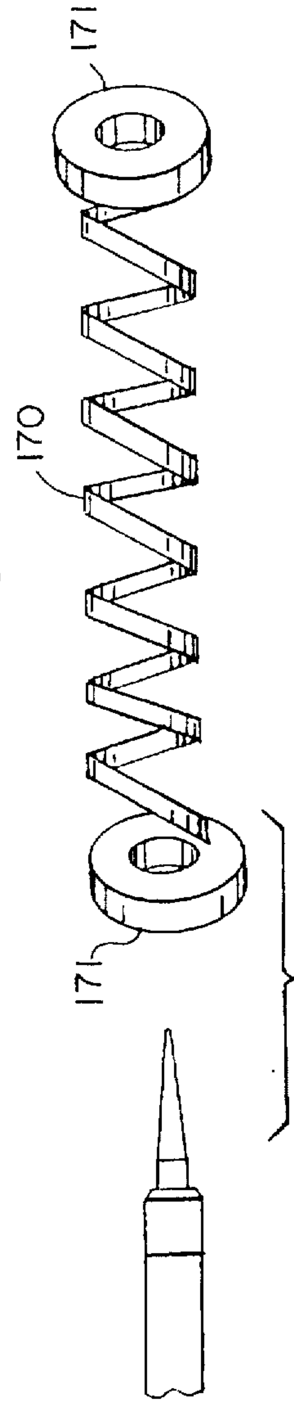
Fig. 32d
