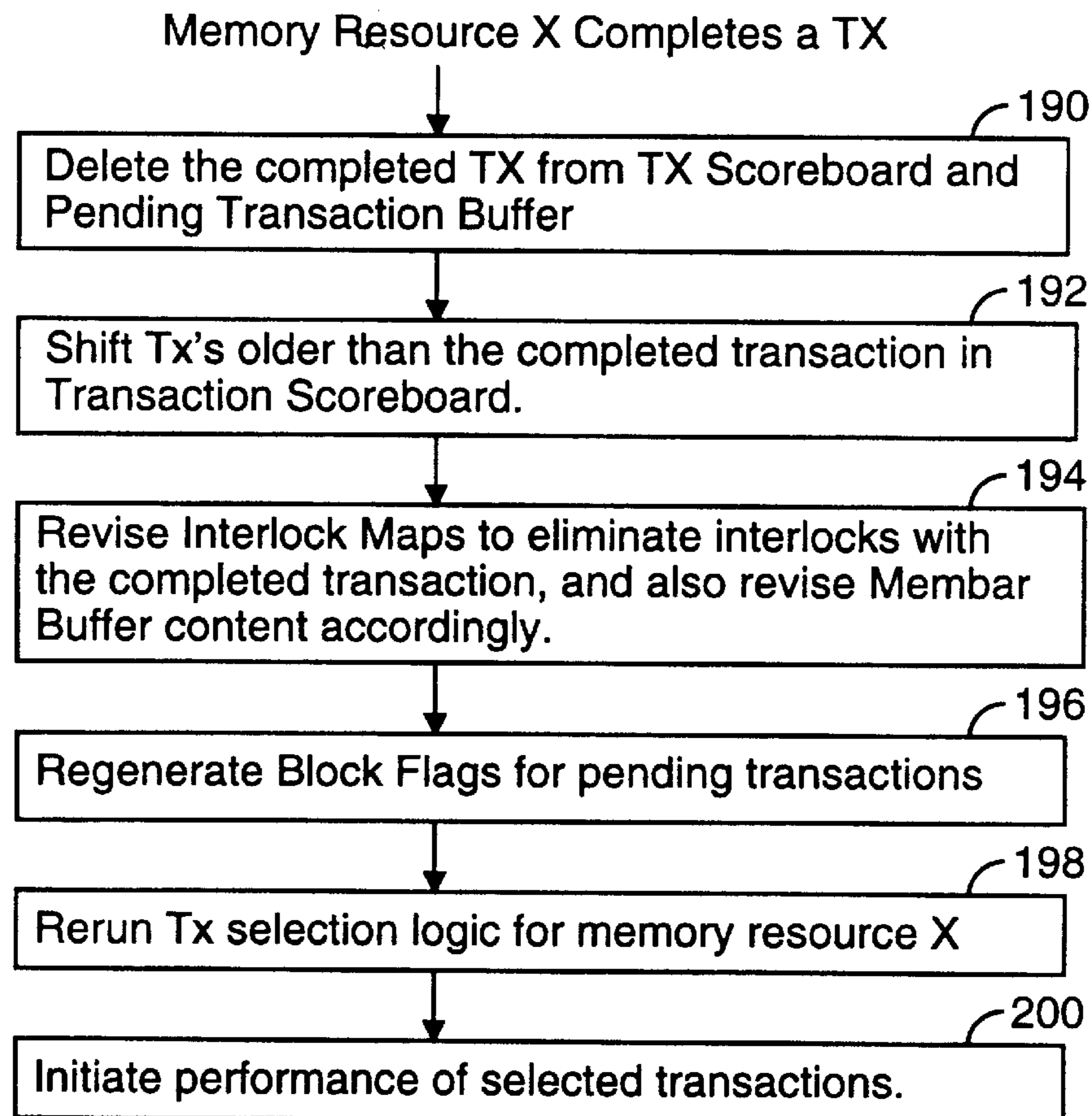
FIG. 7
