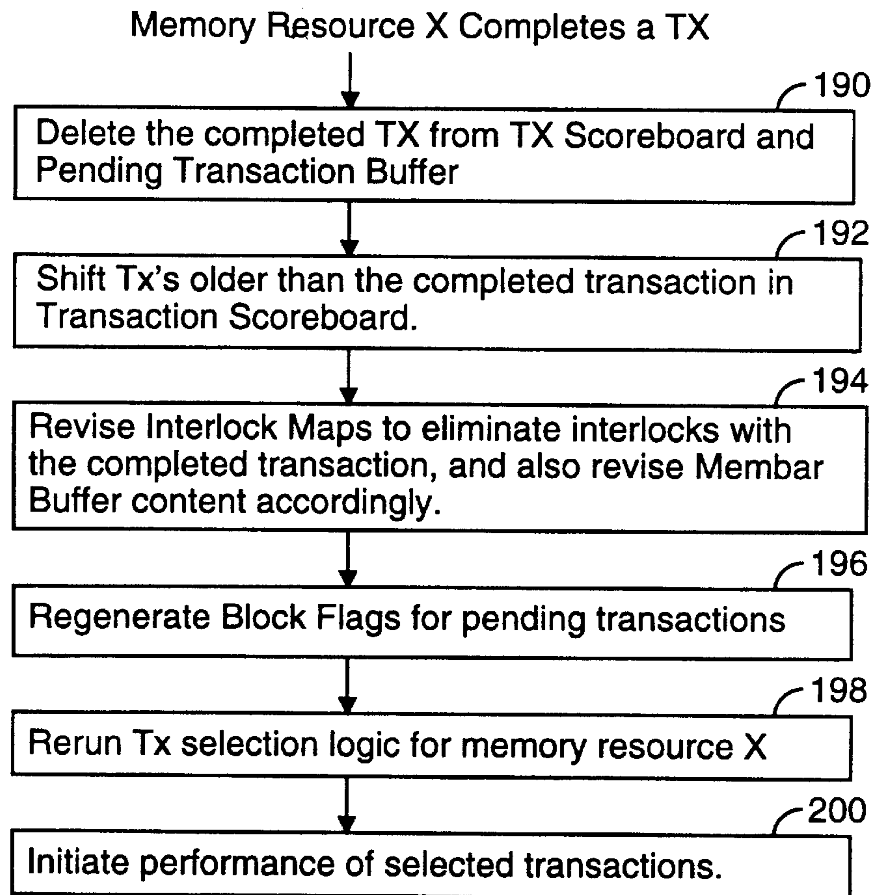
FIG. 7
