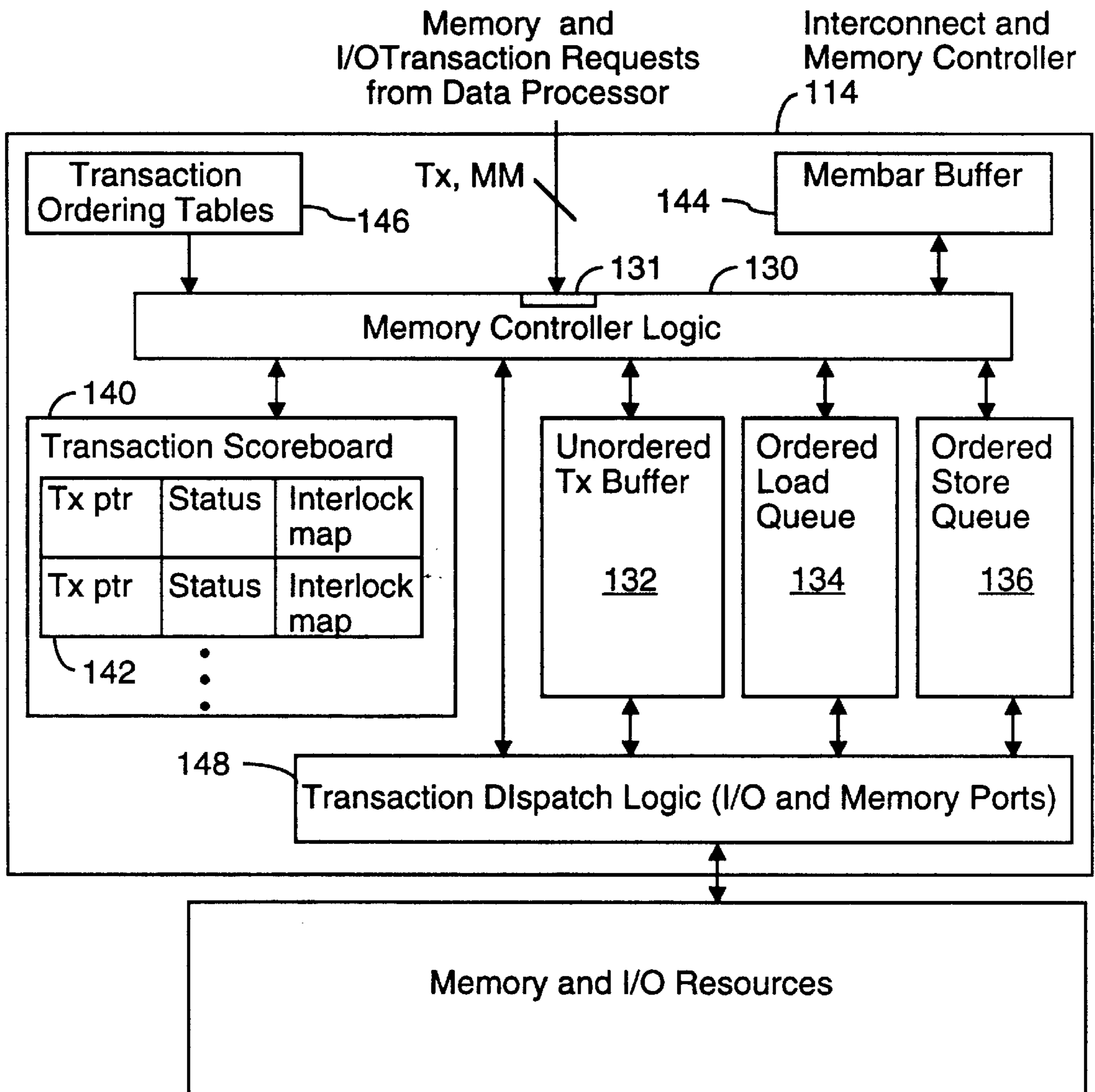
FIG. 2
