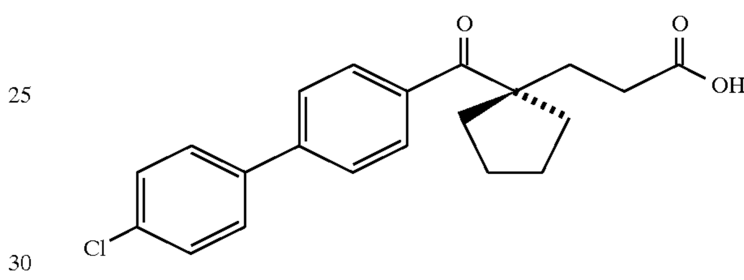
Example 241
