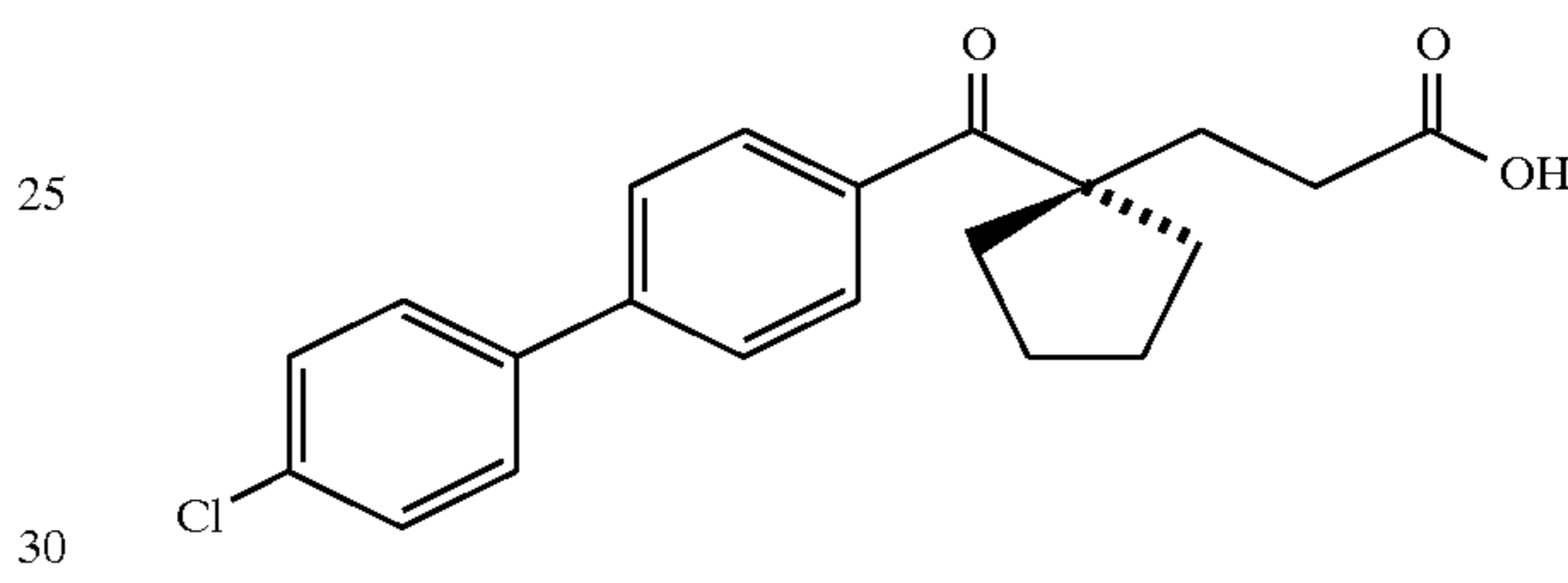
Example 241
