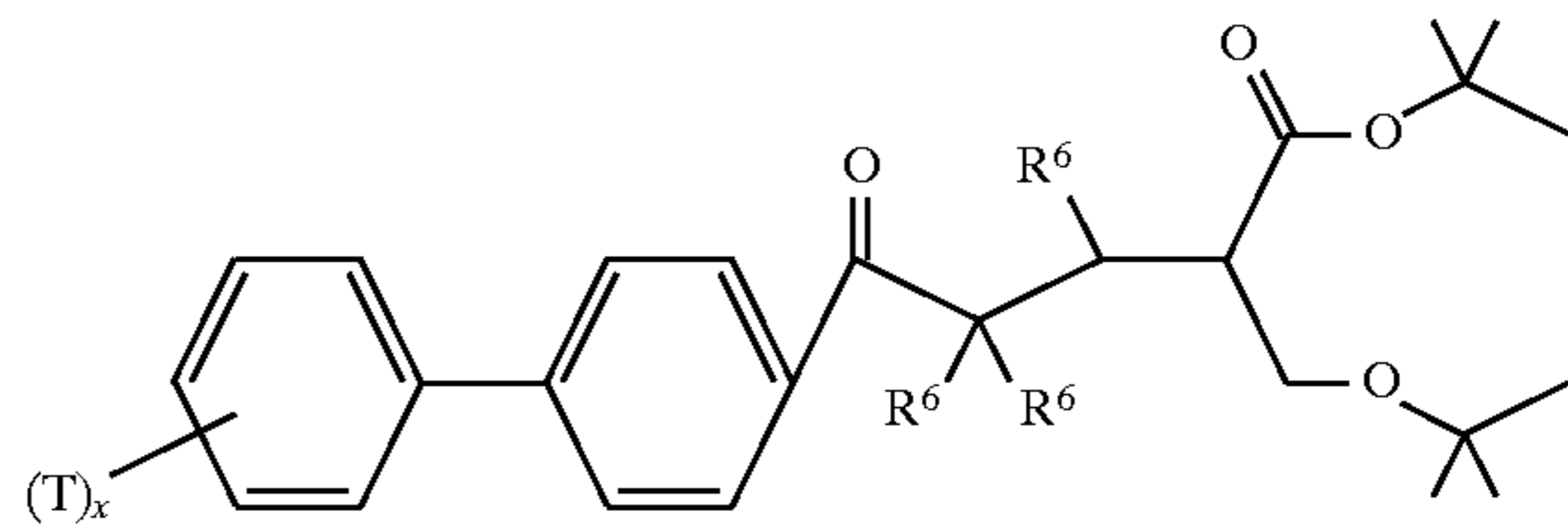
LIII
