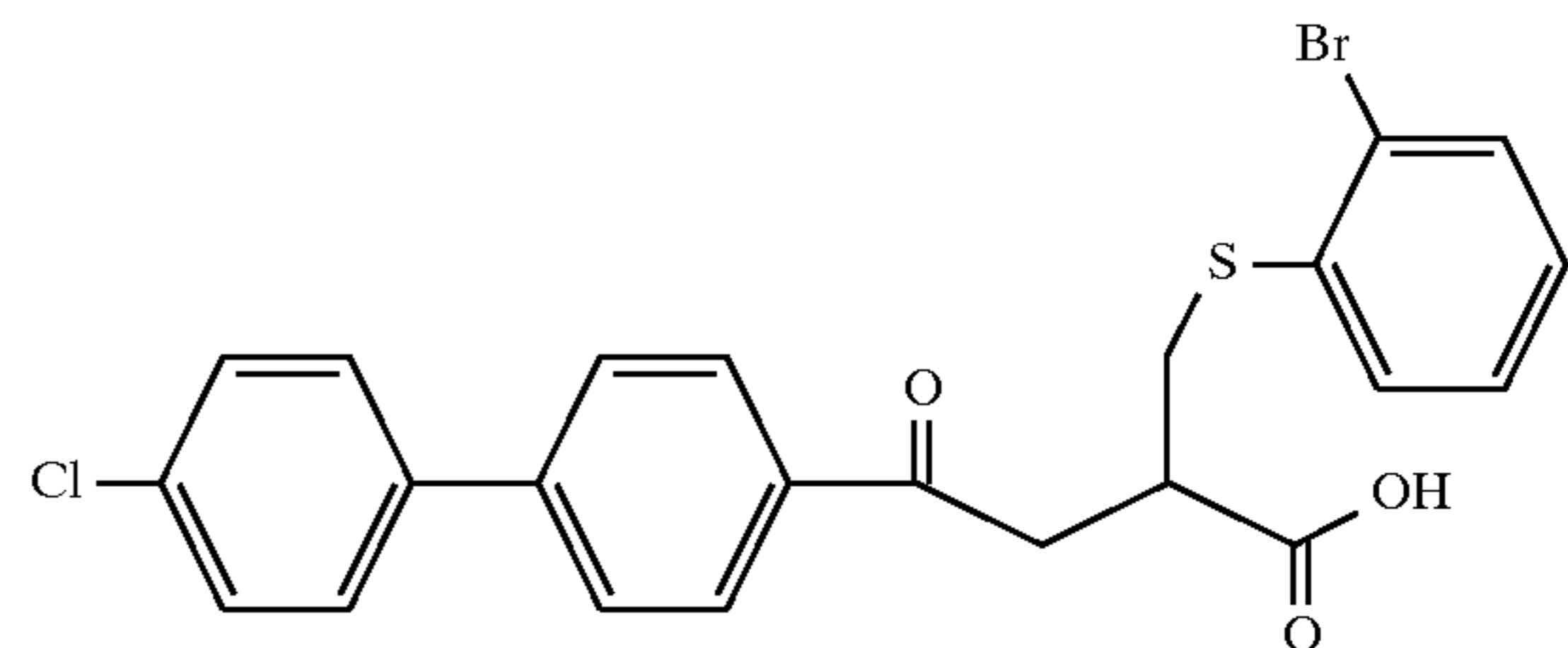
Example 149
