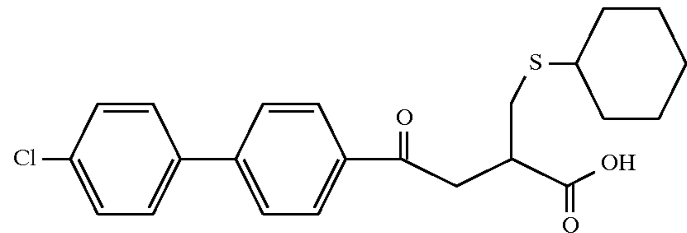
Example 144
