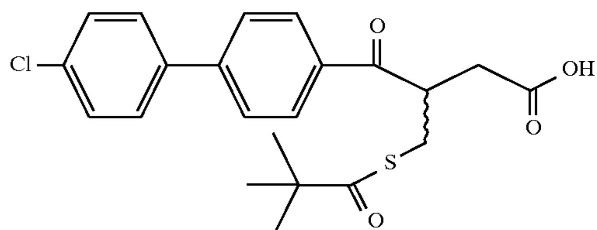
Example 180
