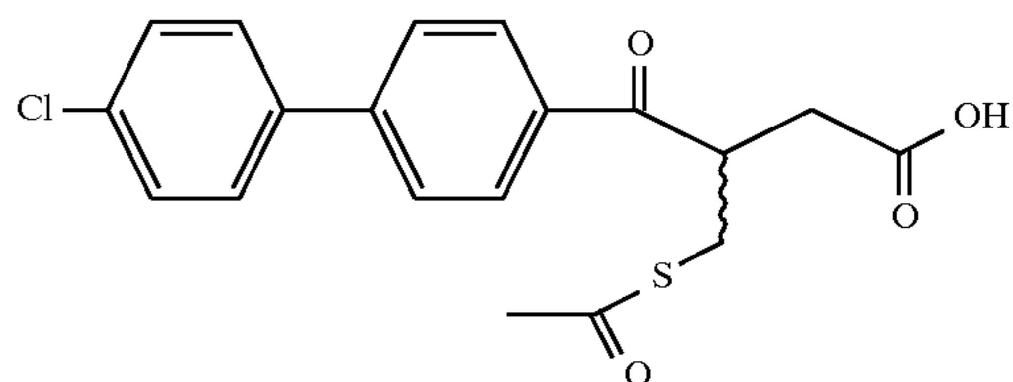
Example 182
