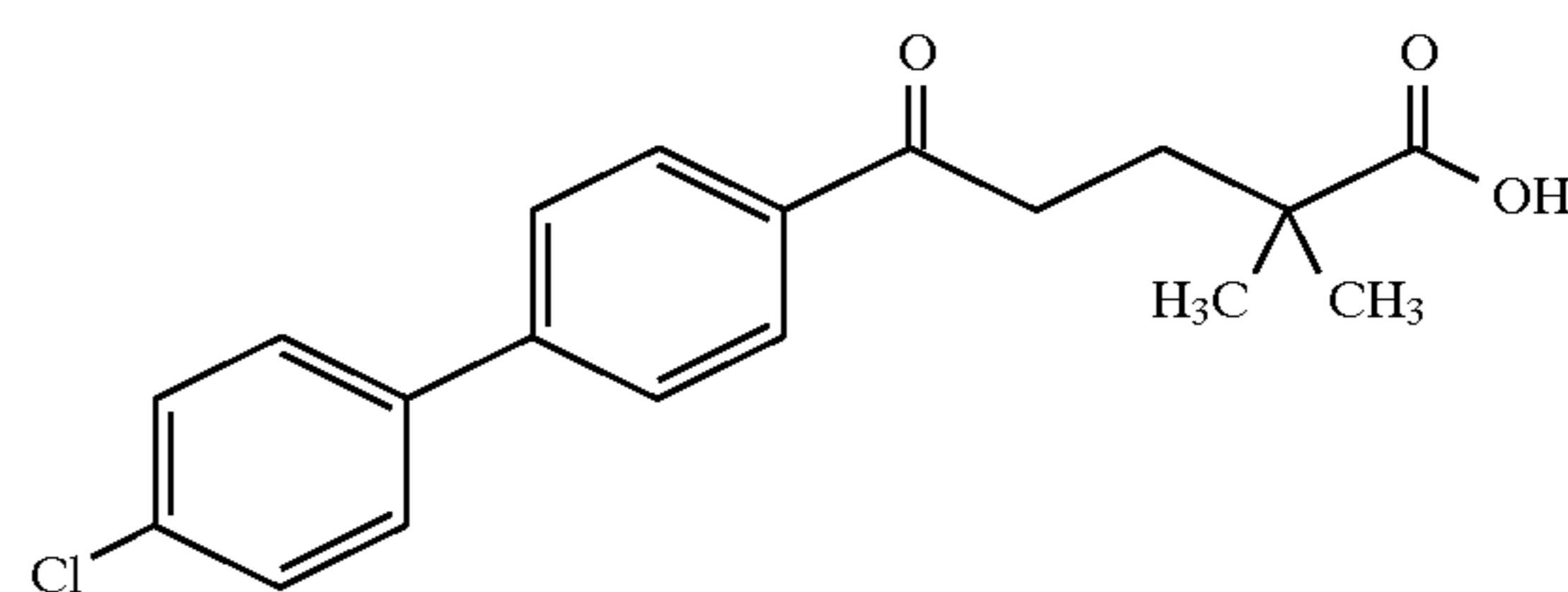
Example 238
