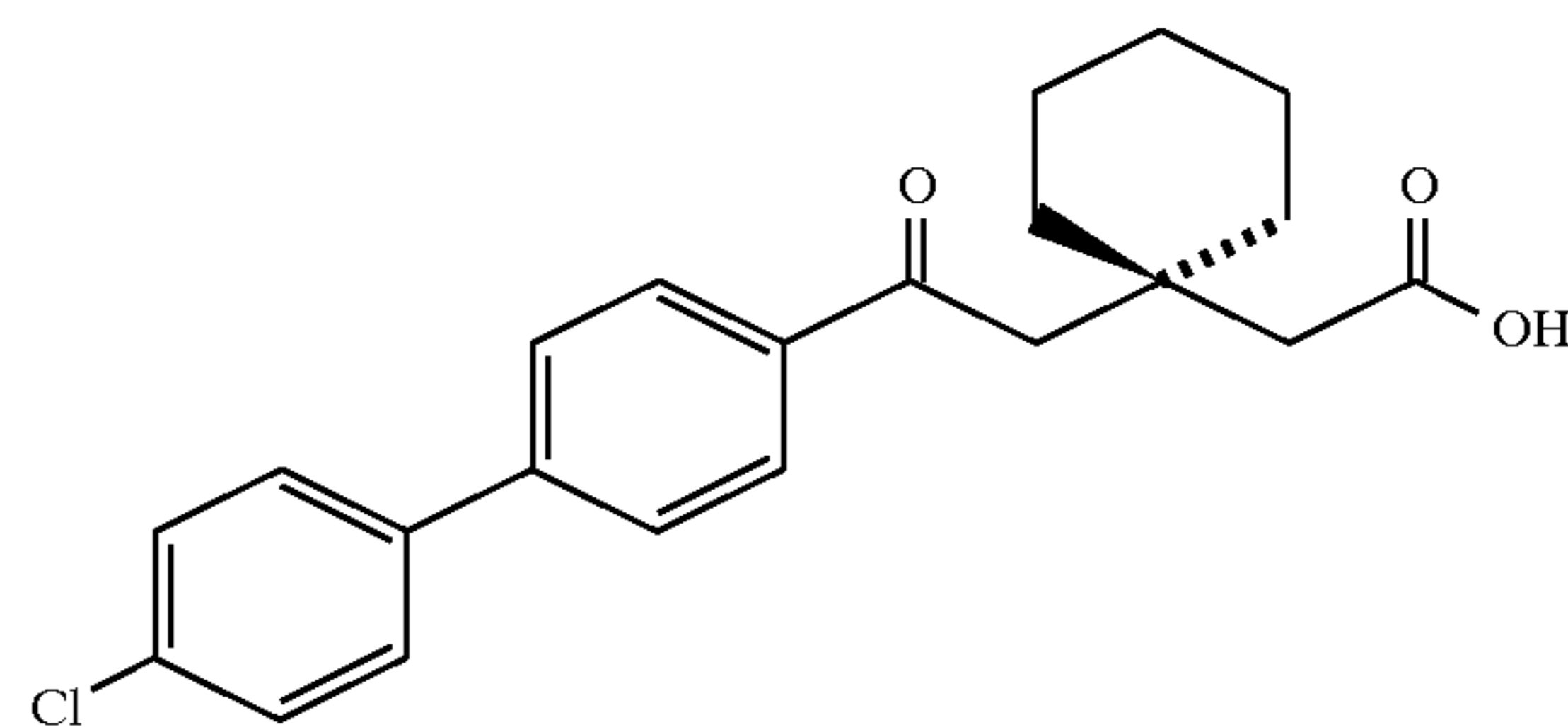
Example 240
