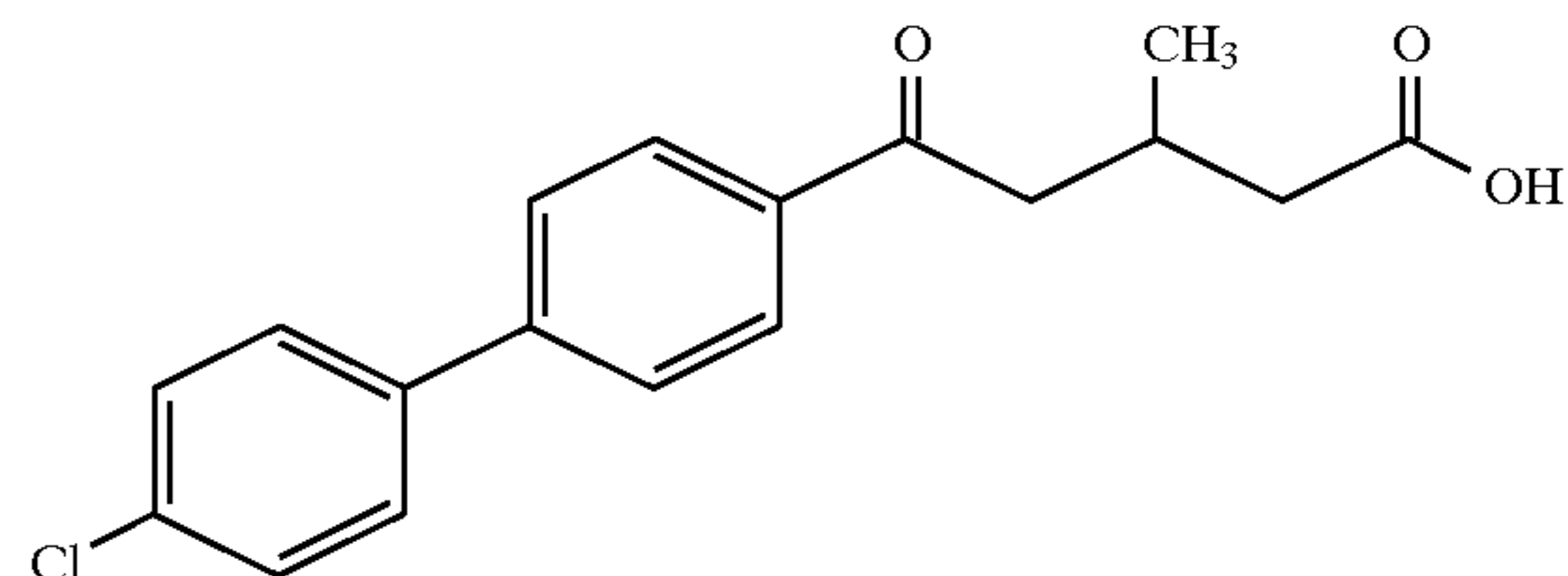
Example 235
