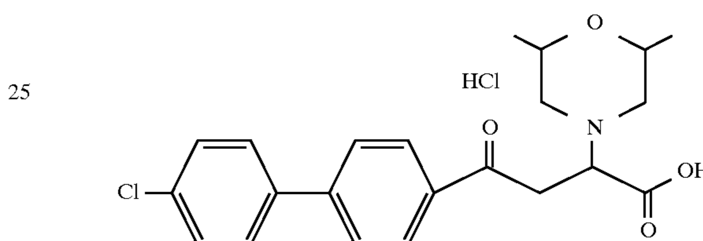
Example 186
