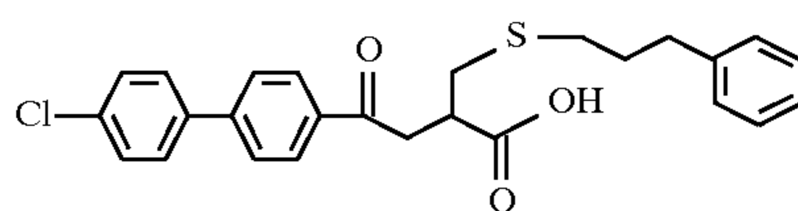
Example 137
