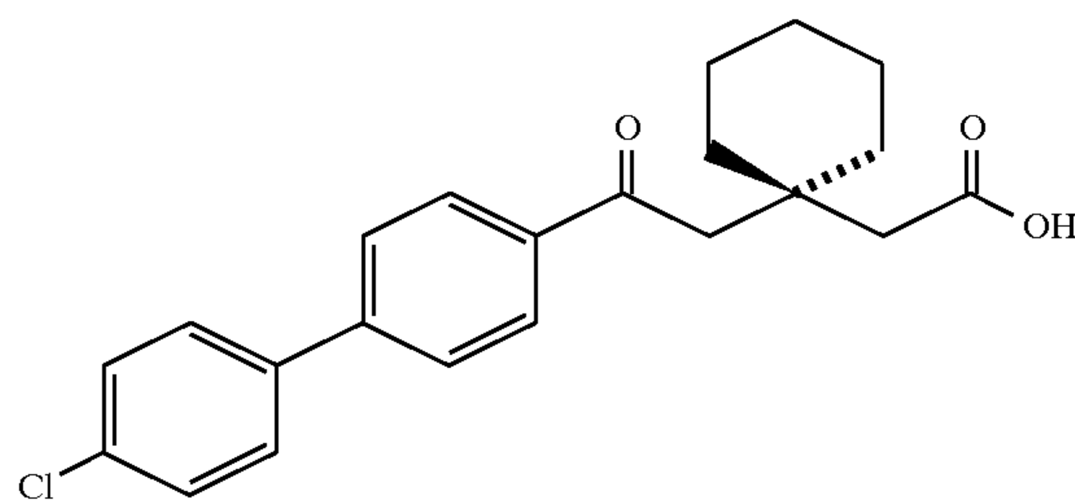
Example 240
