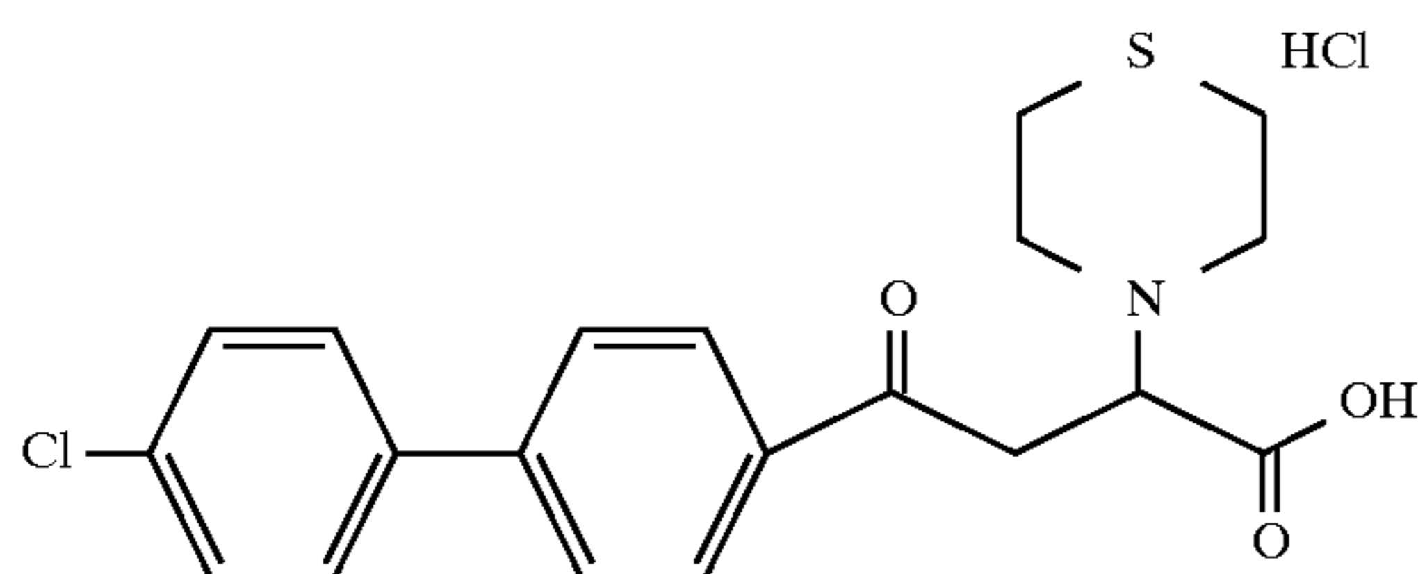
Example 184
