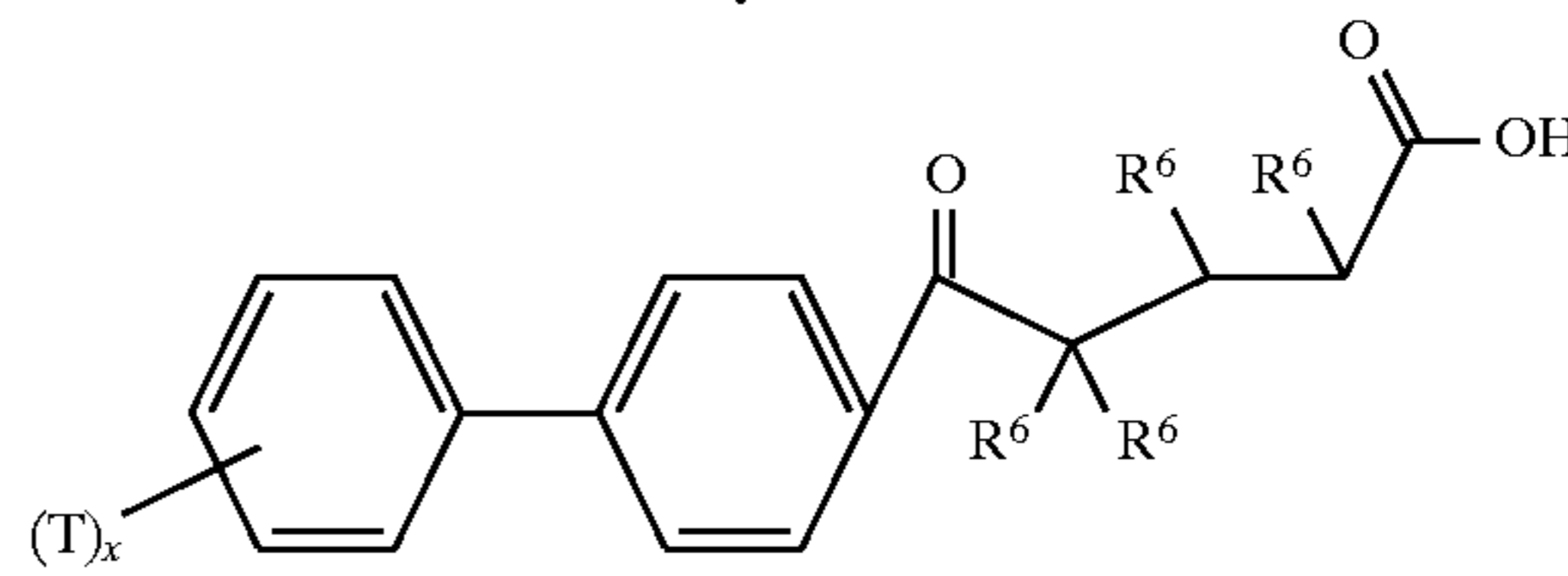
1-L-1
