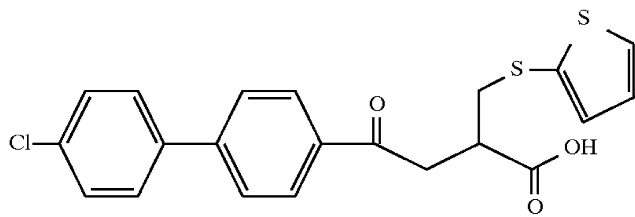
Example 129
