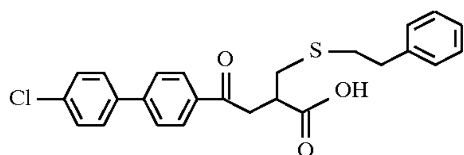
Example 135
