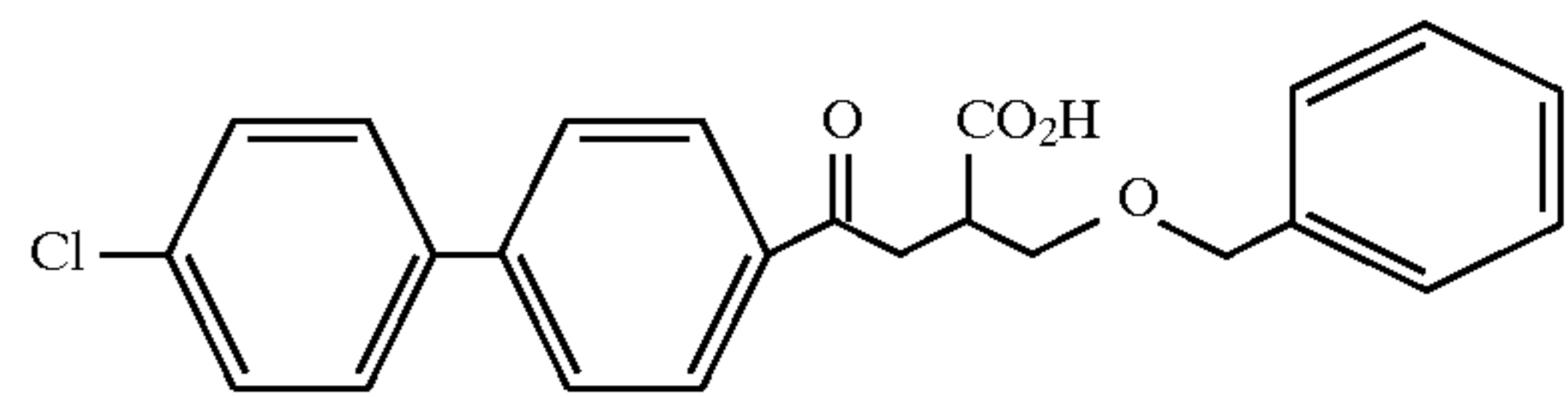
Example 196
