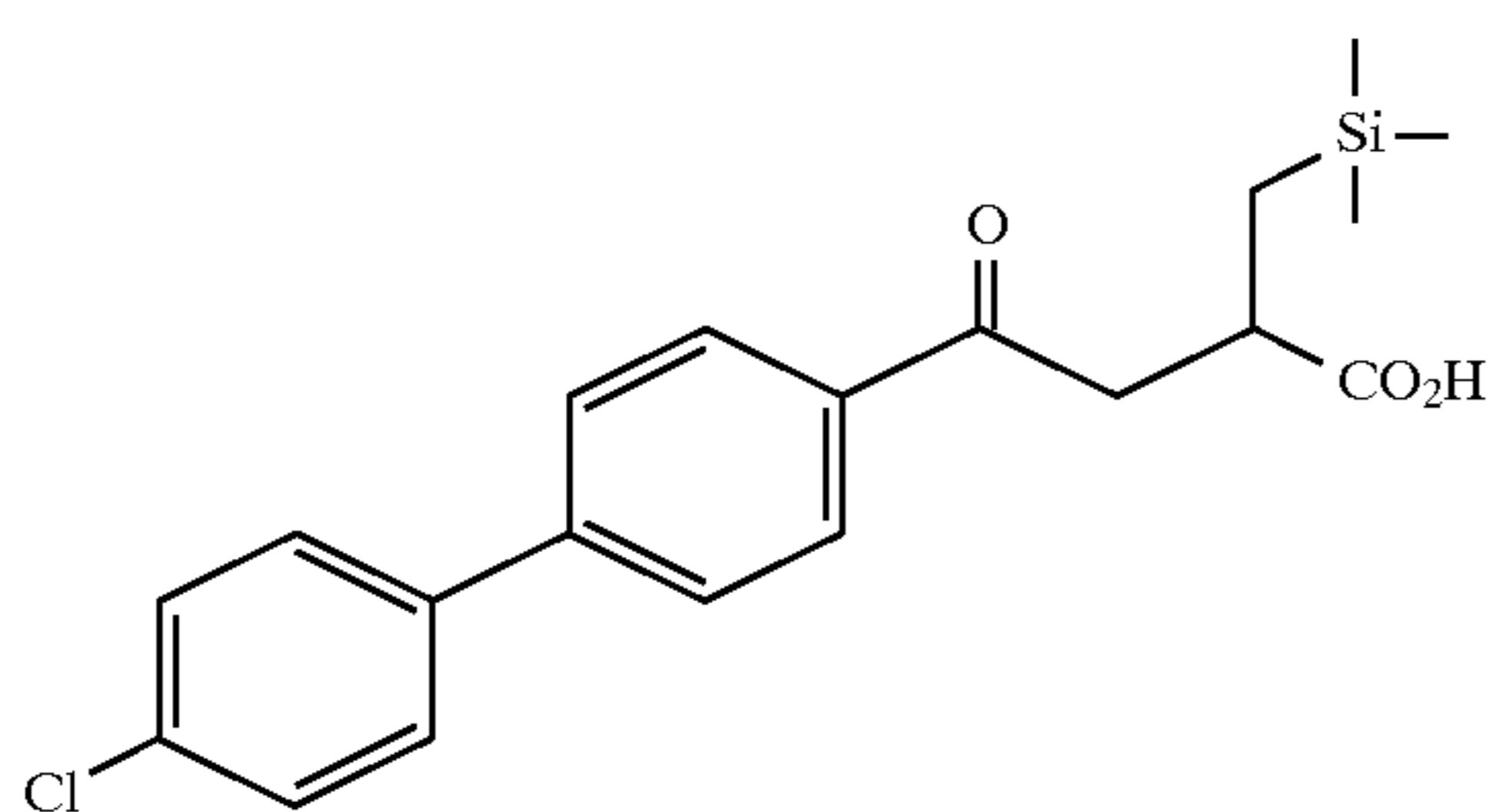
Example 188
