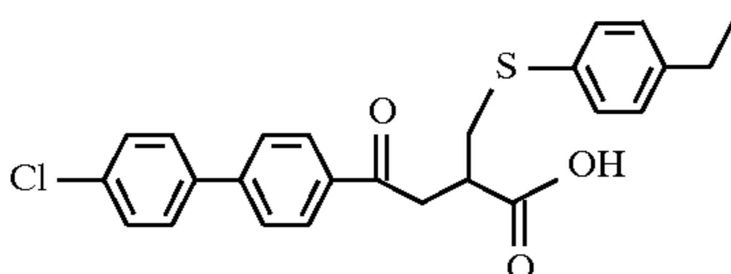
Example 142
