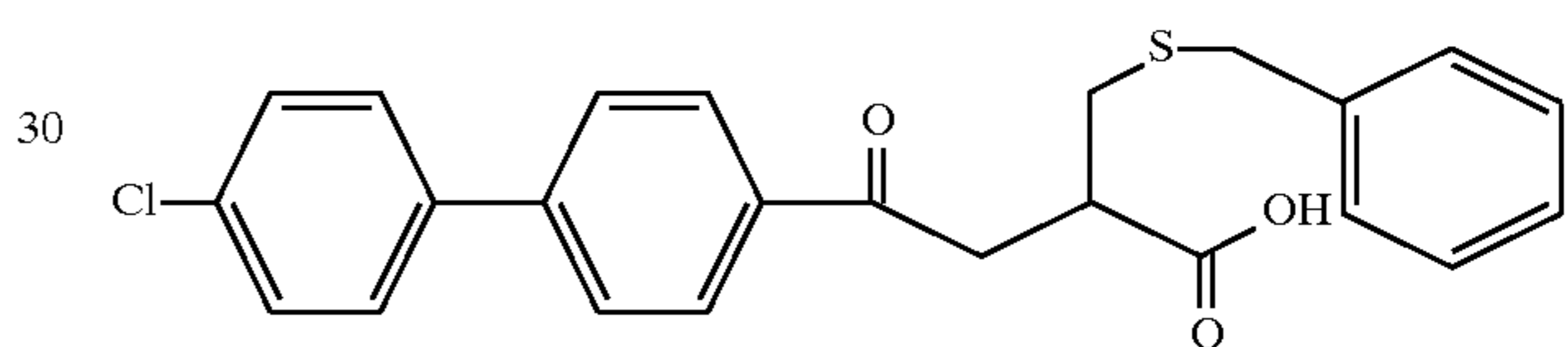
Example 133
