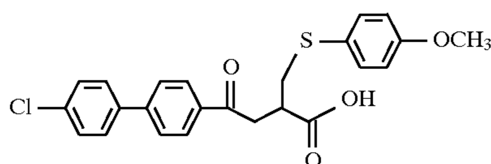
Example 136
