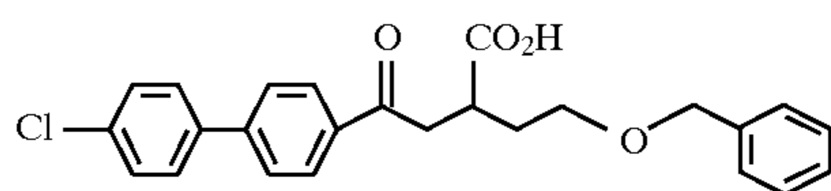
Example 187
