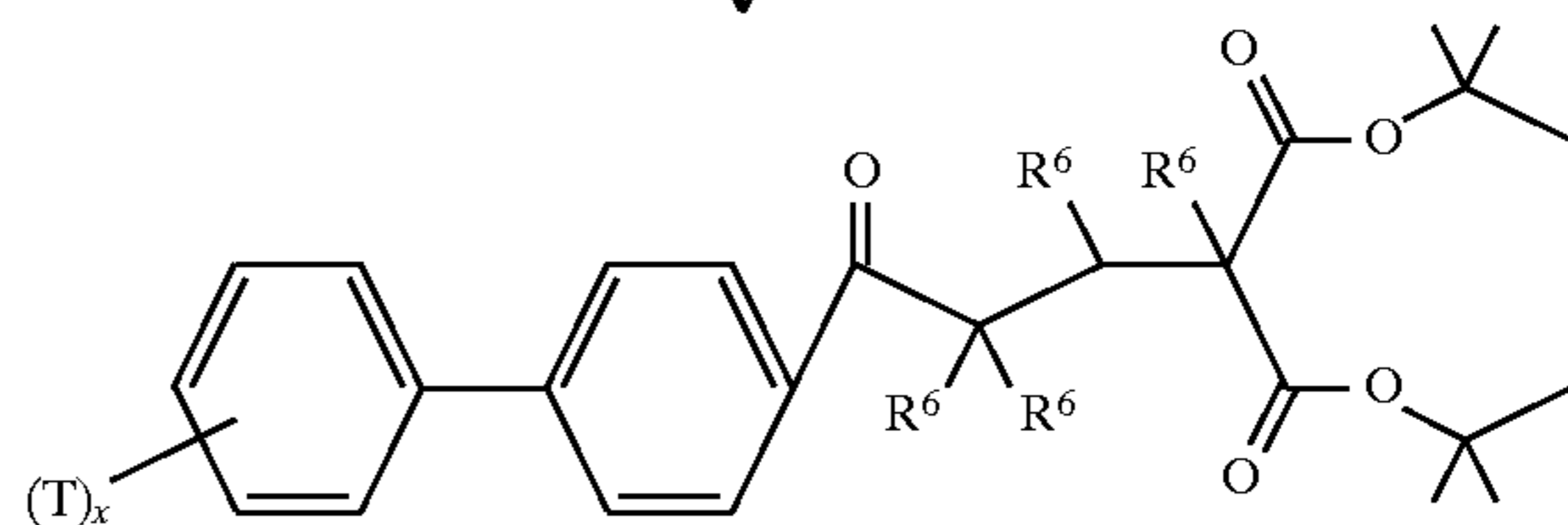
LIV
