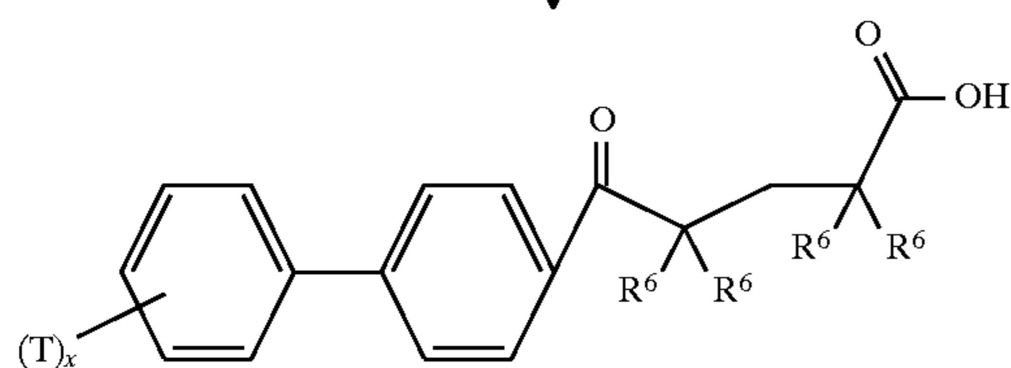
1-L-3
