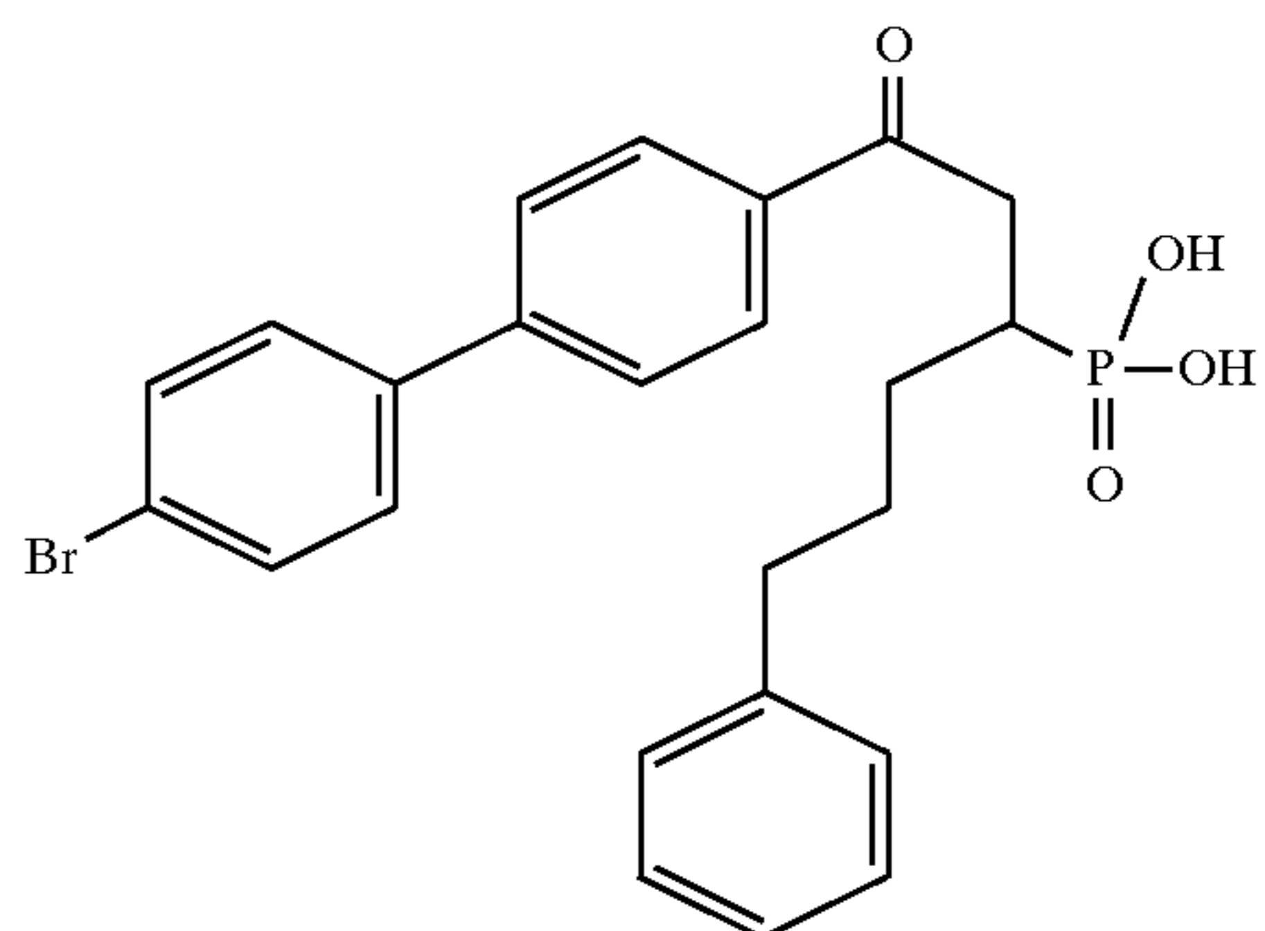
Example 246
