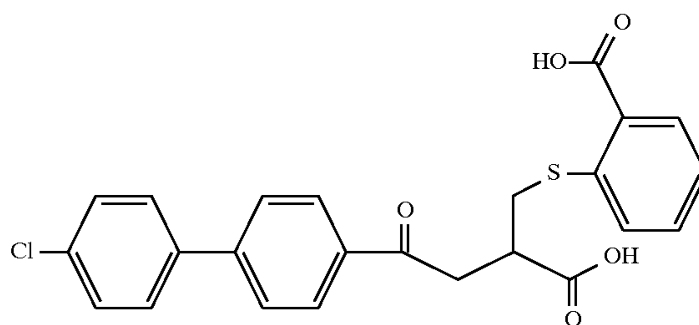
Example 163
