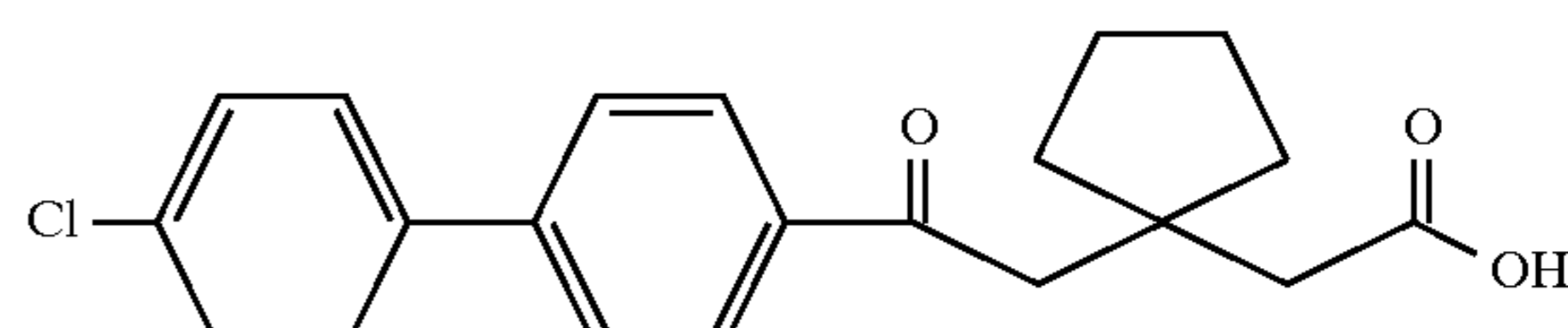
Example 234
