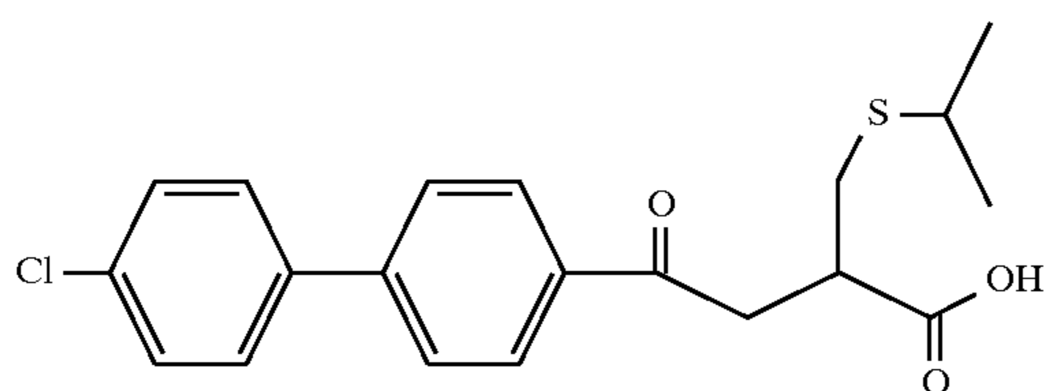
Example 169
