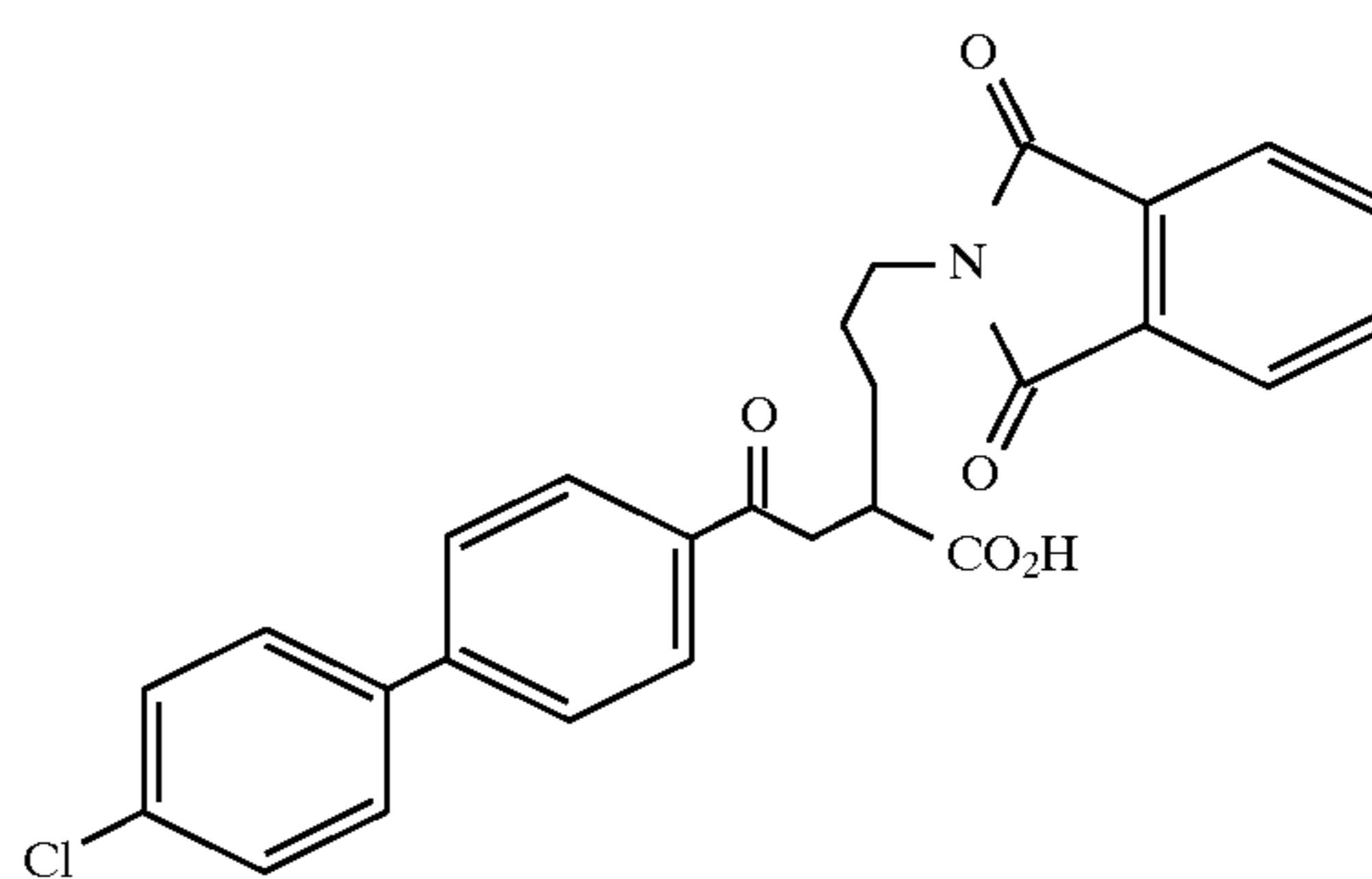
Example 189
