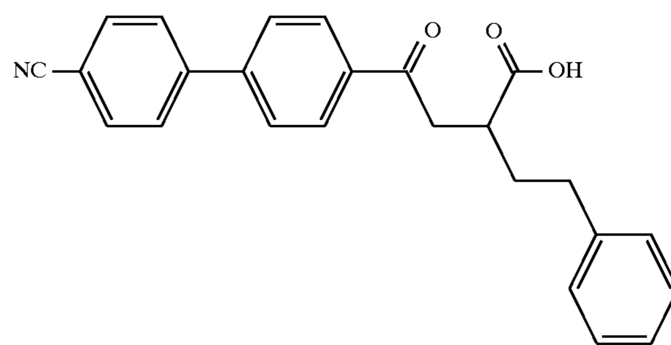
Example 101
