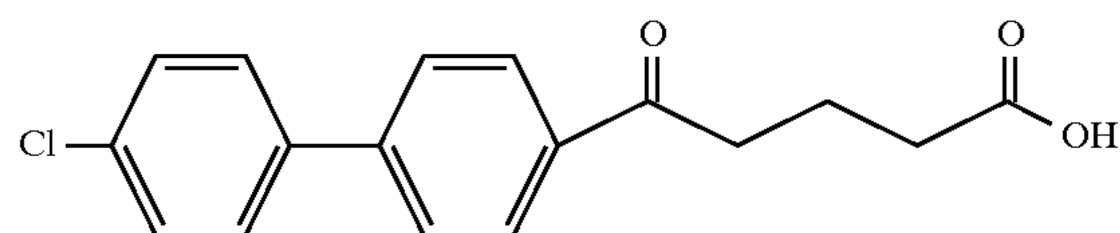
Example 233
