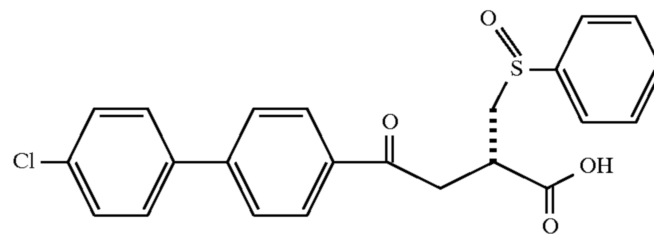
Example 128
