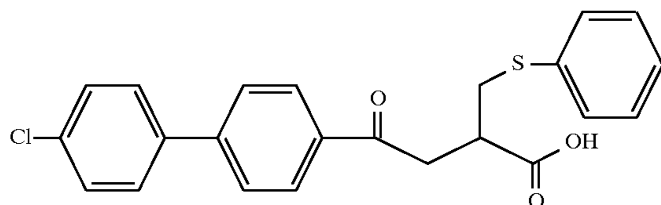
Example 121
