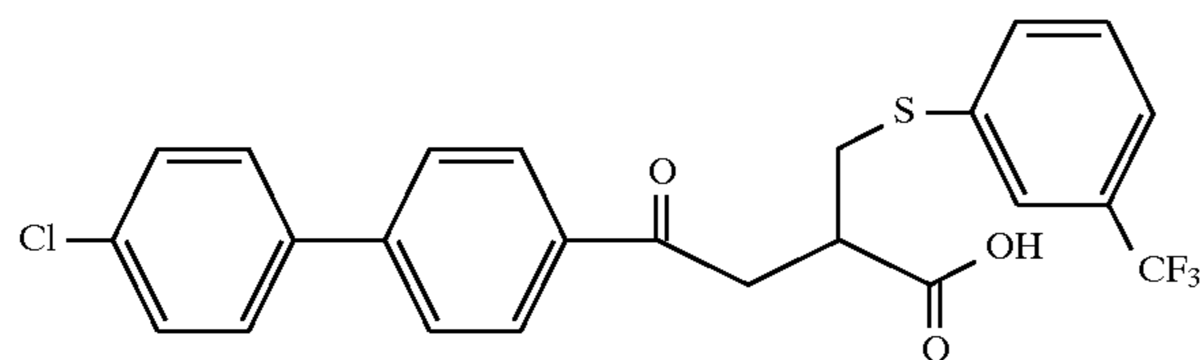
Example 166
