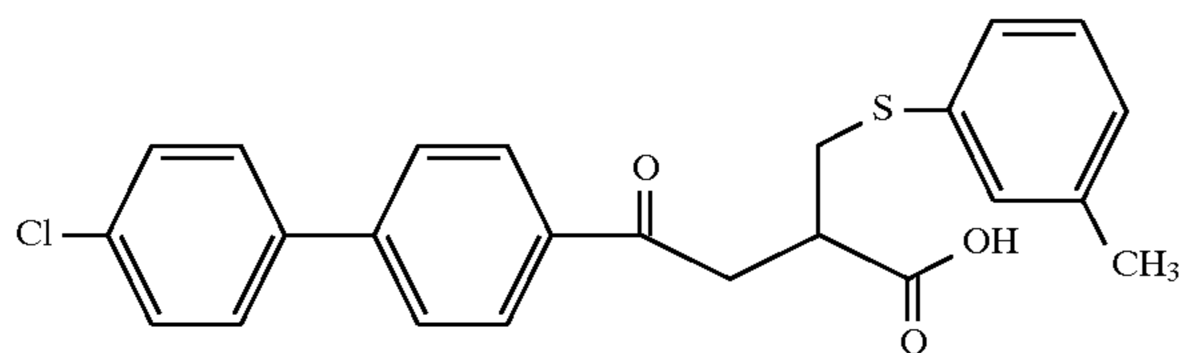
Example 161
