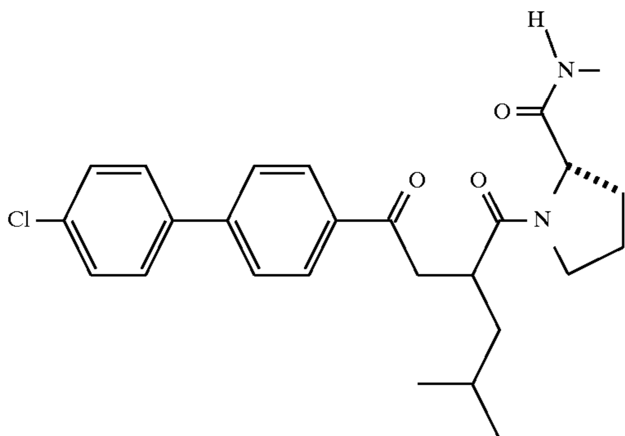
Example 247
