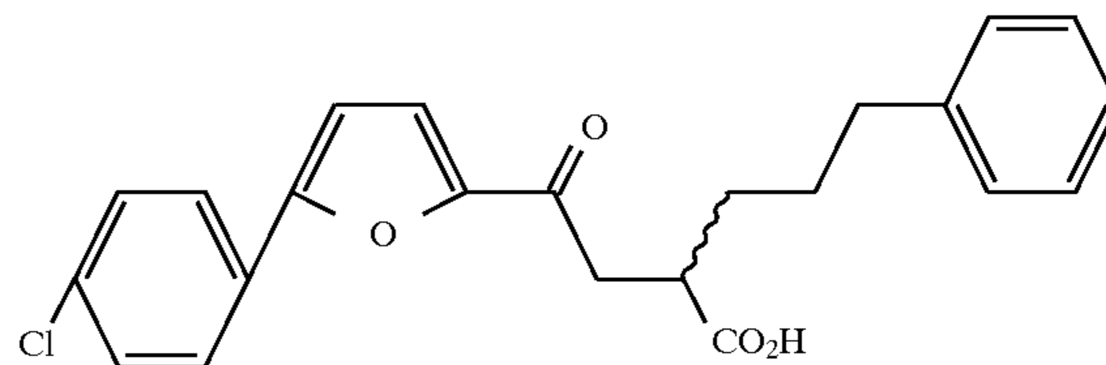
Example 251
