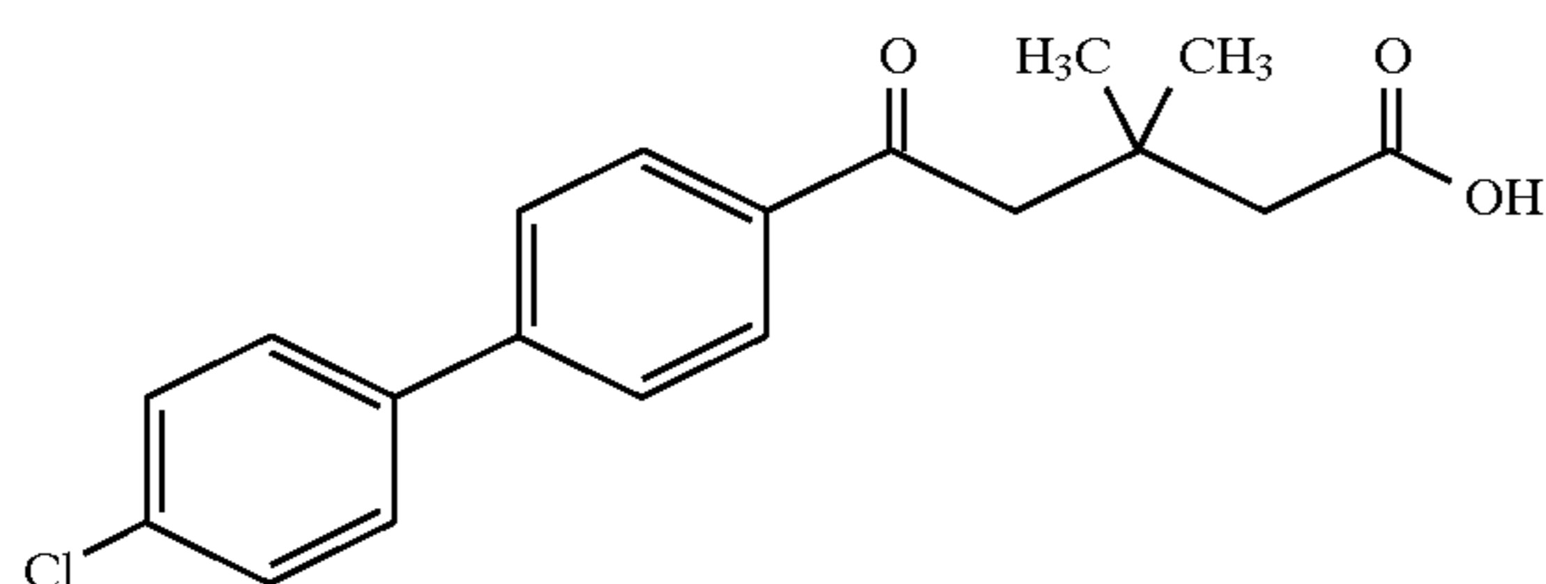
Example 236
