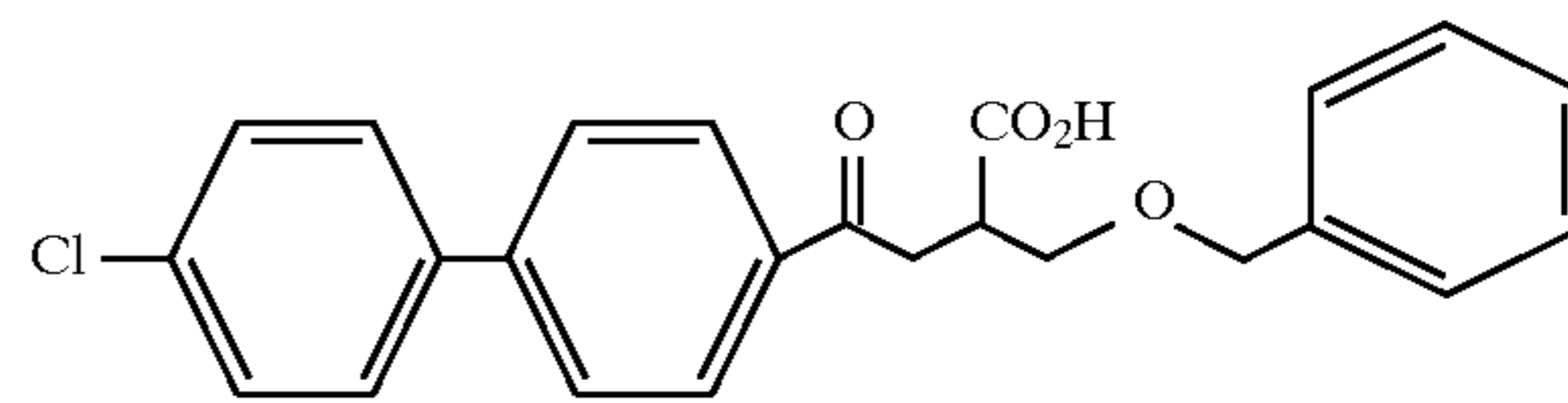
Example 196
