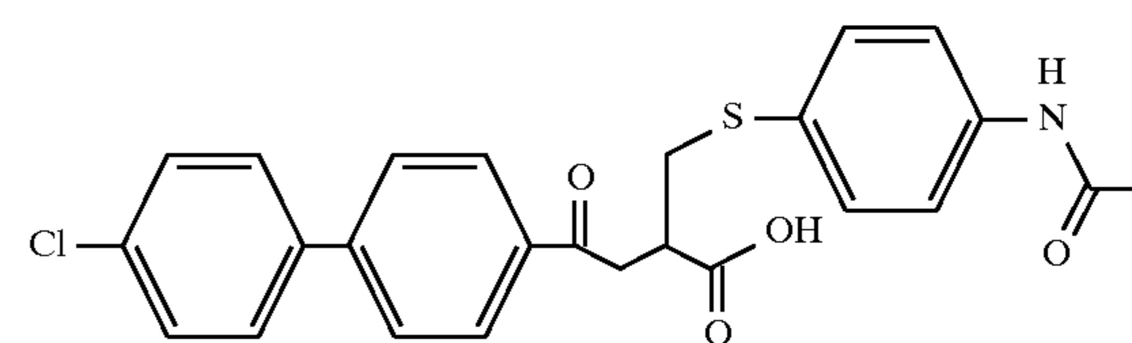
Example 153
