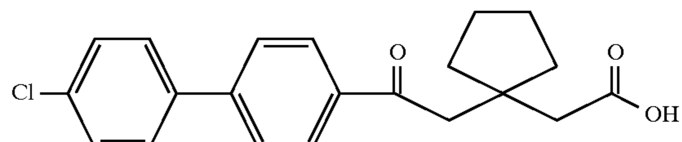
Example 234
