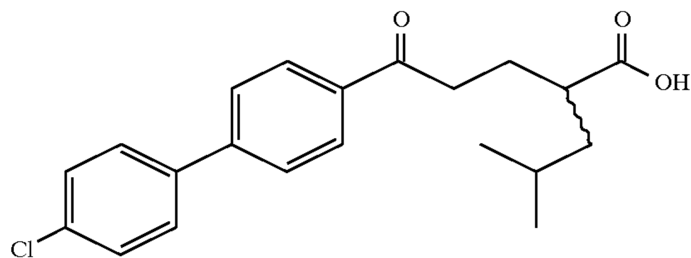
Example 239
