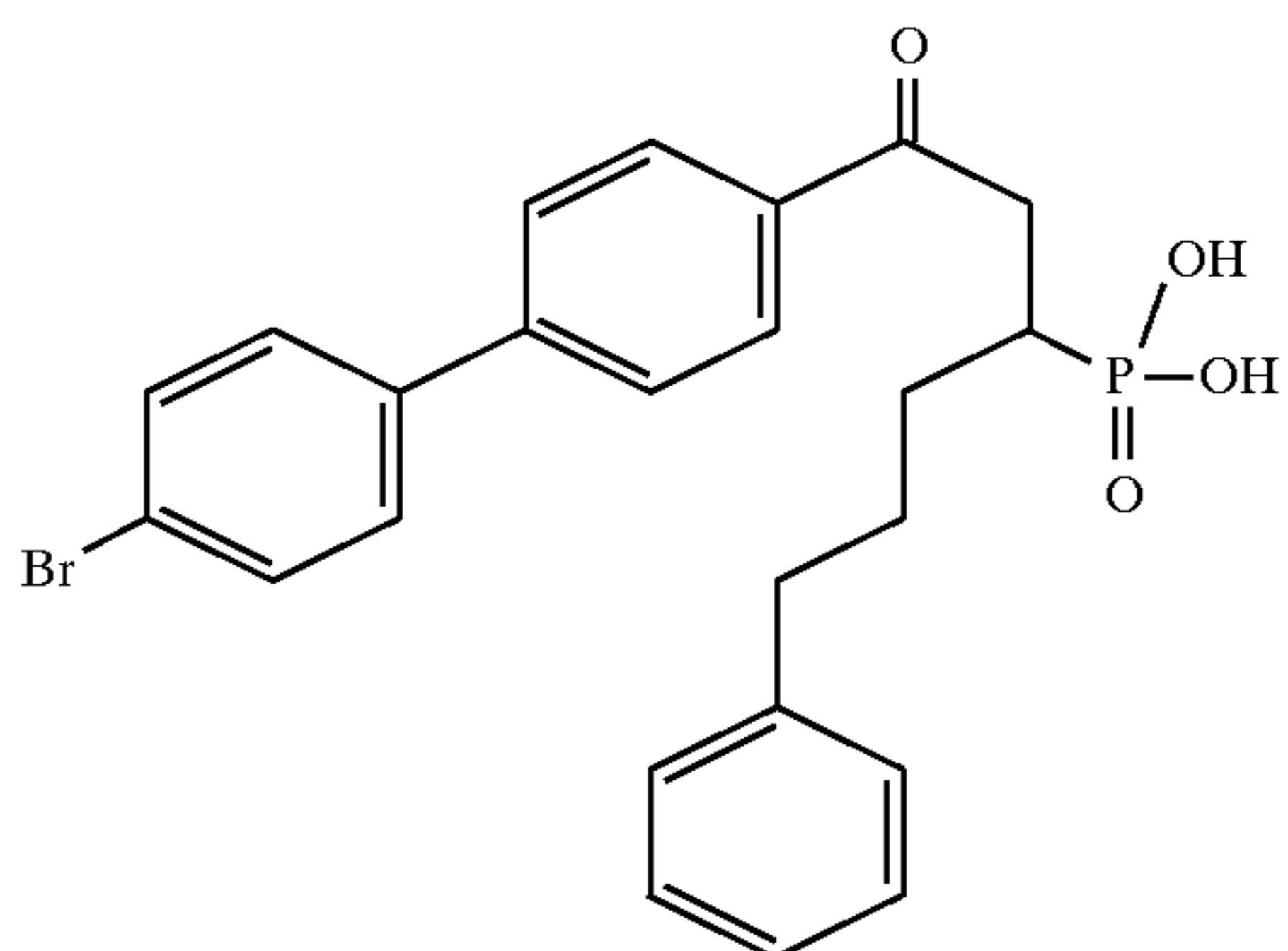
Example 246
