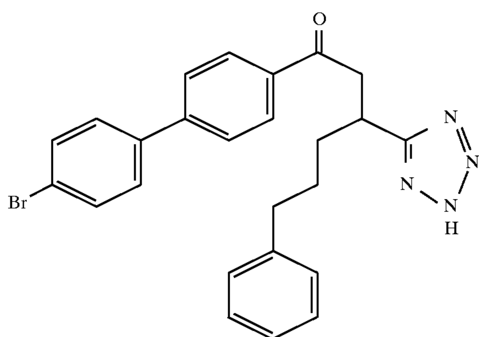
Example 245
