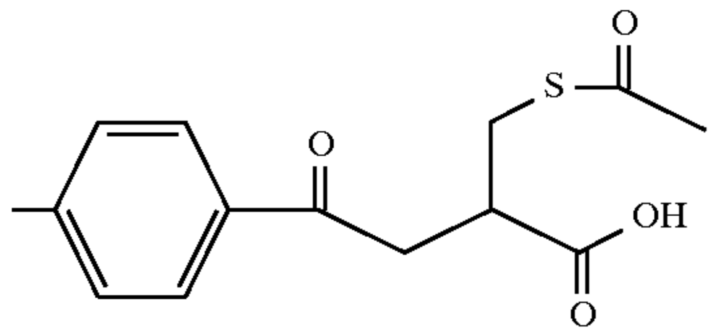
Example 178
