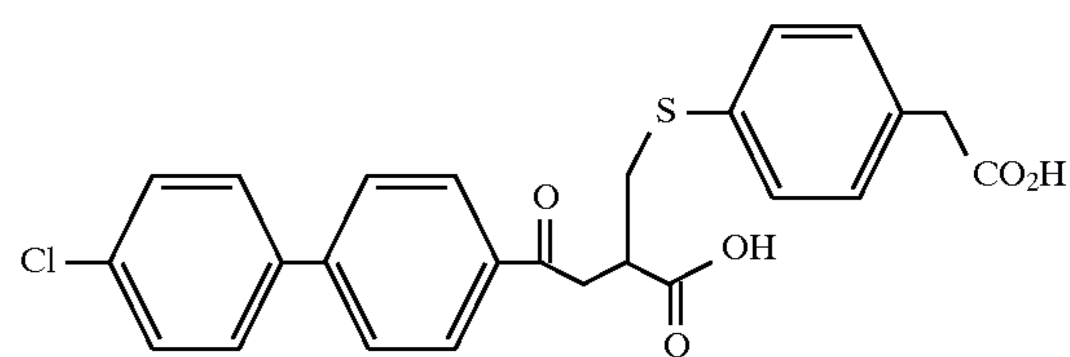
Example 168
