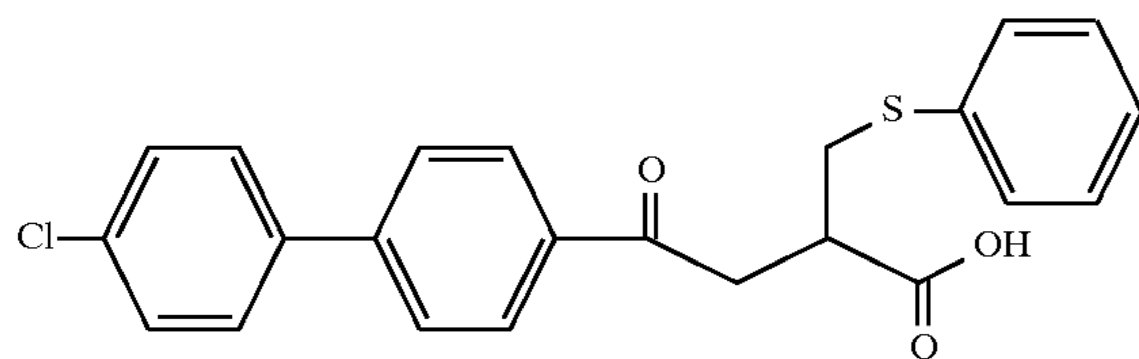
Example 121
