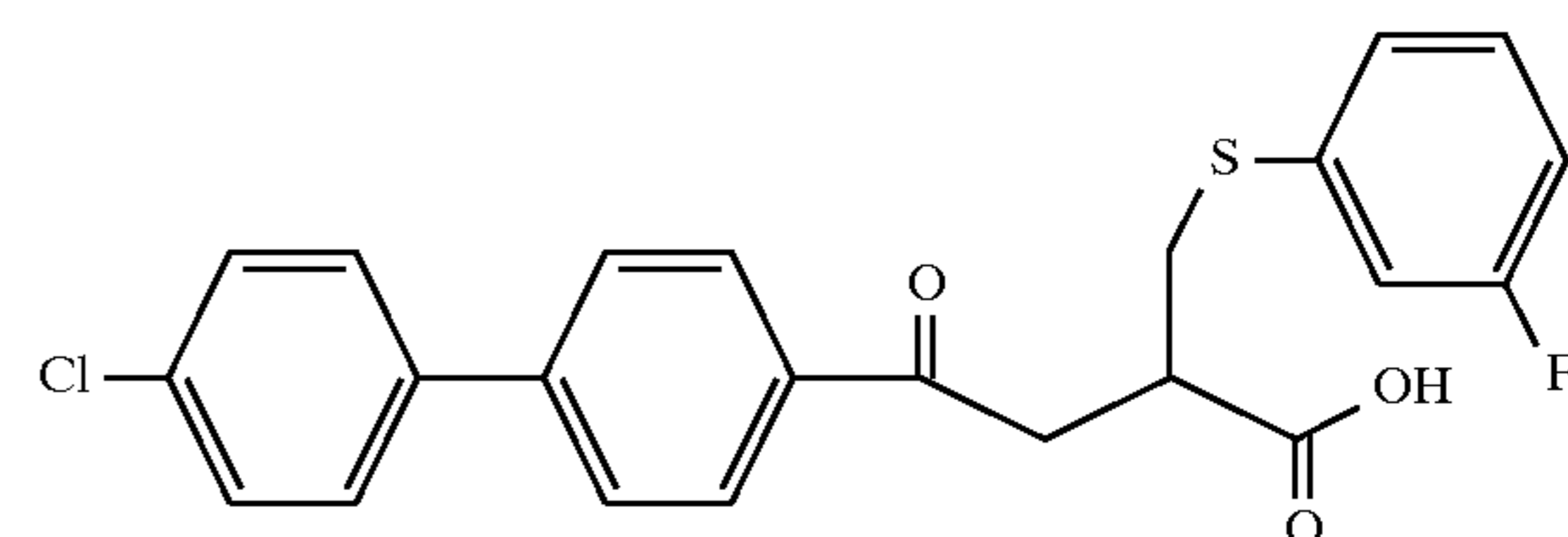
Example 173
