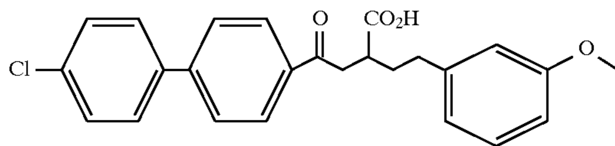
Example 116
