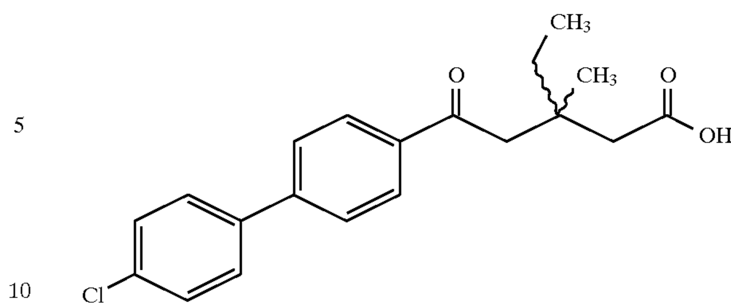
Example 237
