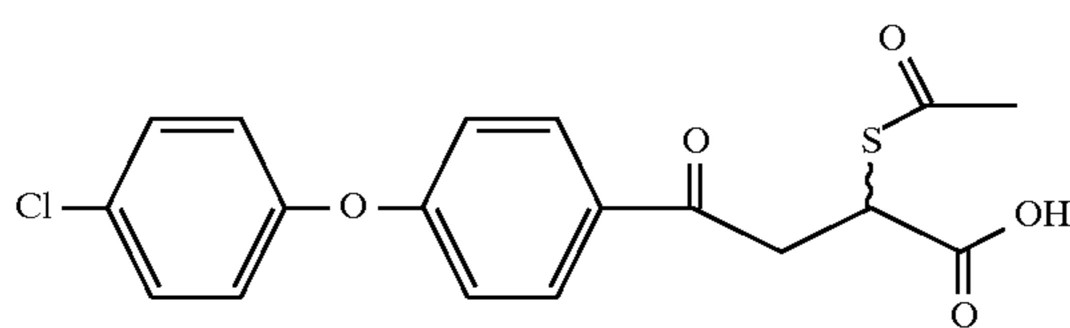
Example 183
