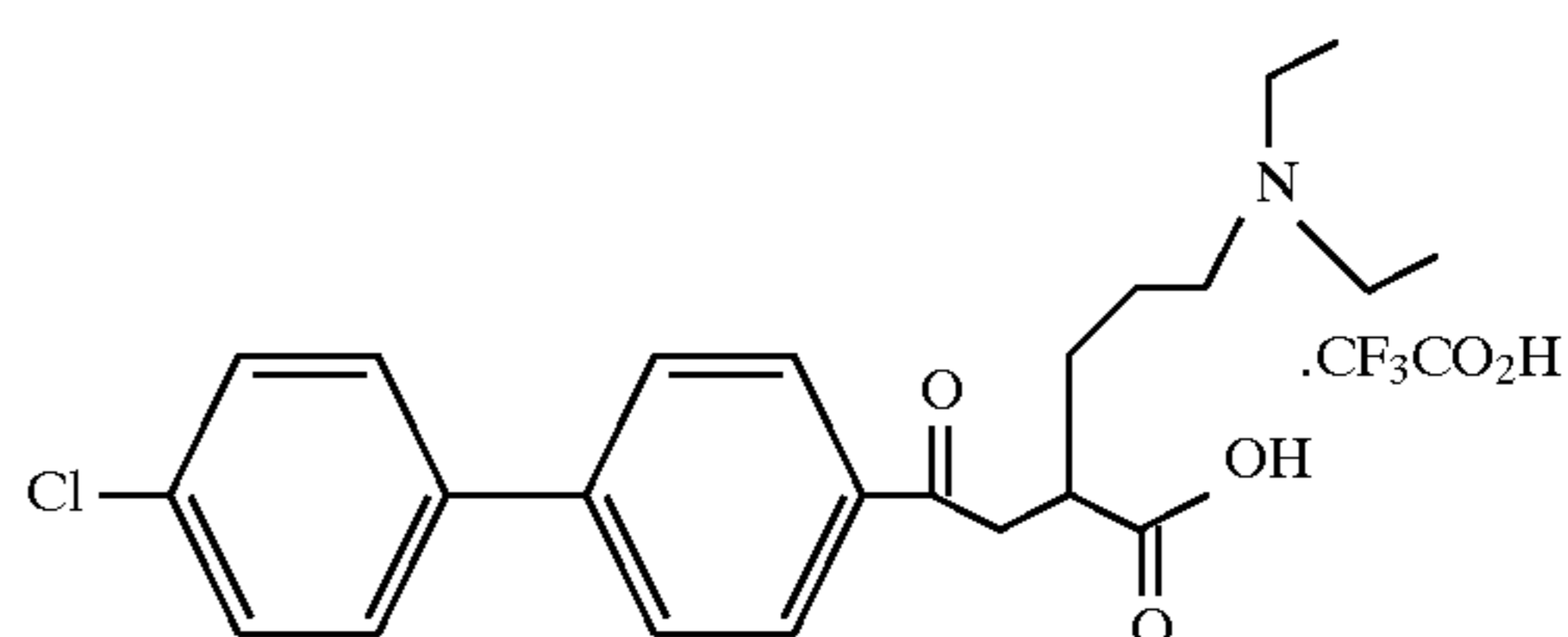
Example 192
