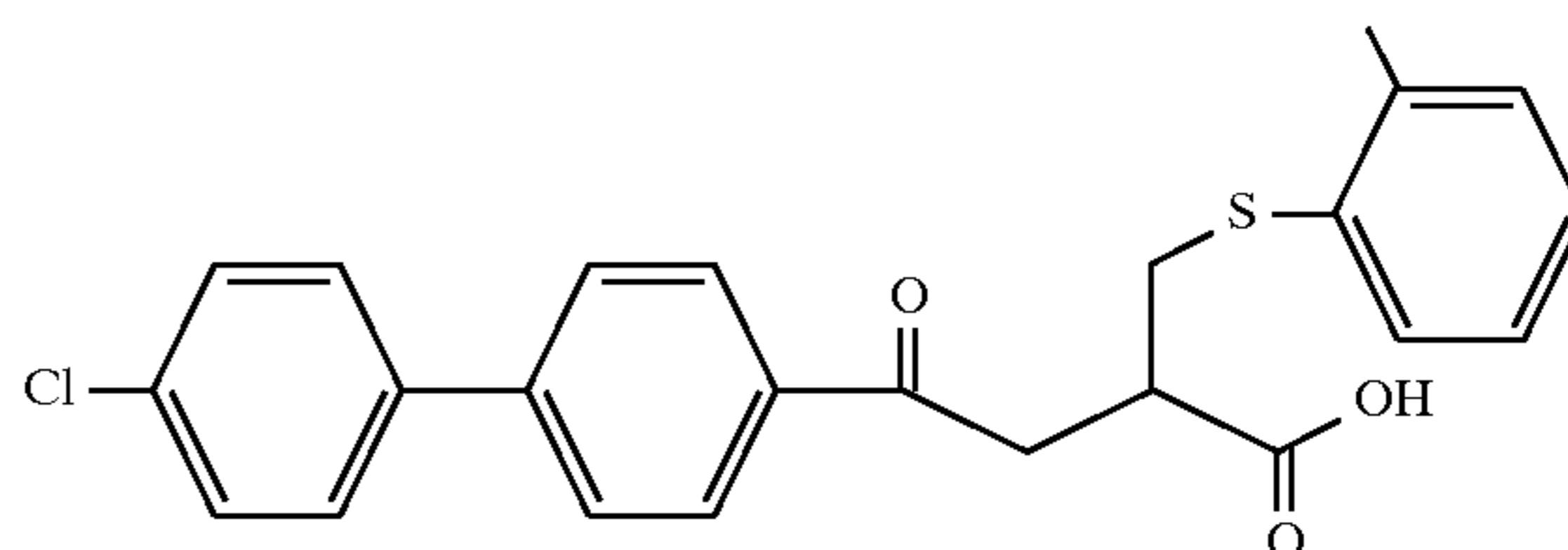
Example 162
