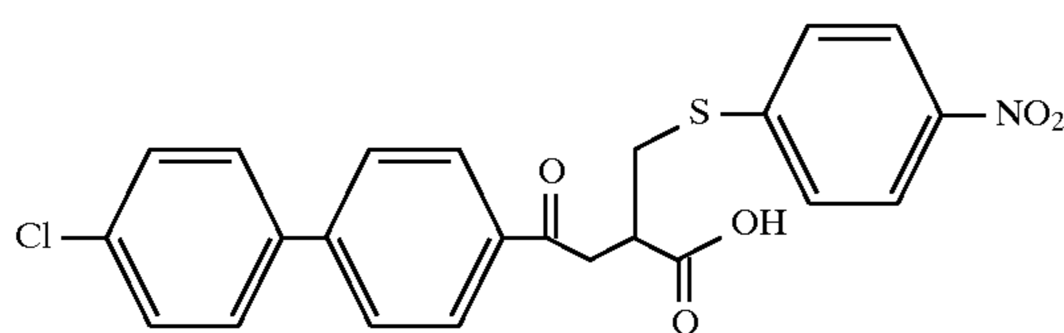
Example 154
