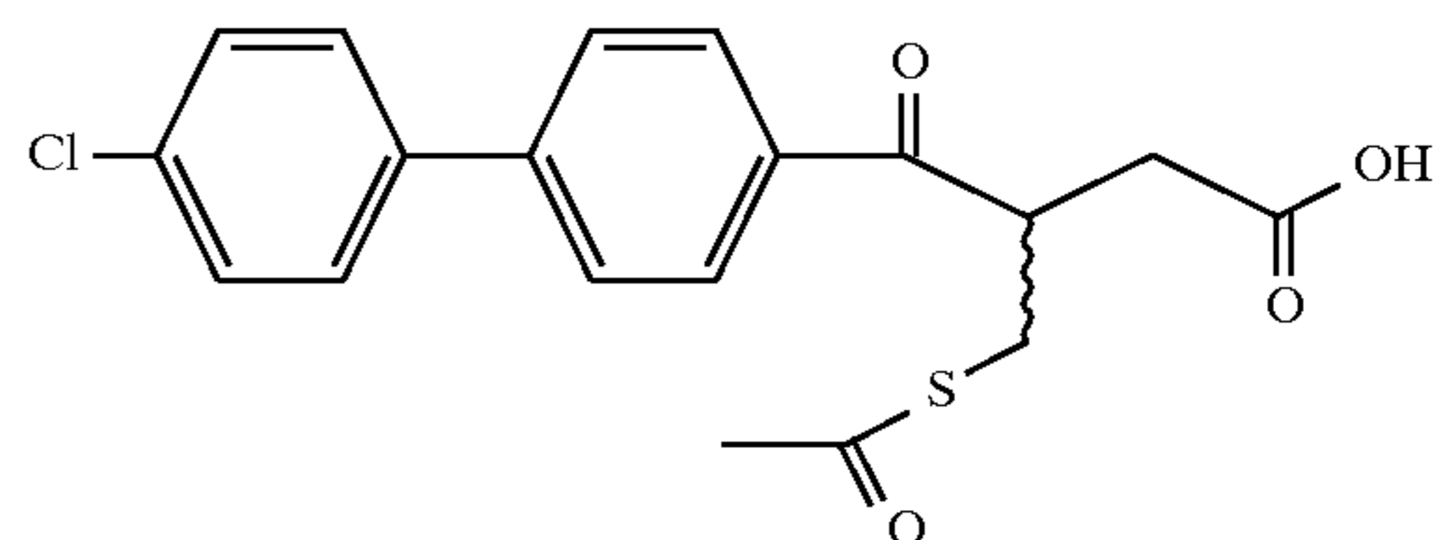
Example 182
