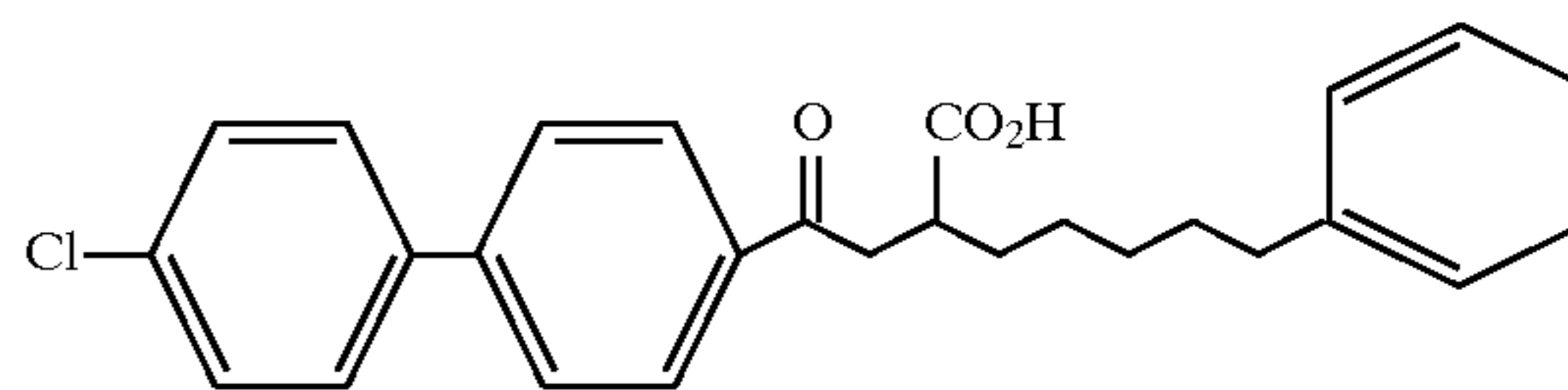
Example 108
