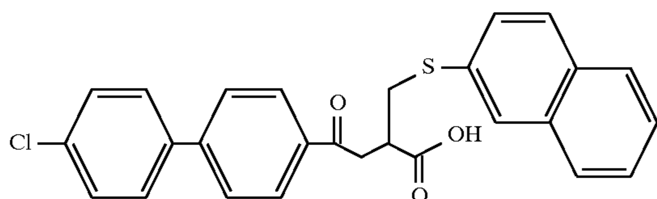
Example 156
