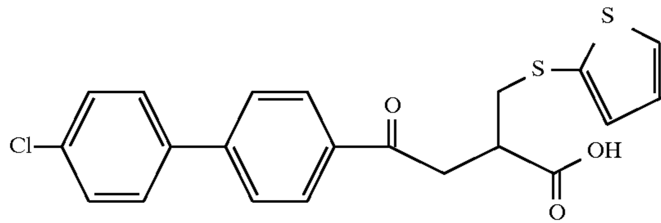
Example 129
