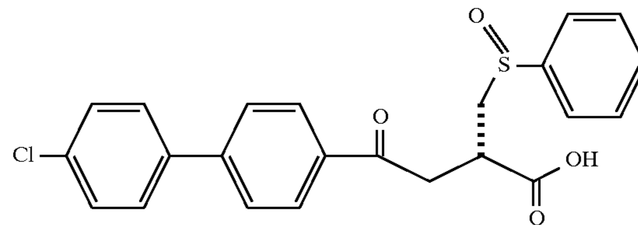
Example 127
