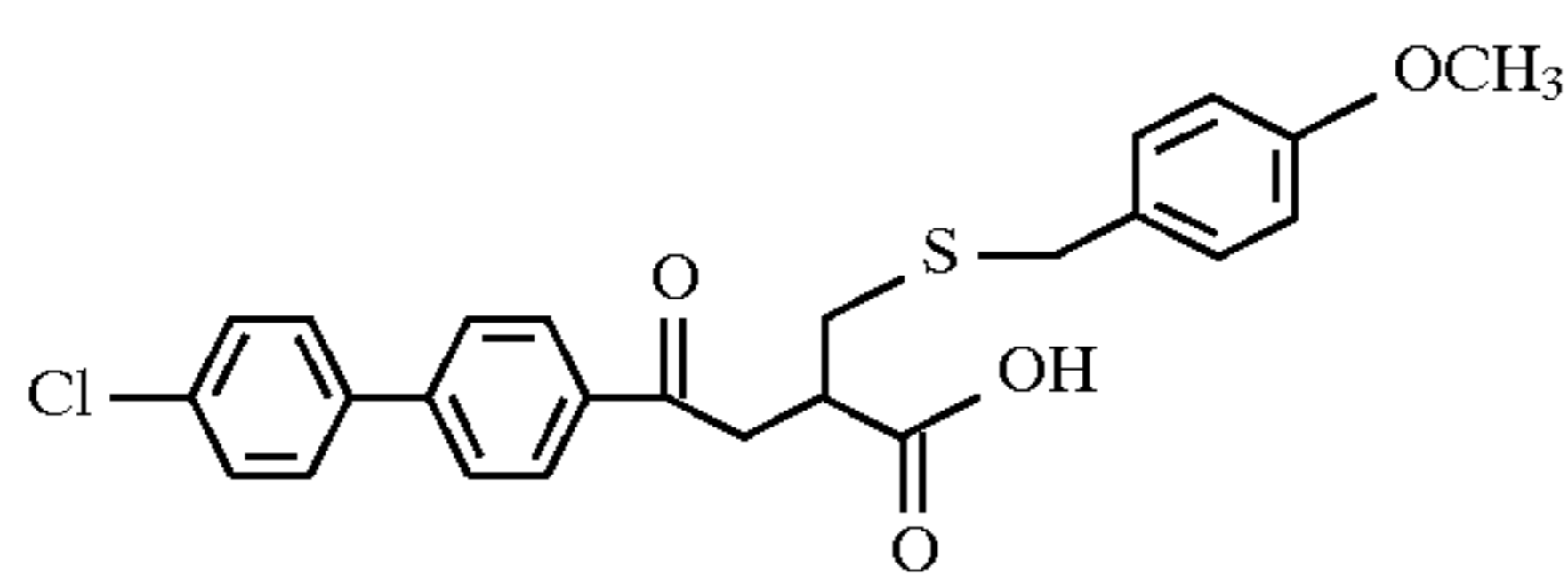
Example 131
