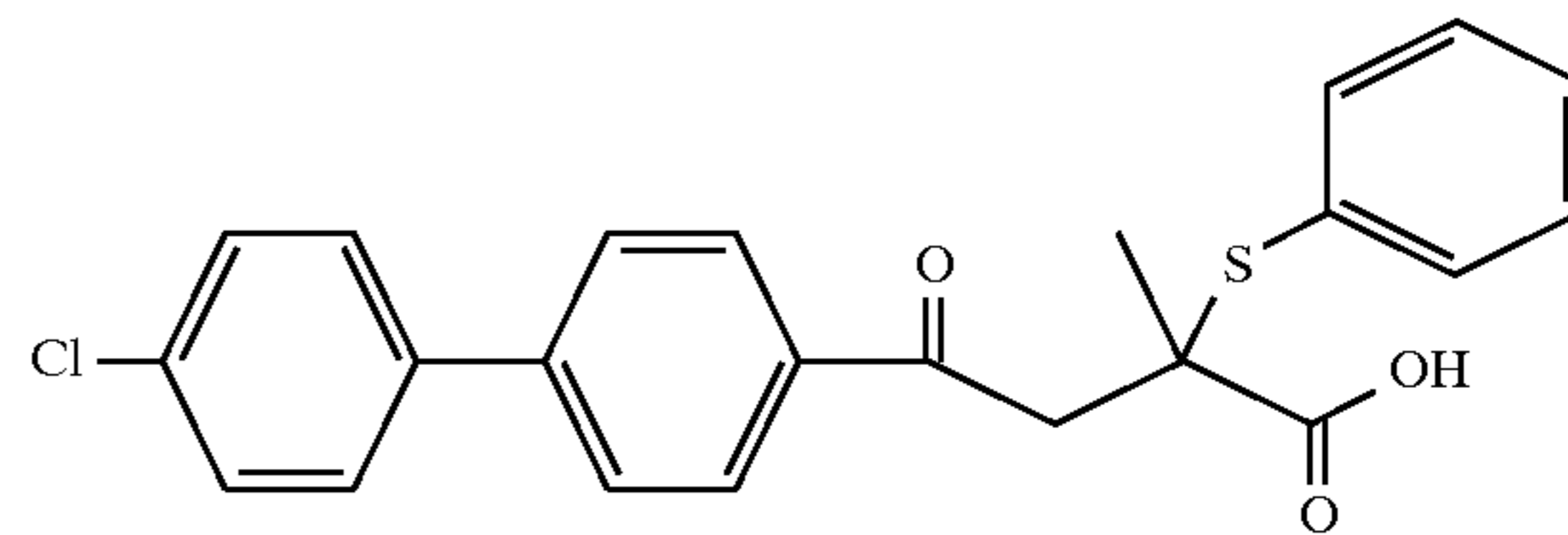
Example 122
