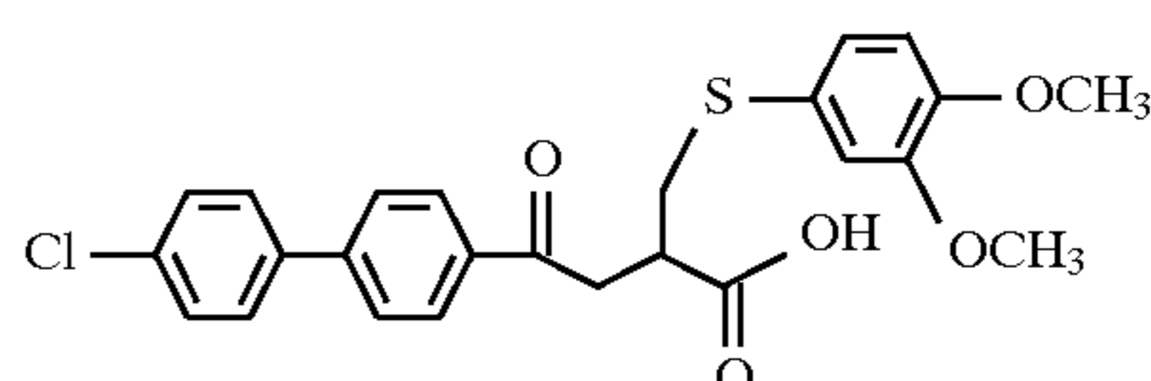
Example 145
