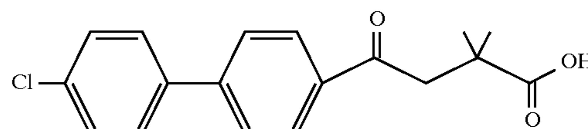
Example 197
