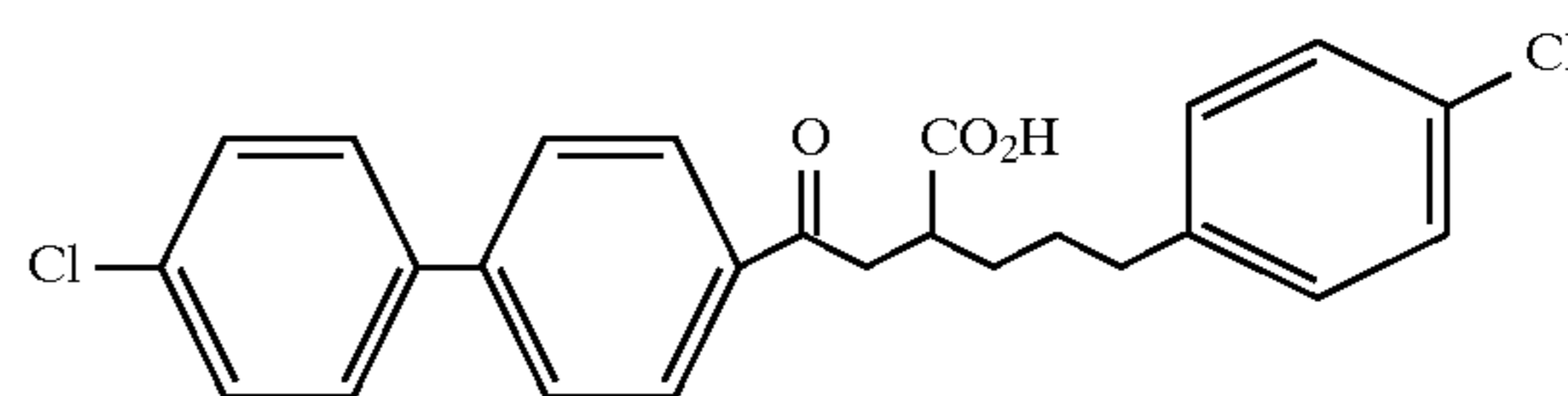
Example 113
