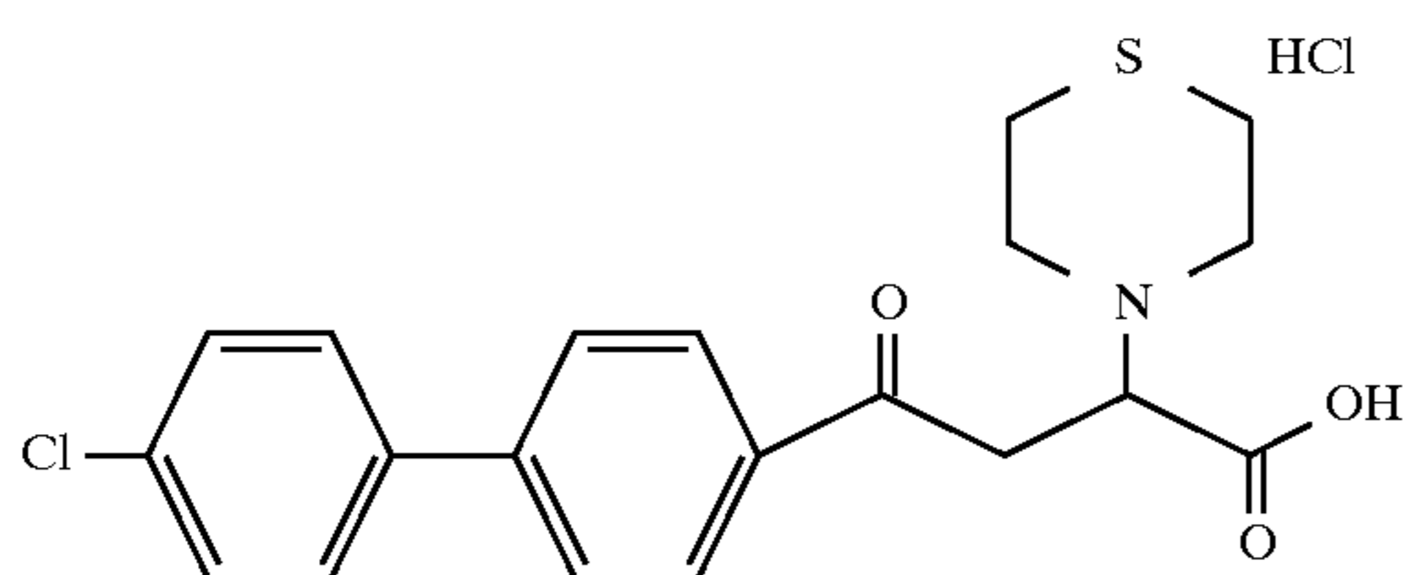
Example 184
