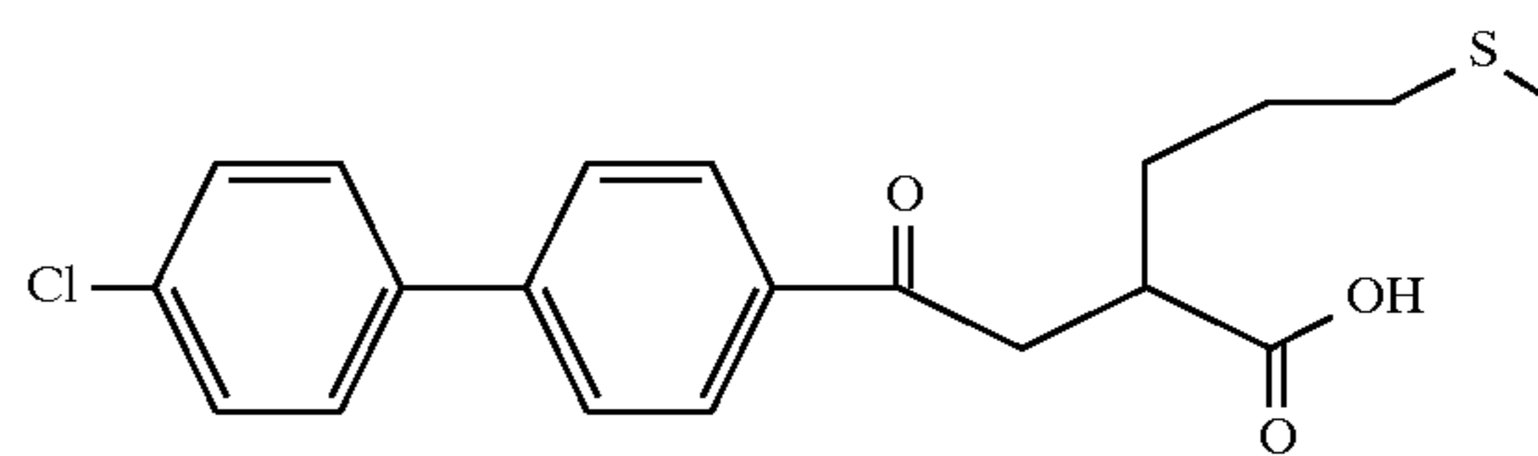
Example 193
