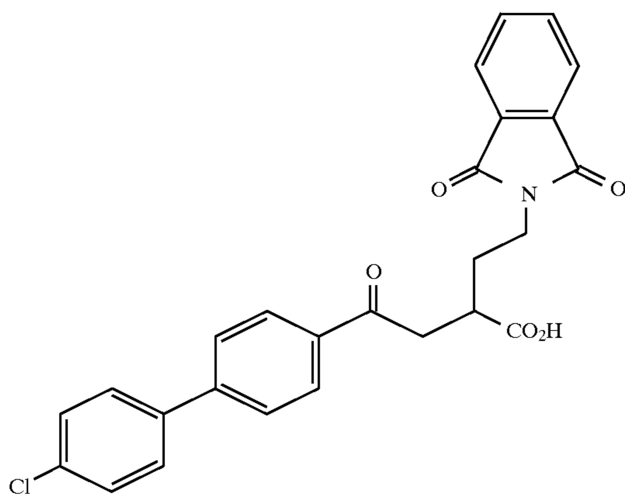
Example 194
