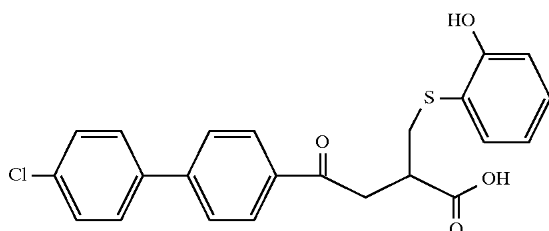
Example 170
