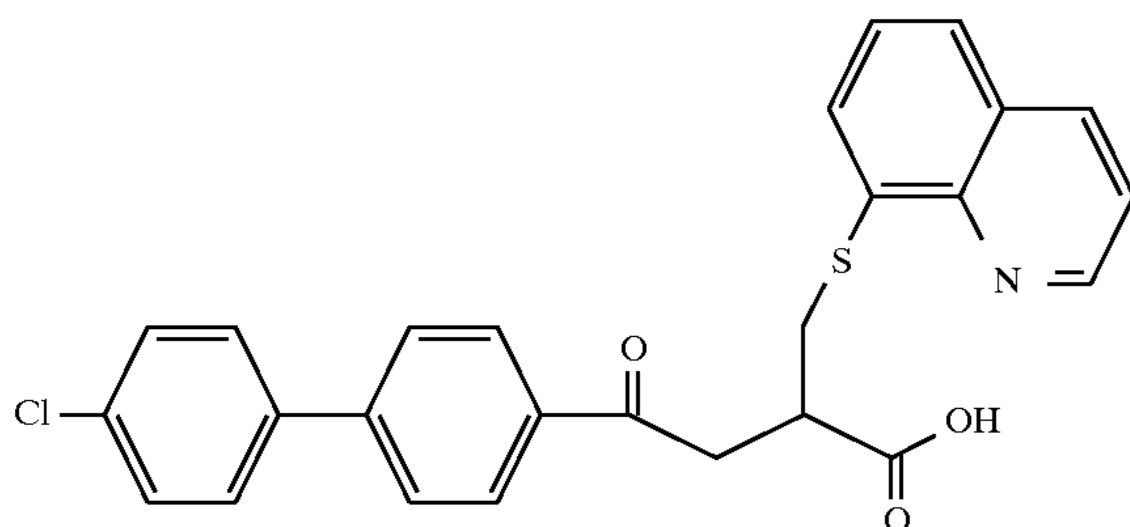
Example 171
