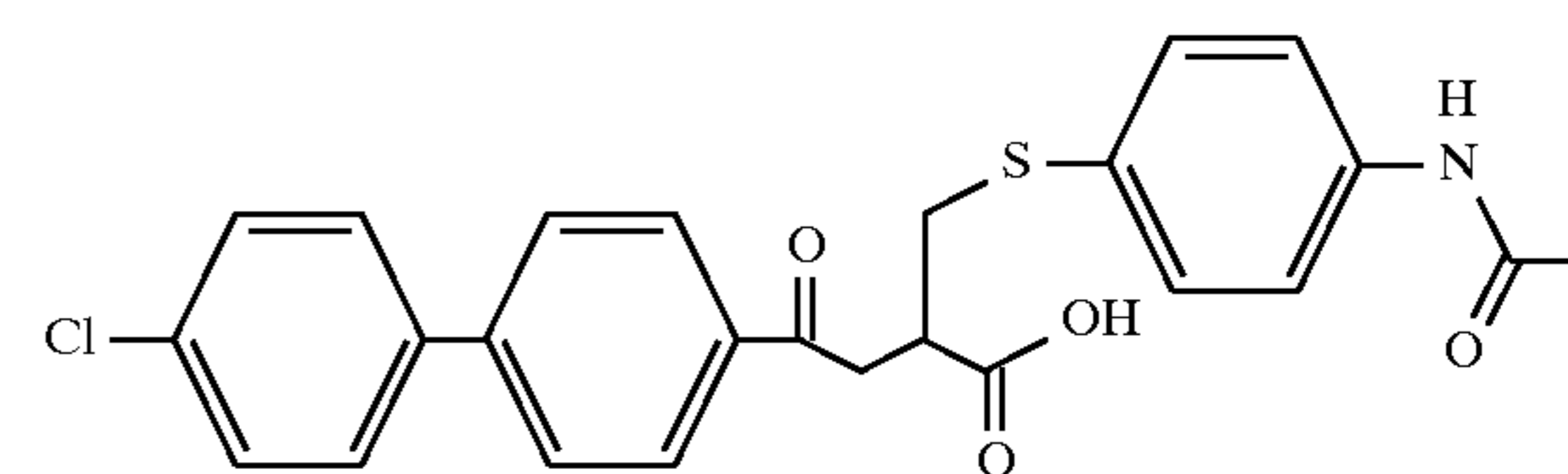
Example 153
