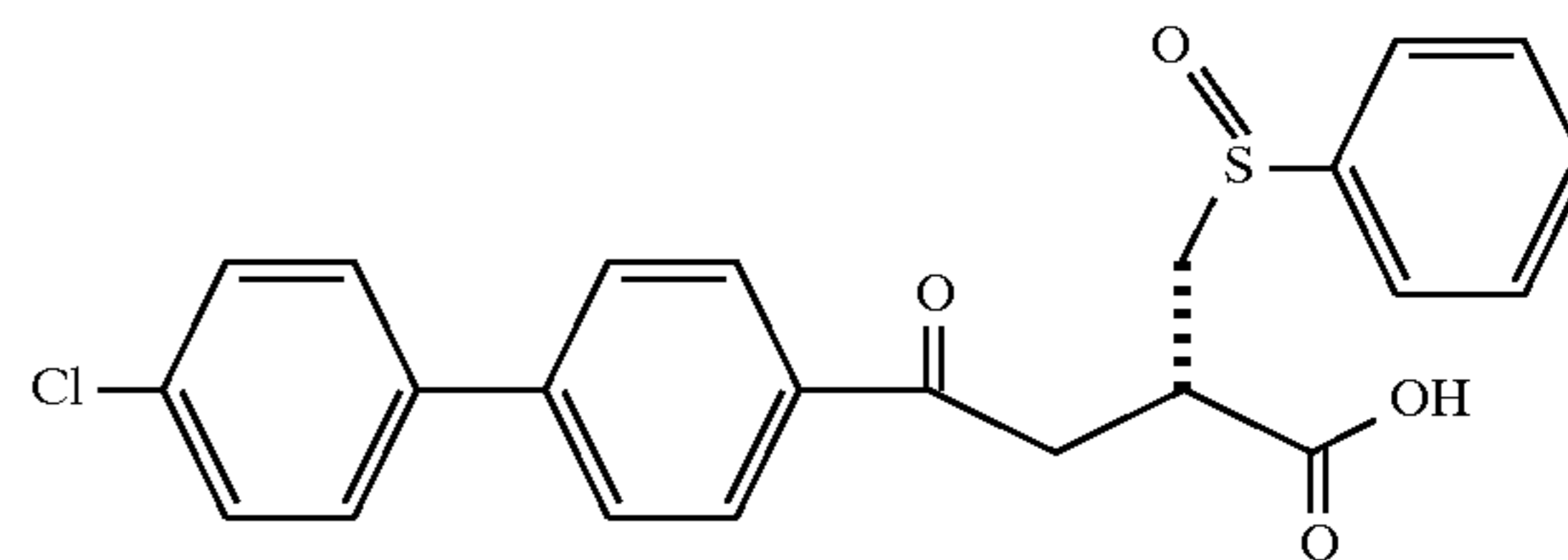
Example 127
