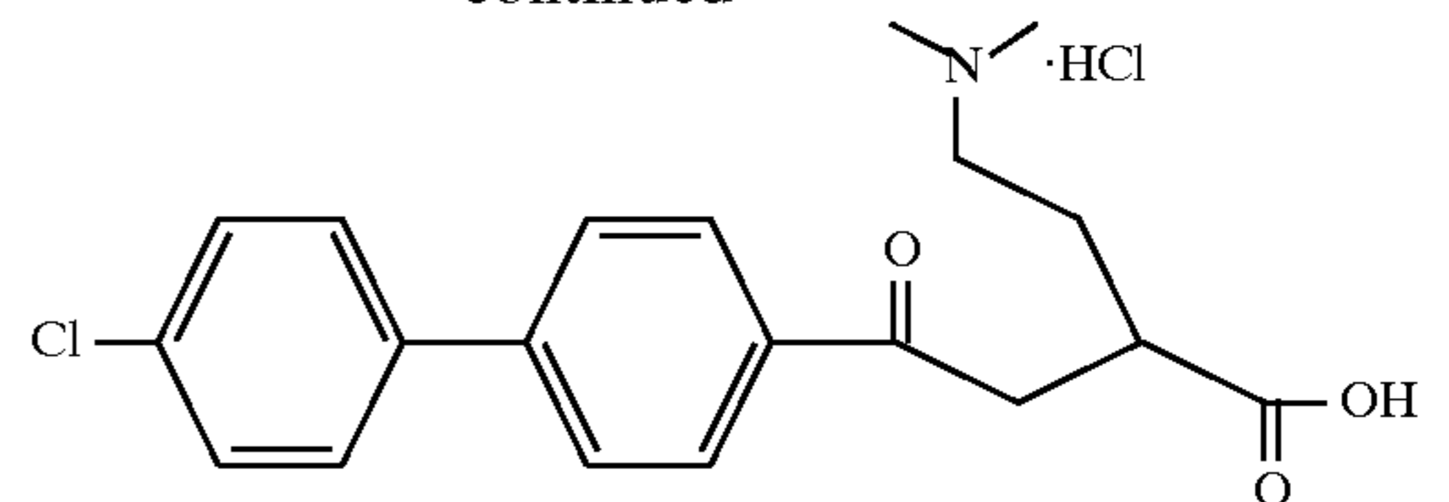
Example 190
