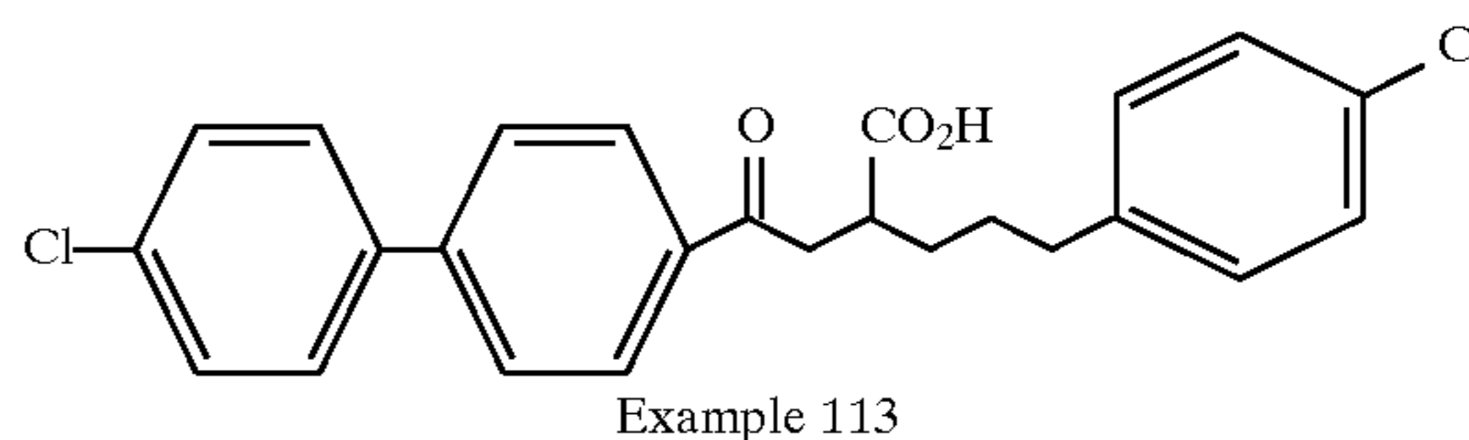
Example 113
