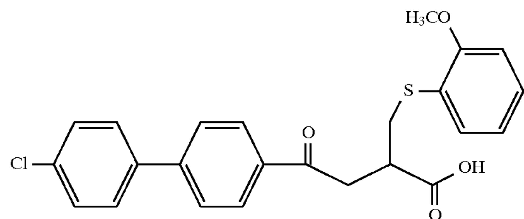
Example 159
