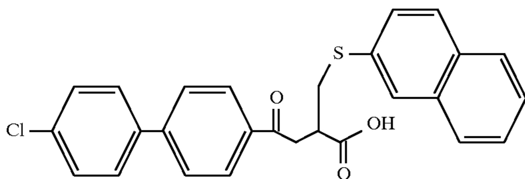
Example 156
