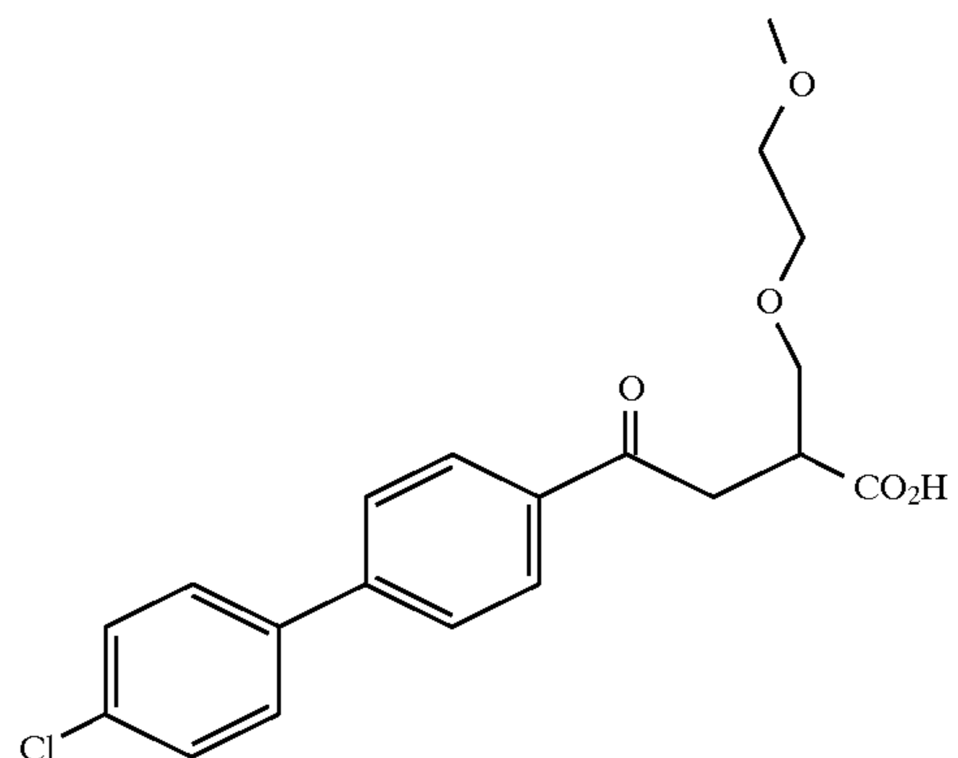
Example 195
