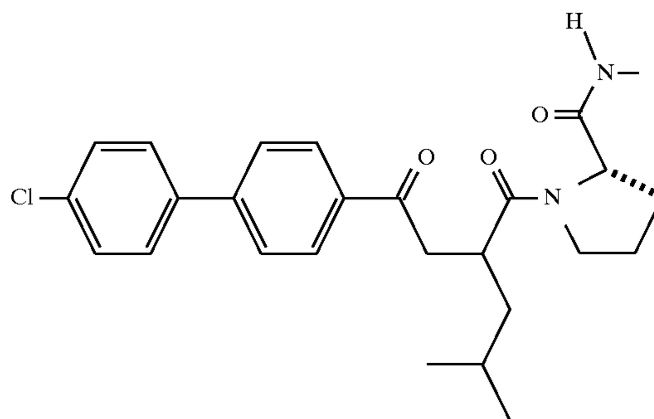
Example 247
