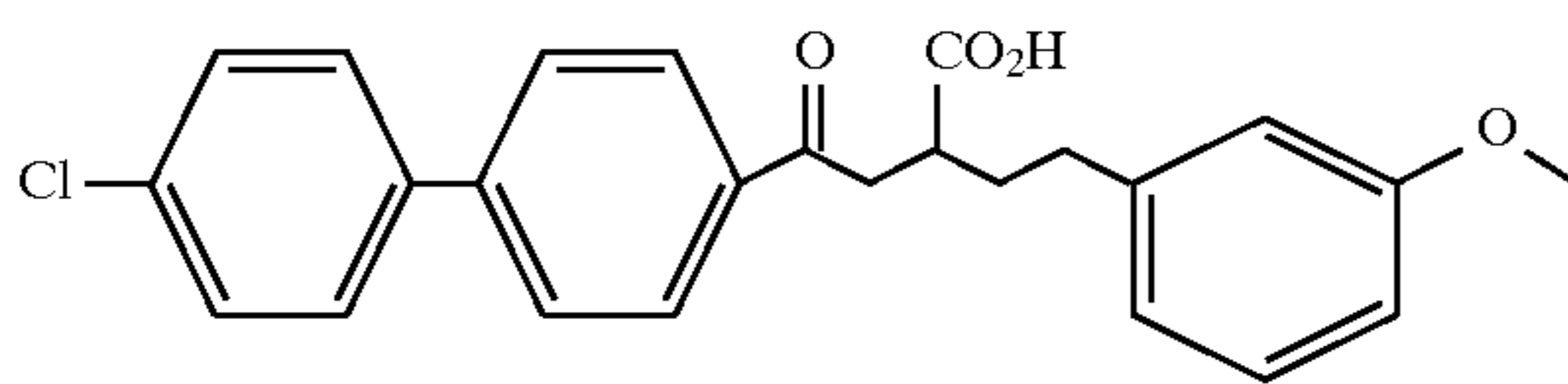
Example 116
