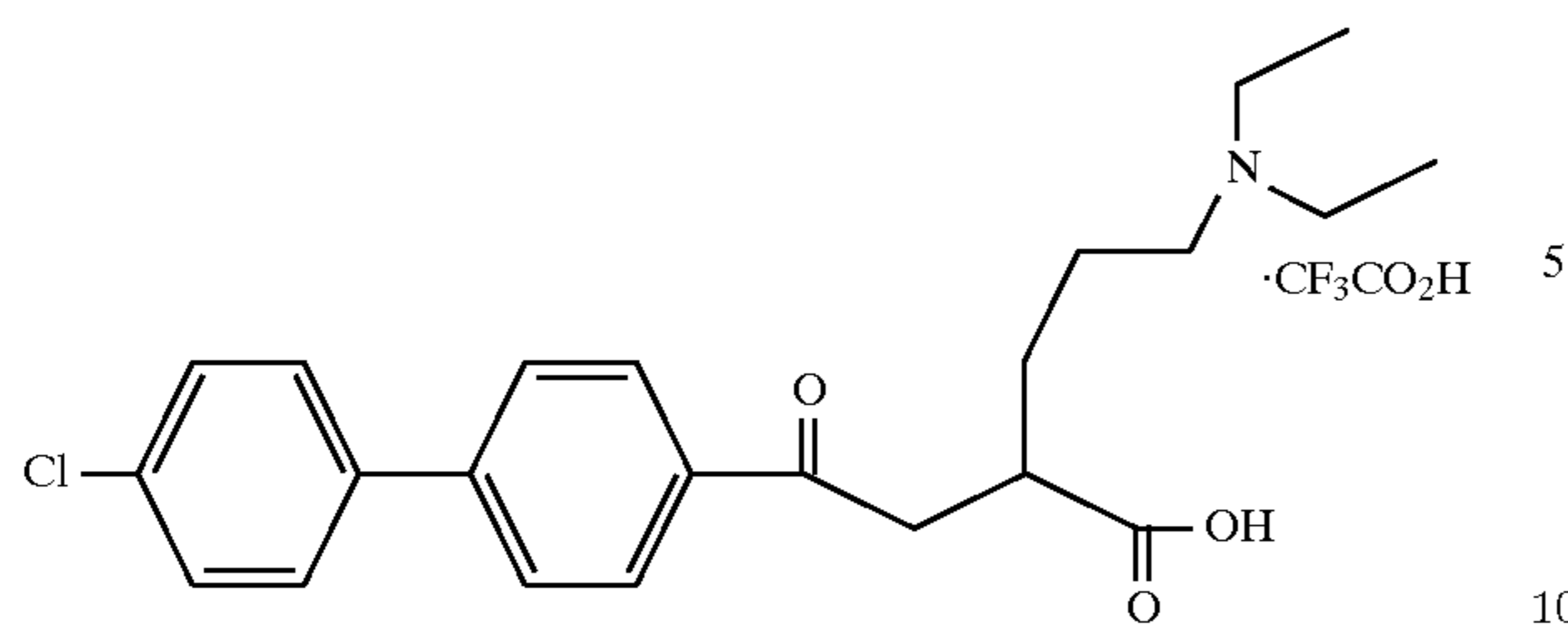
Example 192
