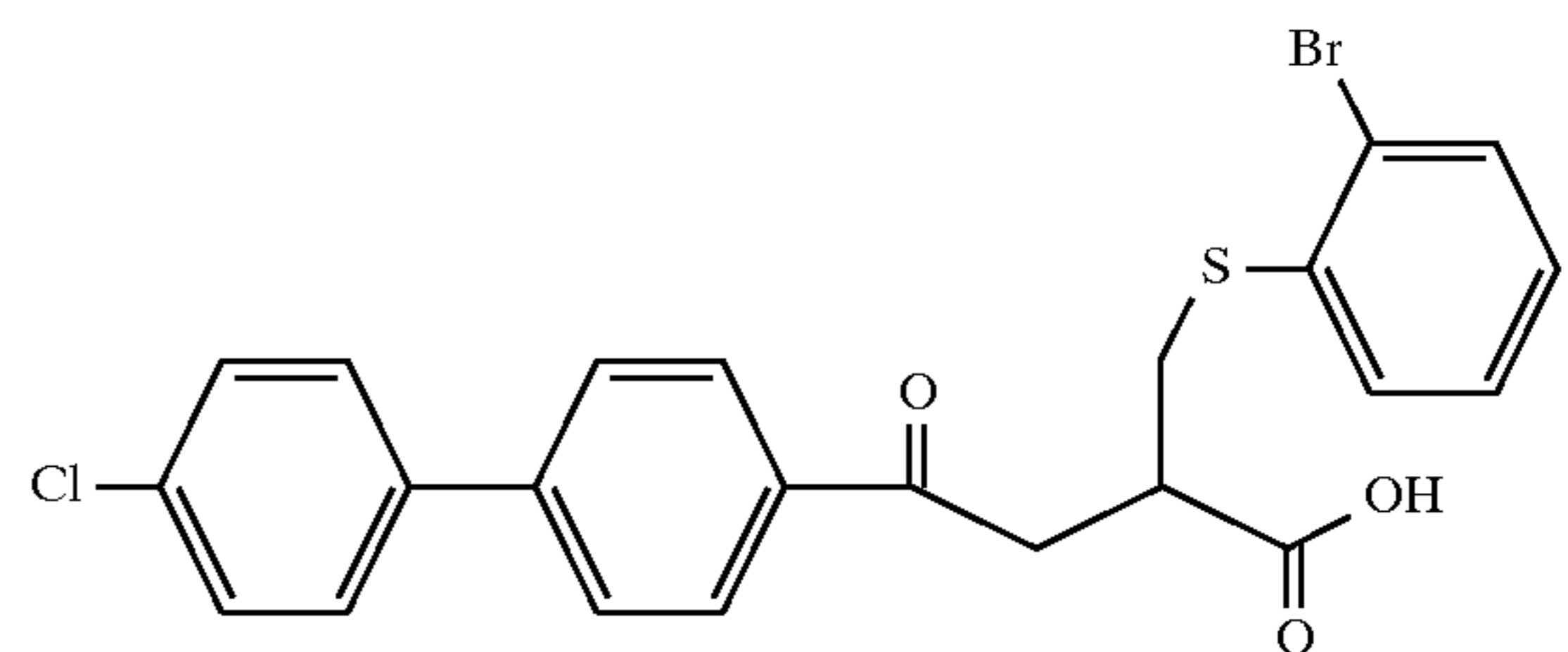
Example 149
