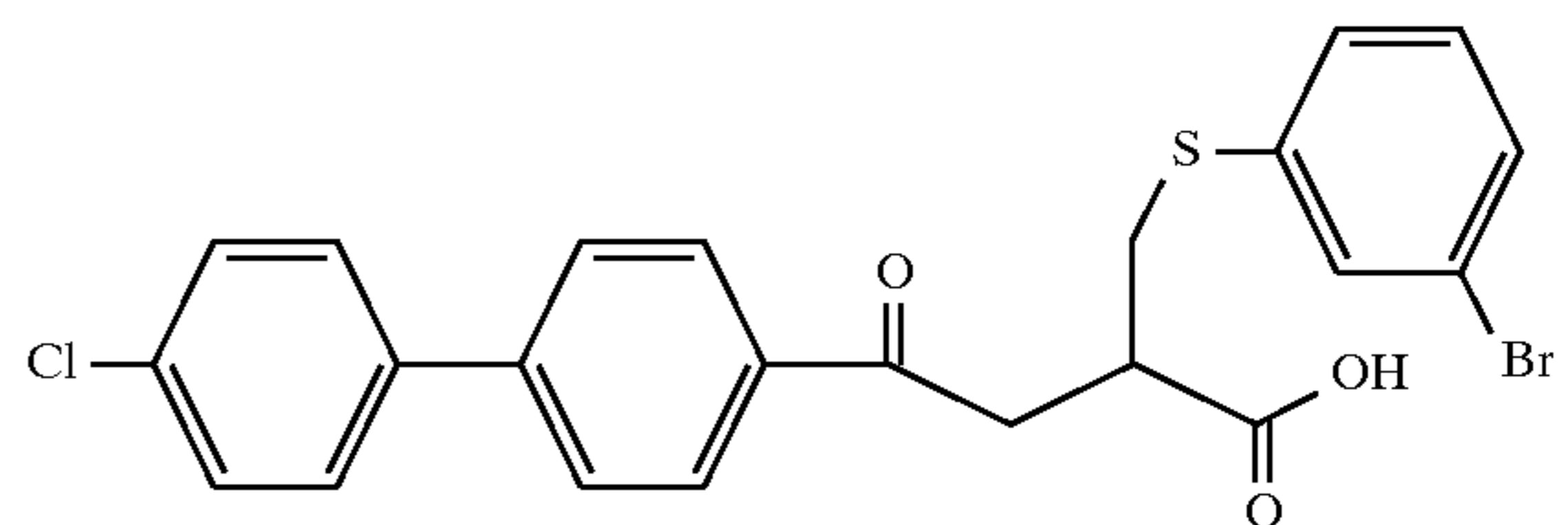
Example 158
