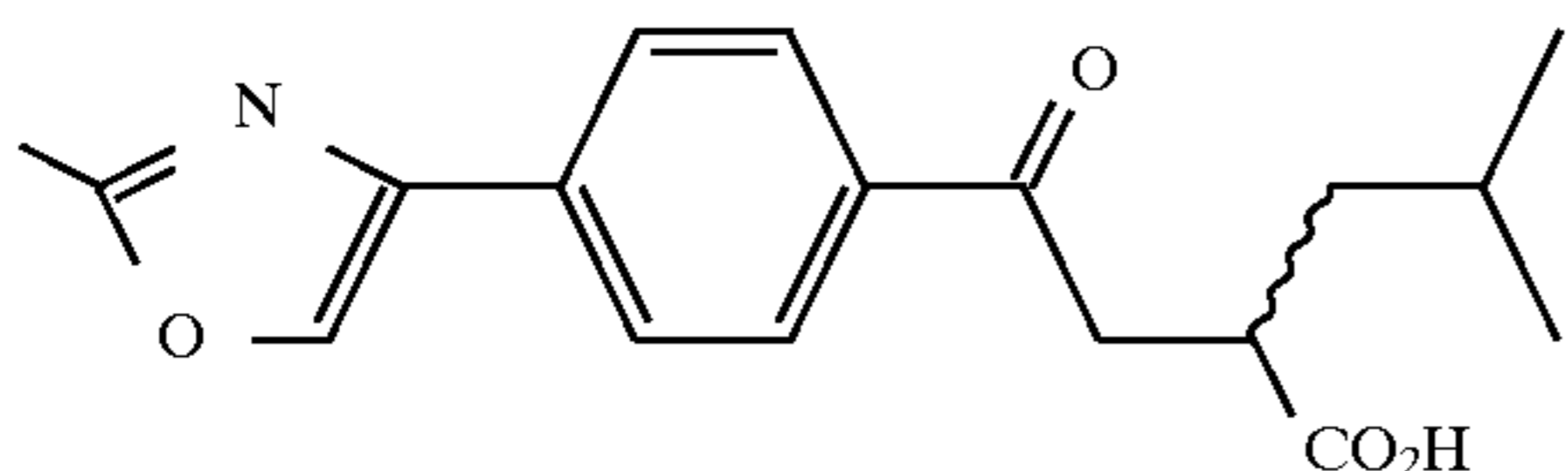
Example 248
