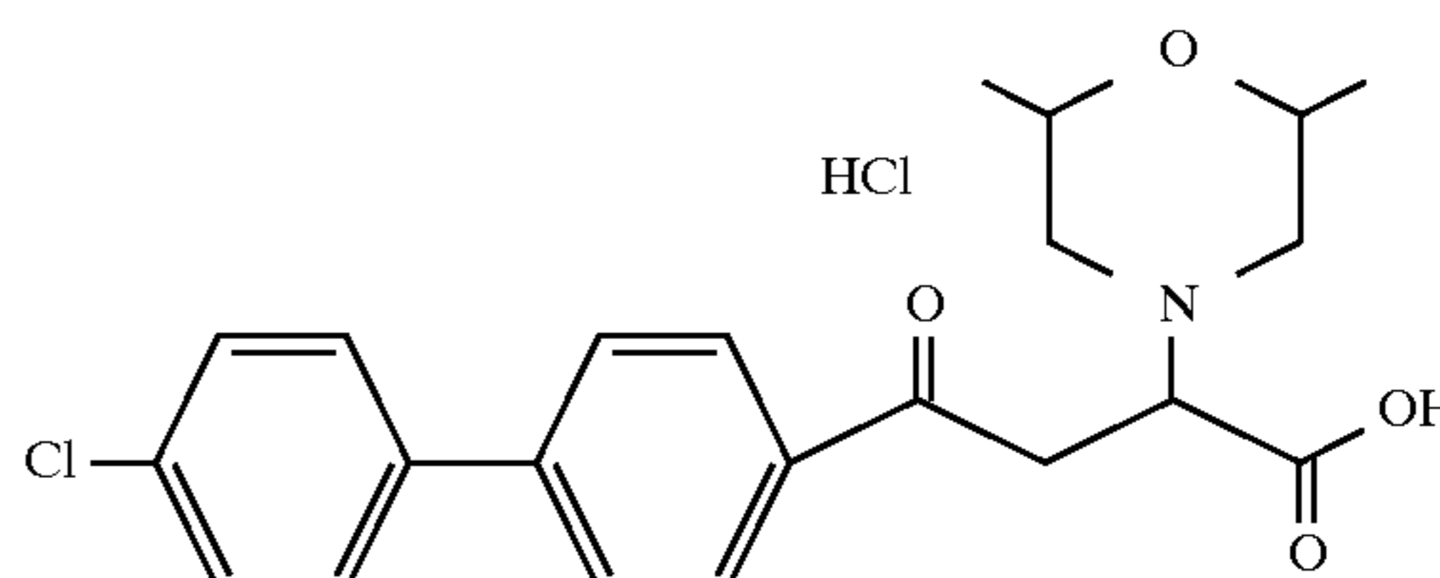
Example 186
