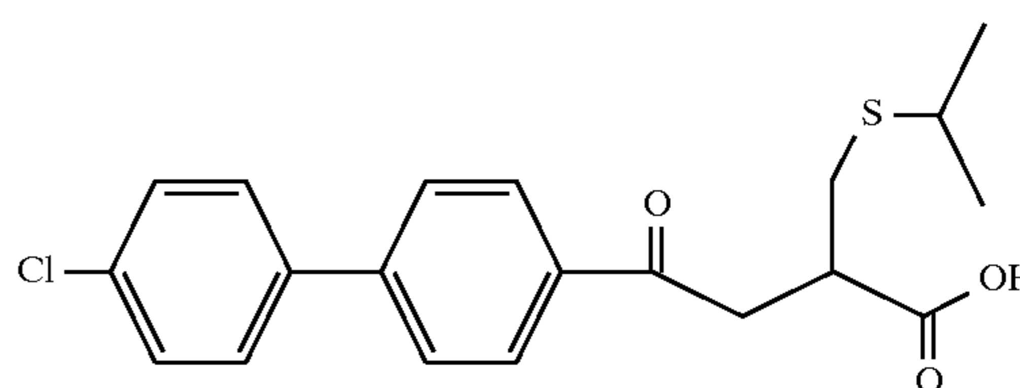
Example 169
