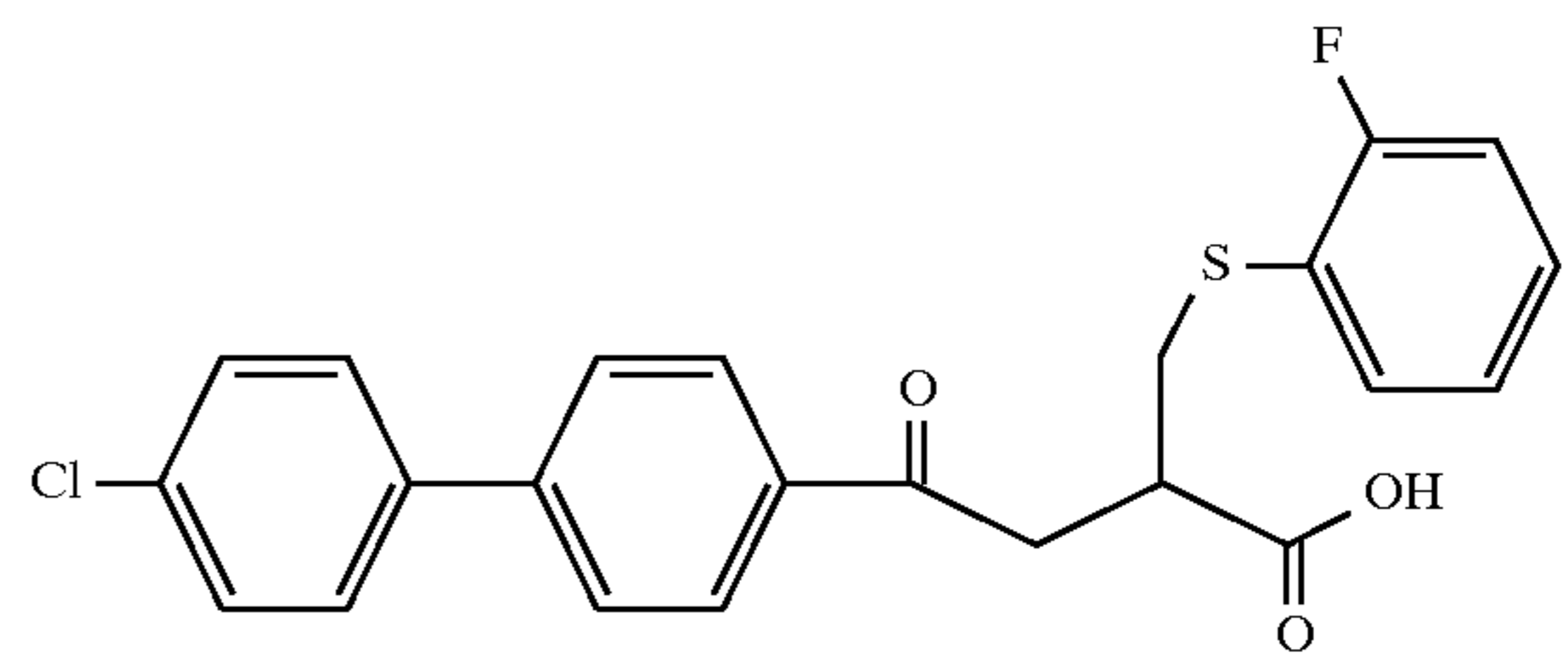
Example 148
