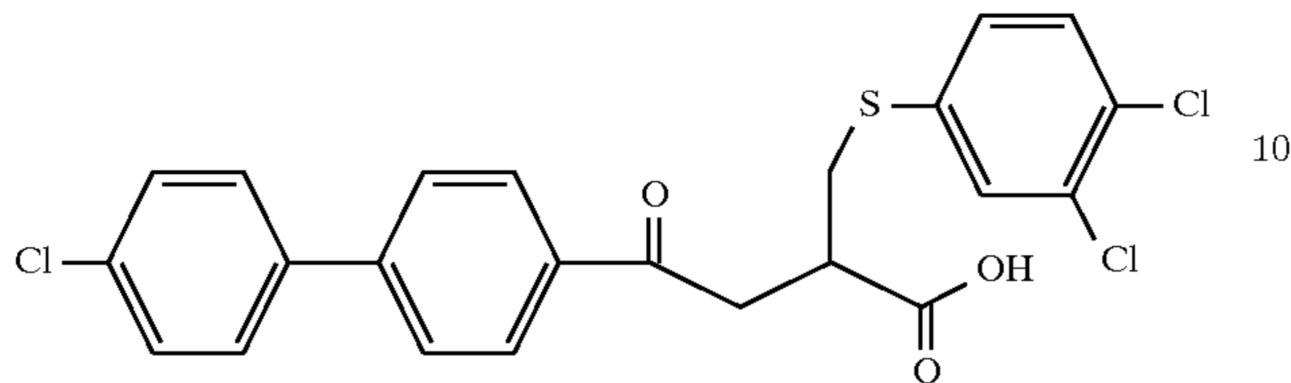
Example 146
