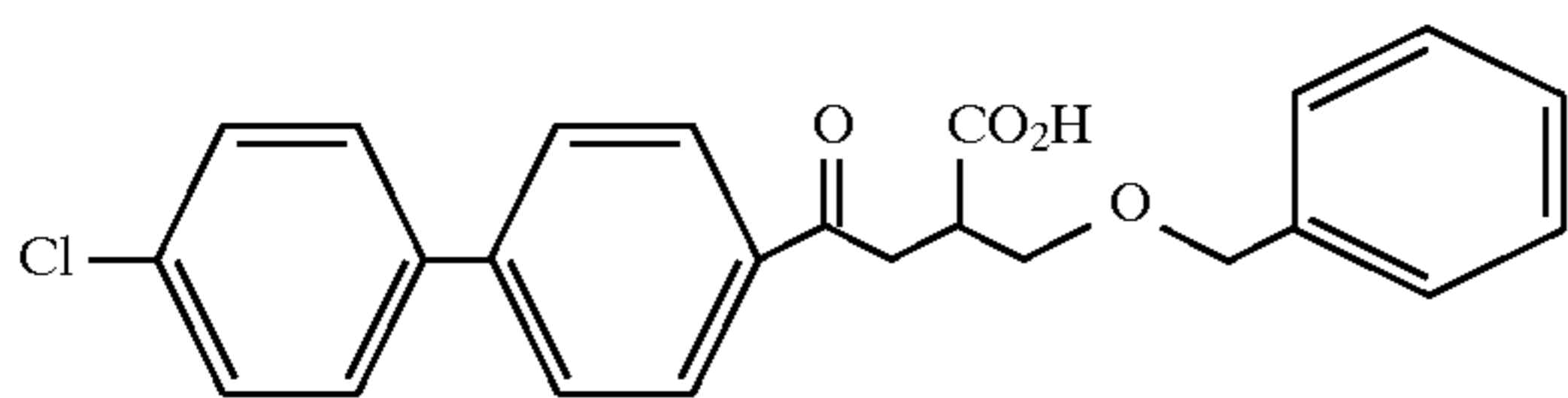
Example 196
