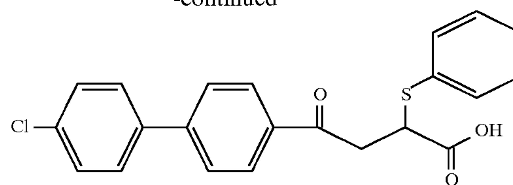
Example 176
