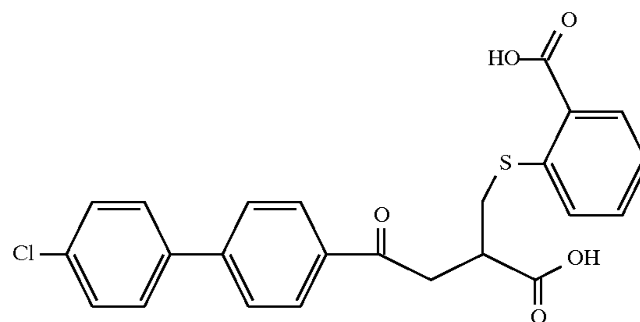
Example 163
