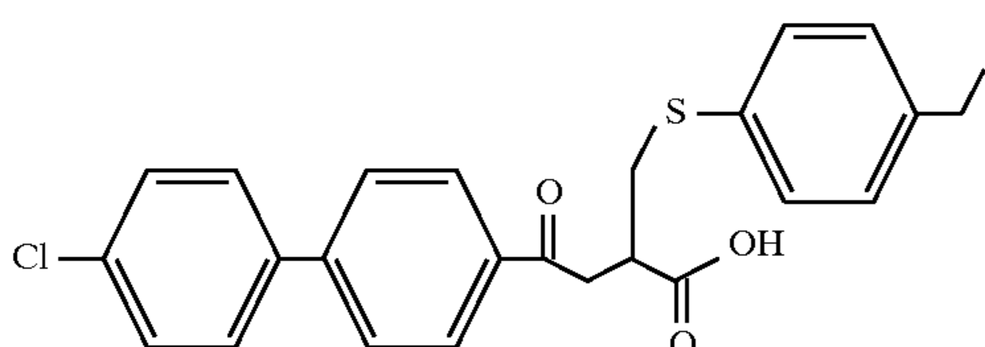
Example 142
