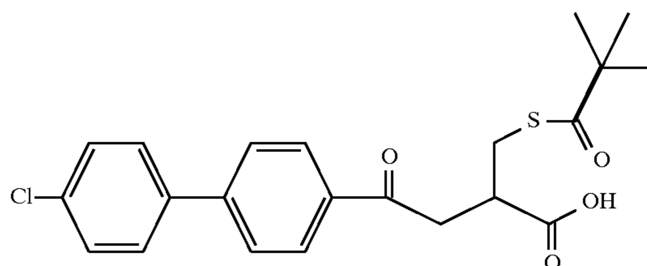
Example 118
