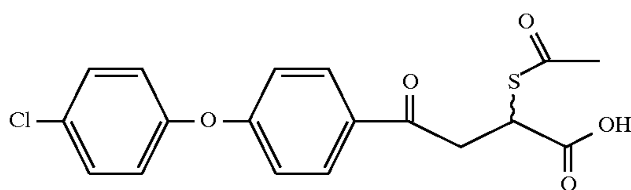
Example 183
