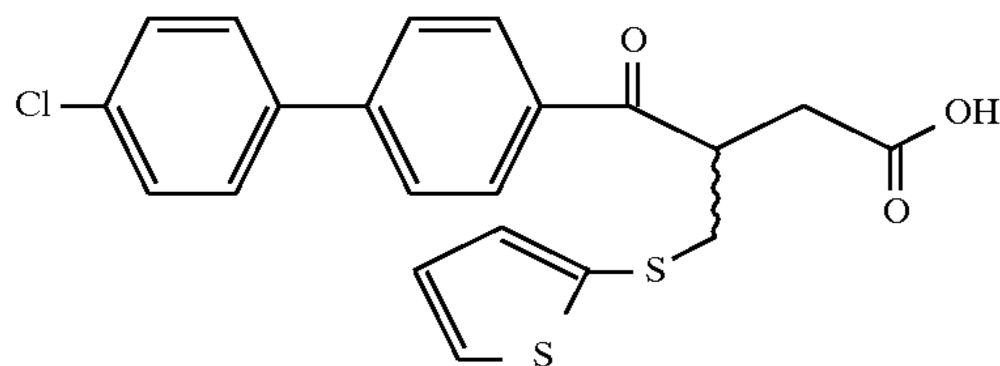
Example 179
