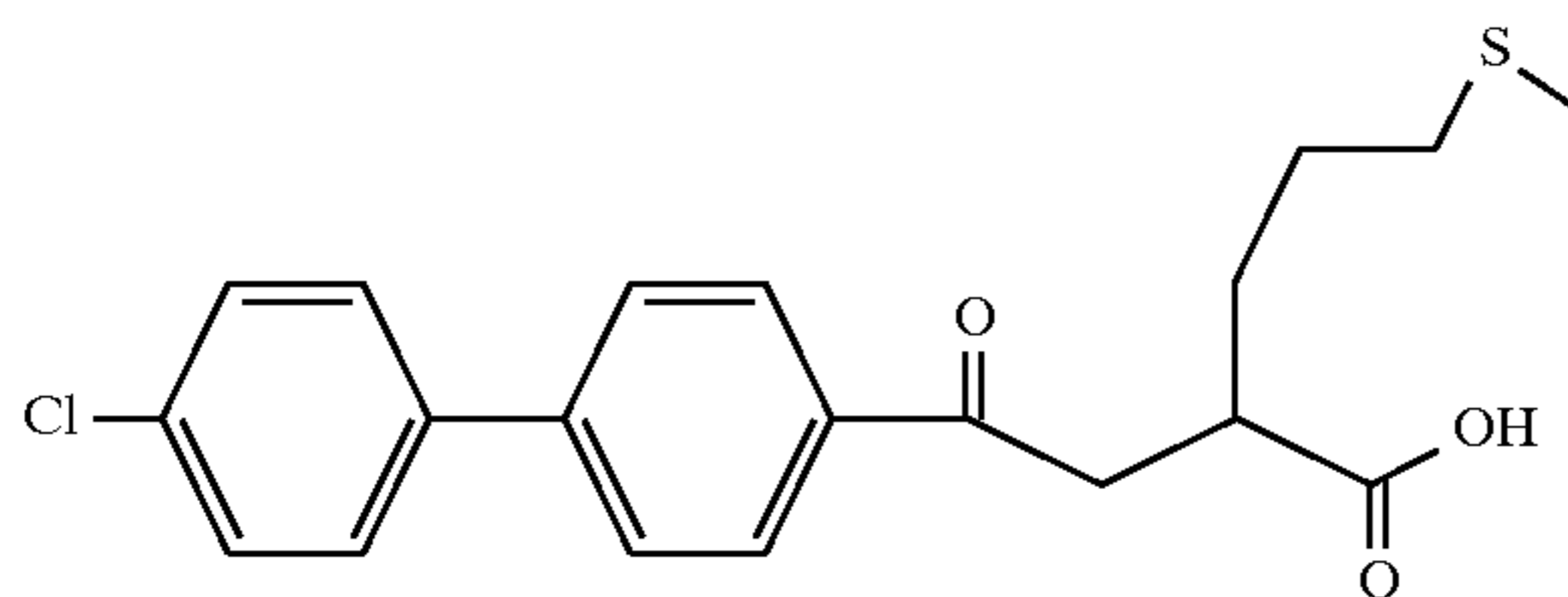
Example 193
