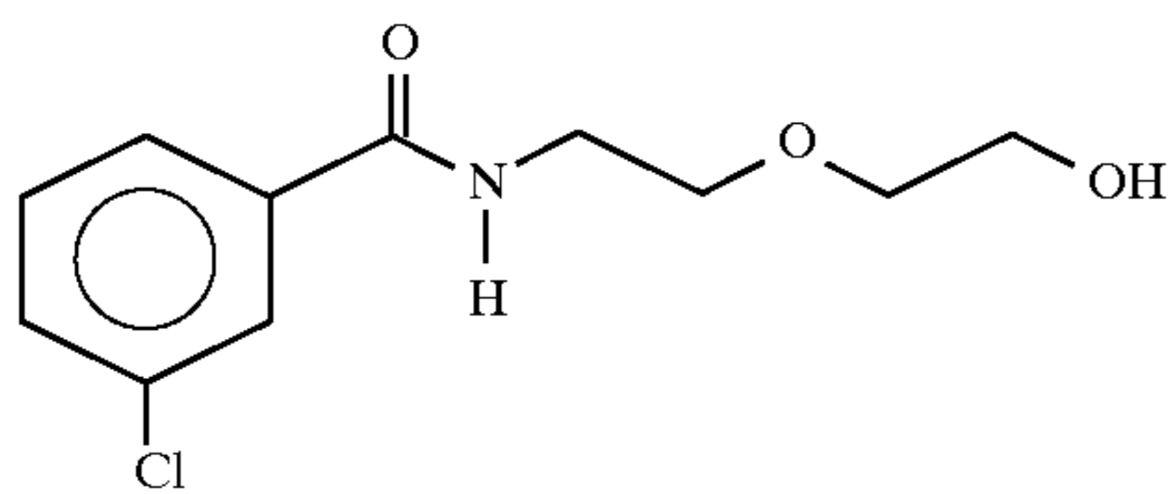
2-[2-N-(3-chlorobenzoyl)aminoethoxy]ethanol
