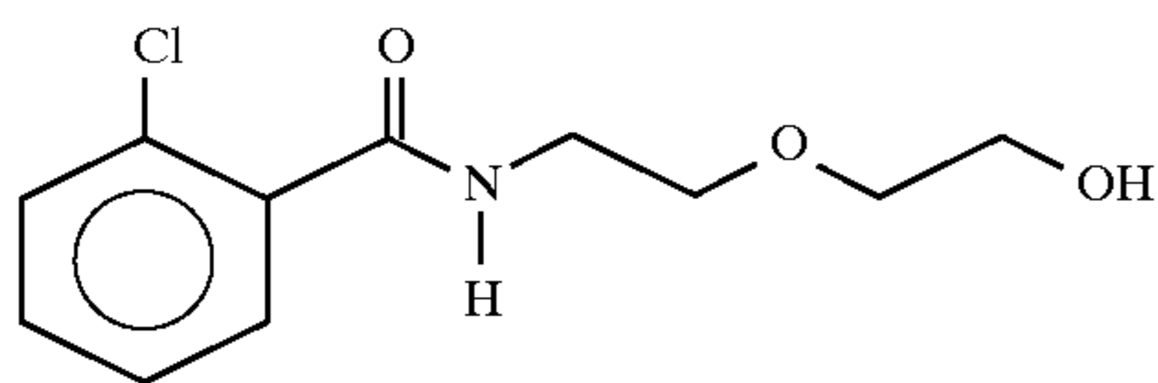
2-[2-N-(2-chlorobenzoyl)aminoethoxy]ethanol
