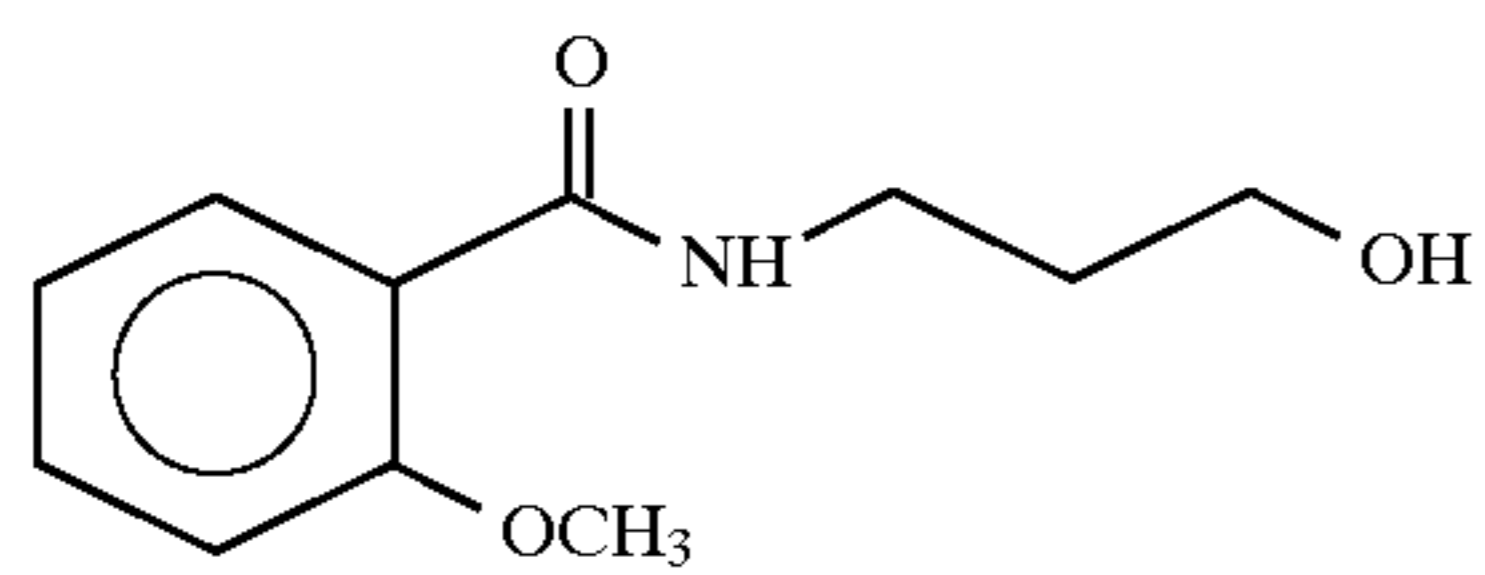
3-(2-methoxybenzoylamino)-1-propanol
