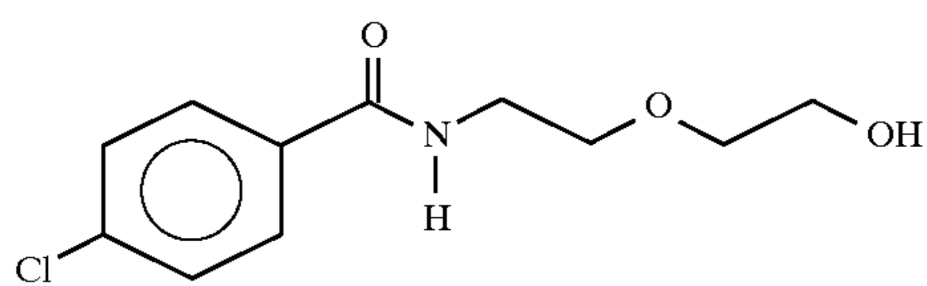
2-[2-N-(4-chlorobenzoyl)aminoethoxy]ethanol
