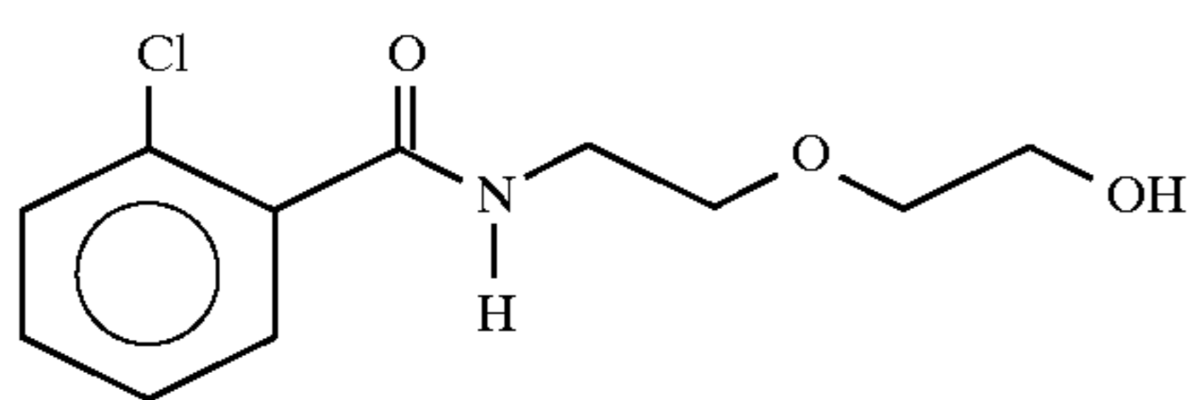
2-[2-N-(2-chlorobenzoyl)aminoethoxy]ethanol
