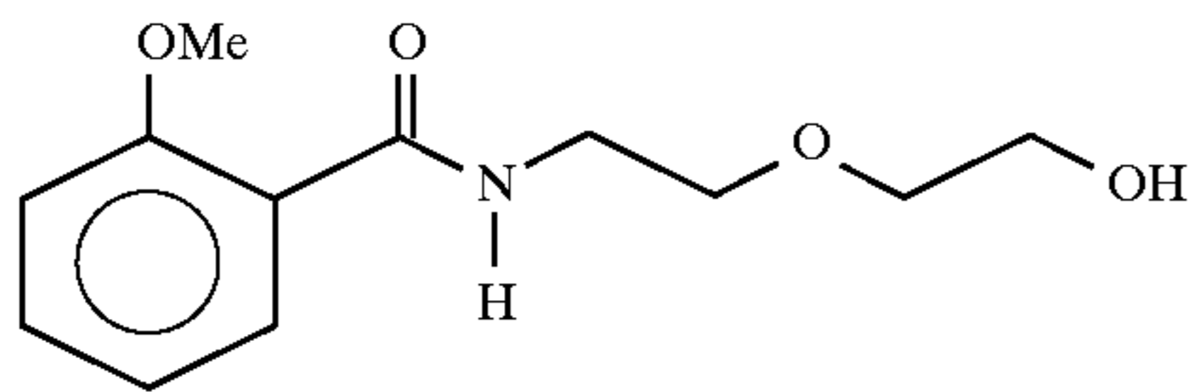
2-[2-N-(2-methoxybenzoyl)aminoethoxy]ethanol
