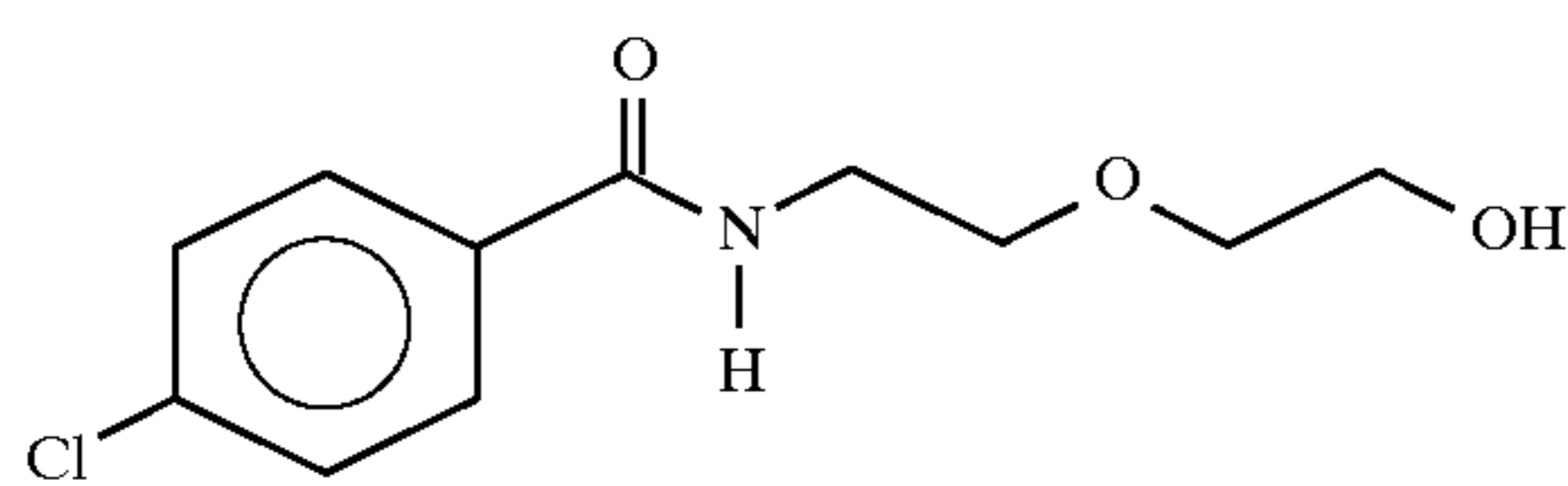
2-[2-N-(4-chlorobenzoyl)aminoethoxy]ethanol
