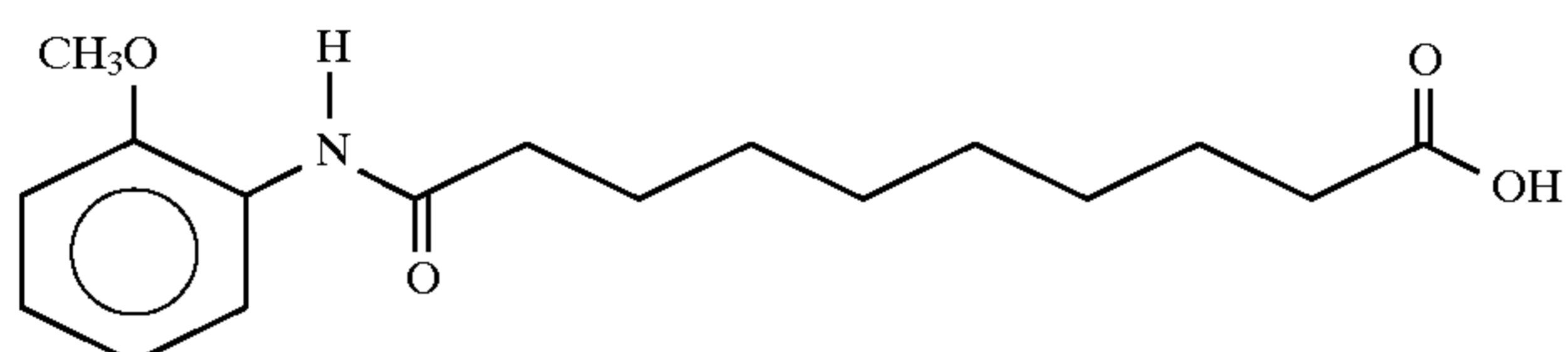
10-(N-2-Methoxyanilino)sebacic acid
