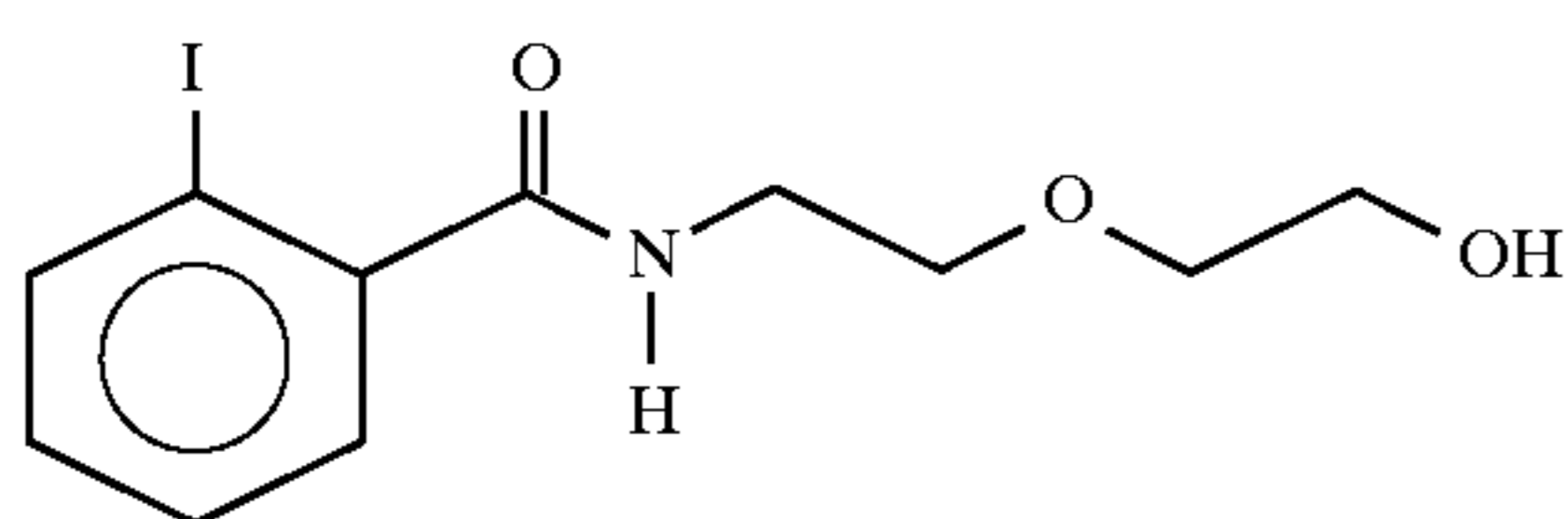
2-[N-(2-iodobenzoyl)aminoethoxy]ethanol
