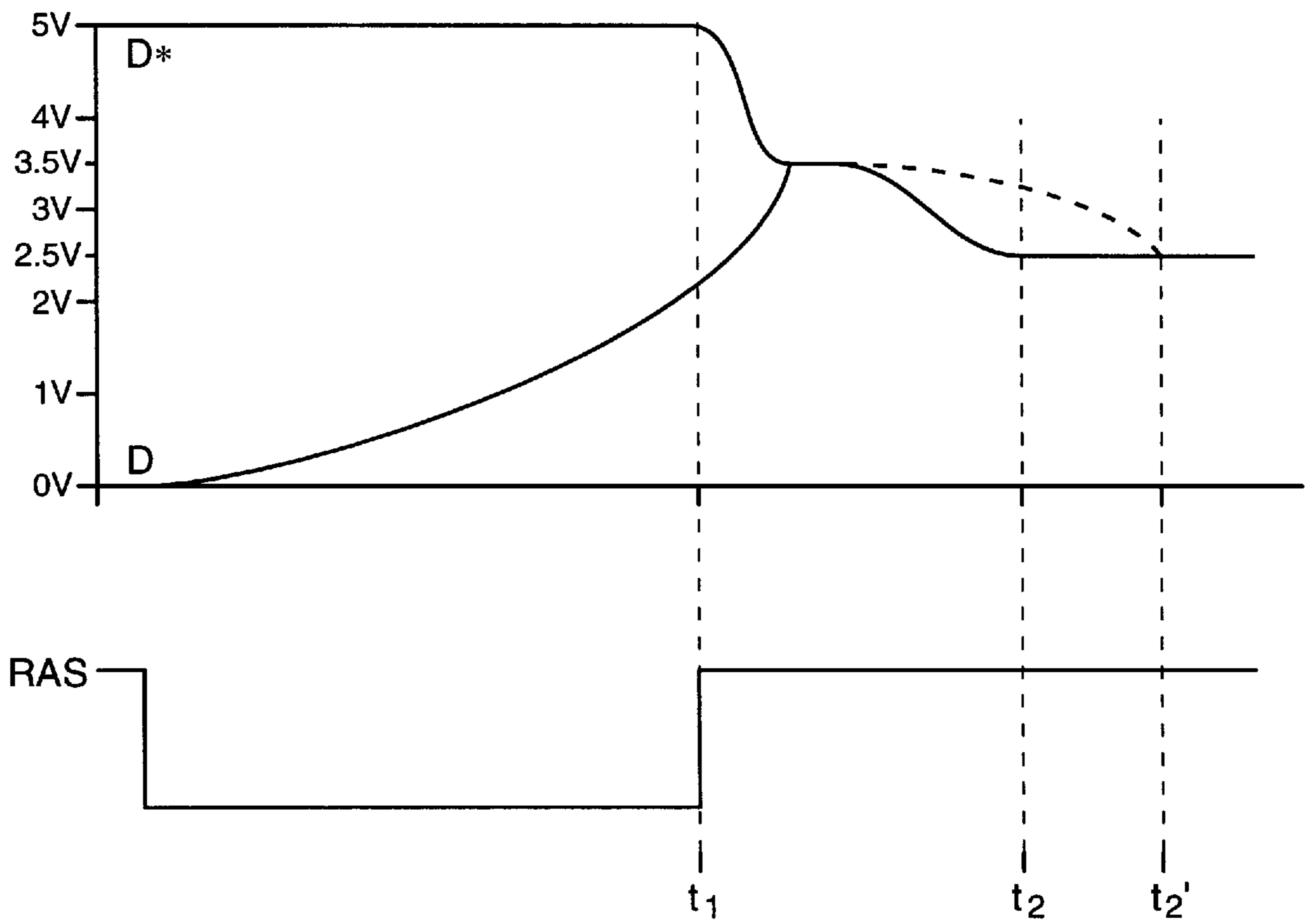
FIG. 8B
