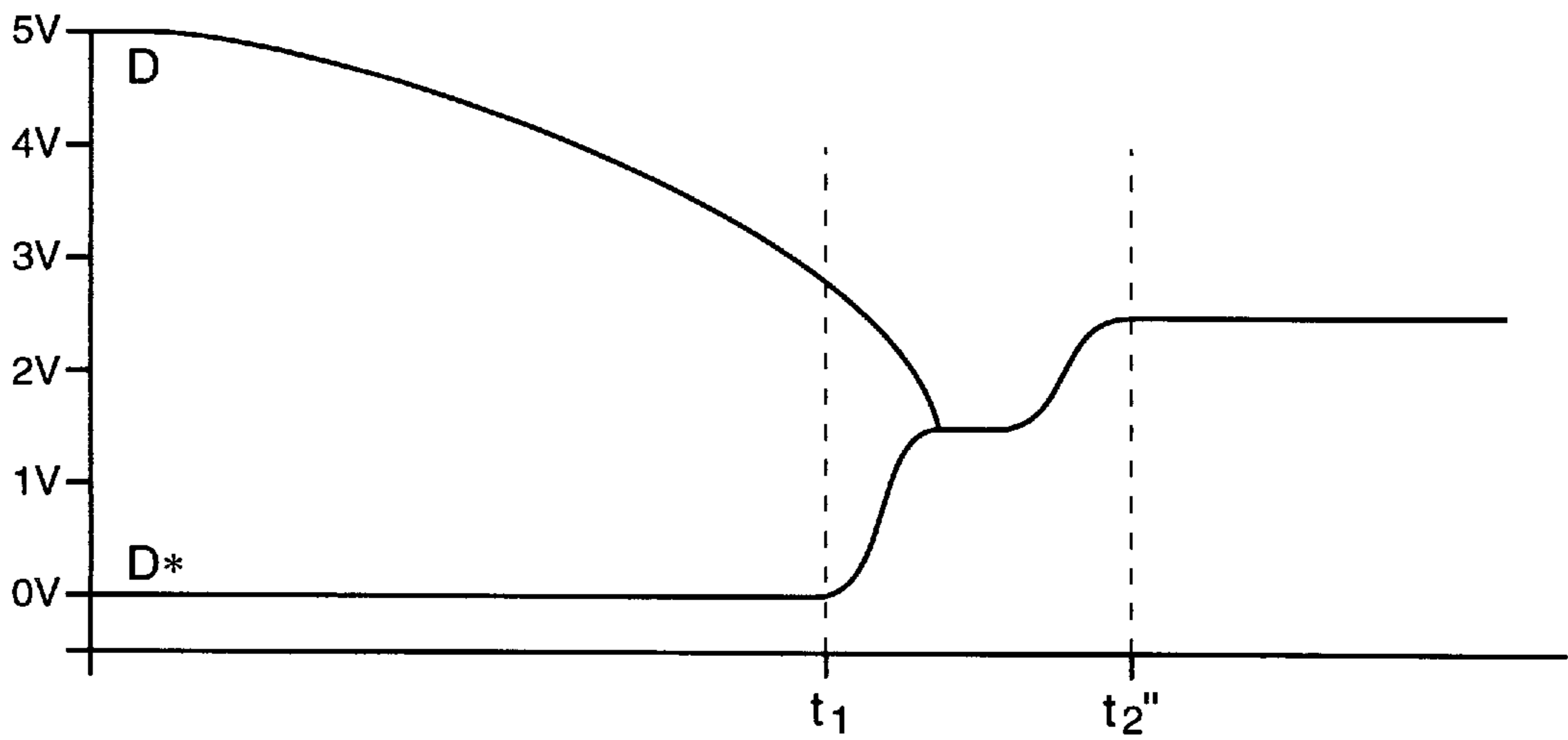
FIG. 8D
