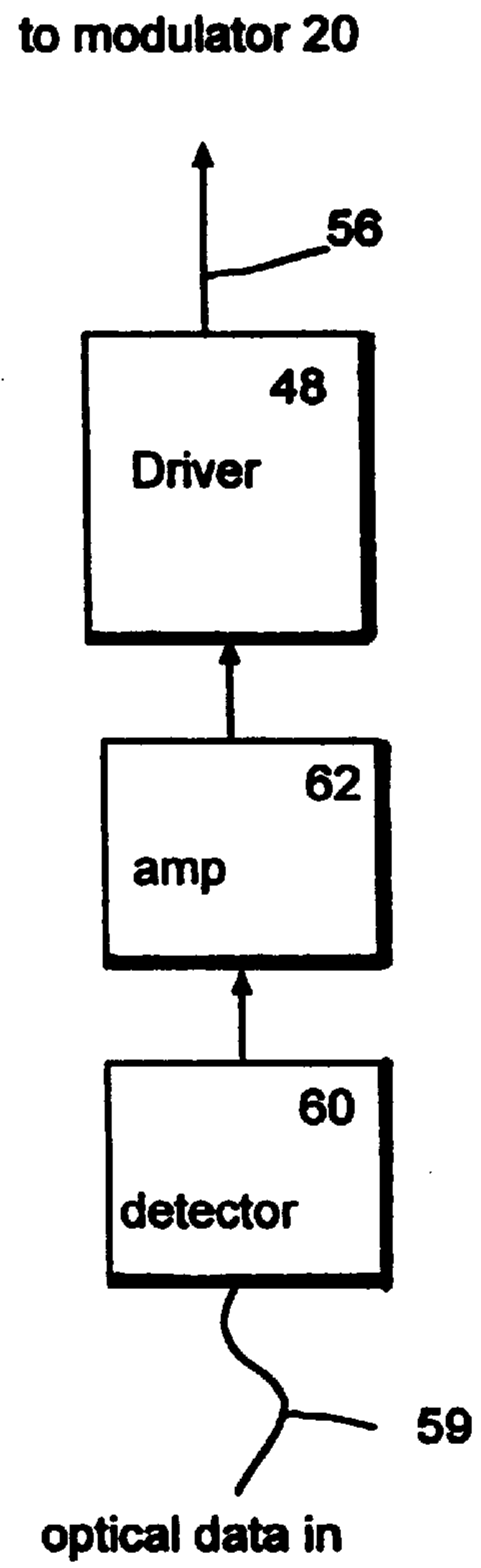
FIG. 3B
