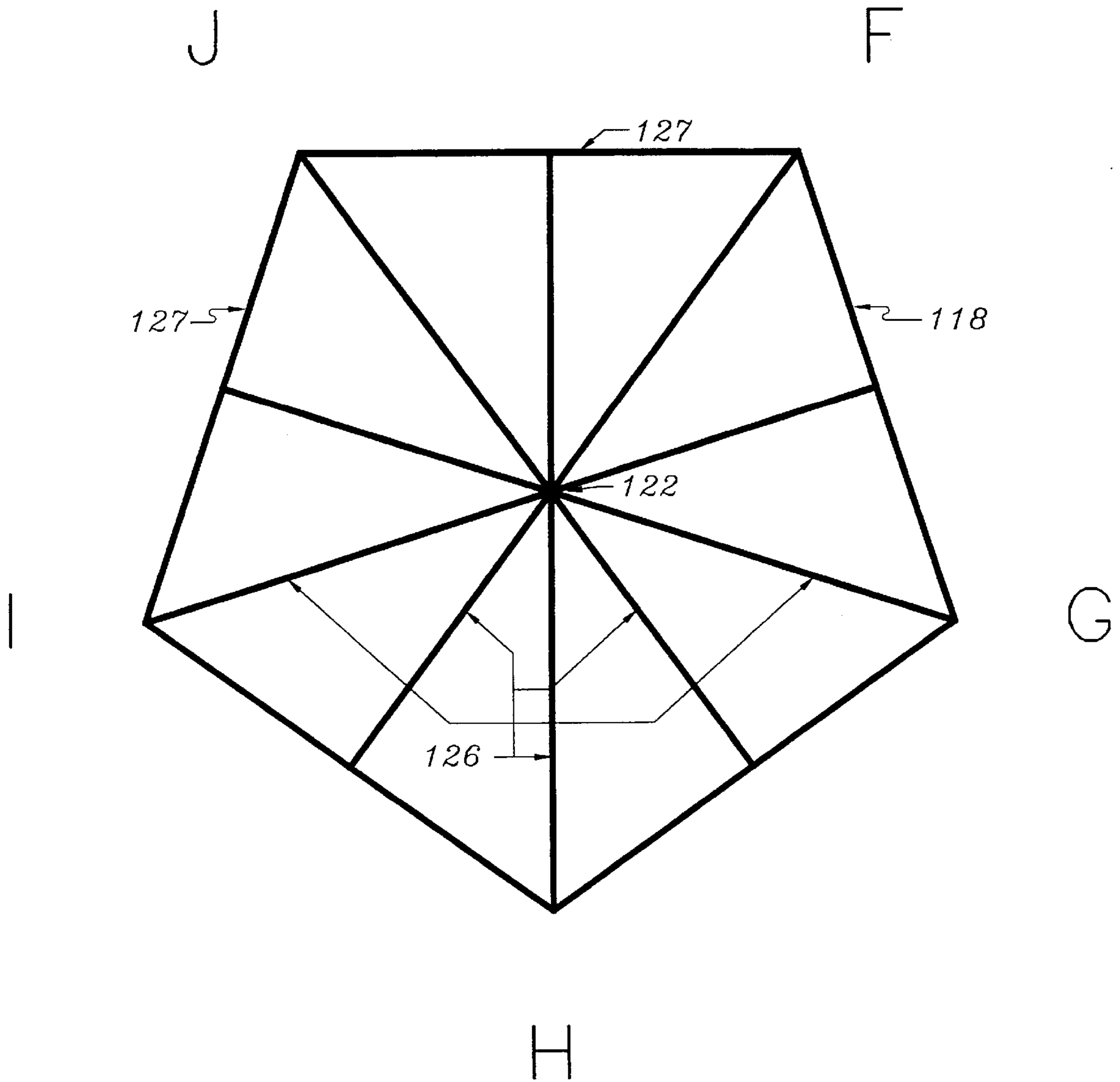
H FIG. 13E
