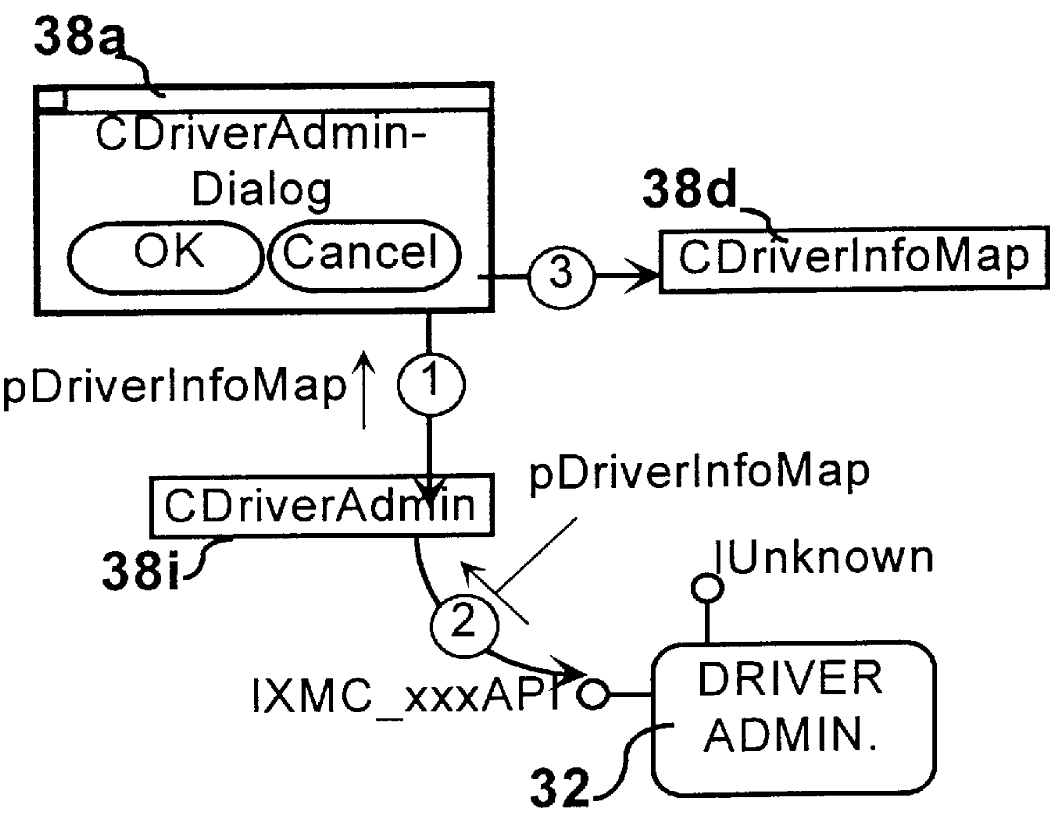
FIG. 54 Scenario-Map - Main Dialog Init.
