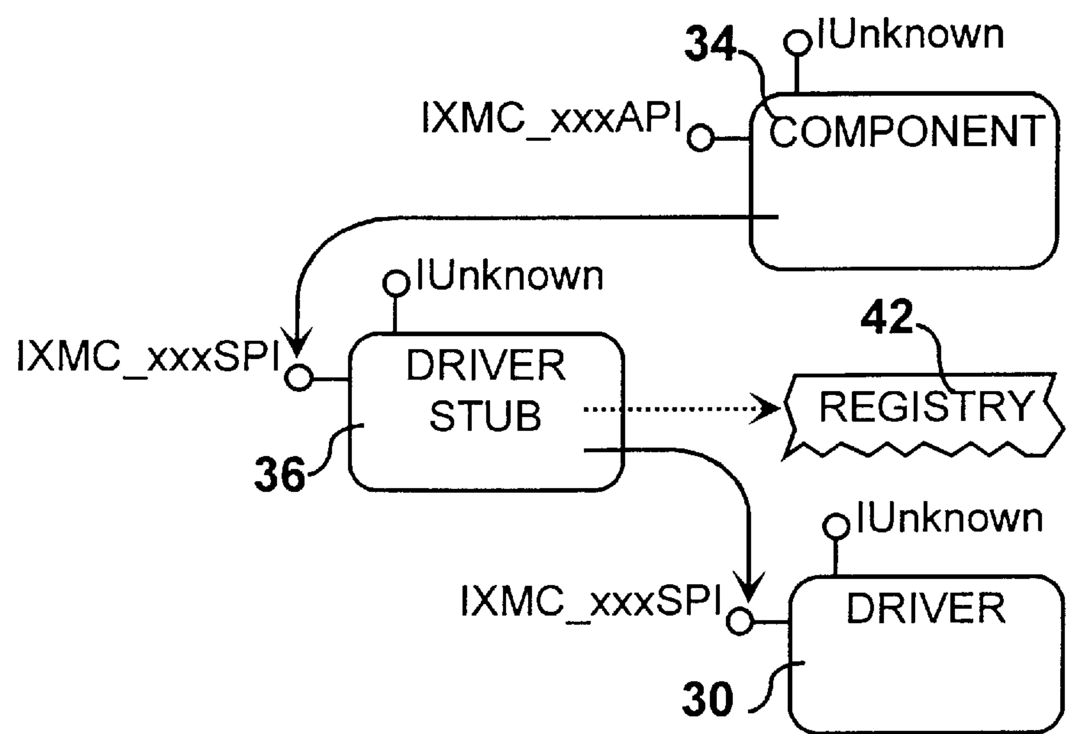
FIG. 34 Module Interaction-Map.
