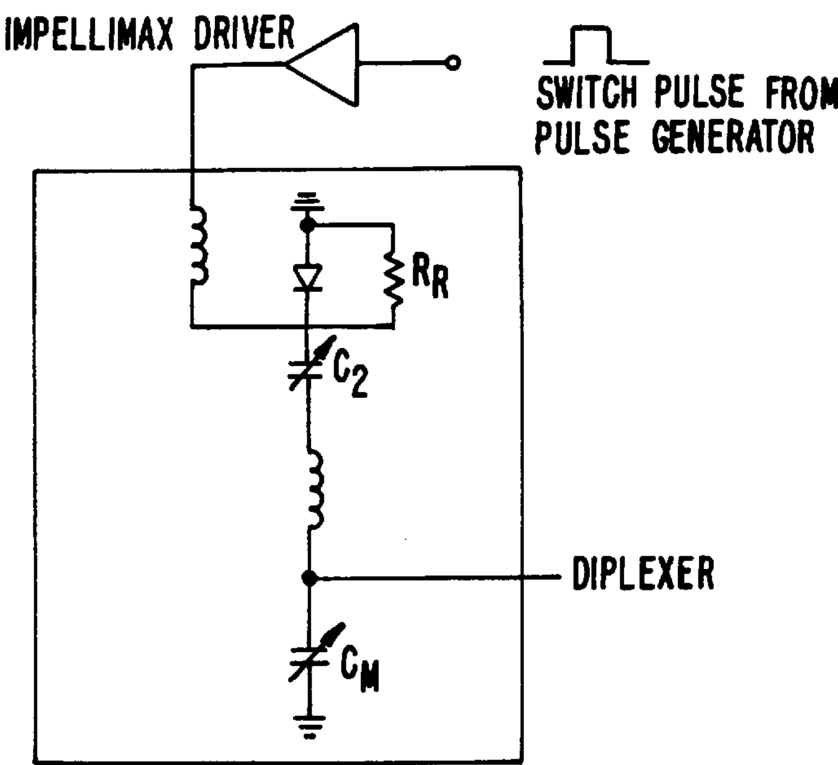
FIG. 2E. Q - SWITCHING
