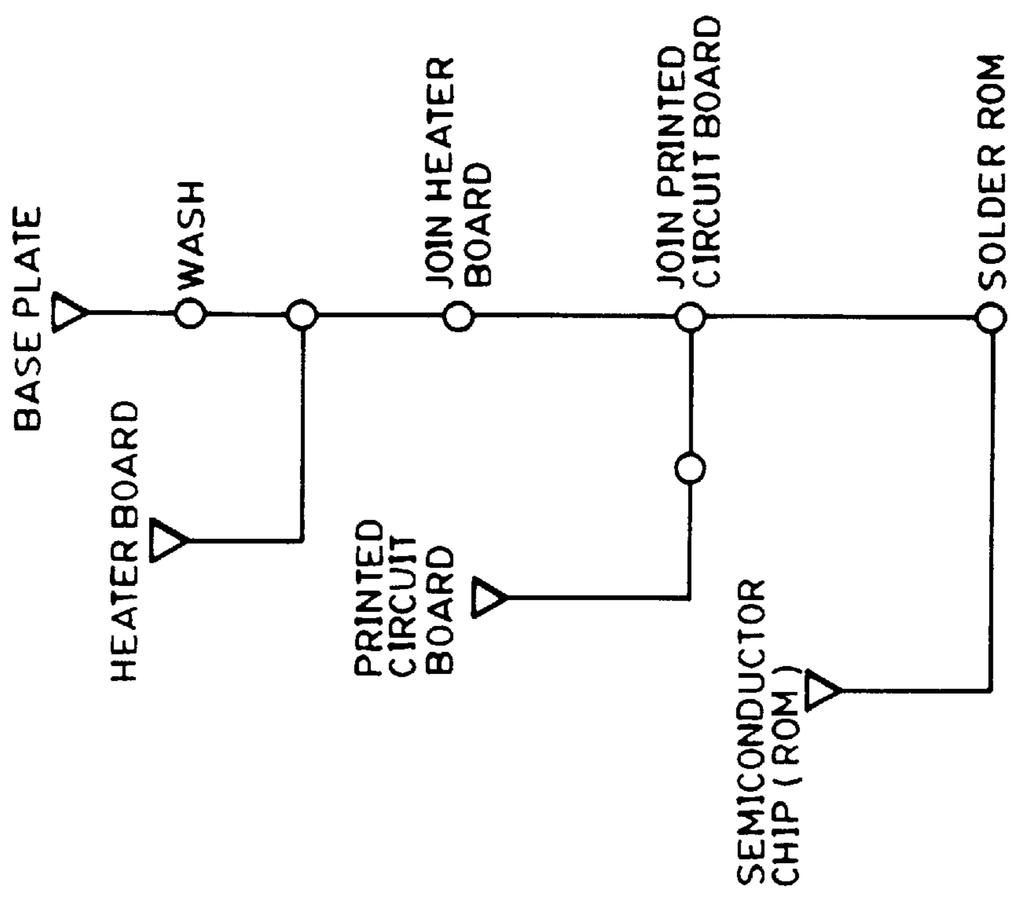
FIG. 12(e) PRIOR ART
