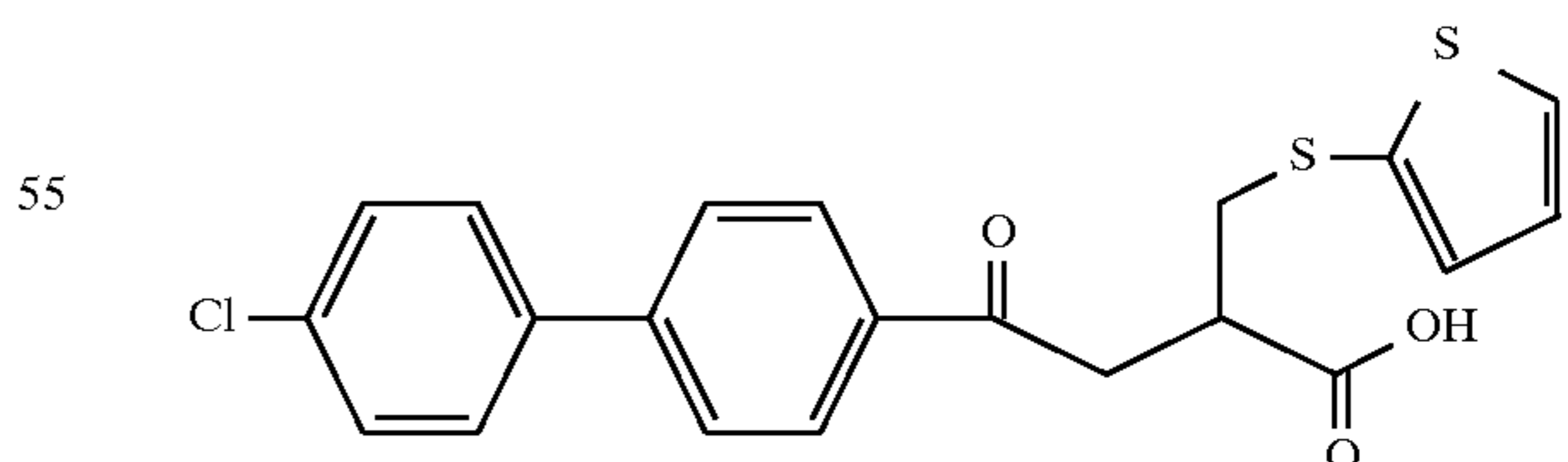
Example 129
