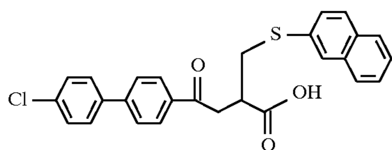
Example 156
