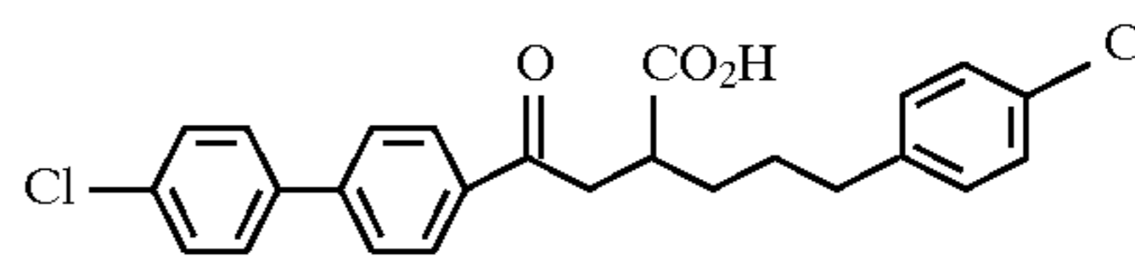
Example 113
