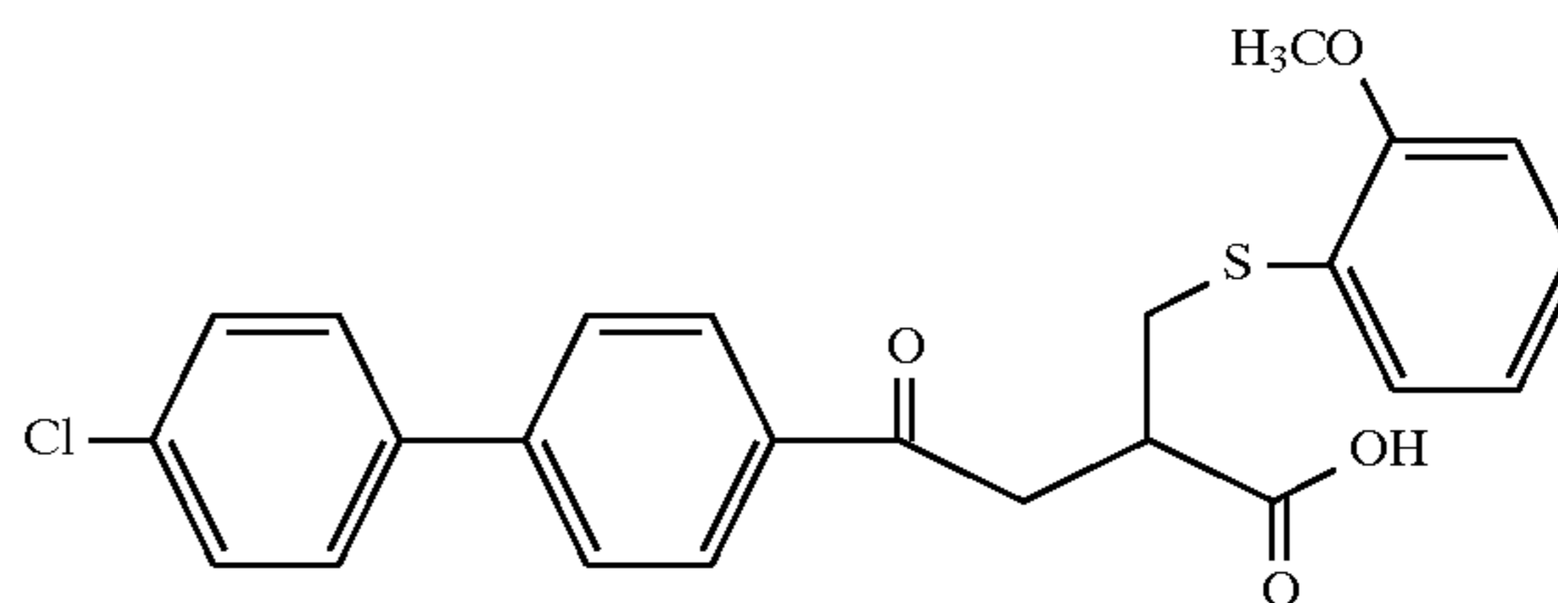
Example 159
