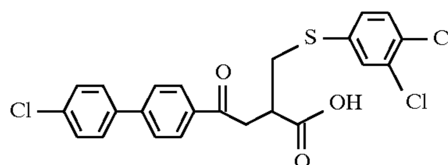
Example 146
