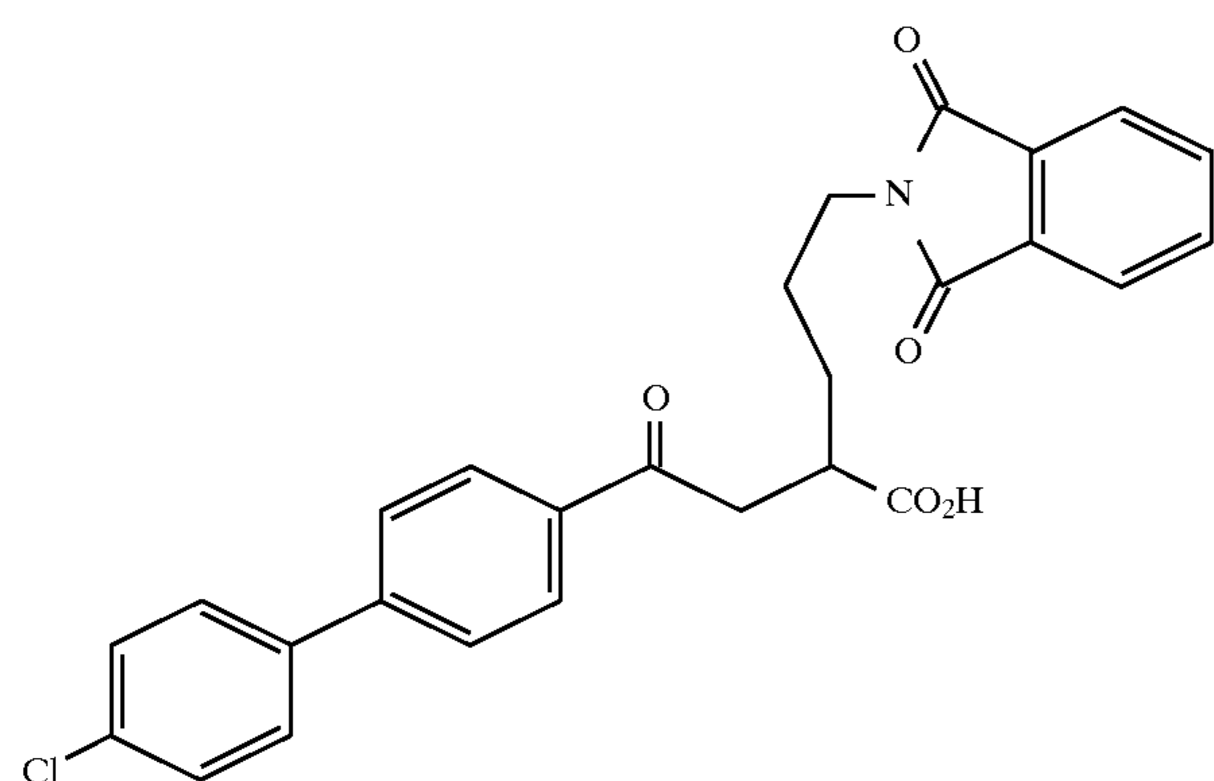
Example 189
