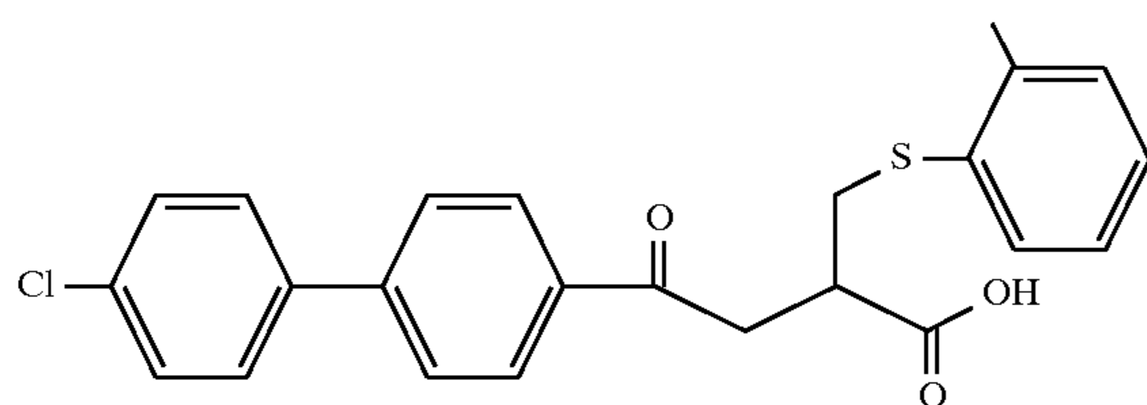
Example 162
