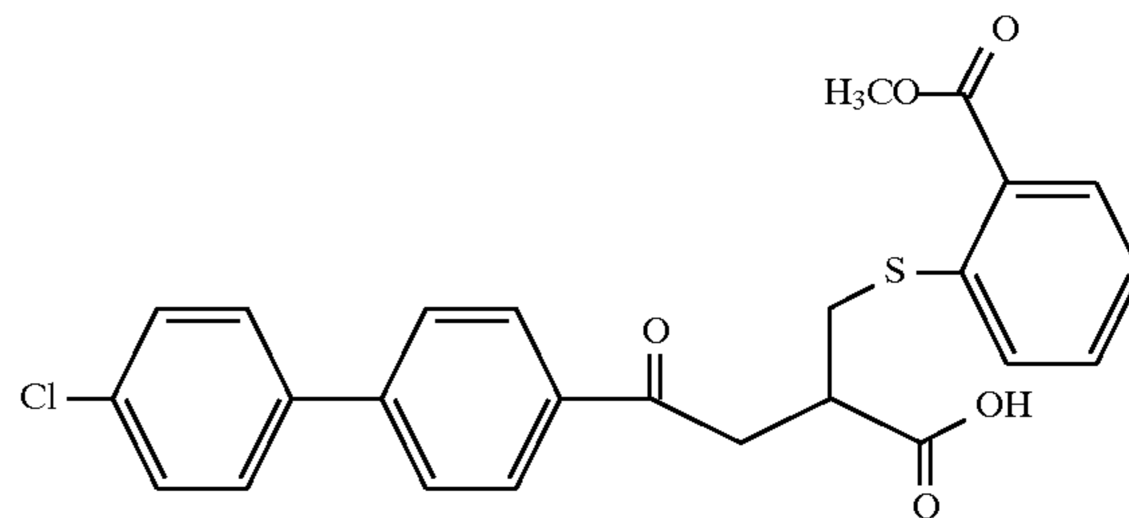
Example 174
