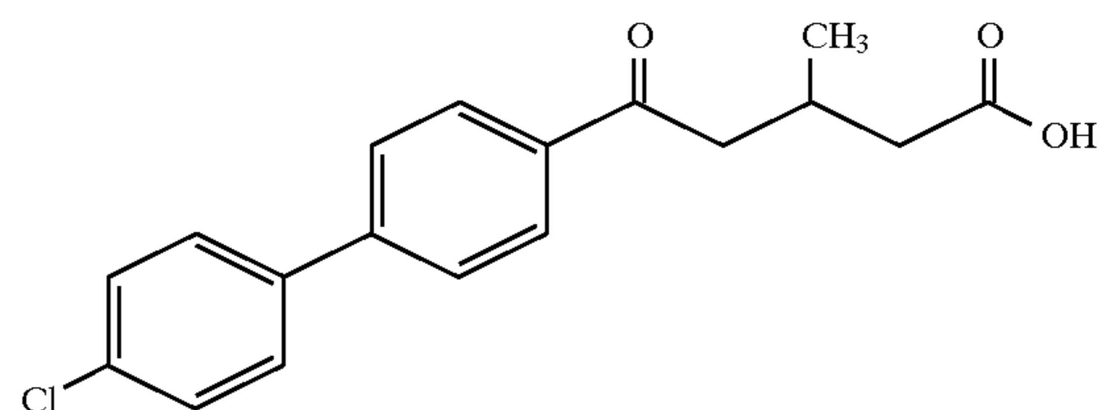
Example 235
