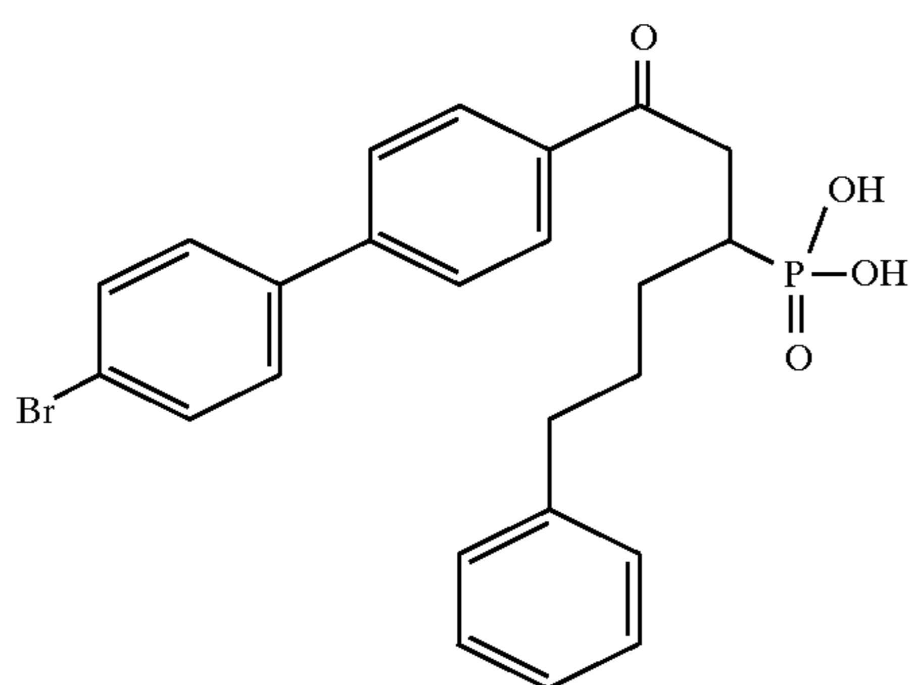
Example 246
