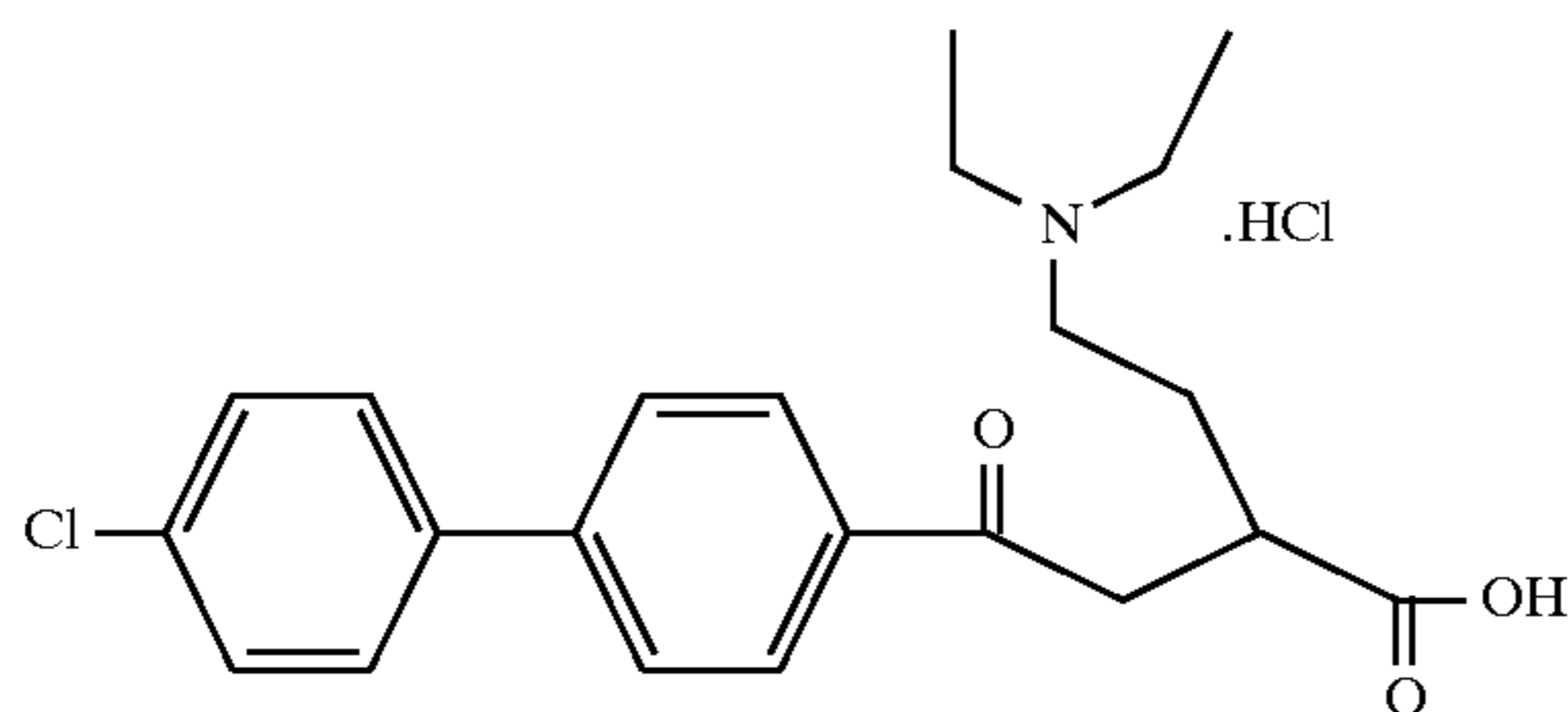
Example 191
