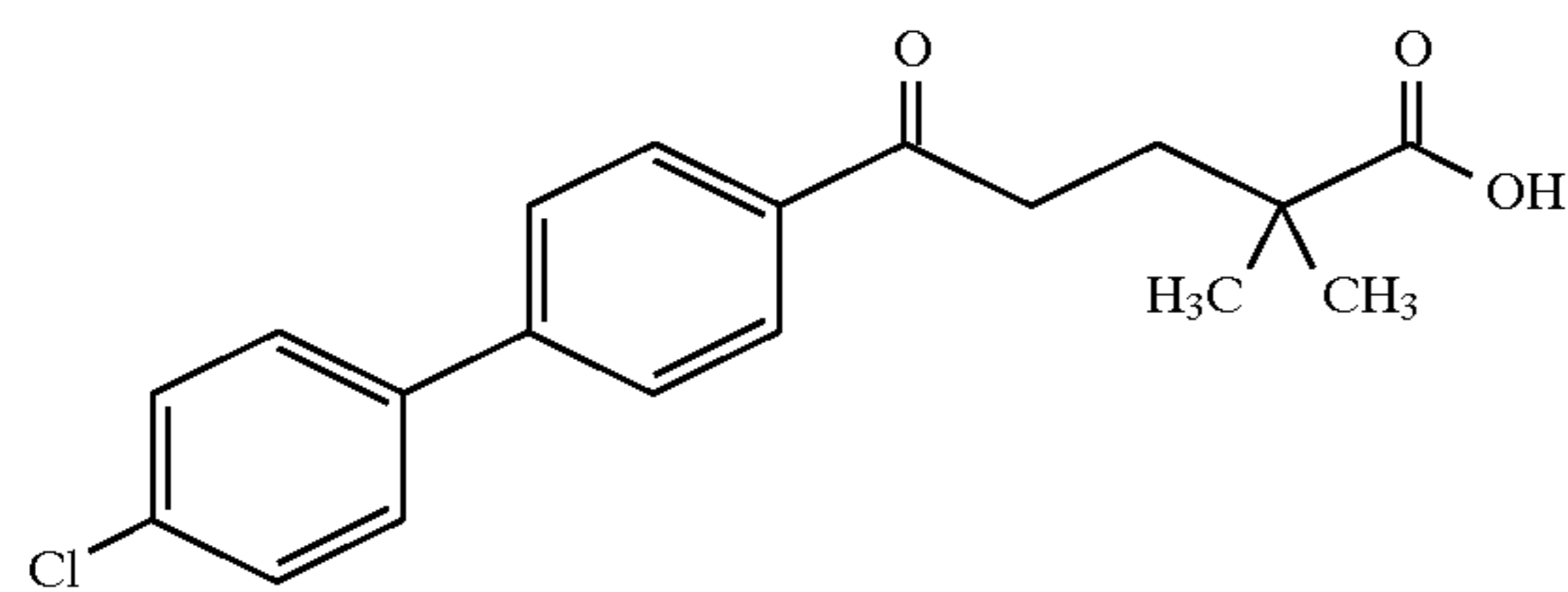
Example 238
