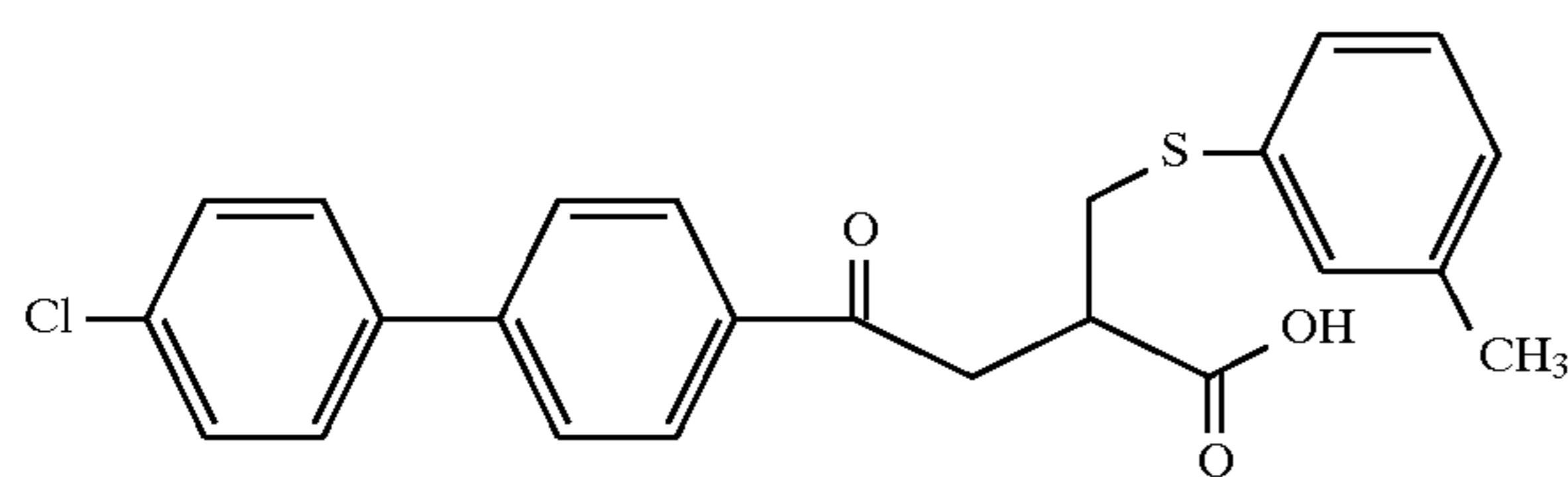
Example 161
