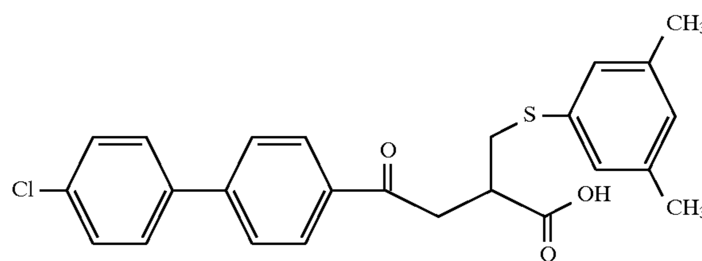
Example 165
