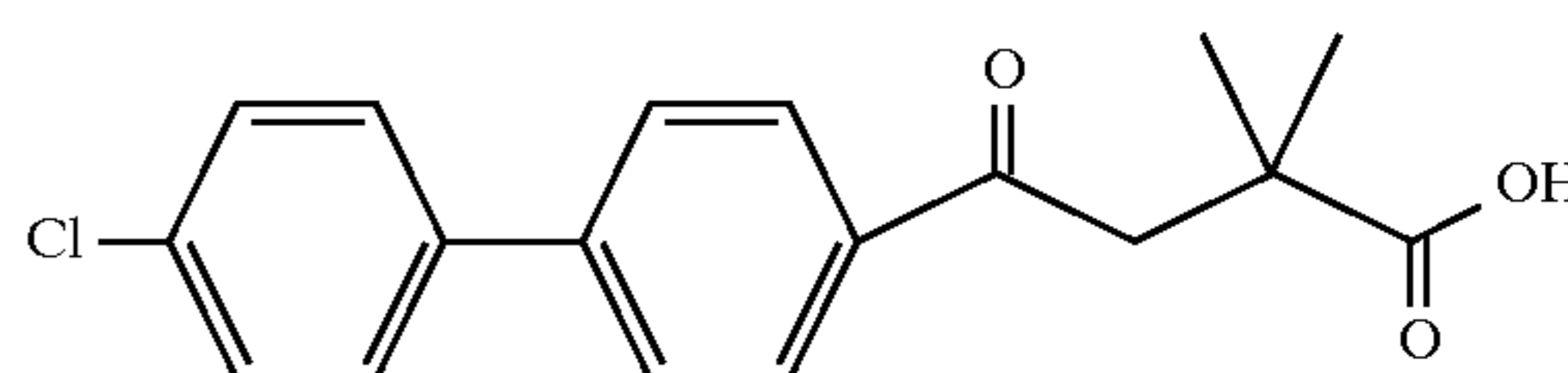
Example 197
