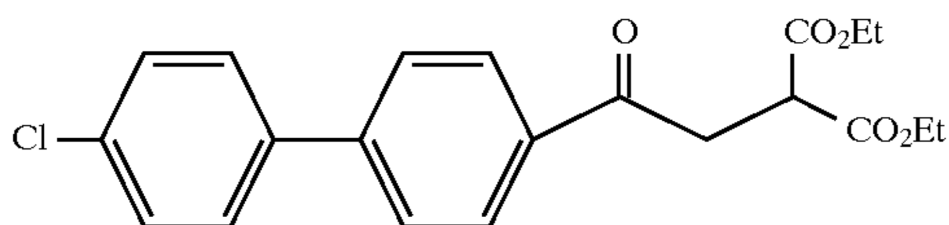
Example 107
