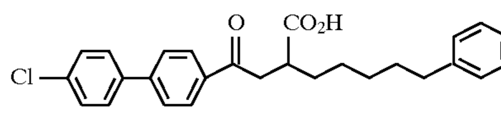
Example 108
