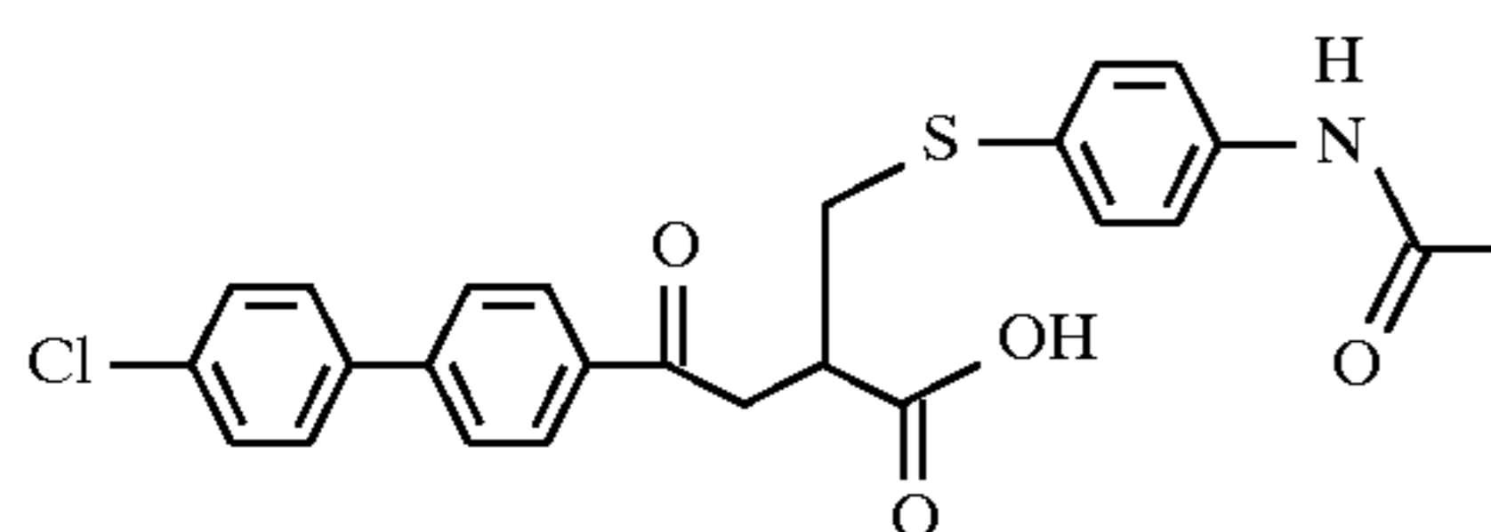
Example 153
