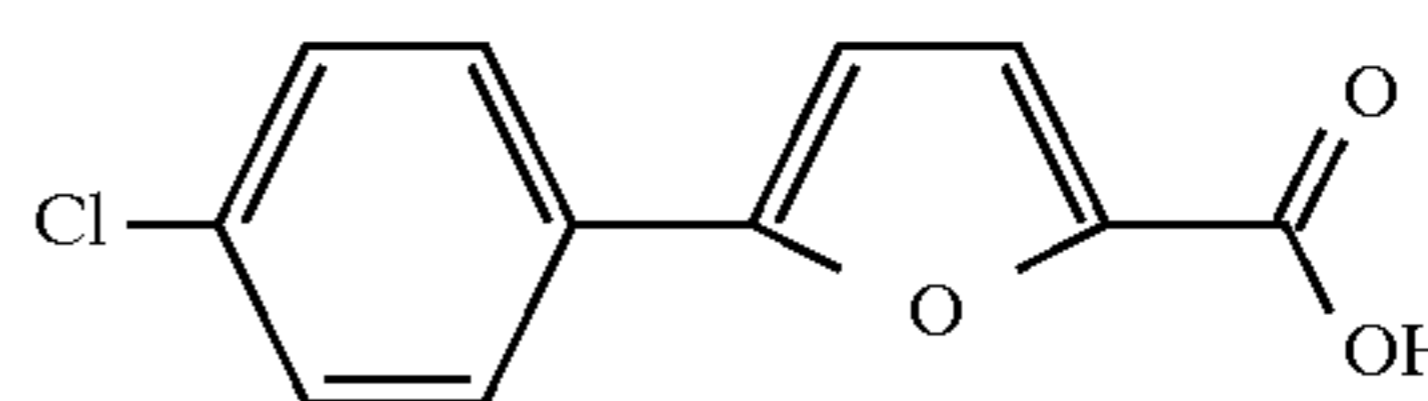
Example 251
