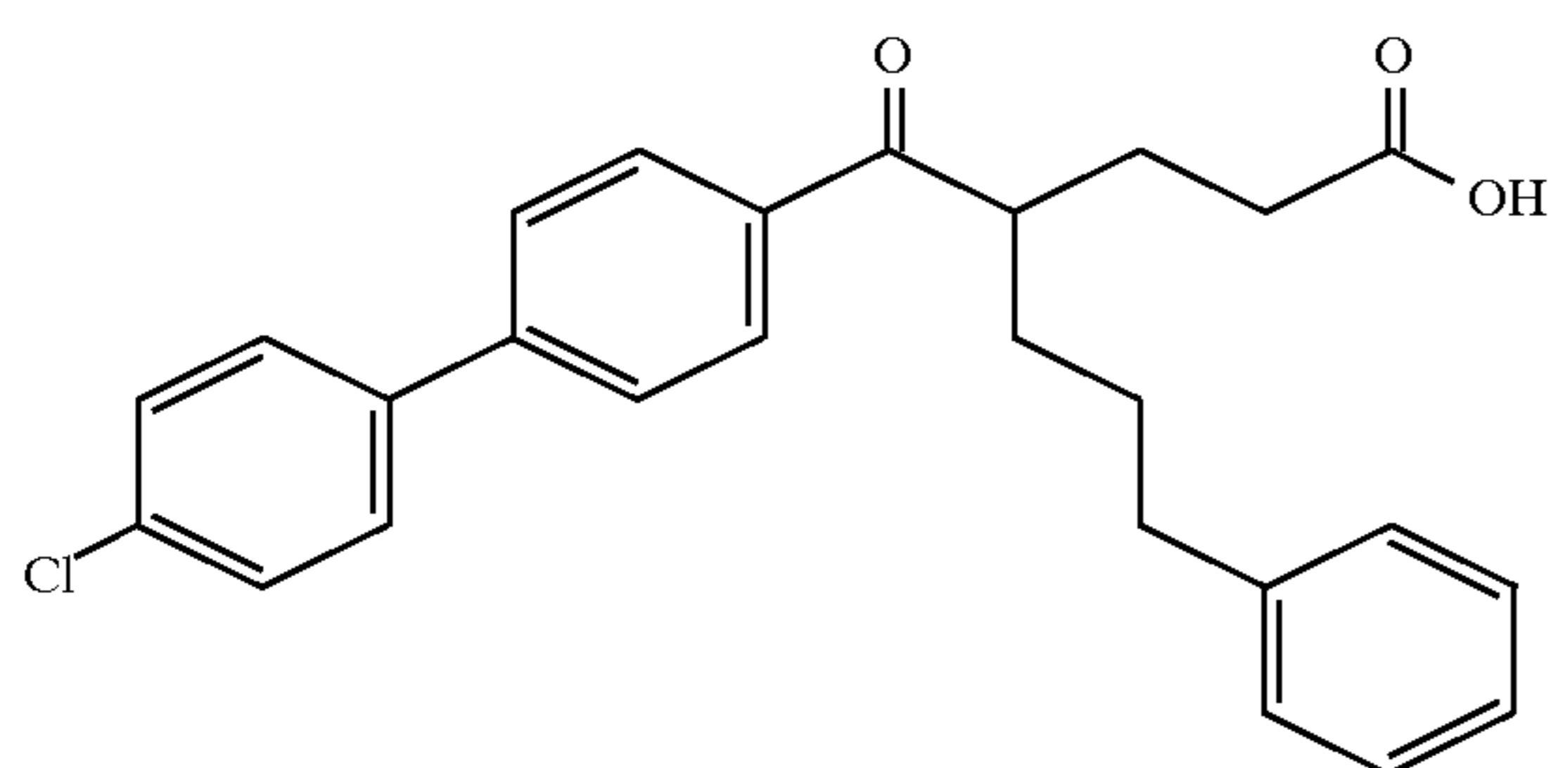
Example 244
