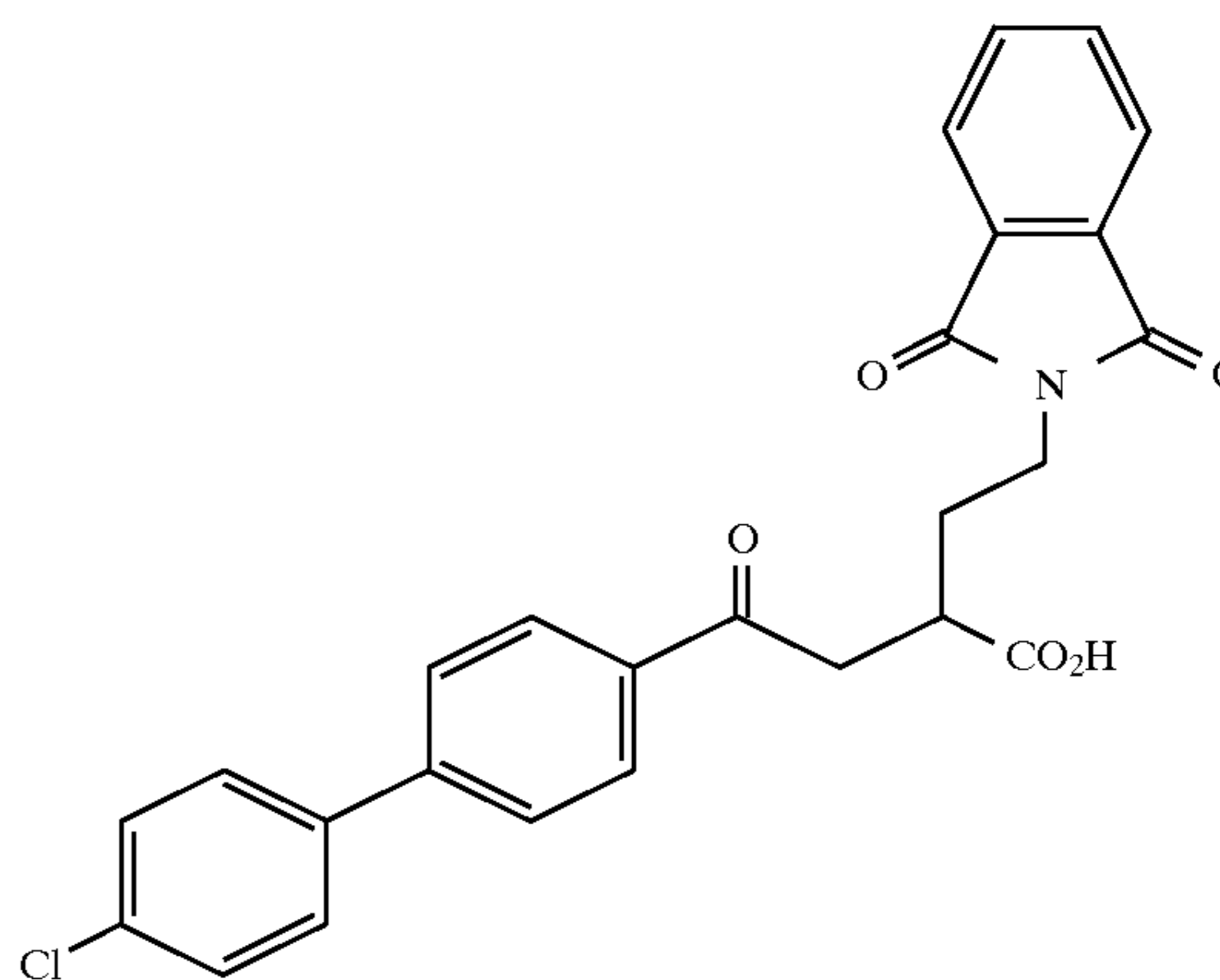
Example 194
