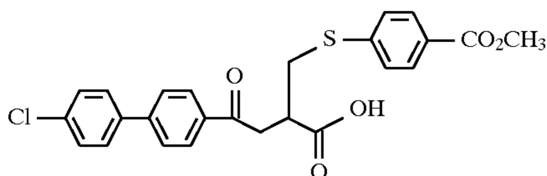
Example 167
