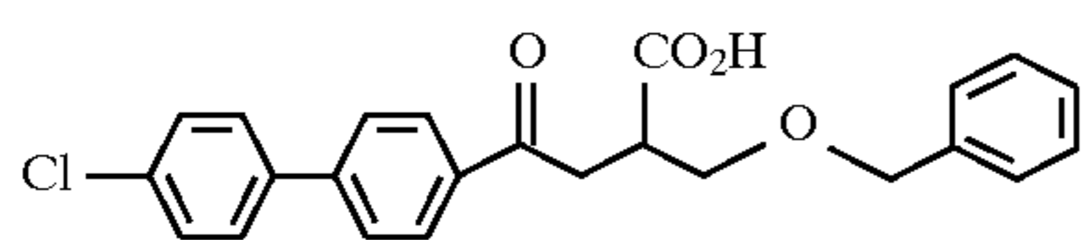
Example 196
