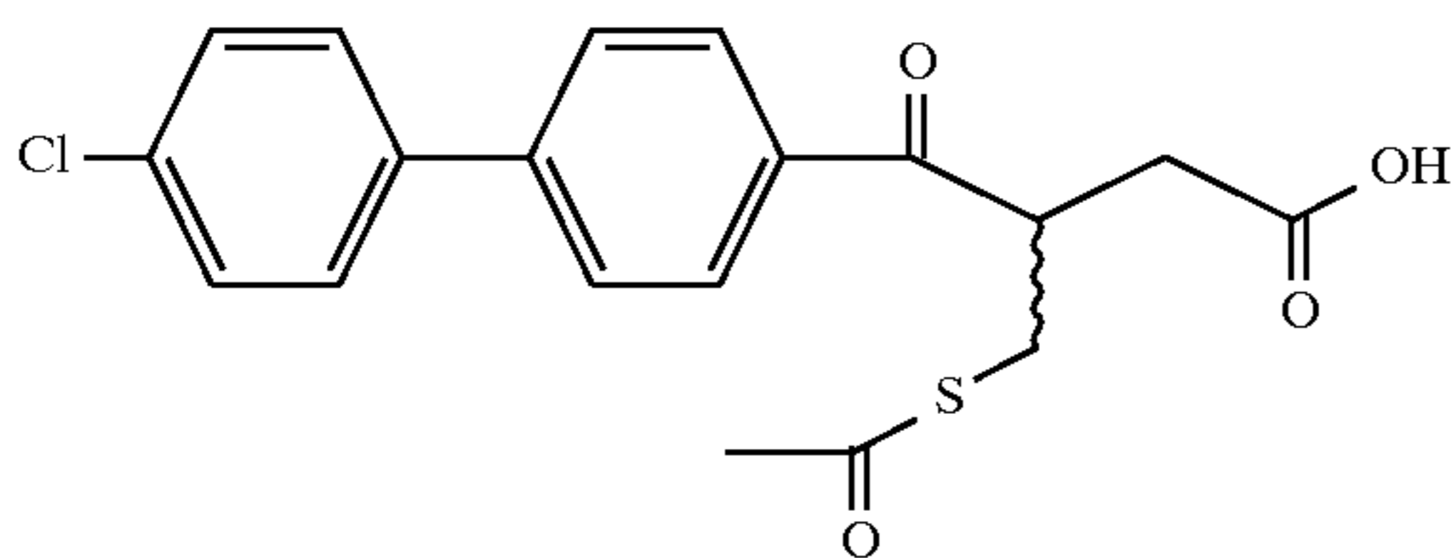
Example 182
