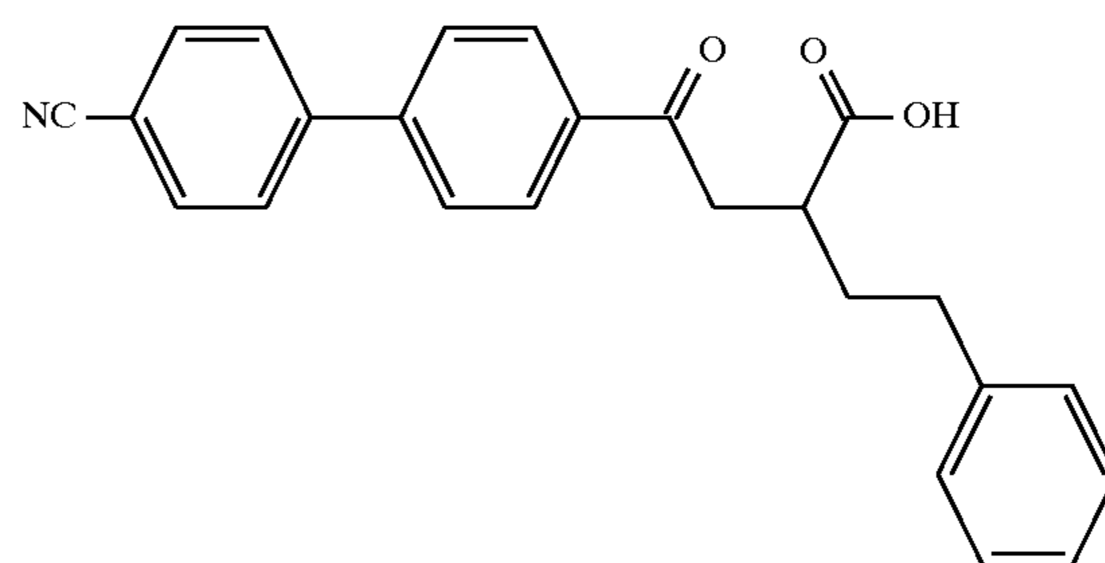
Example 101
