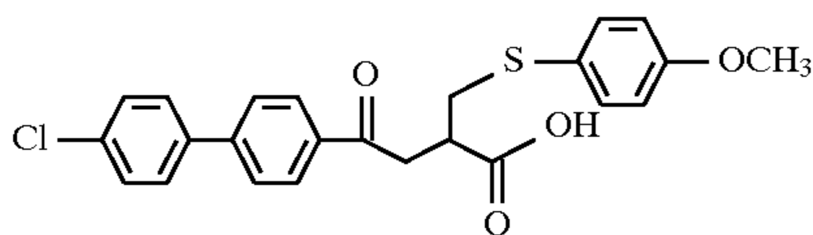
Example 136
