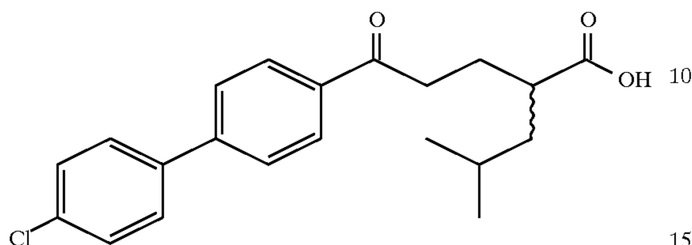
Example 239
