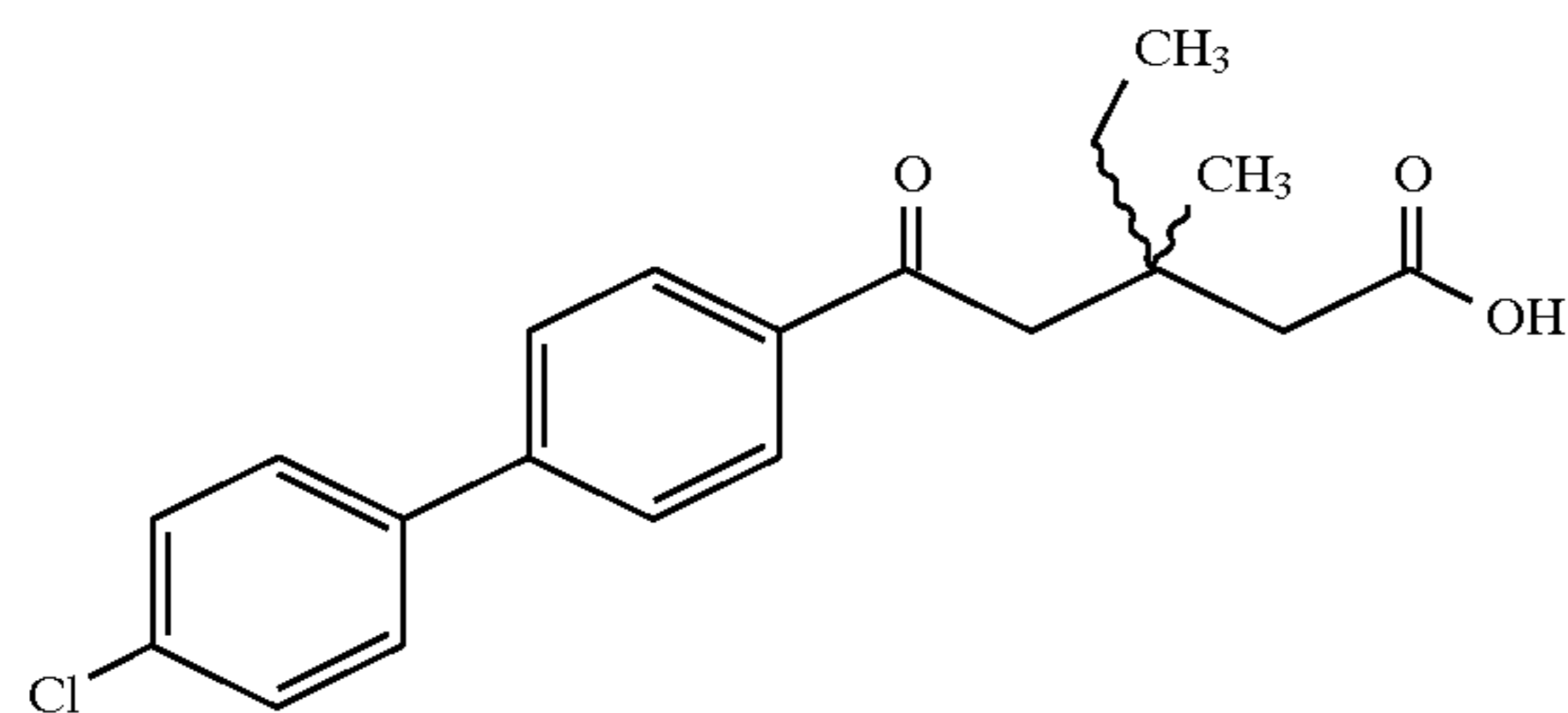
Example 237
