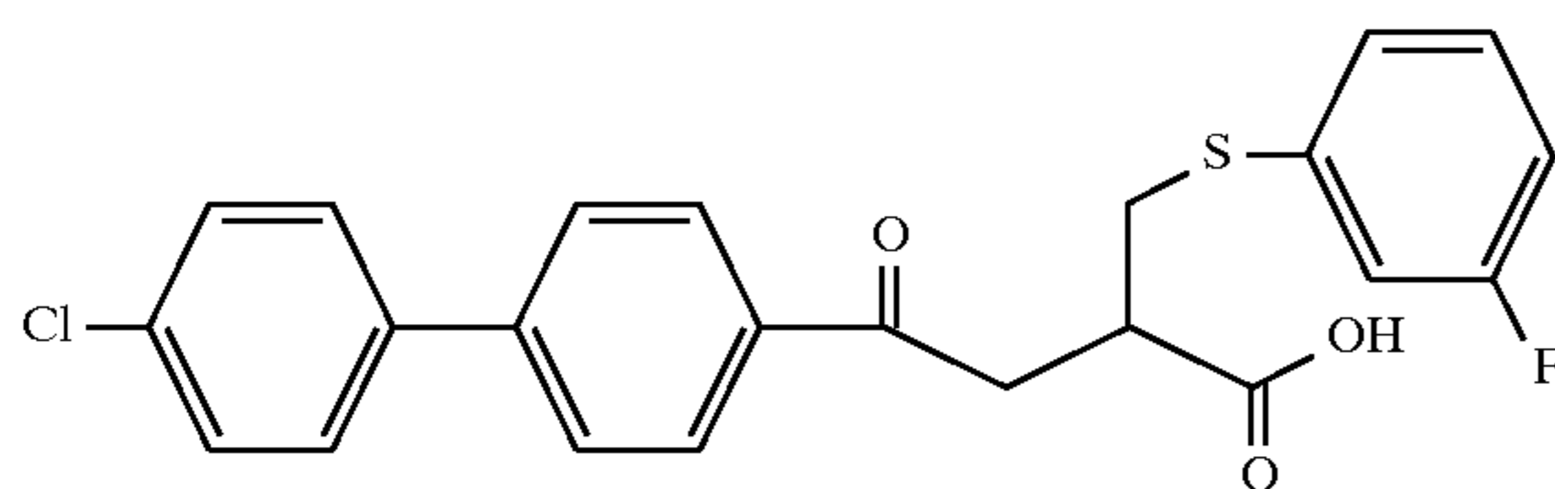
Example 173
