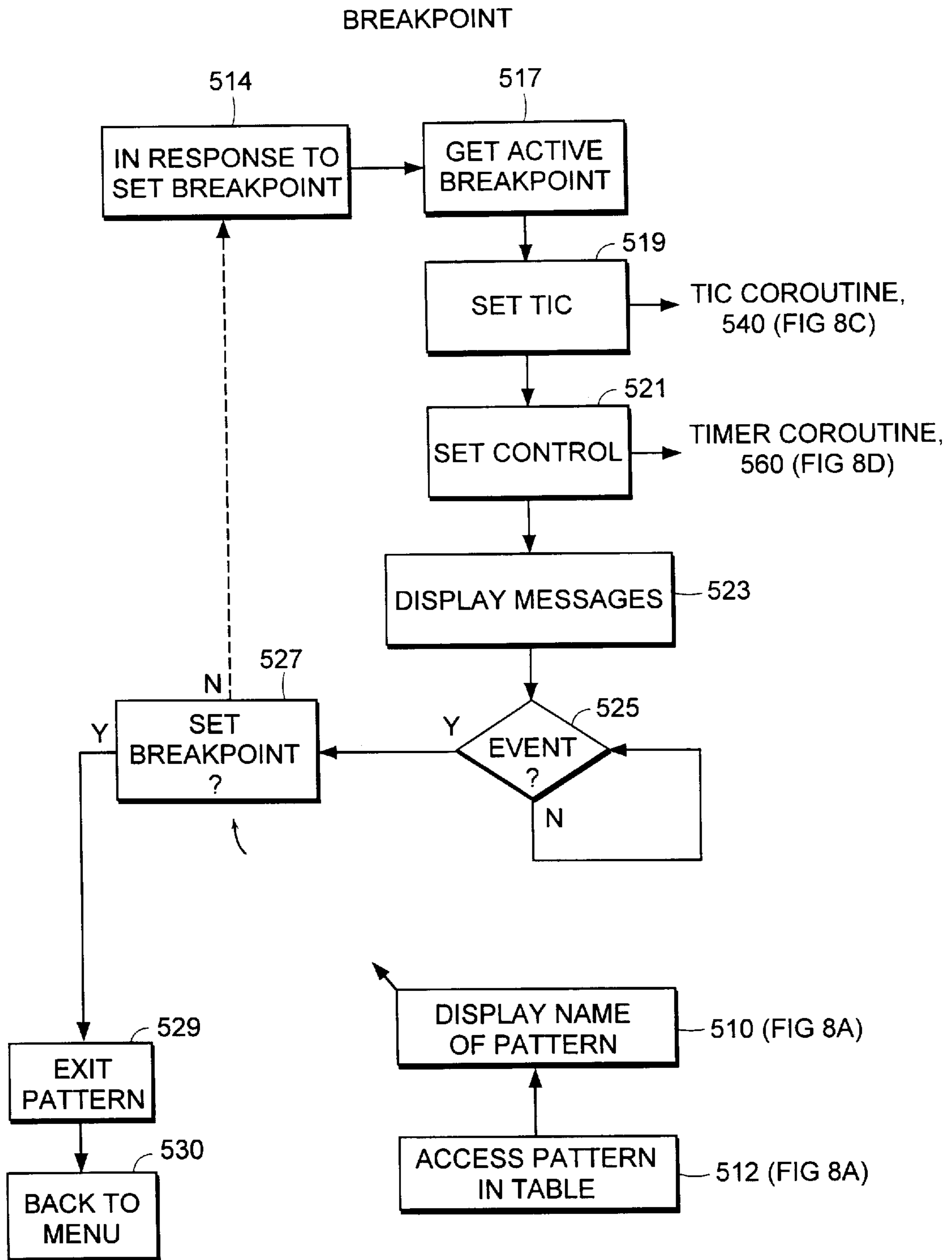
FIG. 8B
