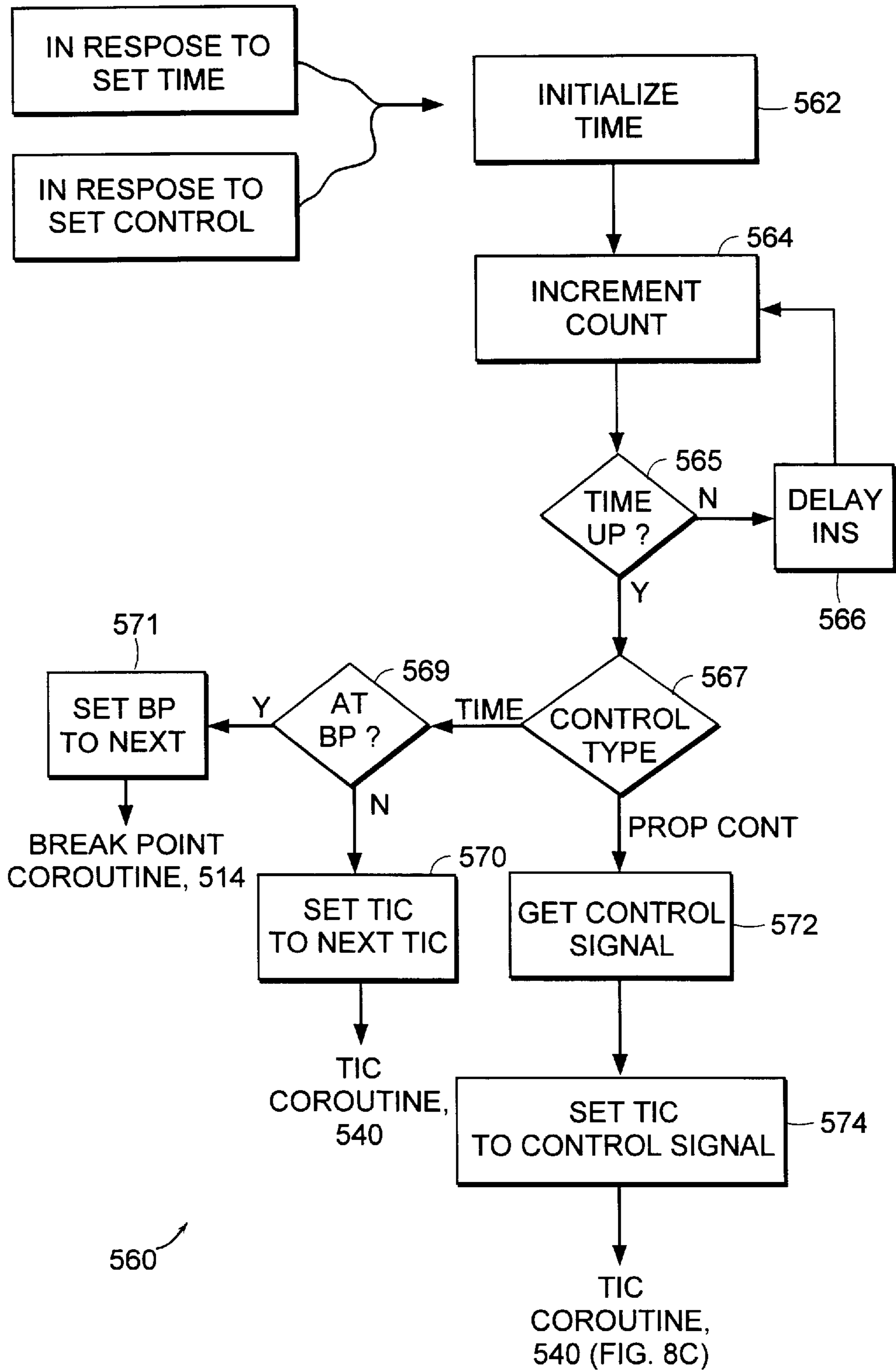
FIG. 8D
