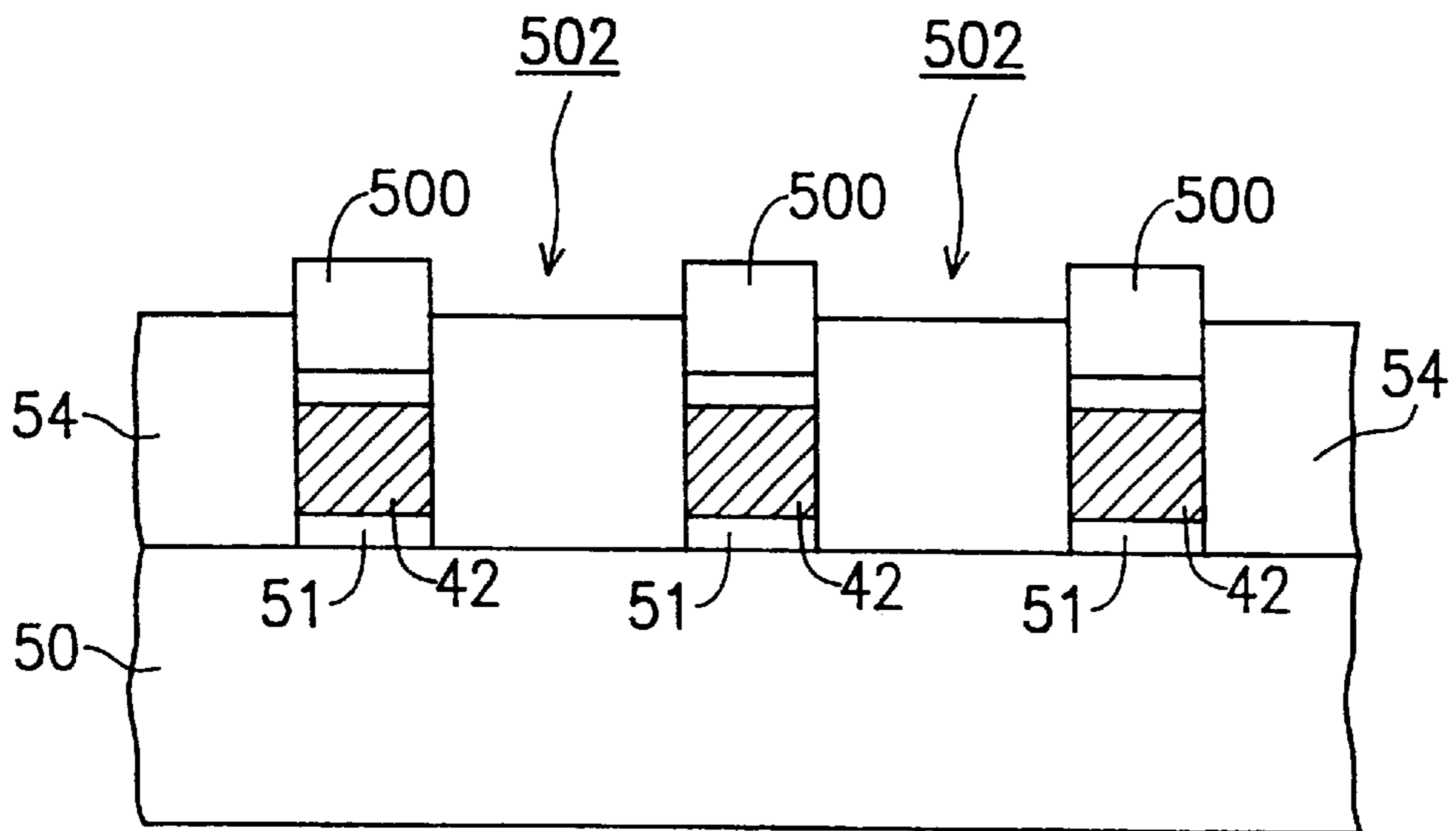
FIG. 5A
