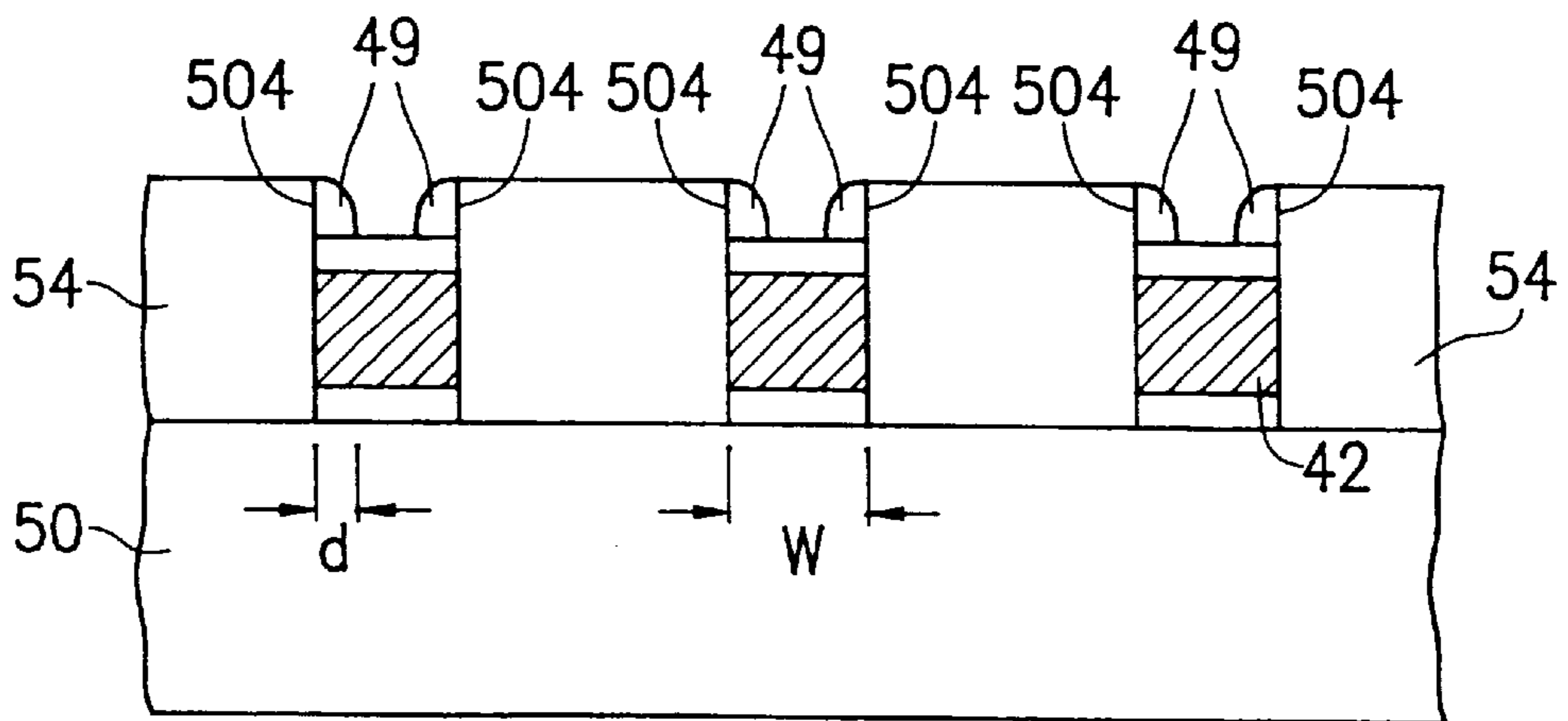
FIG. 5C
