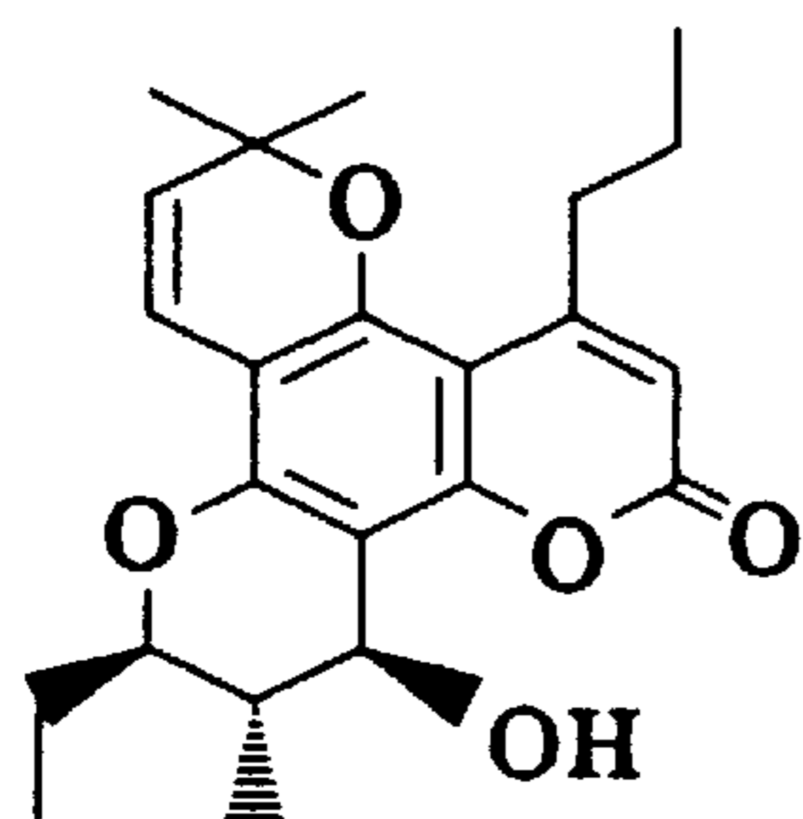
(±)-16f
