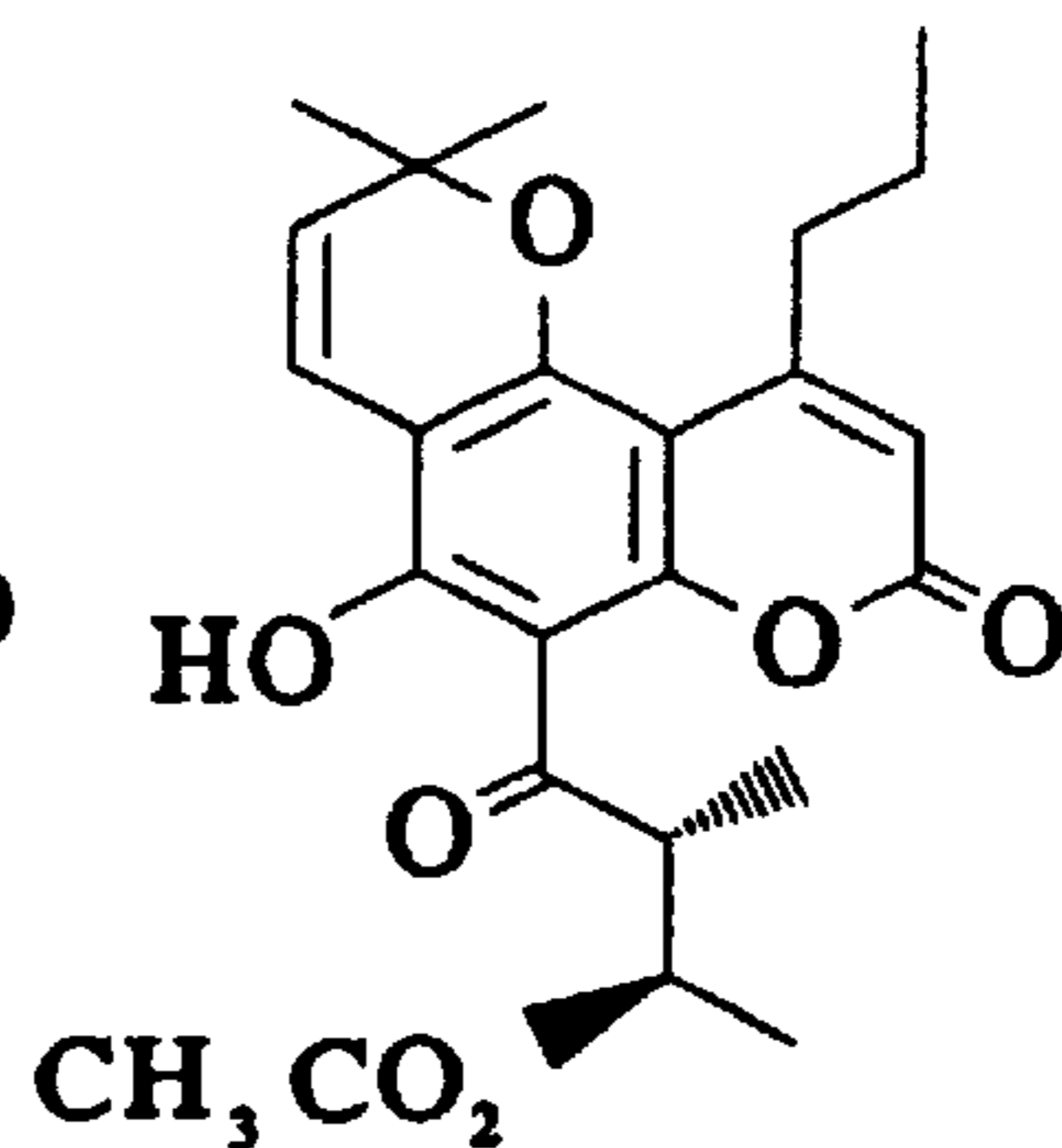
(+)-10
