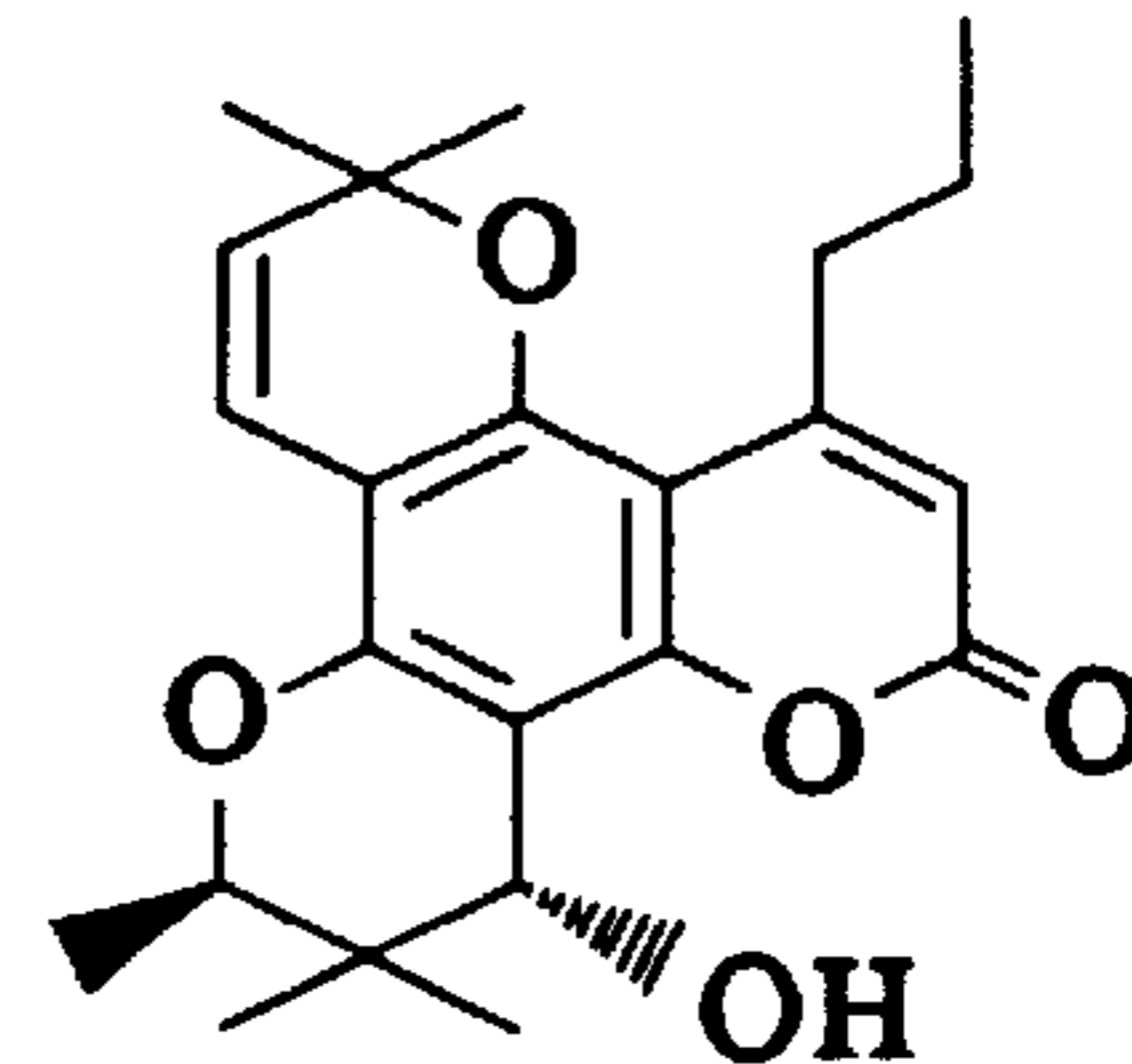
(±)-16b
