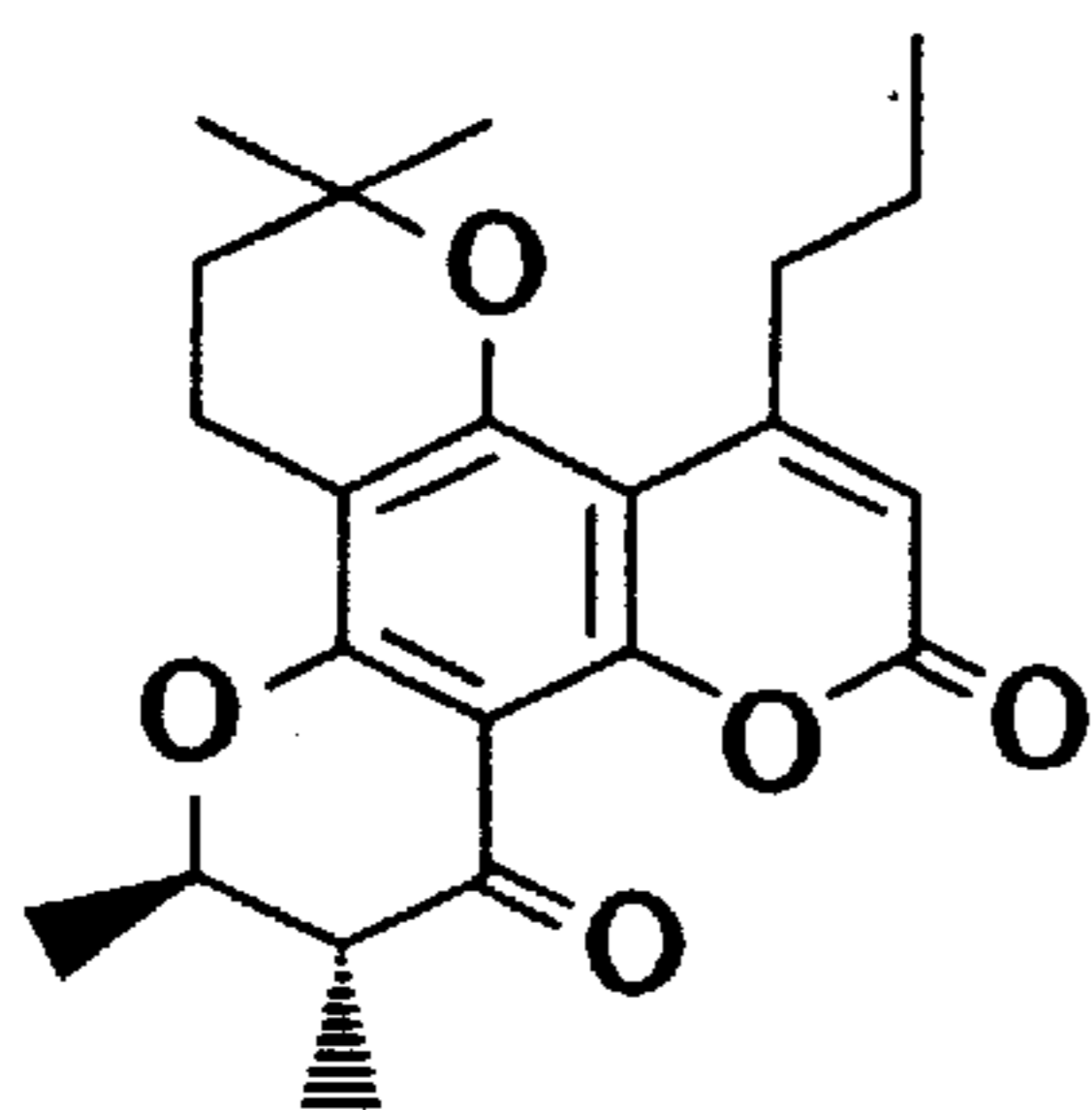
(±)-18a
