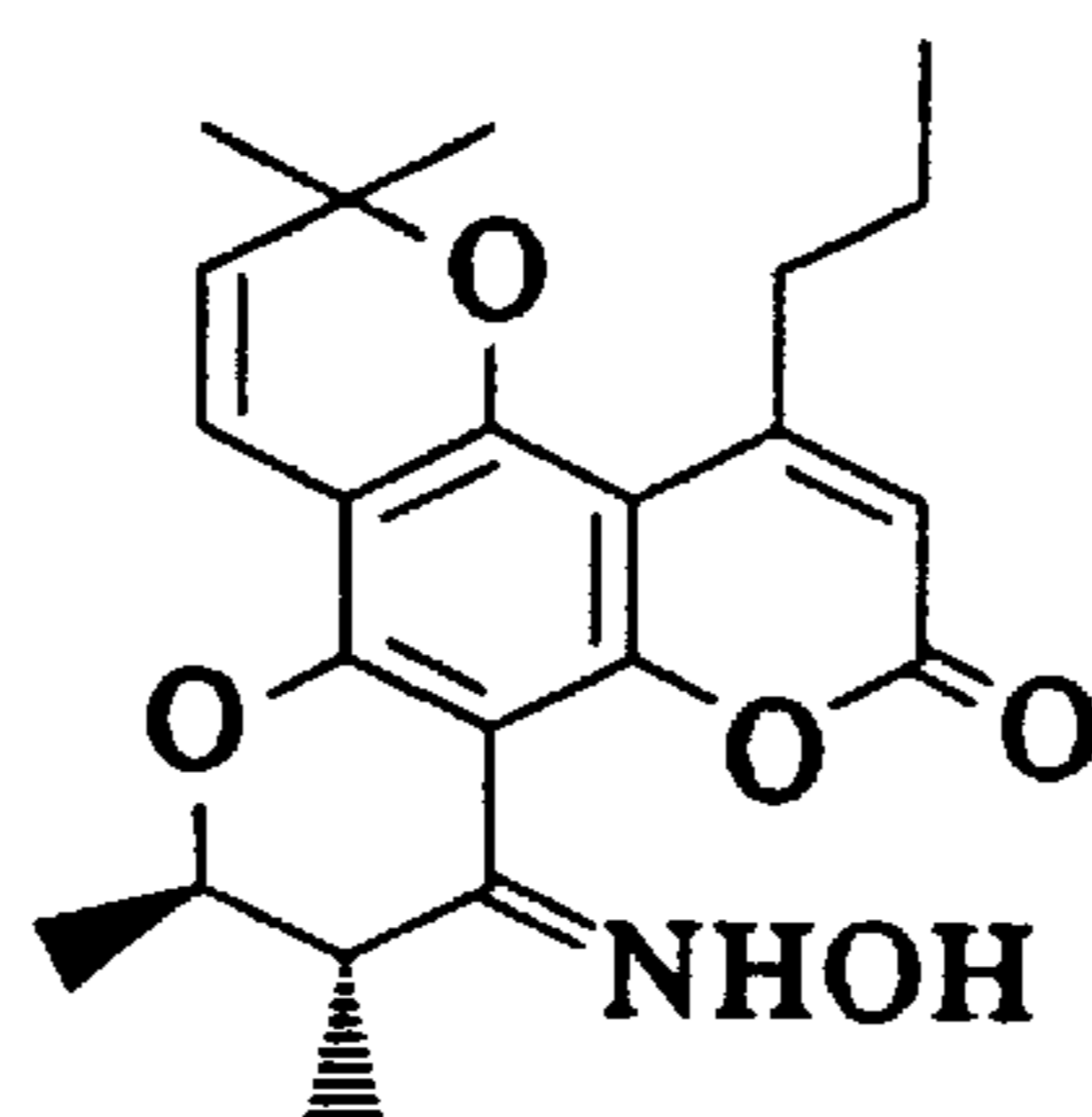
(±)-19a
