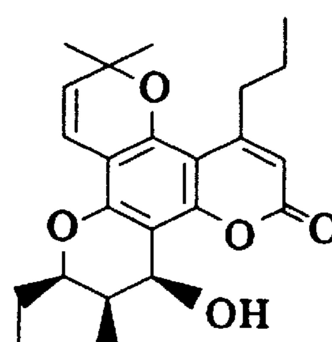
(±)-16h
