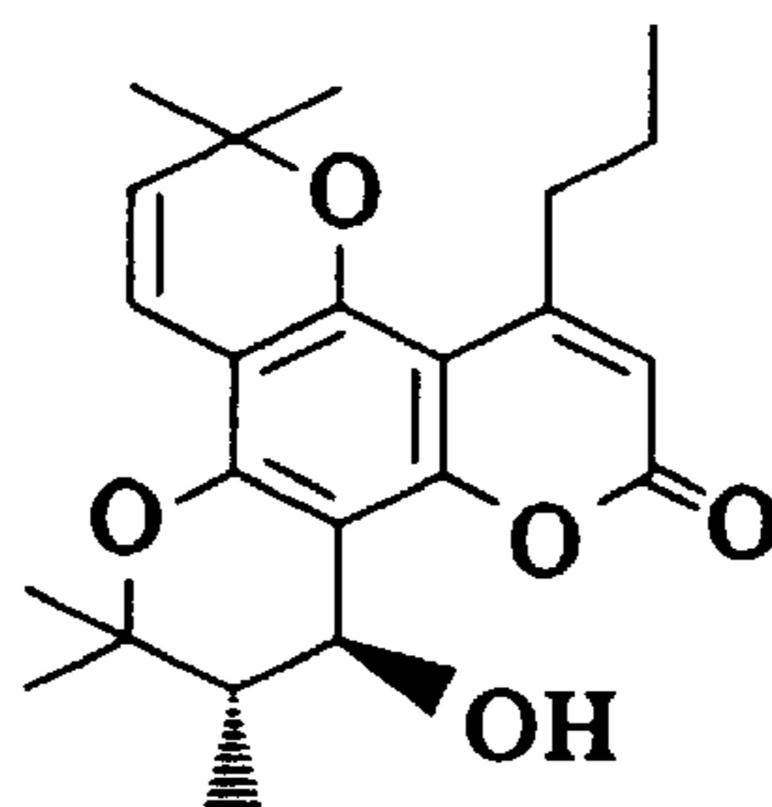
(±)-16d
