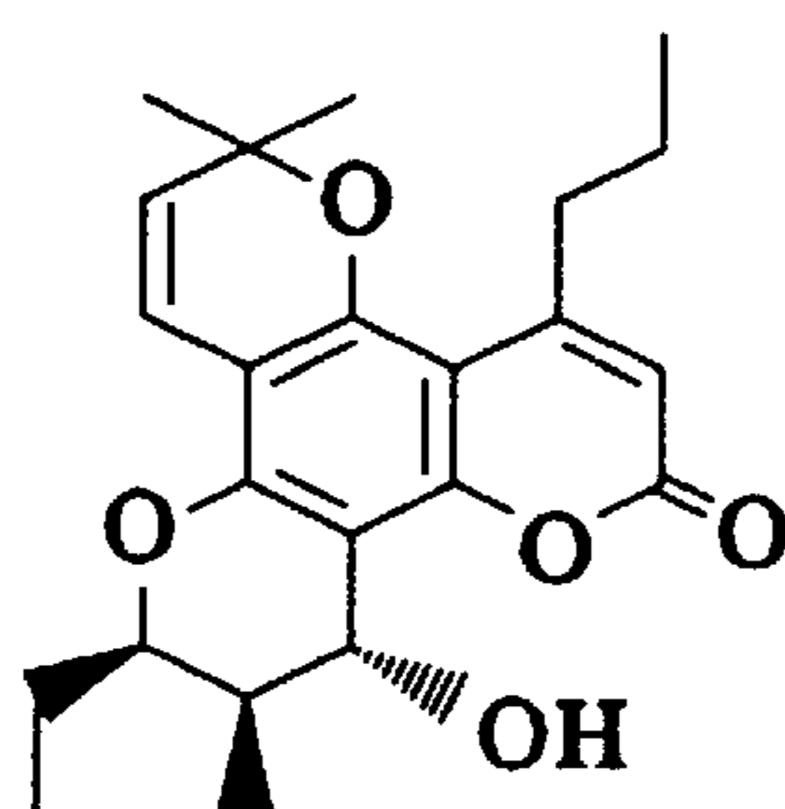
(±)-16g
