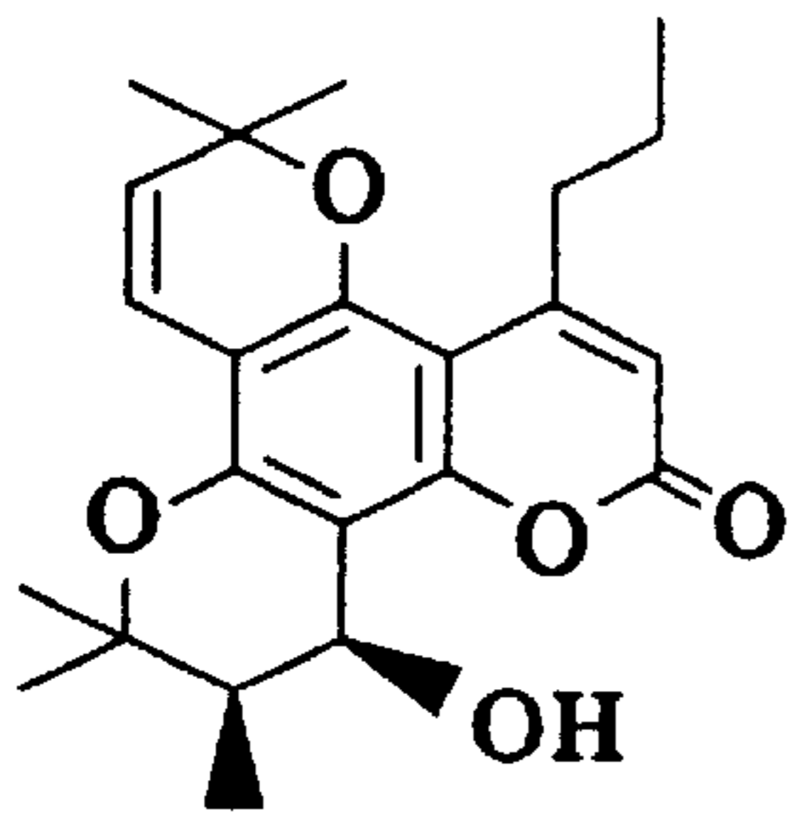
(±)-16c
