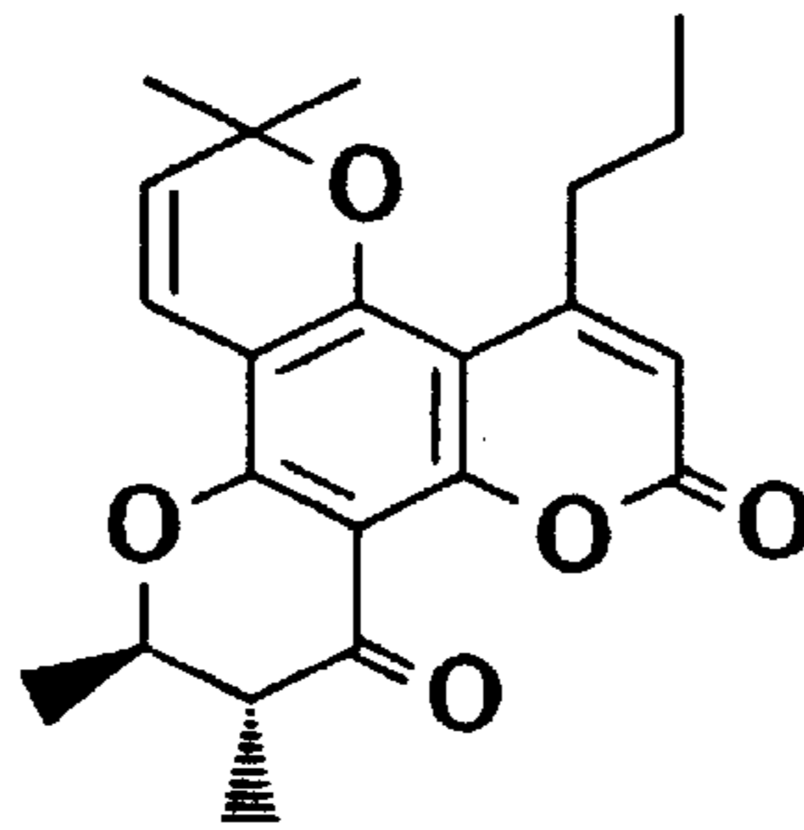
(+)-7
