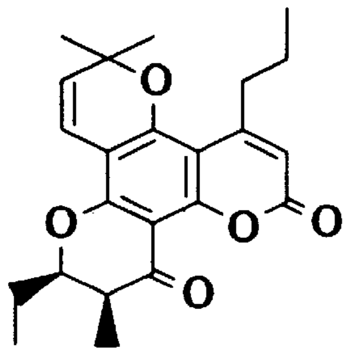
(±)-15d
