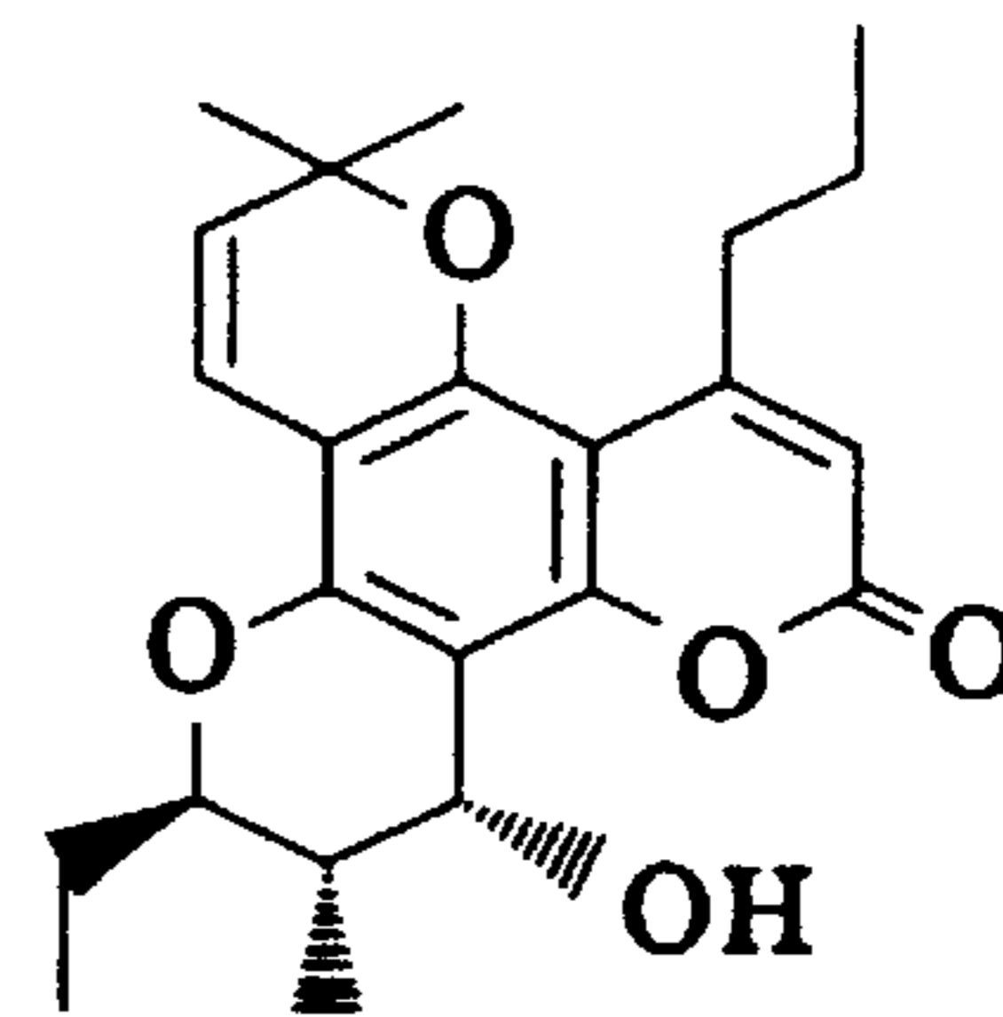
(±)-16b
