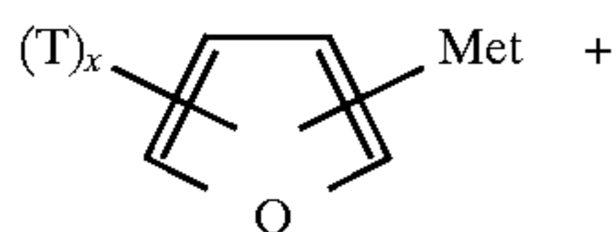
XXVI-B
