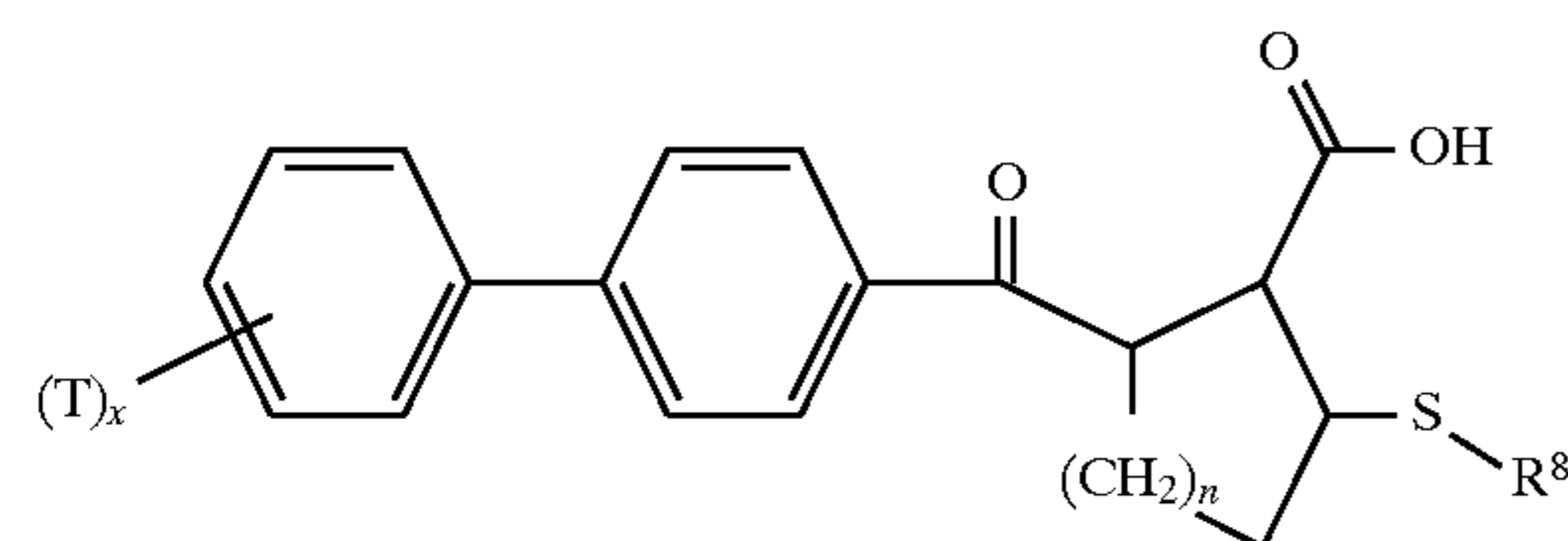
I-I-1
