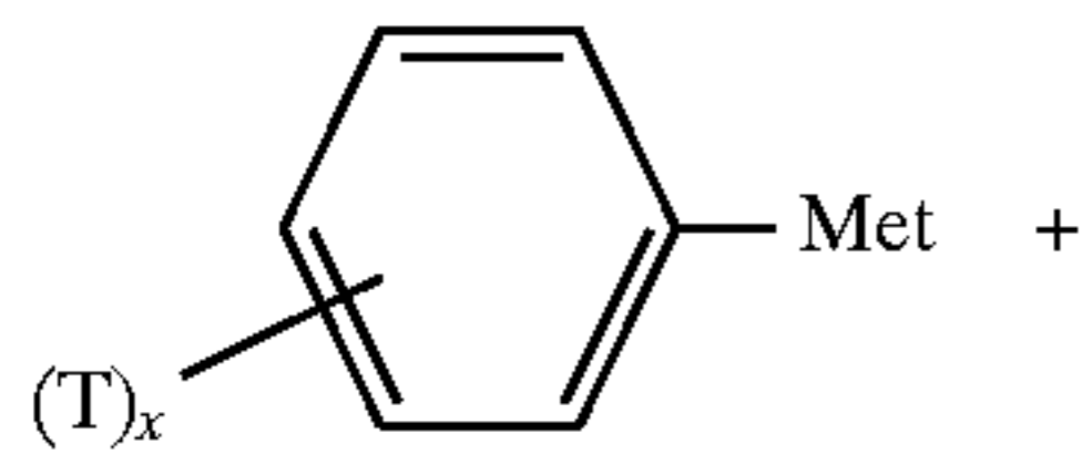
XXVI-A
