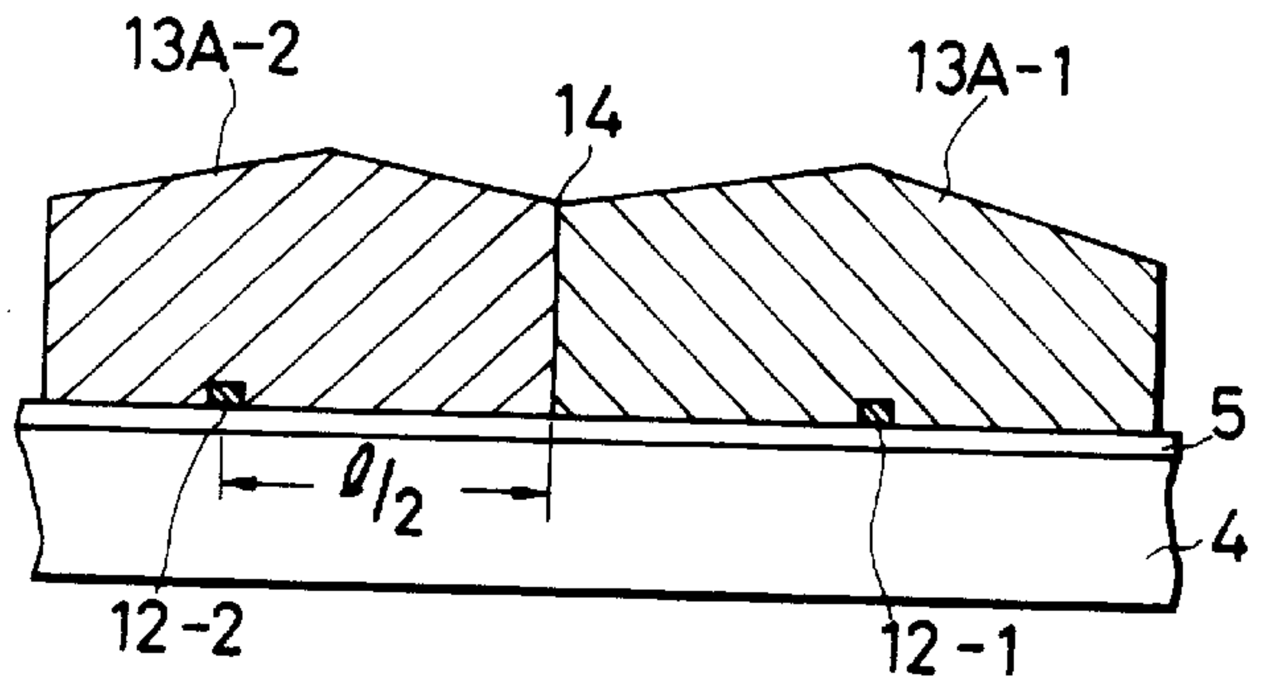
FIG. 9C
