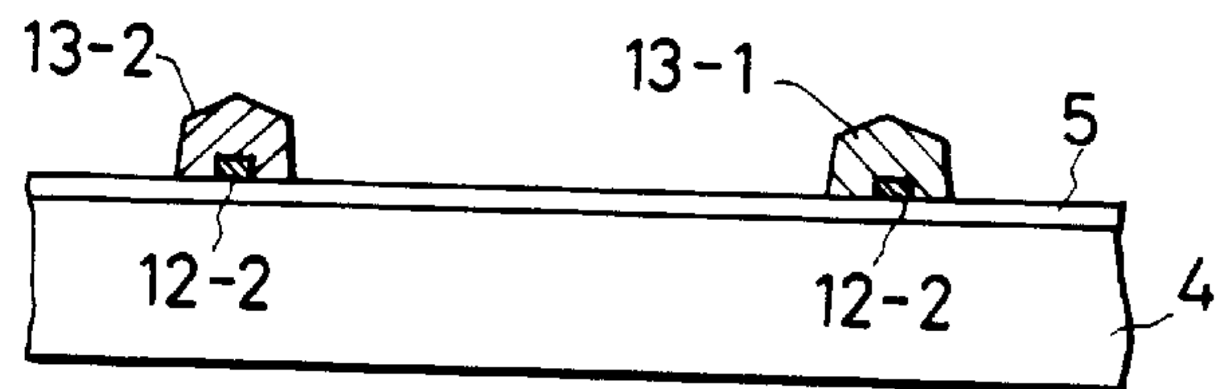
FIG. 9B
