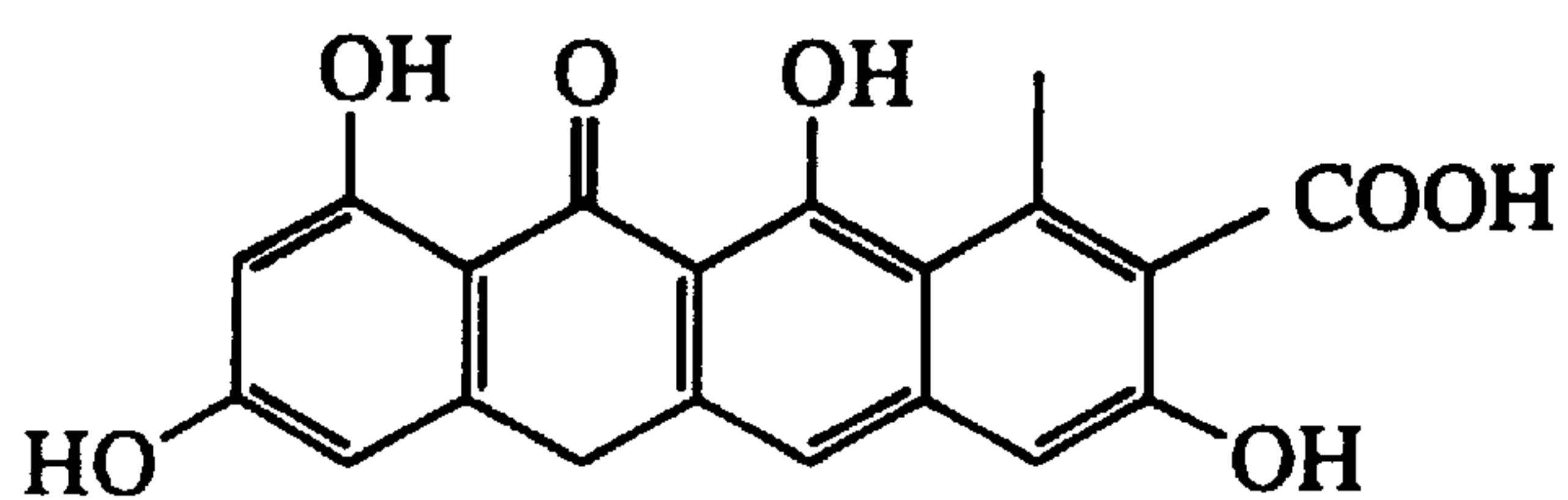
TETRACENOMYCIN F1 (5)
