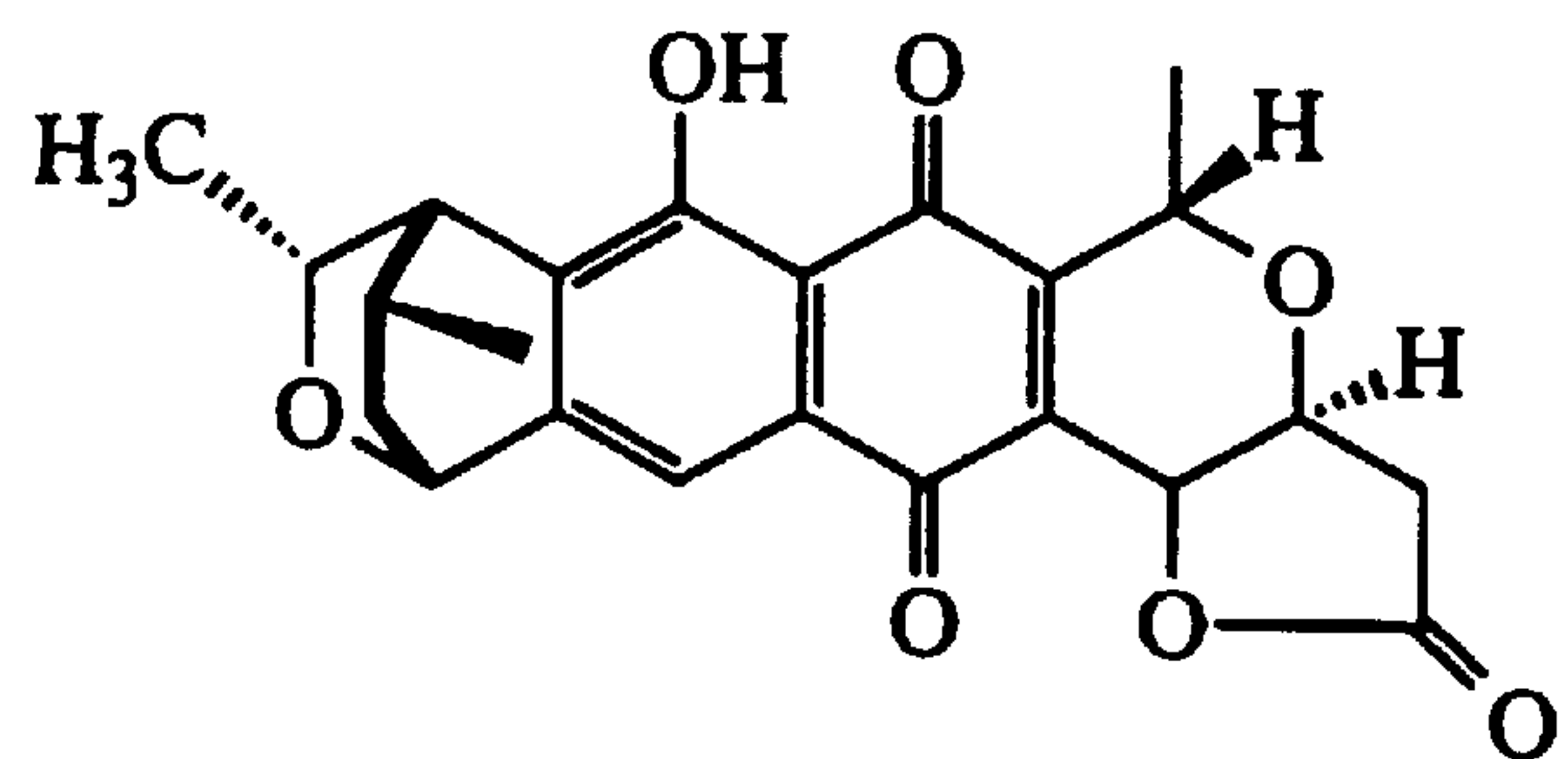
GRANATICIN (4)
