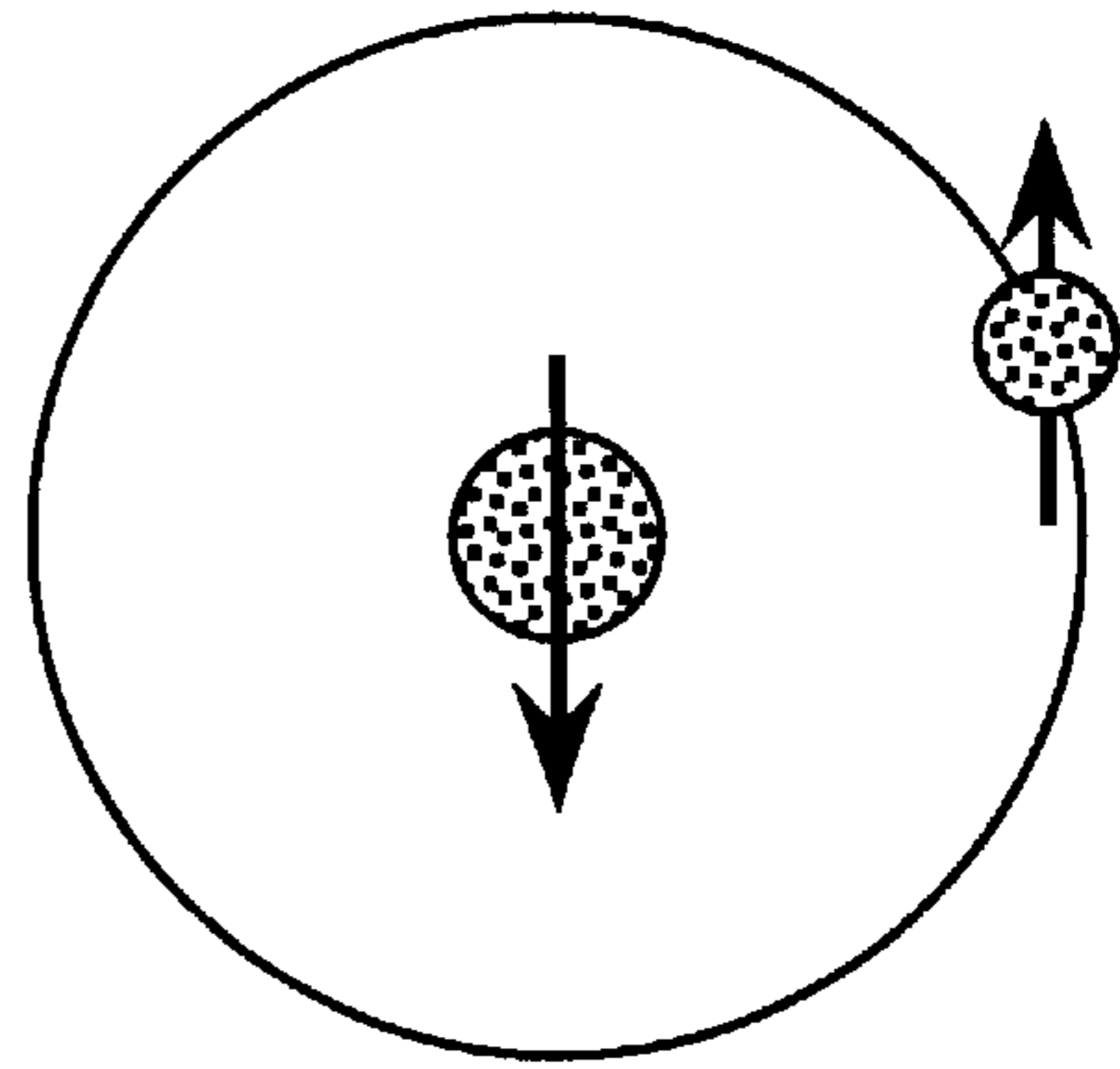
|+ -\rangle FIG. 10(b)
