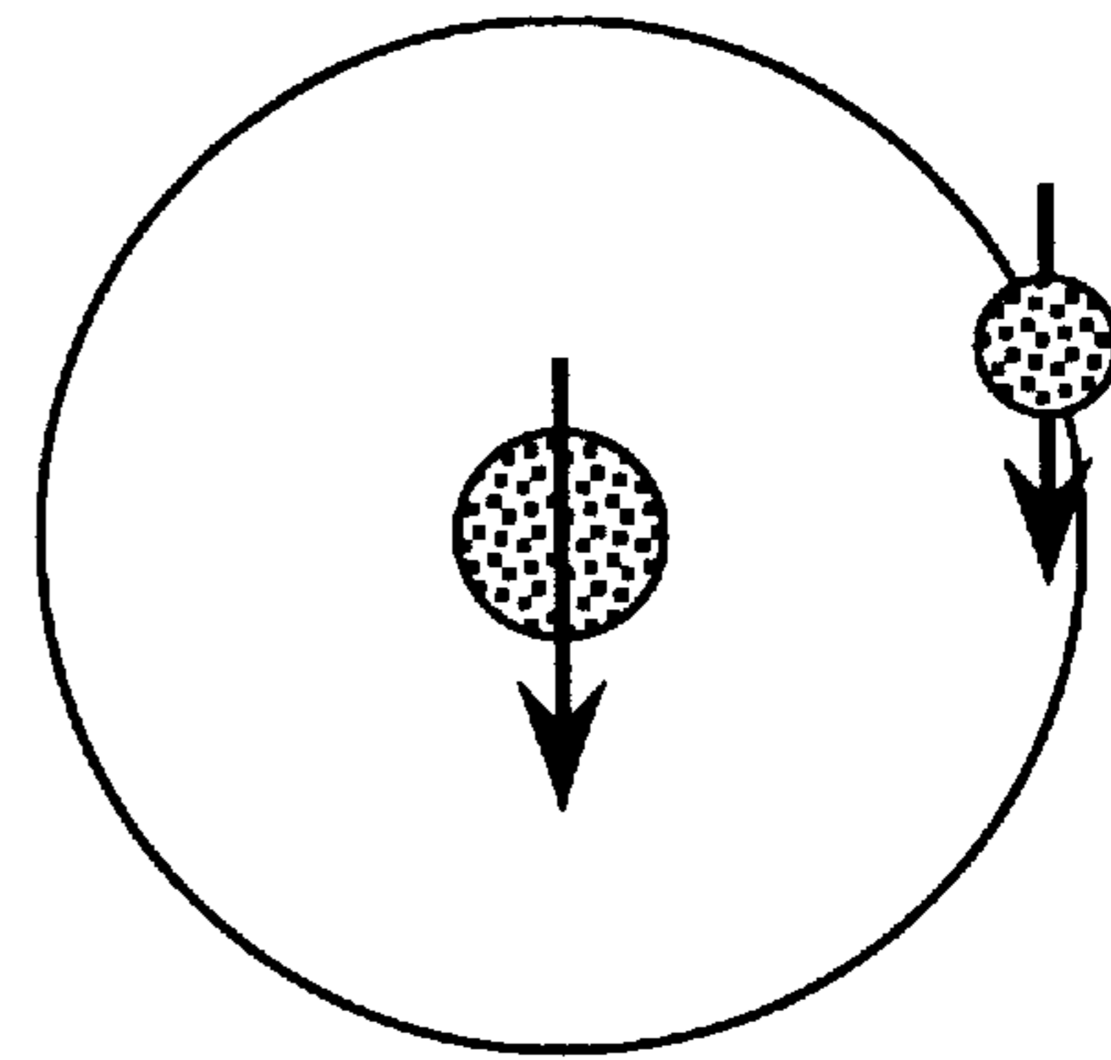
| - -\rangle FIG. 10(d)
