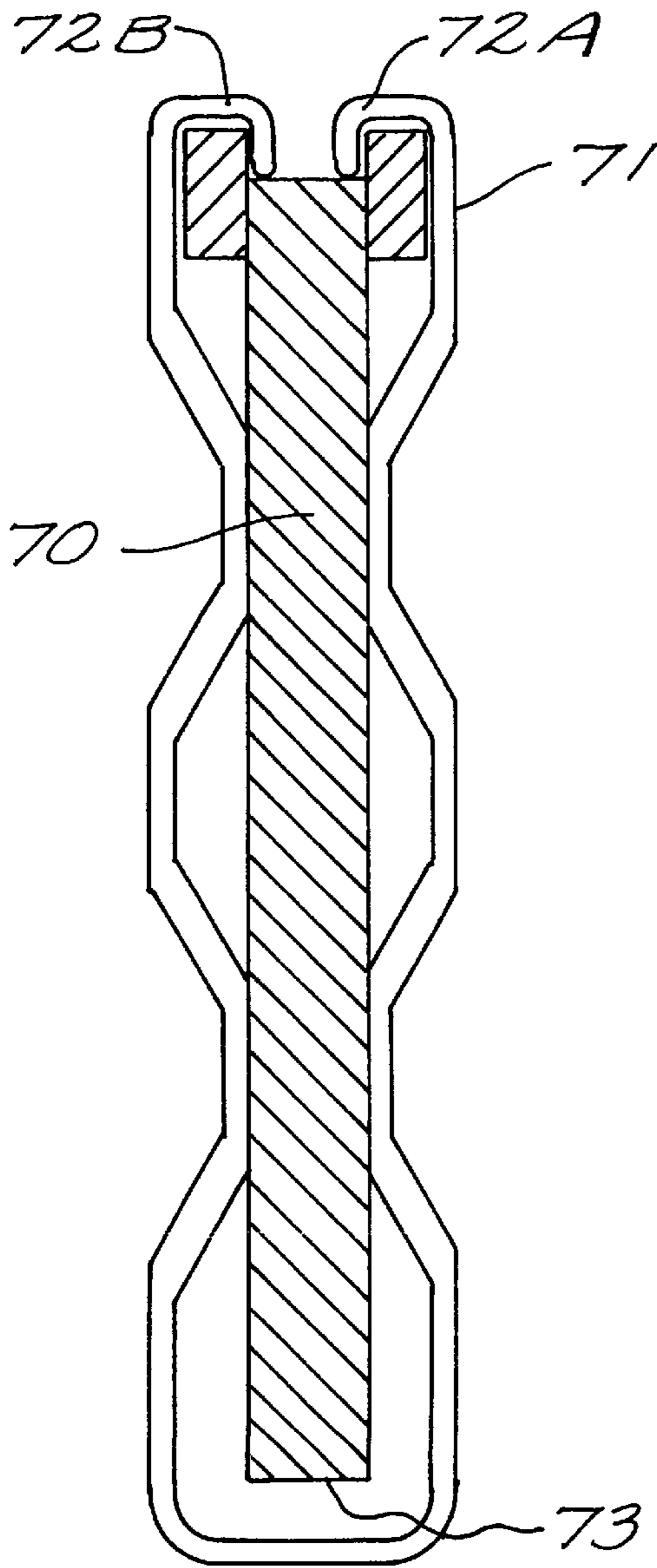
FIG. 7A
