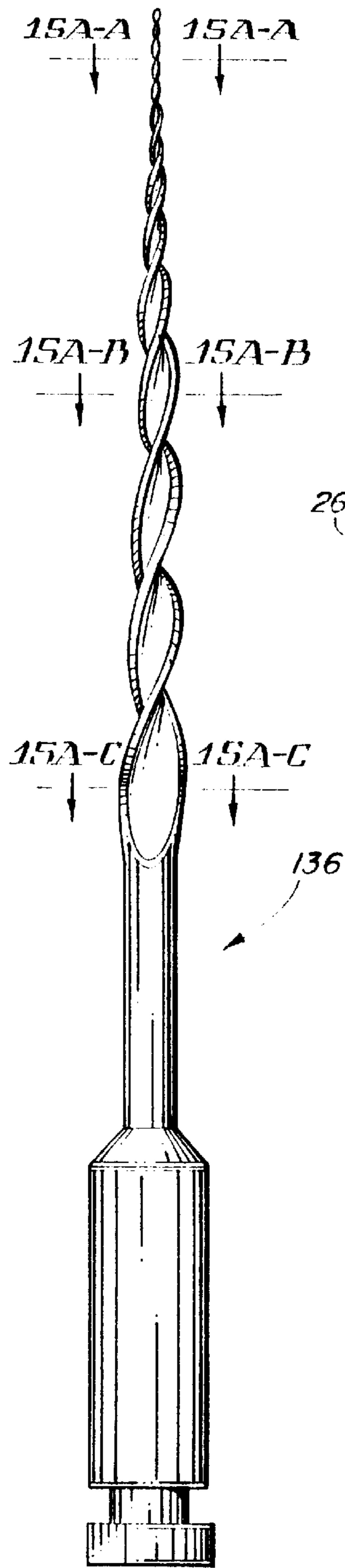
FIG. 15A
