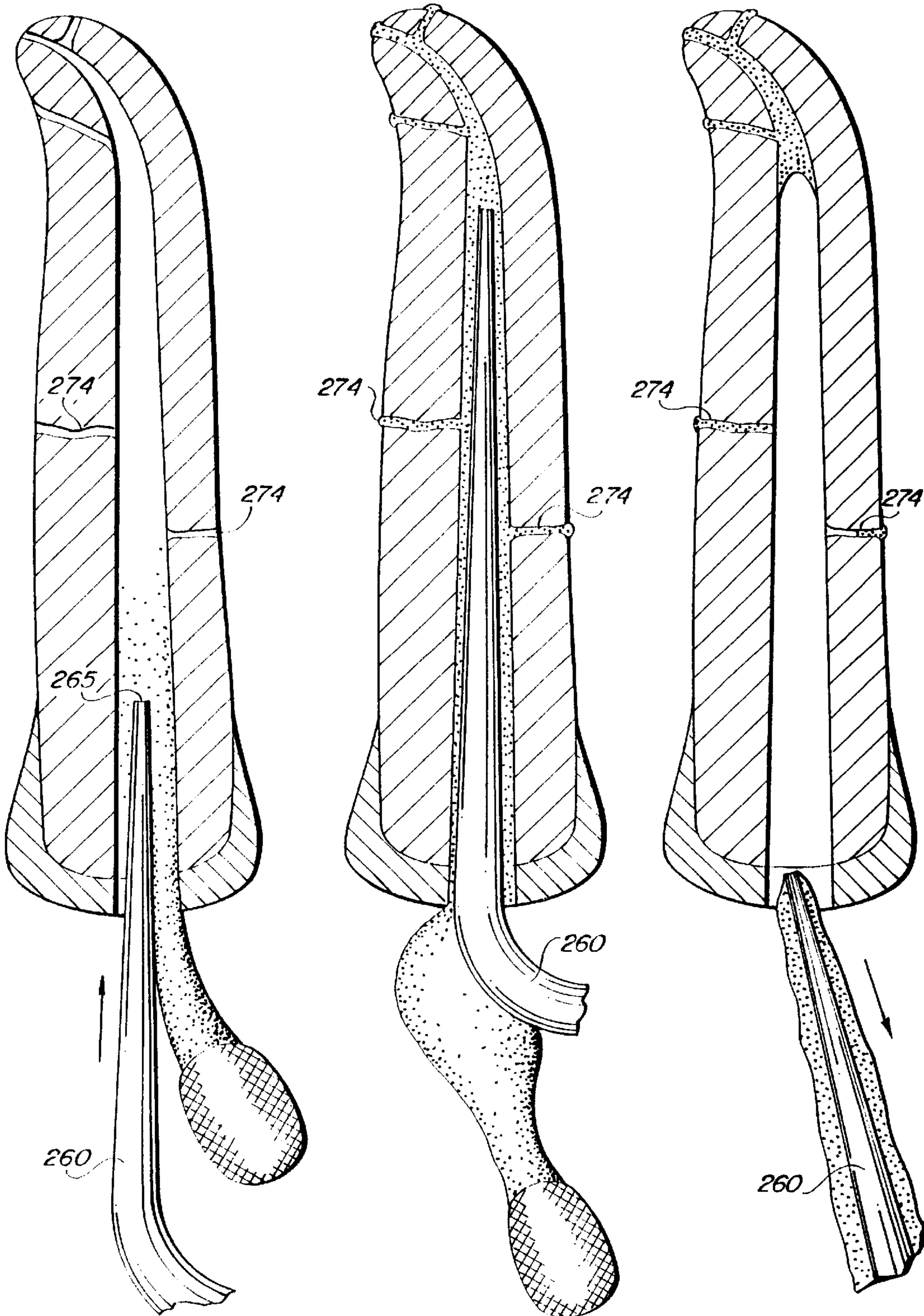
FIG. 19A
