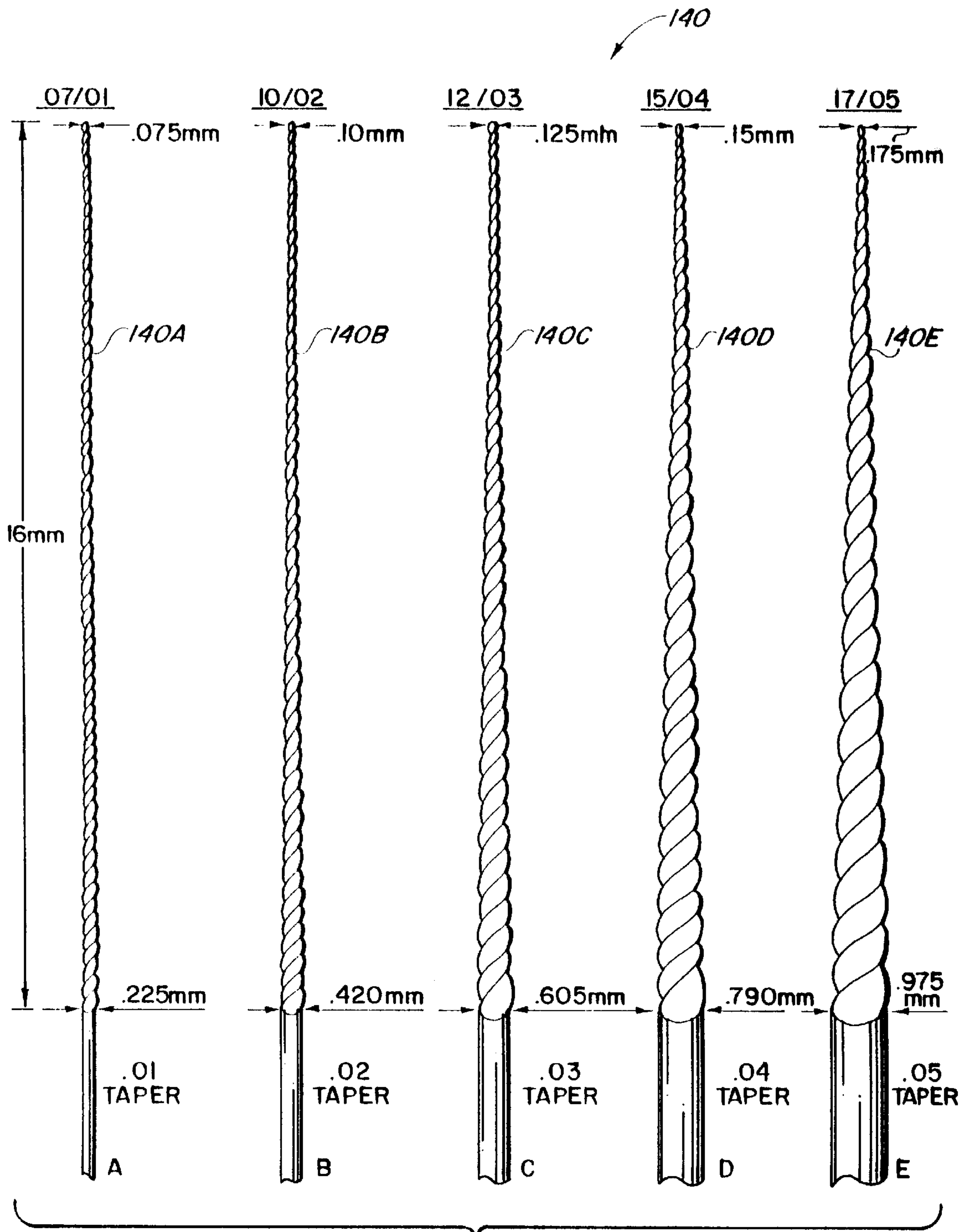
FIG. 15B
