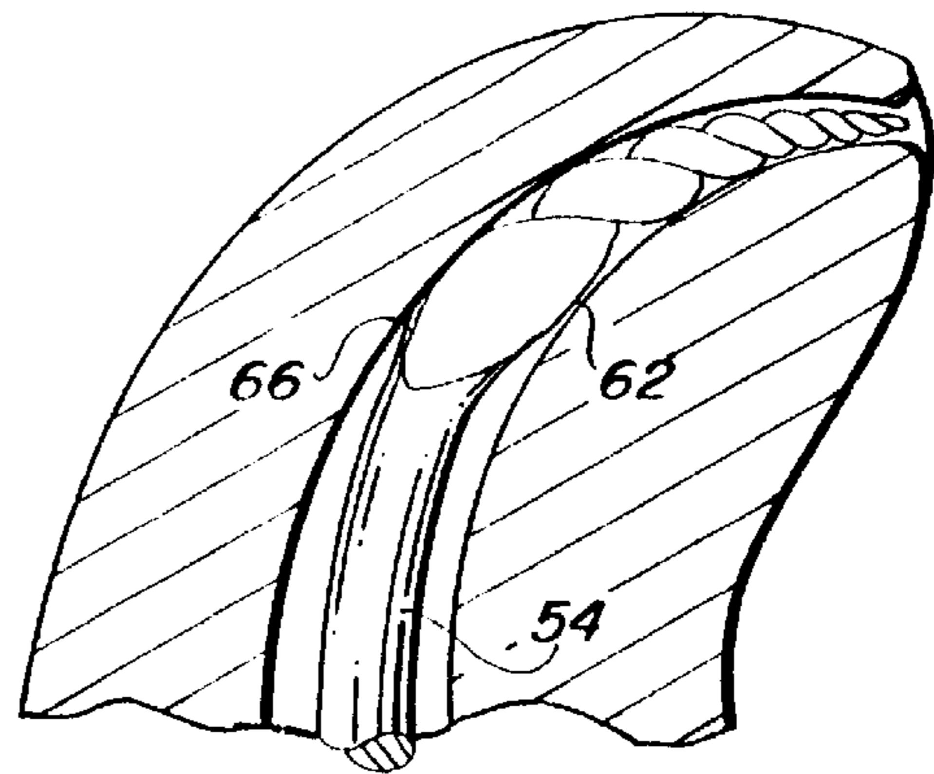
FIG. 6B
