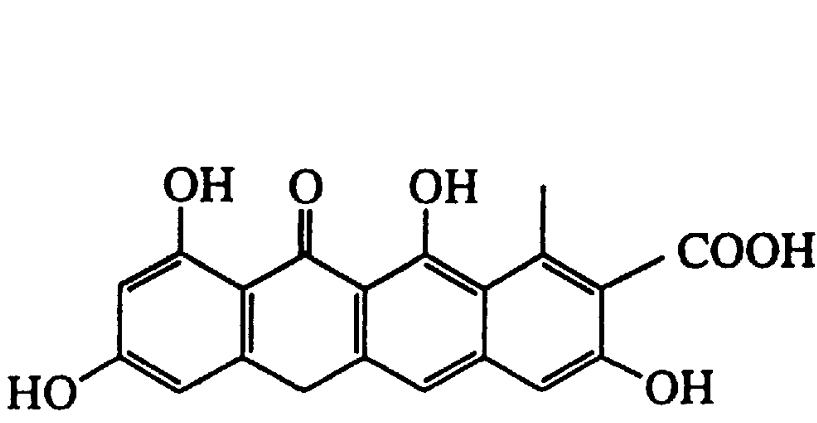
TETRACENOMYCIN F1 (5)
