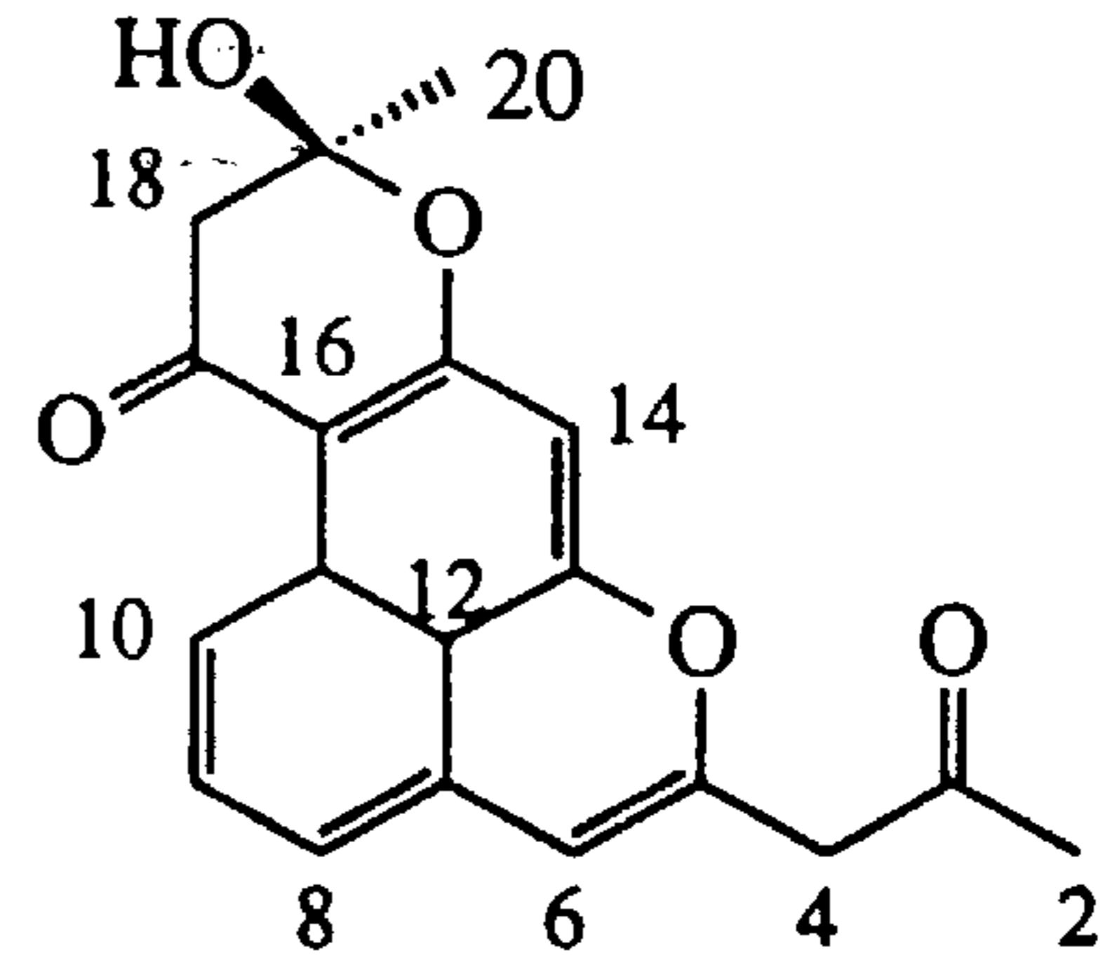
RM 20 (9)
