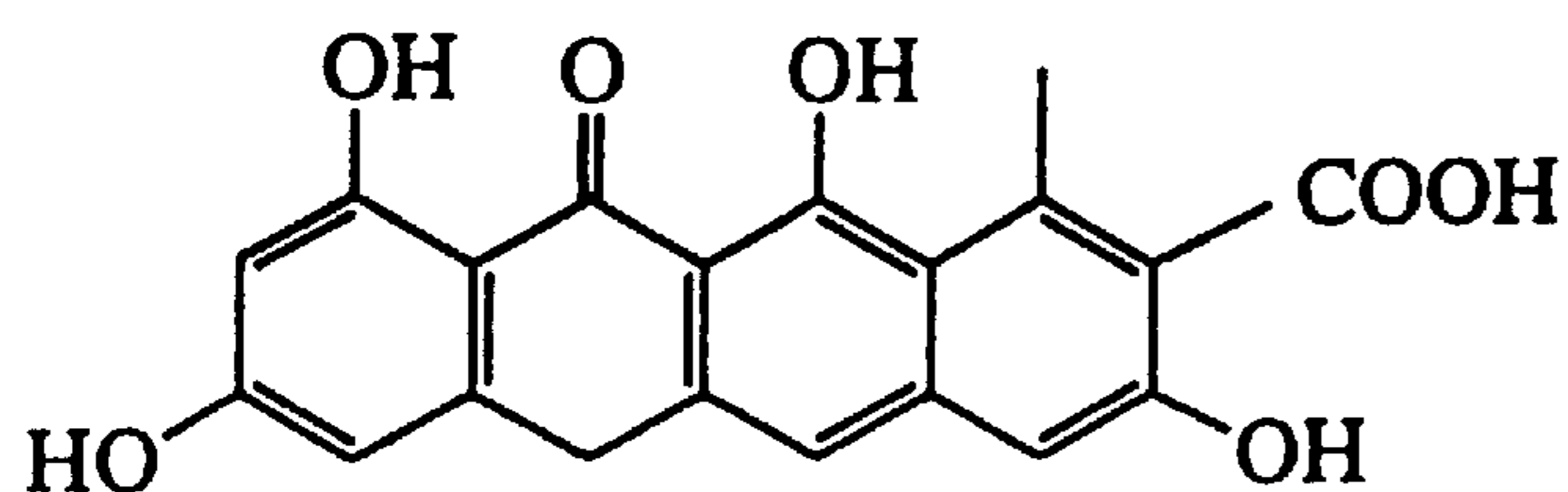
TETRACENOMYCIN F1 (5)
