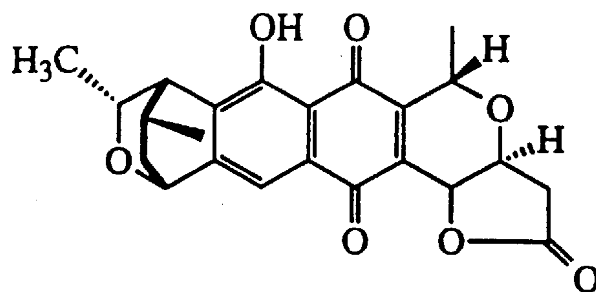
GRANATICIN (4)
