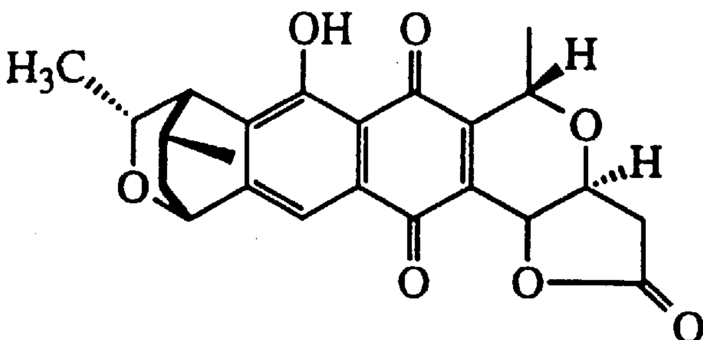
GRANATICIN (4)
