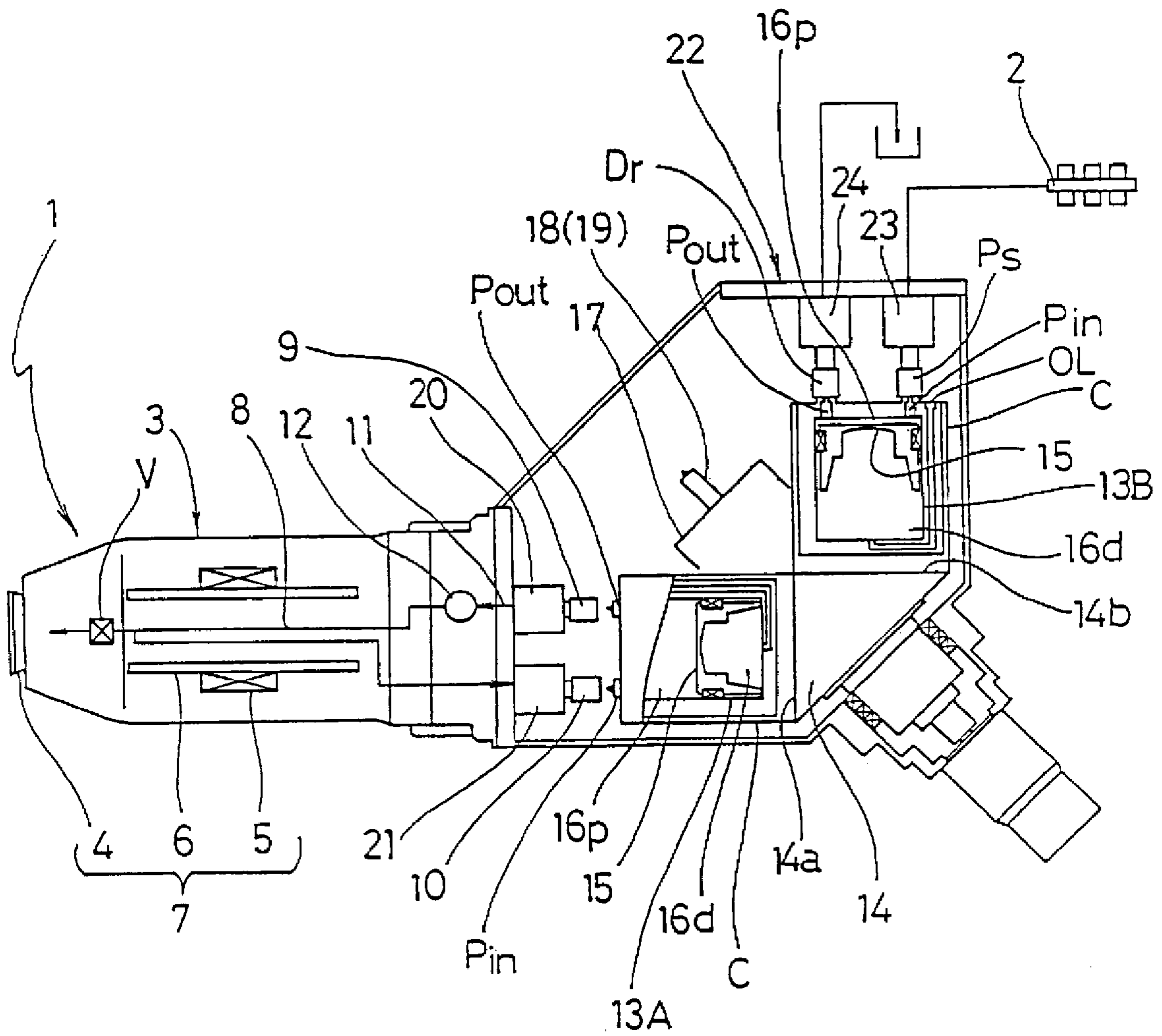
FIG. 1
