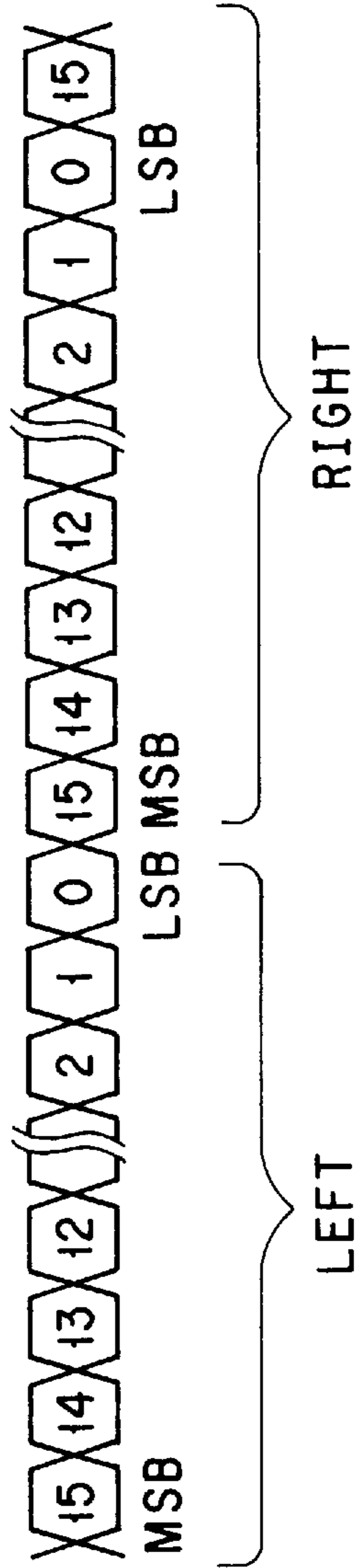
FIG. 5C sdata
