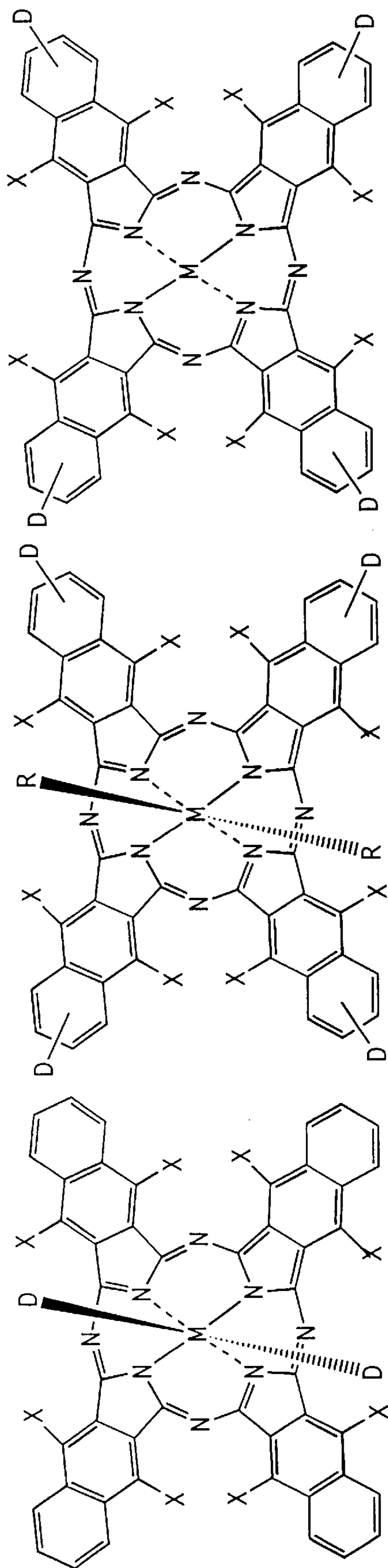
FIG. 7.
