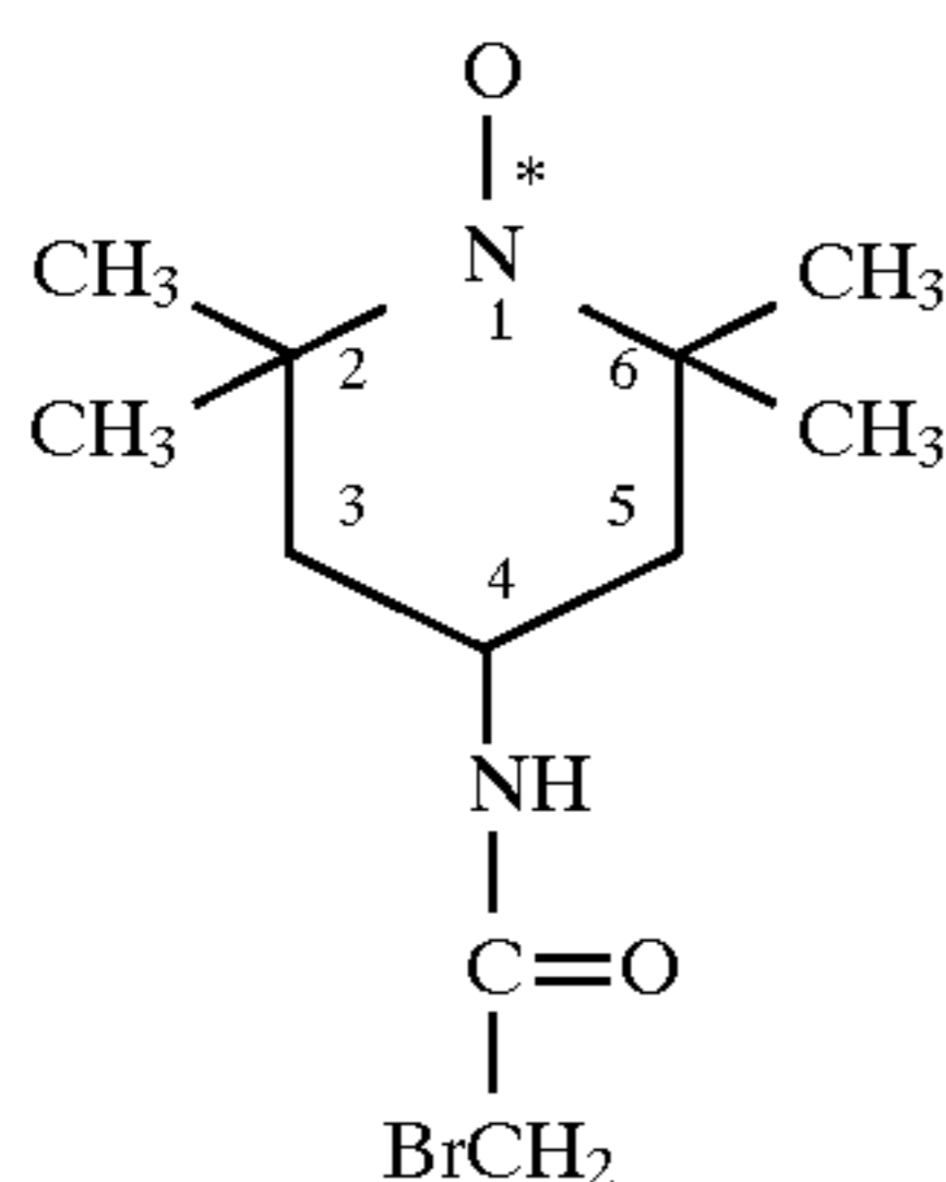
4-(2-Bromoacetamido)-TEMPO
